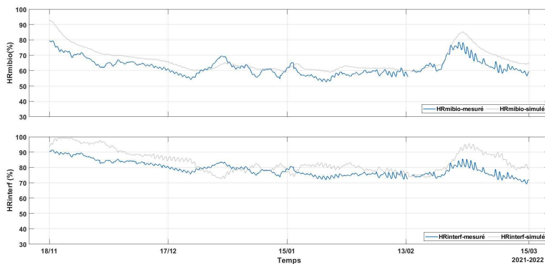
Figure 131 - Comparaison des résultats d'humidité relative mesurés et simulés pour les plaques en LTCH au R+2.
