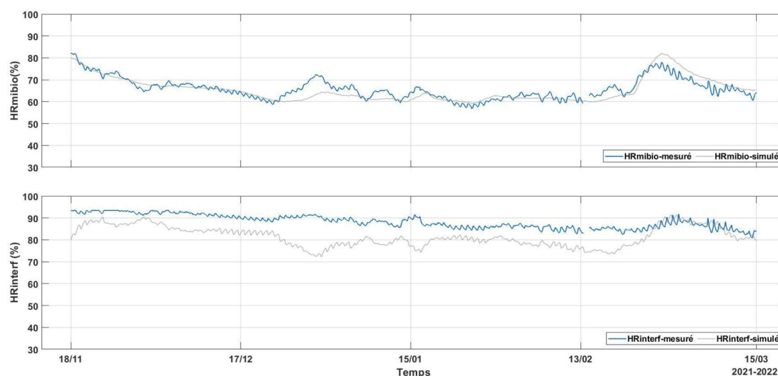
Figure 129 - Comparaison des résultats d'humidité relative mesurés et simulés pour les plaques en CHMK au R+2.
