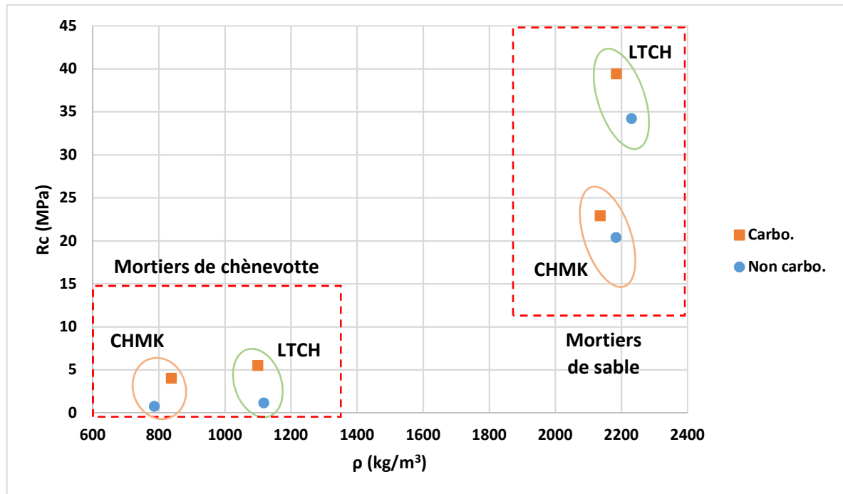
Figure 30 - Résistance en compression des mortiers de sable et de chènevotte en fonction de la masse volumique et selon le type de cure appliqué (carbonatation accélérée ou pas).
