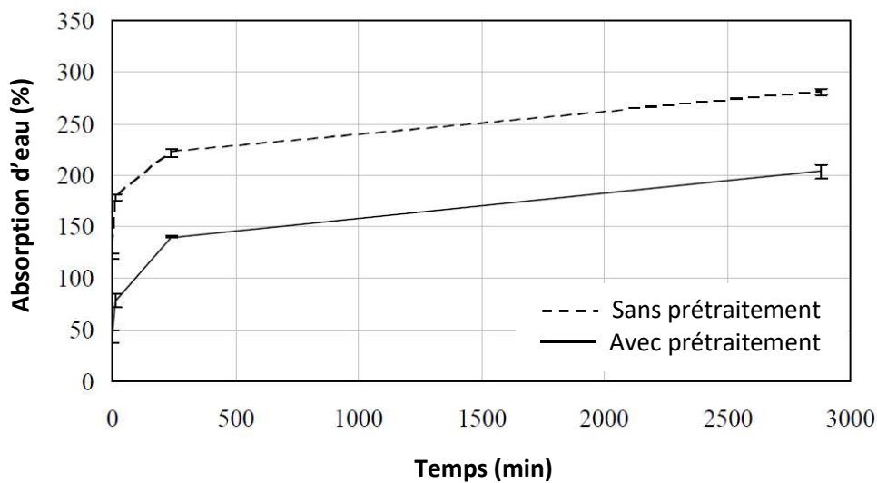
Figure 10 - Absorption d'eau des granulats de chanvre (avec et sans prétraitement) en fonction du temps (The Manh, 2014).
