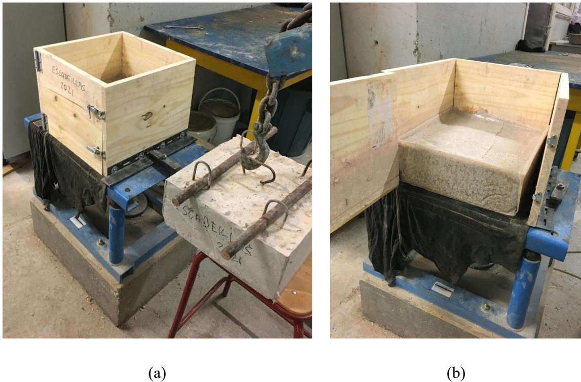
Figure 35 - Production des plaques préfabriquées en béton de chanvre.
