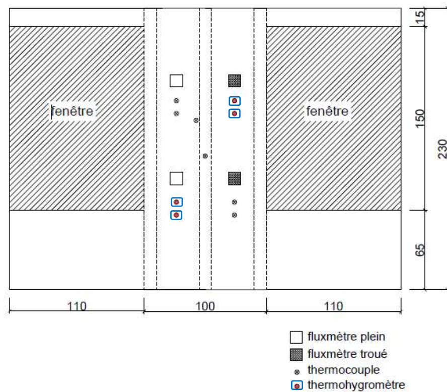
Figure 74 - Vue du côté intérieur de la paroi étudiée - configuration en polystyrène et plâtre.
