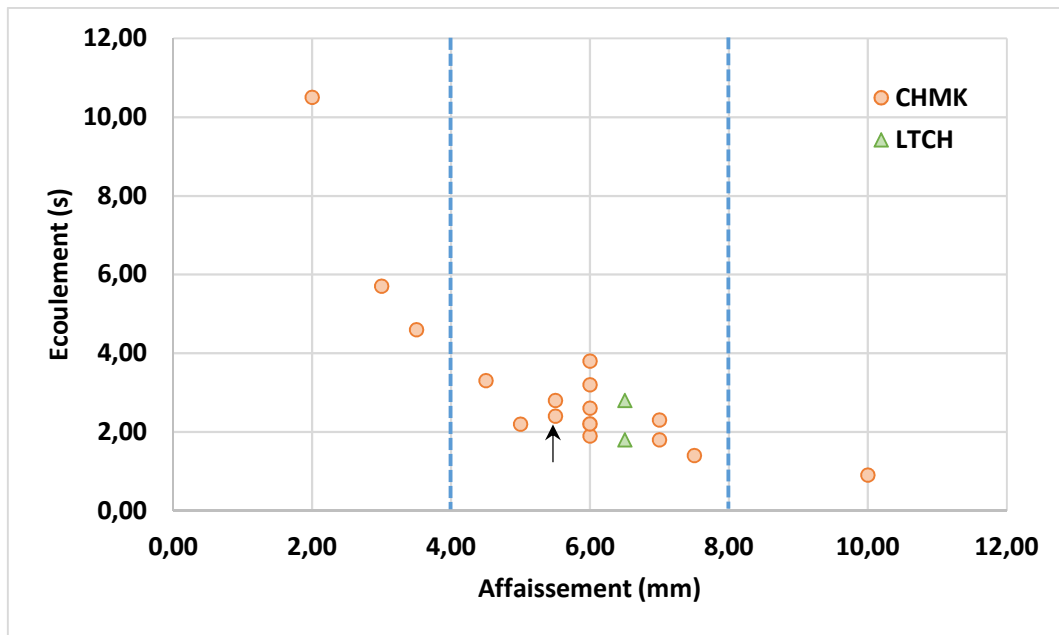
Figure 25 - Ecoulement et affaissement des mortiers de sable étudiés. La flèche indique l'adjuvant retenu et les lignes en pointillés la plage d'affaissement visée.
