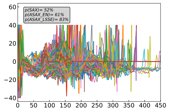
(d) GesturePebbleZ1
