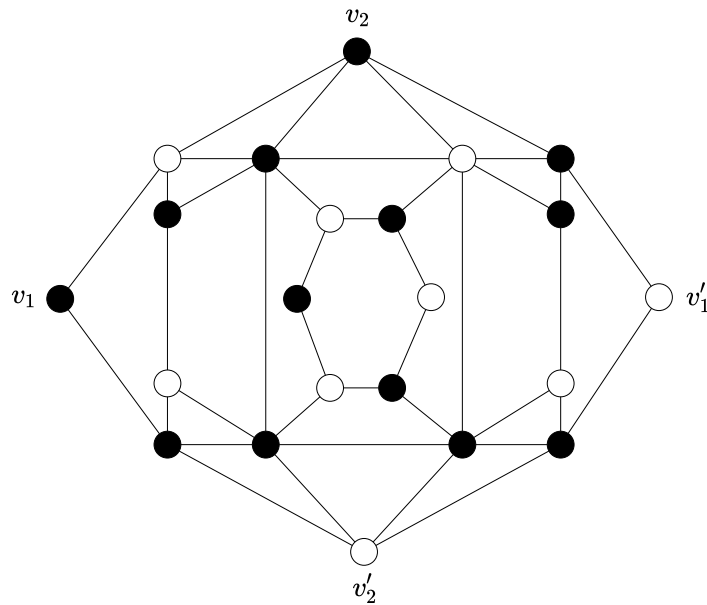
FIGURE 4.2 – Le graphe planaire H où les sommets noirs forment une couverture des sommets minimaux de H .
