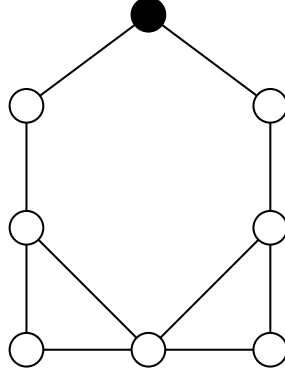
FIGURE 3.4 – Un graphe G sans trou impair et sans (K_{1,3}, K_4, \text{net}, \text{diamant}) . Le sommet noir est dans \text{core}(G) \cap V^0 et \gamma(G) = 2 .
