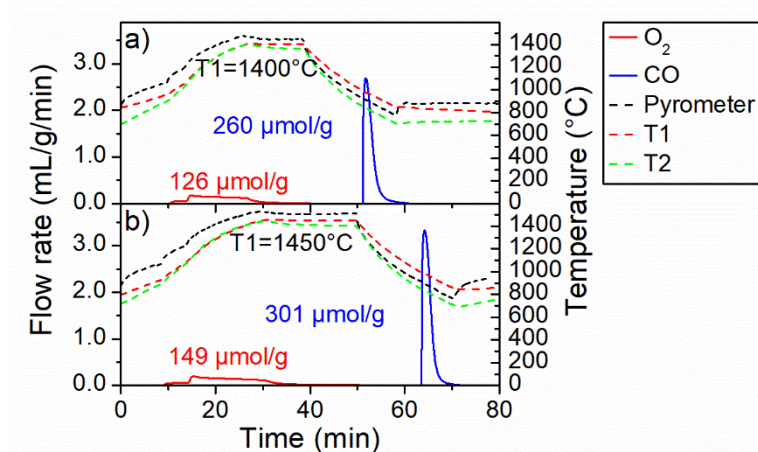
Figure SF-7: Evolution des vitesses de production de O_2 et CO associées à la température pour deux cycles thermochimiques avec une température de réduction de a) 1400\text{ }^\circ\text{C} et b) 1450\text{ }^\circ\text{C} sous pression atmosphérique avec une mousse en cérine (CF-20)
