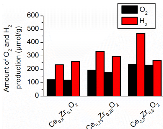
Figure SF-2 : Quantités de O 2 et H 2 produites durant deux cycles thermochimiques utilisant de la poudre Ce 1-x Zr x O 2 (x=0.1, 0.25 et 0.5) avec des température de réduction et d'oxydation de 1400 °C et 1050 °C respectivement [93]
