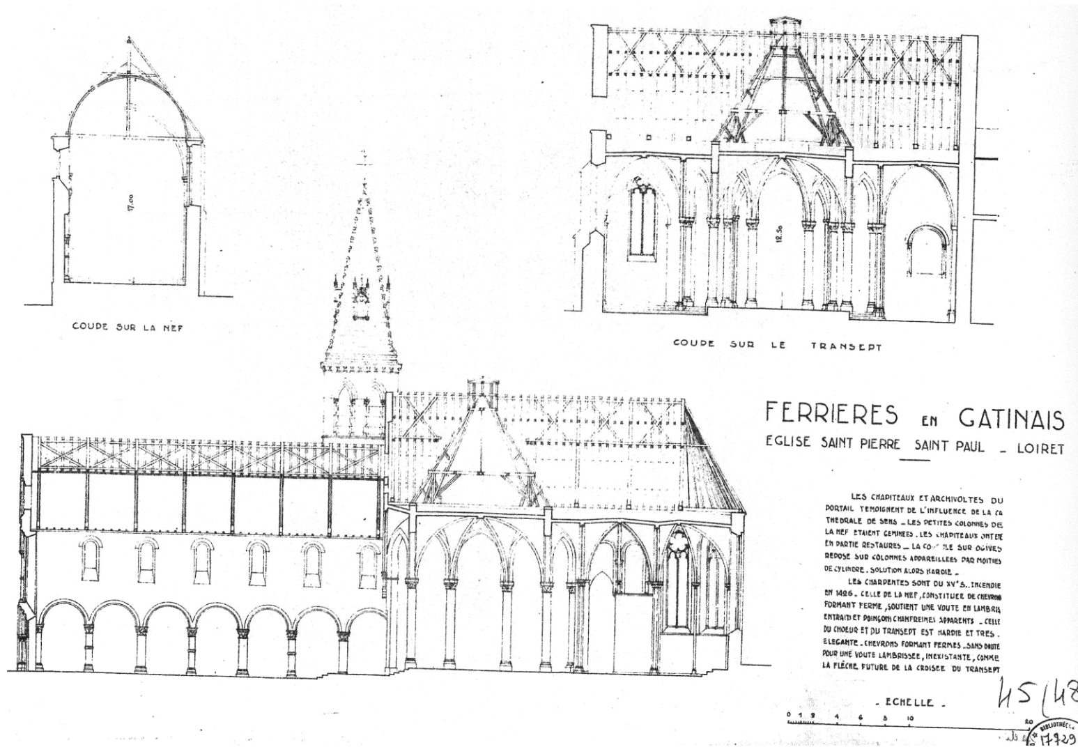
Fig. 5 : Coupes sur l'église par Frottier en 1944.
