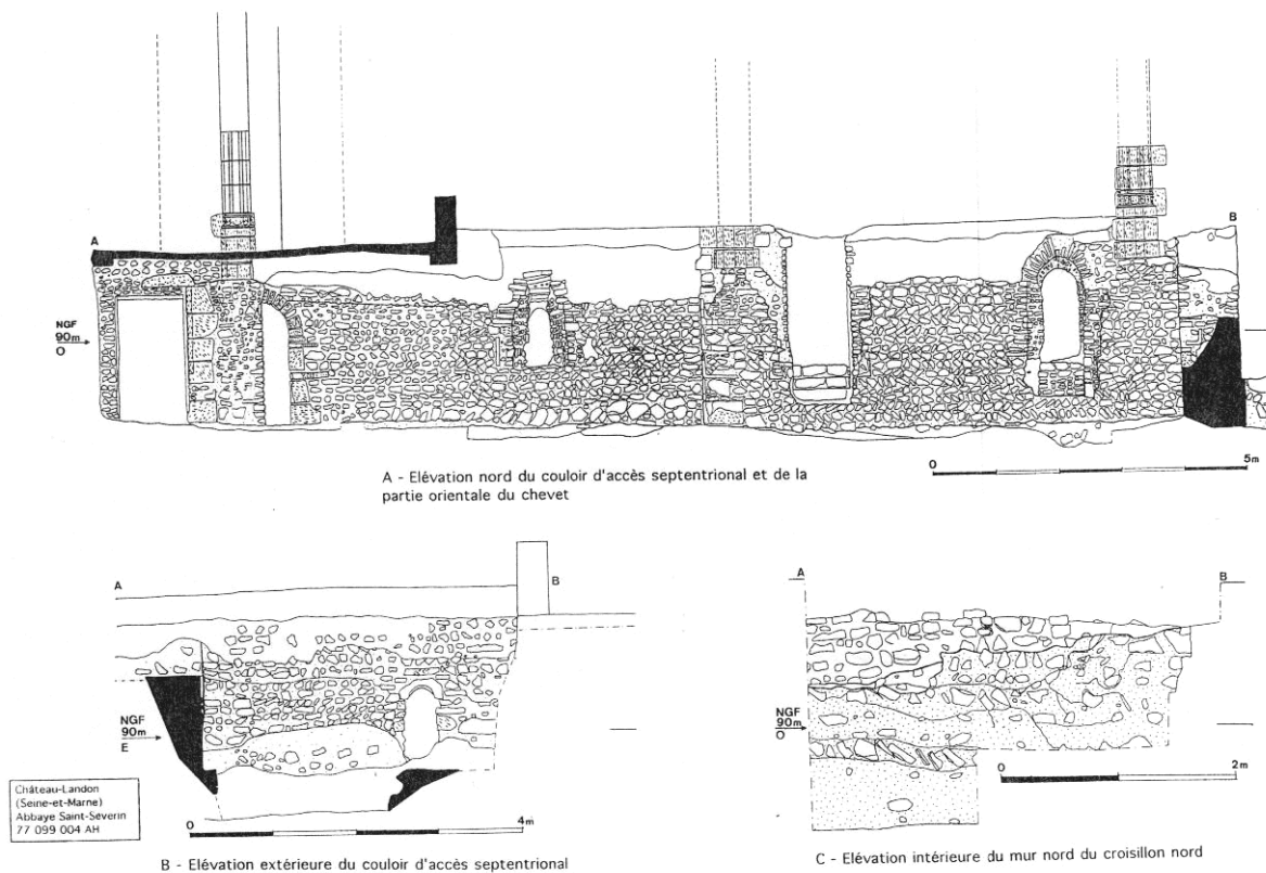
Fig. 24 : Relevés des élévations du couloir d'accès nord de la crypte.
