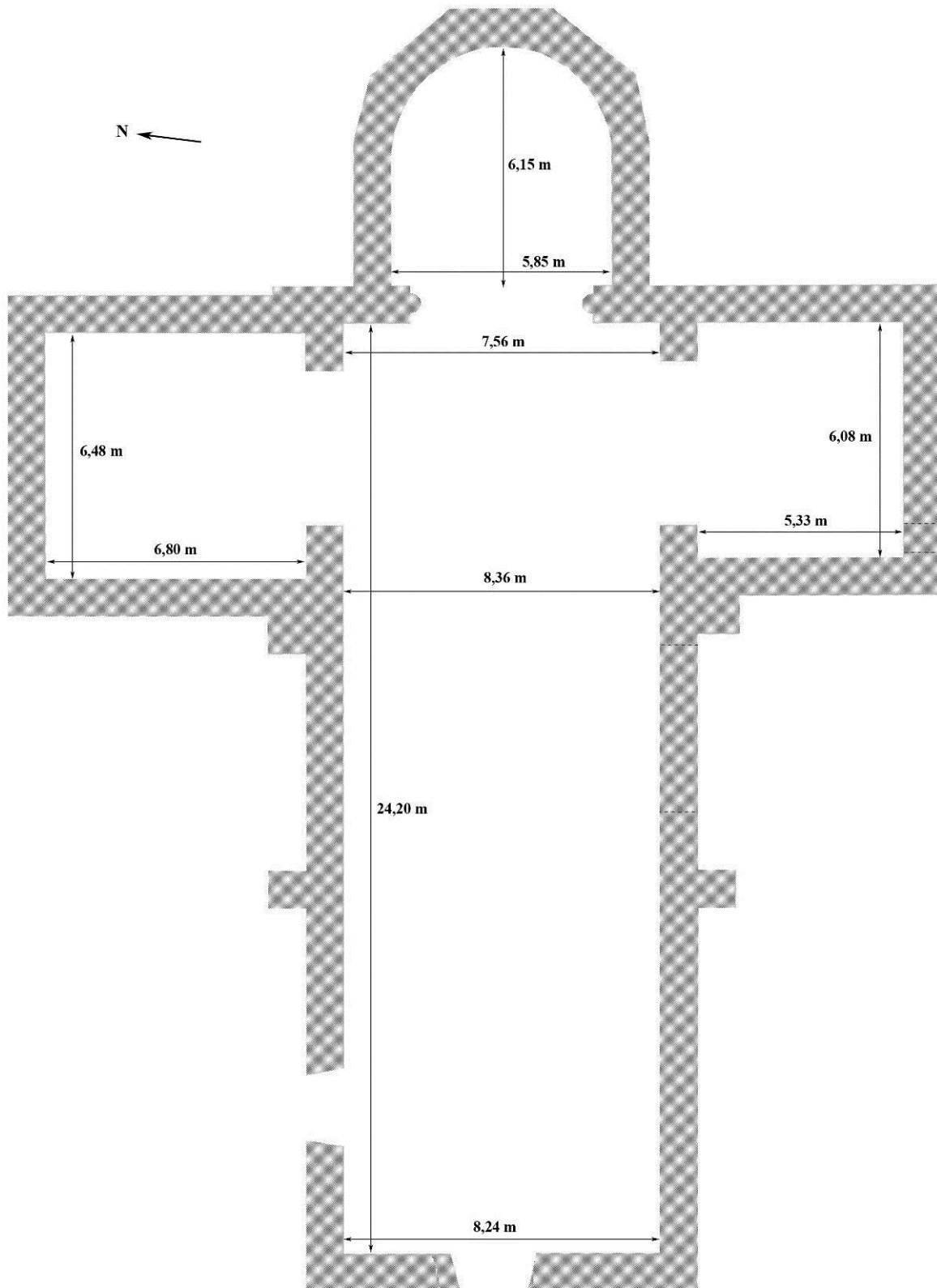
Fig. 8 : Plan schématique de l'église.
