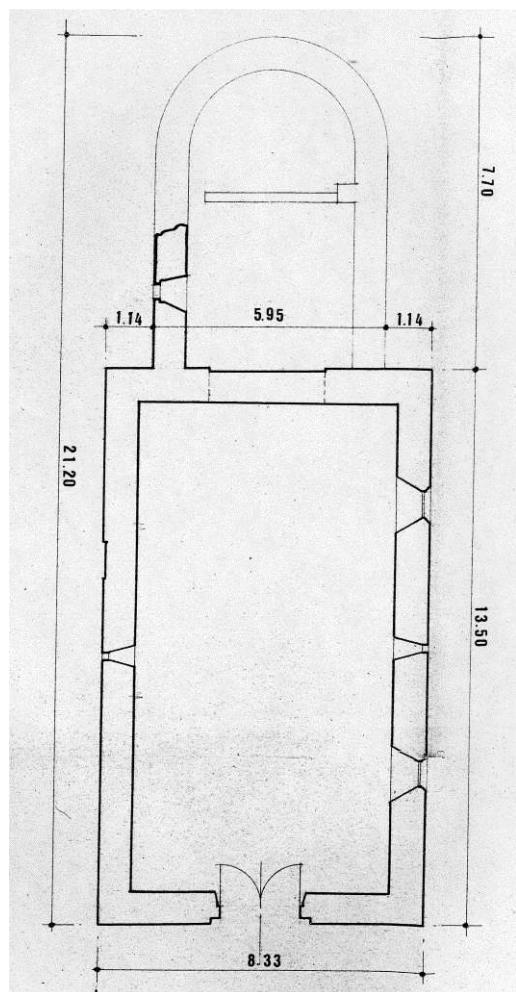
Fig. 5 : Plan de l'église par l'architecte de Boitel.
