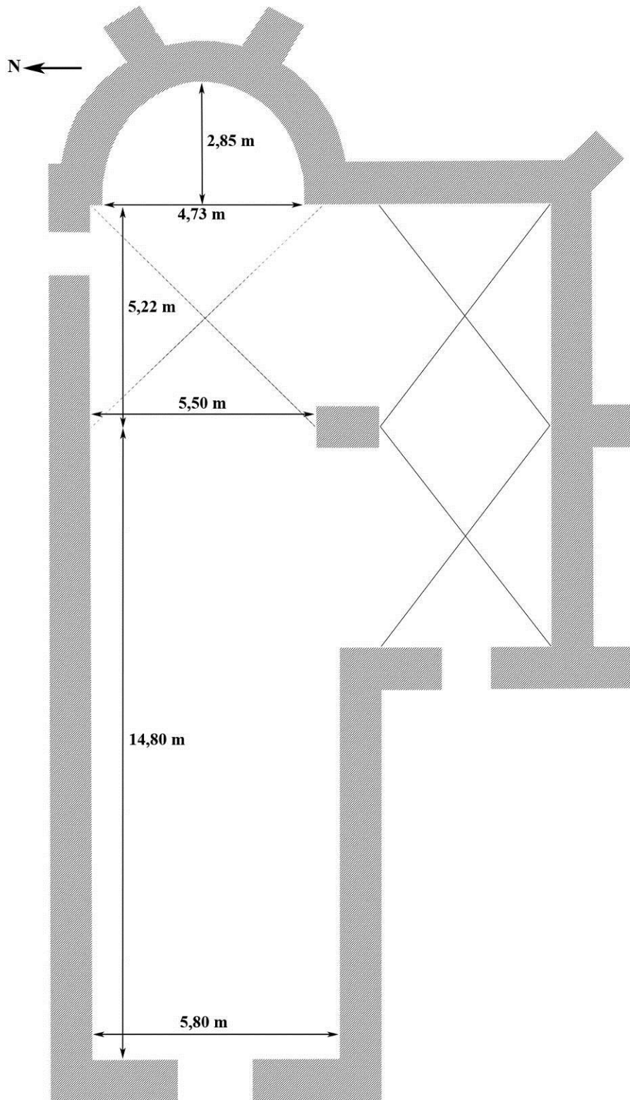
Fig. 4 : Plan schématique de l'église.
