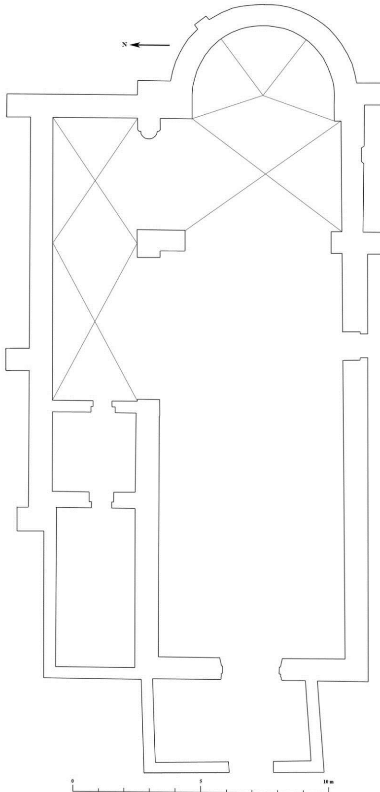
Fig. 4 : Plan de l'église de Chevry-sous-le-Bignon.
