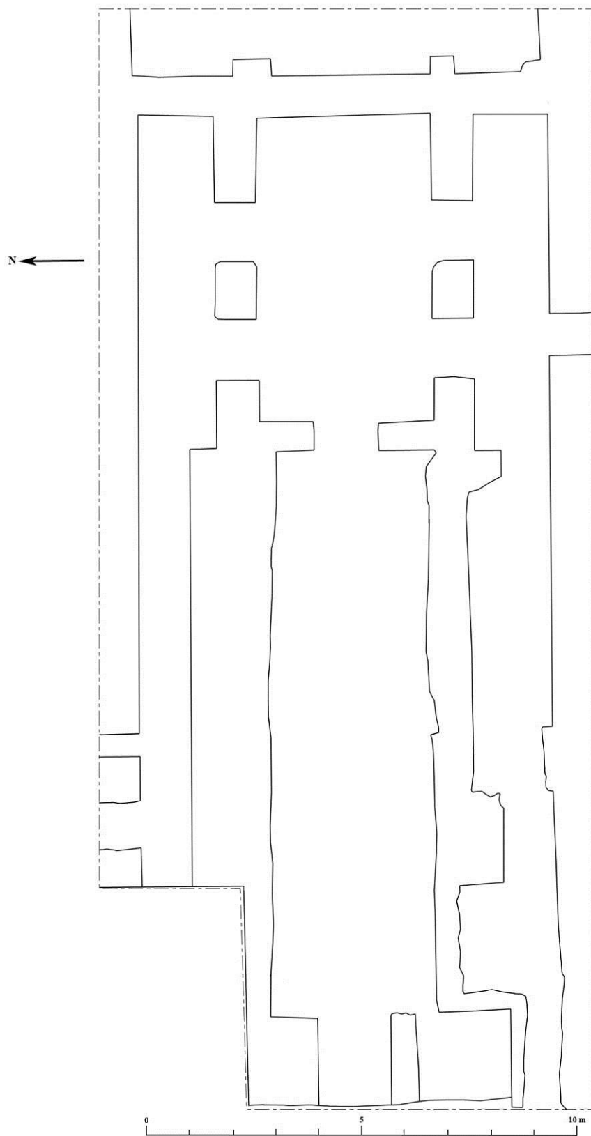
Fig. 15 : Plan de la crypte de Saint-Séverin de Château-Landon.
