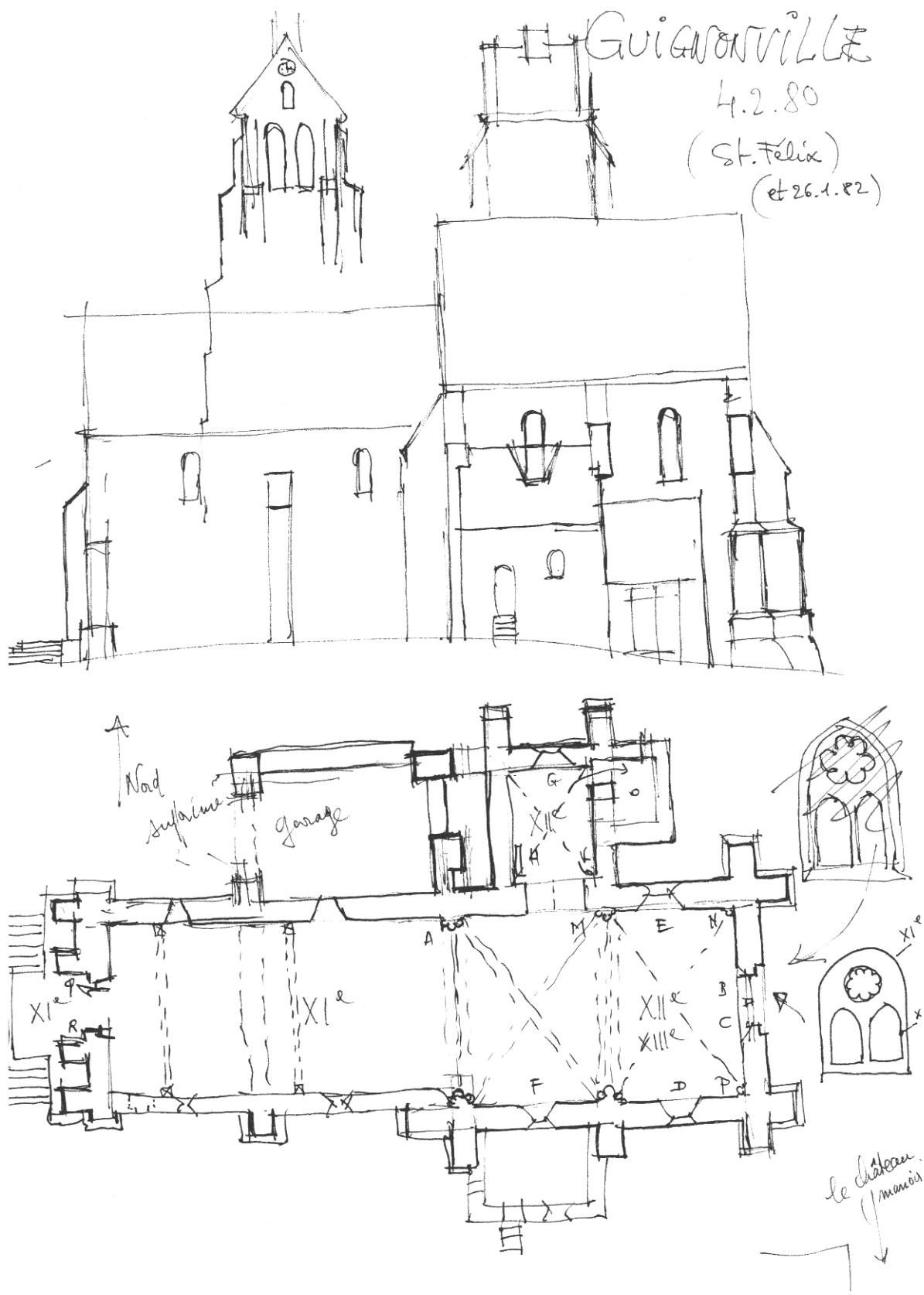
Fig. 5 : Croquis de l'église par un architecte des Bâtiments de France en 1980. In : Guignonville : dossier travaux (Orléans – Service départemental de l'architecture et du patrimoine – Dossier de la commune de Guignonville).
