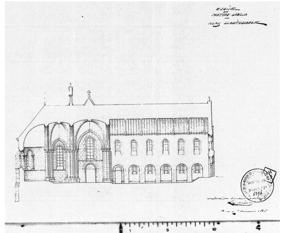
Fig. 9 : Coupe longitudinale de l'église, par Millet, en 1863 (projet ?). Millet E., Coupe longitudinale , s. é., 1863, Médiathèque de l'architecture et du patrimoine, 0082/077/2007 (Série 0082/077 : Plans d'édifices de la Seine-et-Marne).
