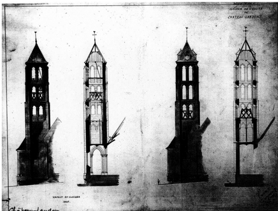
Fig. 15 : Coupes et élévations sur le clocher, avant et après restauration.
