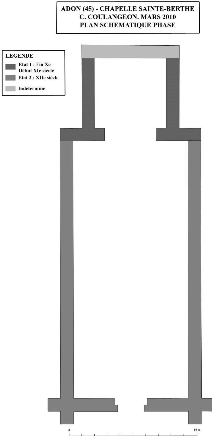
Fig. 6 : Plan schématique phasé de la chapelle Sainte-Berthe à Adon.
