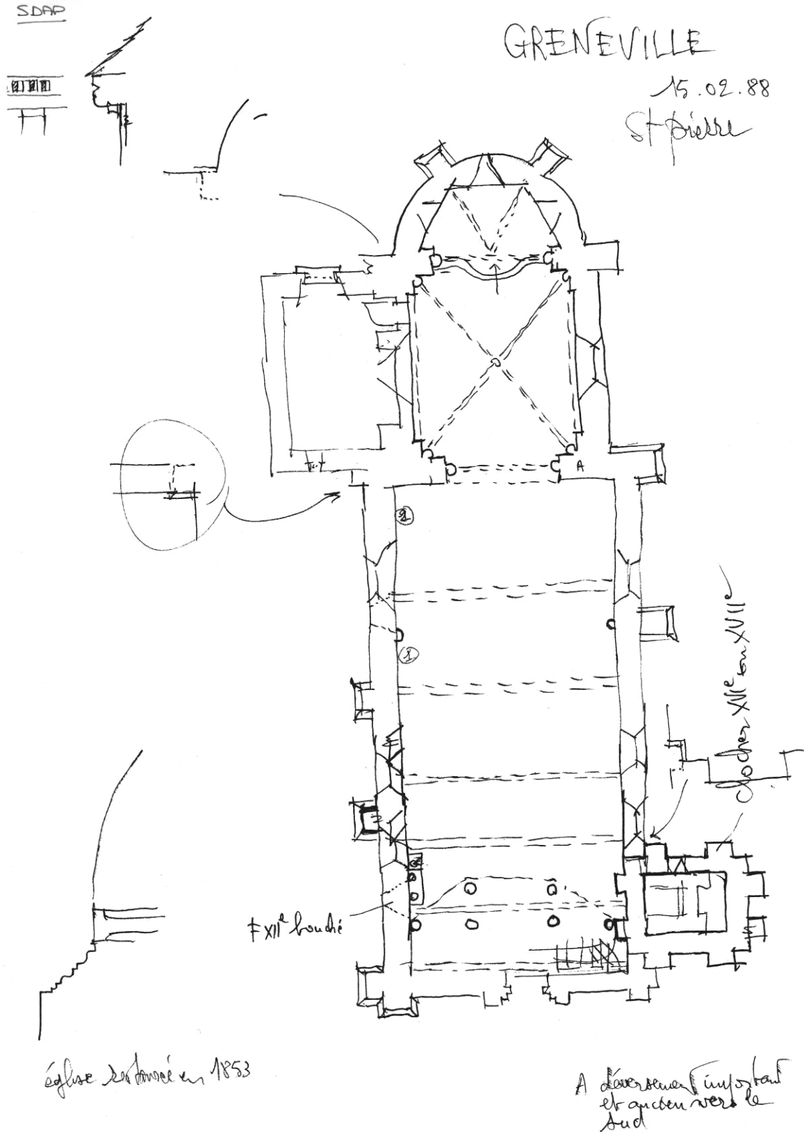
Fig. 5 : Croquis schématique de l'église.
