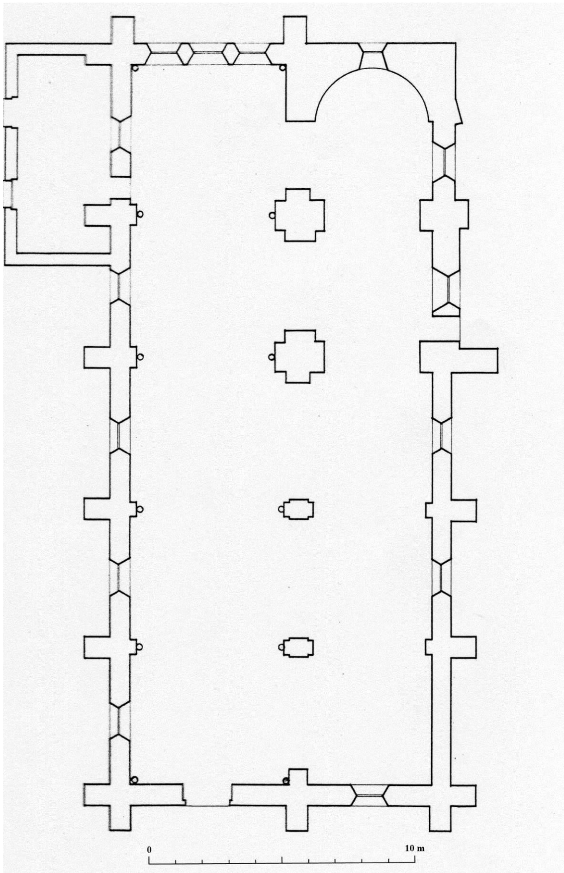
Fig. 5 : Plan de l'église, non daté. Commune d'Escrennes. L'église, plan, s. é., s. d.
