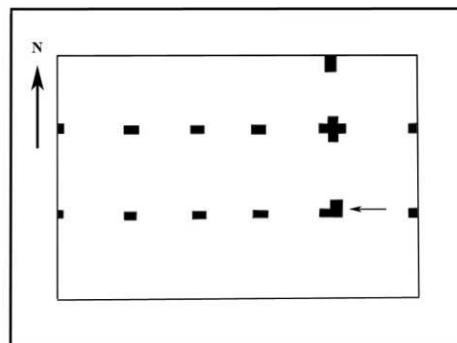
Fig. 9 : Relevé pierre à pierre de la pile sud-ouest du chœur.
