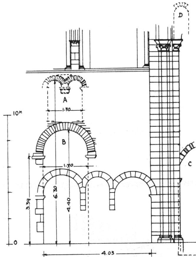
Fig. 14 : Relevé des traces de baies dans le mur sud du chevet par Rousseau.
