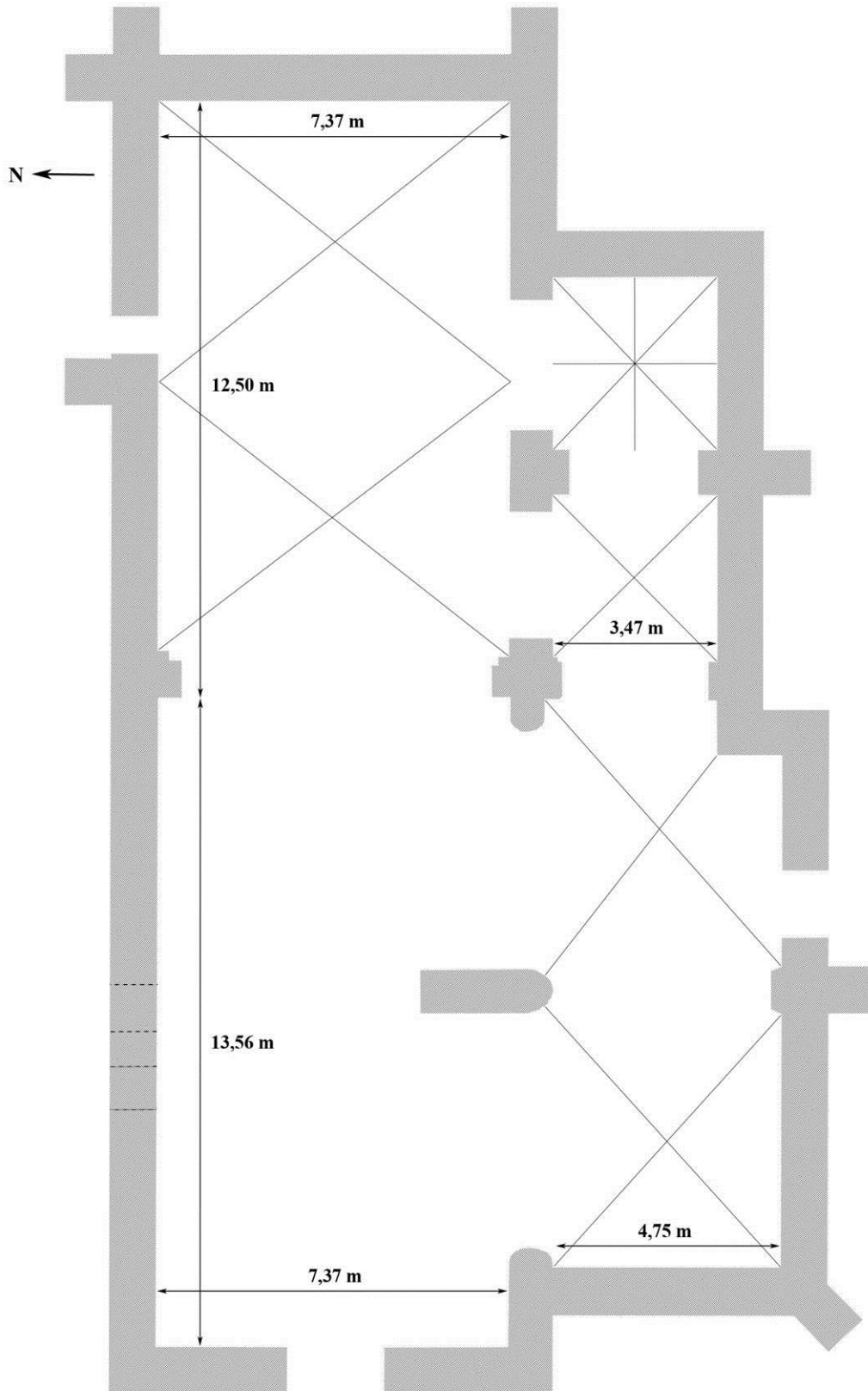
Fig. 4 : Plan schématique de l'église.
