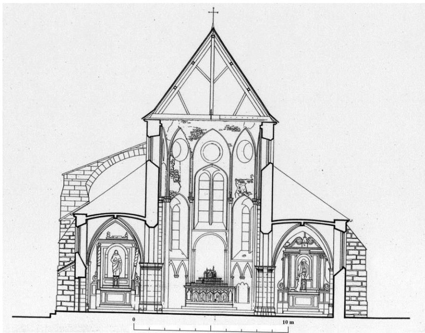
Fig. 10 : Coupe transversale.
