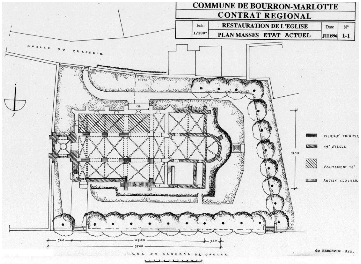
Fig. 9 : Plan de l'église de Bourron-Marlotte, en 1996. Bergevin O. de, Commune de Bourron-Marlotte. Contrat régional. Restauration de l'église, juillet 1996, Cahier de plans, fig. 1-1.
