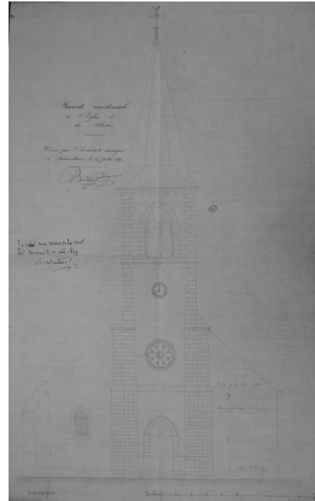
Fig. 6 : La façade ouest de l'église en 1858. Bidault M., Façade occidentale de l'église et du clocher , Échelle 0,02, 12 juillet 1859, Melun AD 77, 2 O 57 (ex 1 Fi 29/4 Op 48/1).
