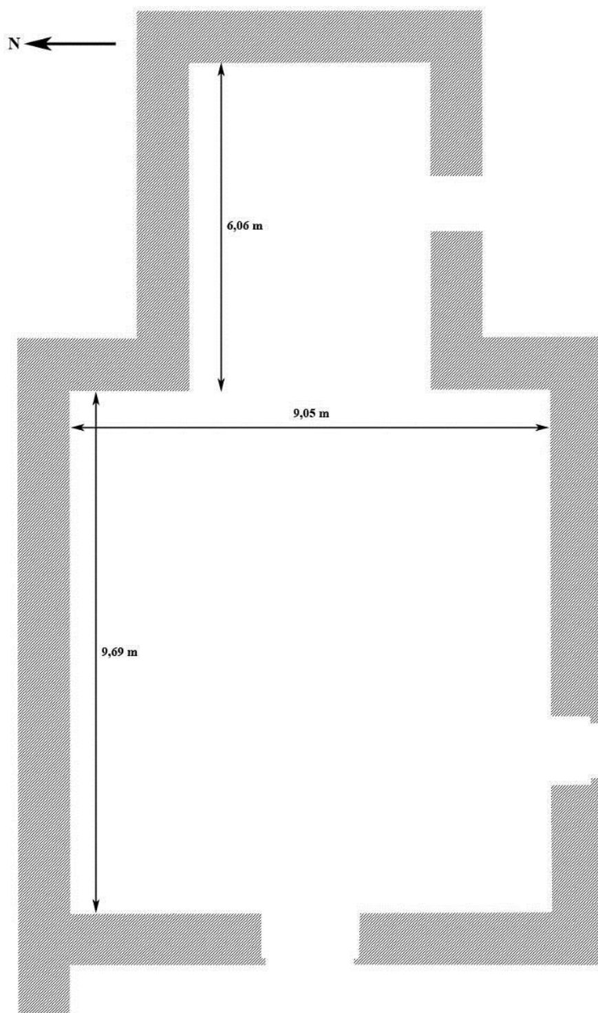
Fig. 4 : Plan schématique de l'église.
