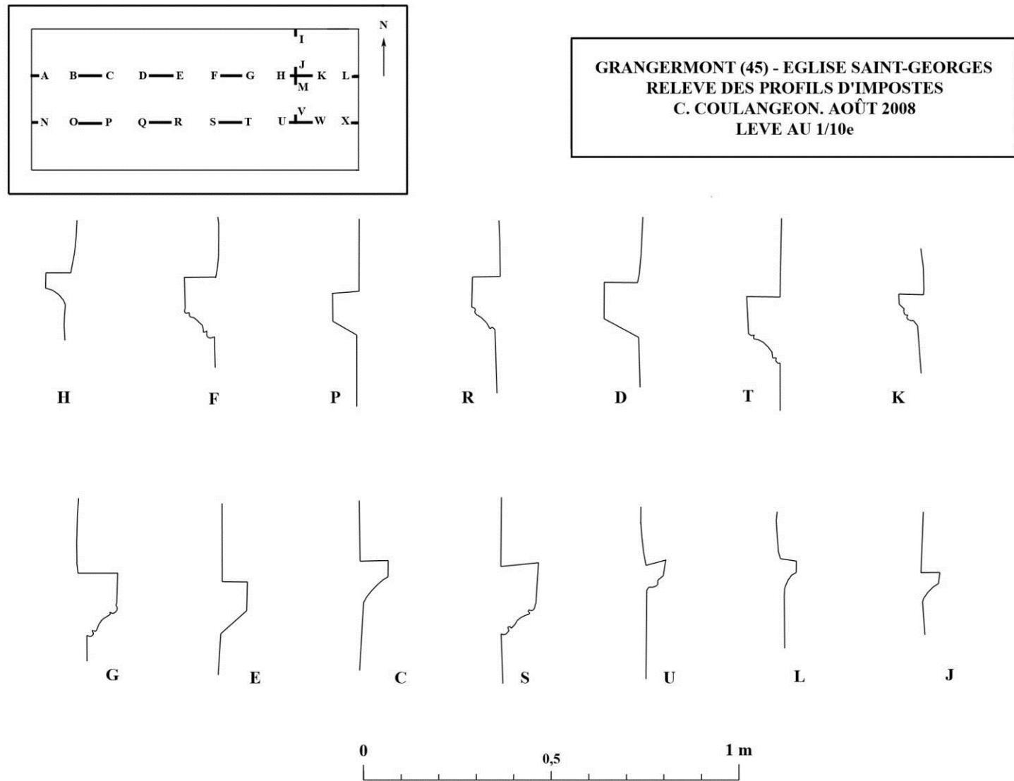
Fig. 10 : Relevés des profils d'impostes de l'église.
