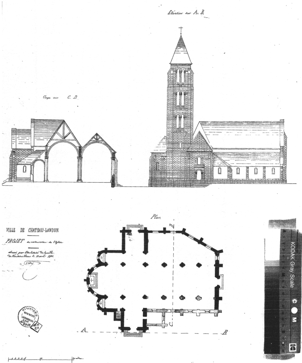
Fig. 7 : Projet pour la restauration de l'église par Lebois, en 1861. Lebois M., Ville de Château-Landon. Projet de restauration de l'église. Plan, Coupe sur CD, Élévation sur AB , Échelle 0,02, 1861, Médiathèque de l'architecture et du patrimoine, 0082/077/2007.
