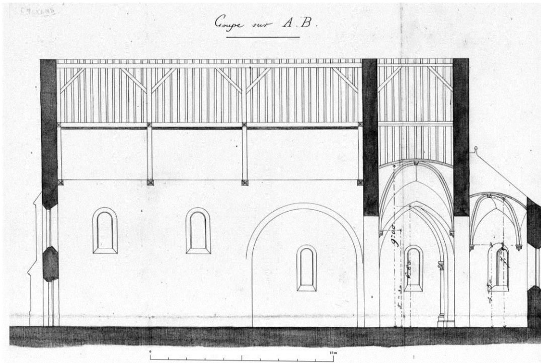
Fig. 7 : Coupe longitudinale de l'église.
