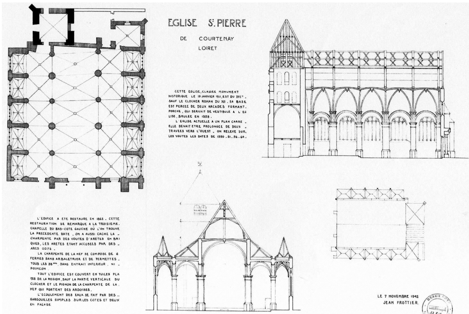
Fig. 5 : Plans et coupes de l'église par l'architecte Frottier, en 1942. Frottier J., Église Saint-Pierre de Courtenay. Loiret. Plans et coupes , s. é., 1942 (CRMH, DRAC Centre, Orléans, dossiers sur la commune de Courtenay, 45115-1 G1).
