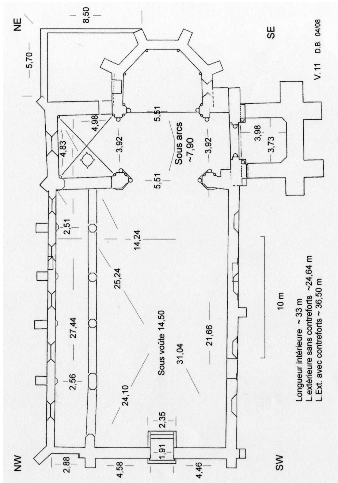
Fig. 6 : Plan de l'église.
