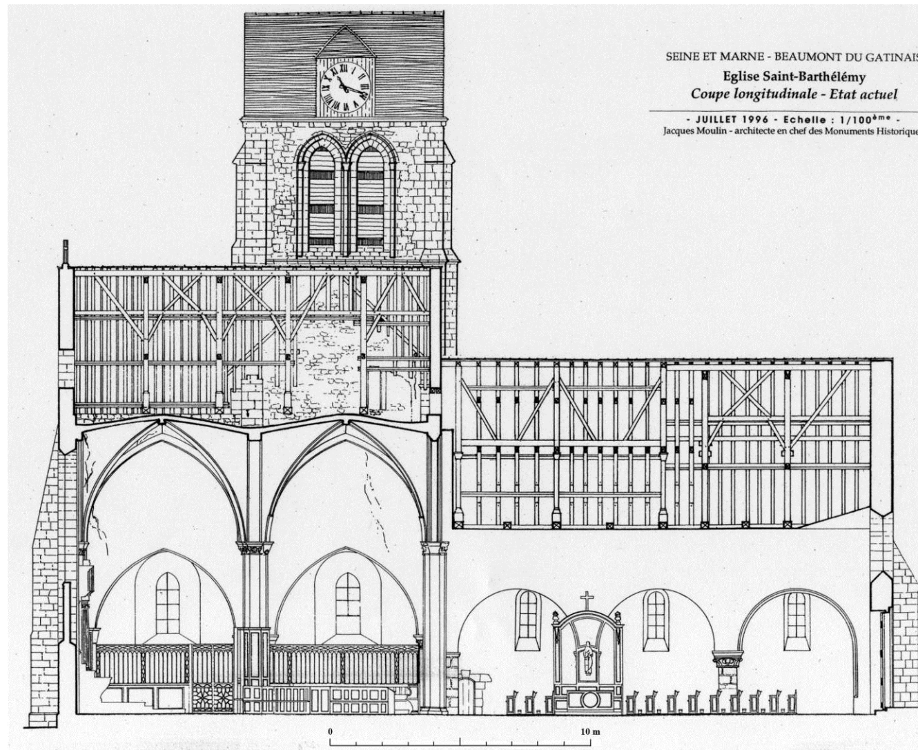
Fig. 13 : Coupe longitudinale de l'édifice.
