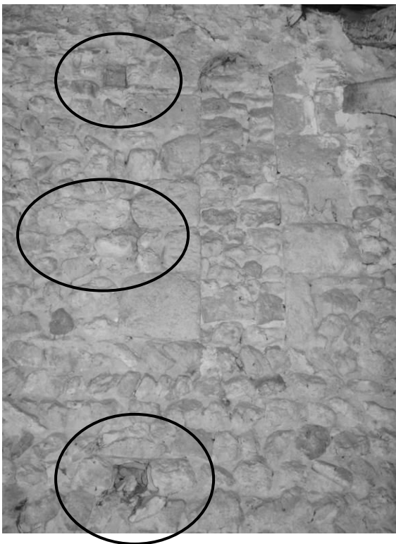
Fig. 54 : Mur gouttereau nord : fenêtre centrale et alignement de trois trous de boulin (entourés).
