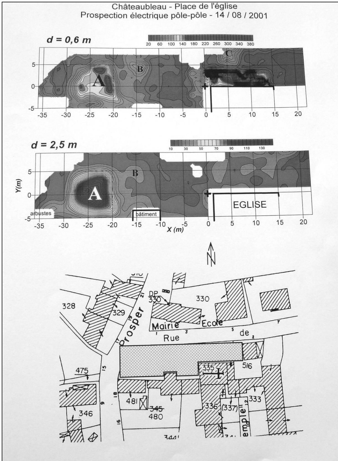
Fig. 8 : Relevés des prospections géophysiques réalisées au sud-ouest de l'église en 2001. In : Martinaud M., Châteaubleau - Prospections électriques , 2001, fig. 6.
