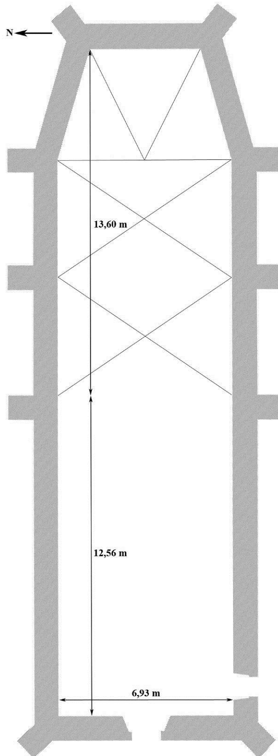
Fig. 4 : Plan schématique de l'église de Boismorand.
