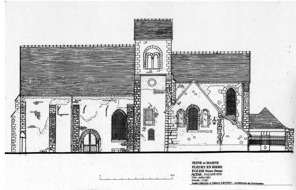
Fig. 7-8 : Plan et élévation de la façade sud de l'église, par Thierry Leynet et André Drozd, en 2003.
