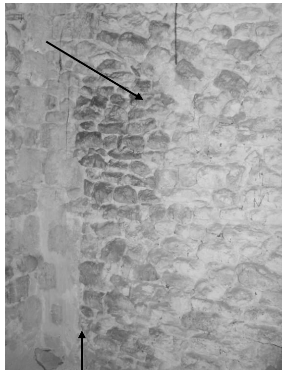
Fig. 59 : Angle entre le pignon occidental du bas-côté nord et le mur gouttereau (les flèches indiquent les vestiges de toiture et la rupture dans le mur avant l'angle).
