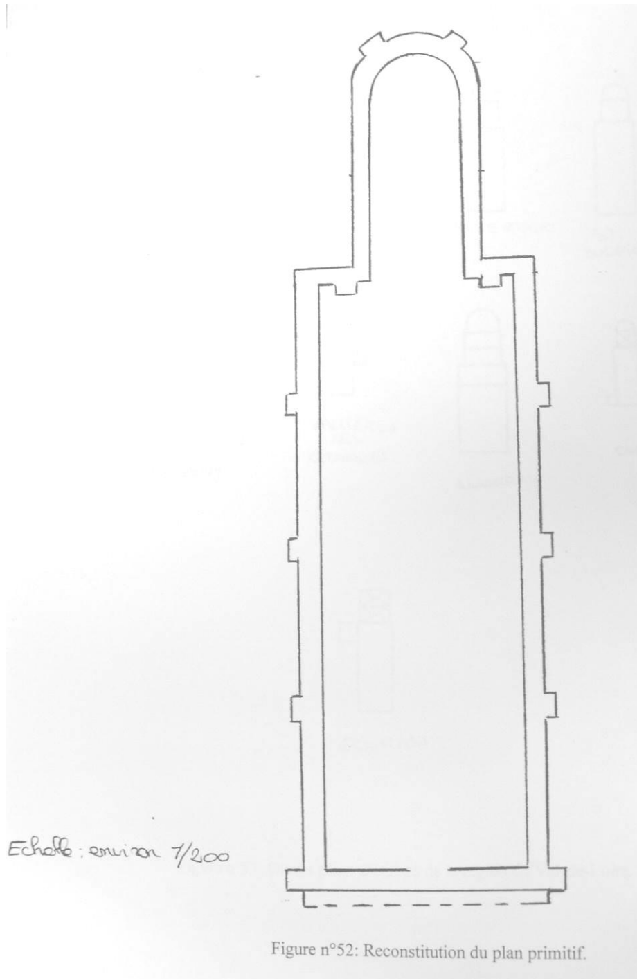
Fig. 9 : Hypothèse pour la restitution du plan de l'église du XI e siècle, par Bérangère Bertrand.
