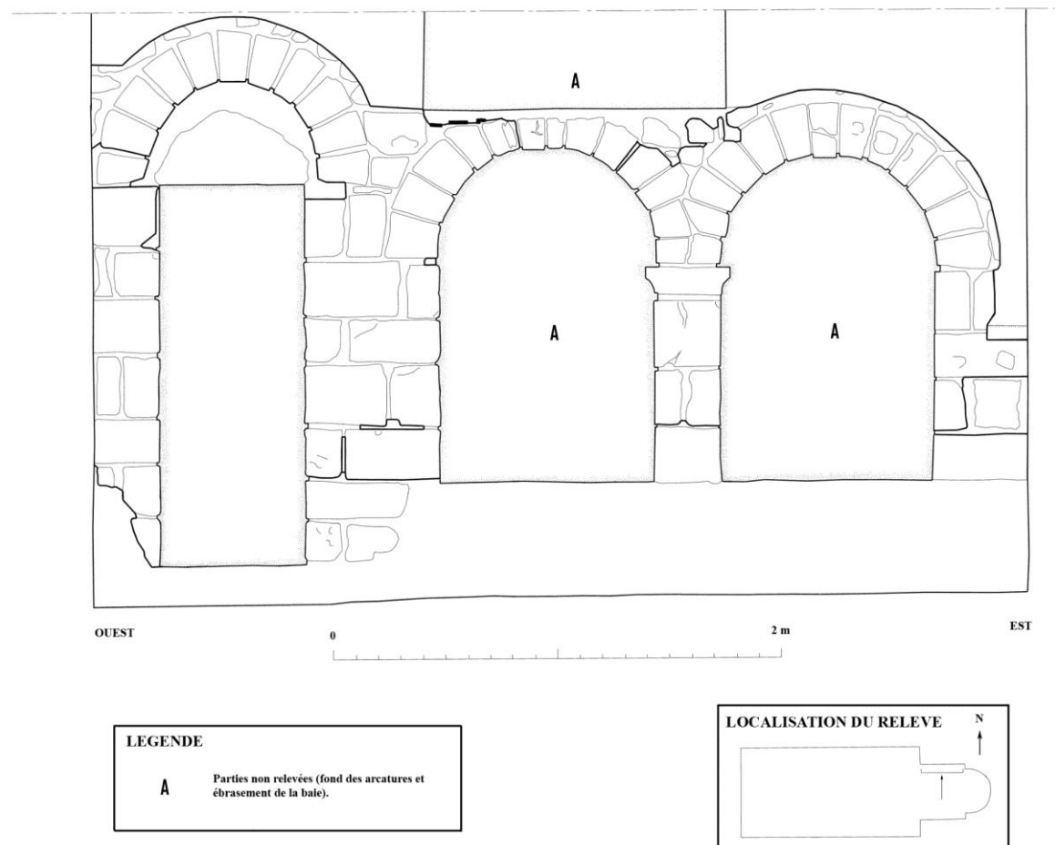
Fig. 12 : Relevé pierre à pierre du mur nord de la travée droite du chœur. Voir planche A3 : volume VI.
