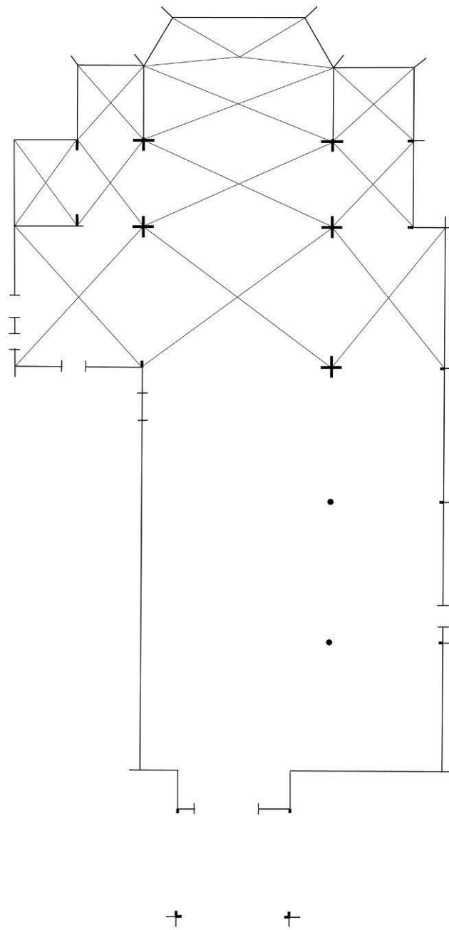
Fig. 3 : Schéma de l'église.
