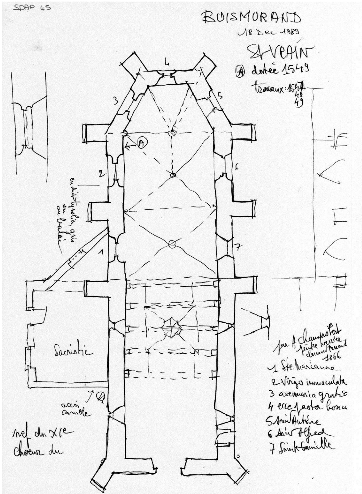
Fig. 5 : Croquis de l'église de Boismorand, par un architecte des Bâtiments de France. In : Boismorand : dossier travaux (Orléans – Service départemental de l'architecture et du patrimoine – Dossier de la commune de Boismorand).
