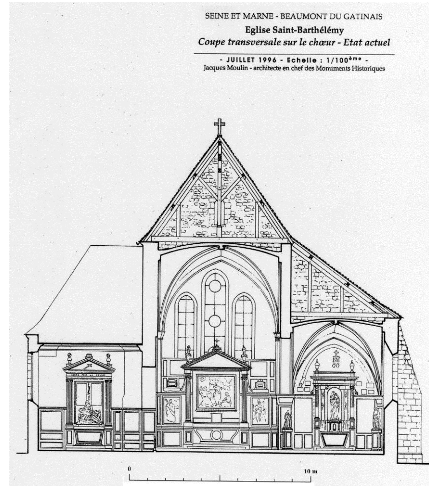
Fig. 15 : Coupe transversale sur le chœur. Moulin J., Seine-et-Marne. Beaumont-du-Gâtinais. Église Saint-Barthélémy. Coupe transversale sur le chœur. État actuel , Échelle 1/100 e , juillet 1996.
