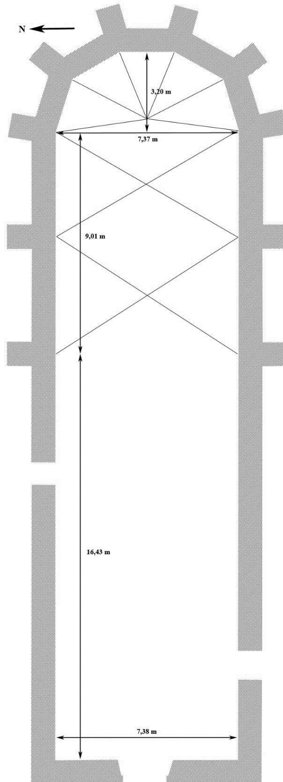
Fig. 4 : Plan schématique de l'église de Chailly-en-Gâtinais.
