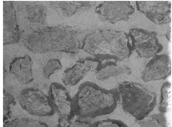
Fig. 19 : Détail du parement en moellons du mur gouttereau sud de la nef.
