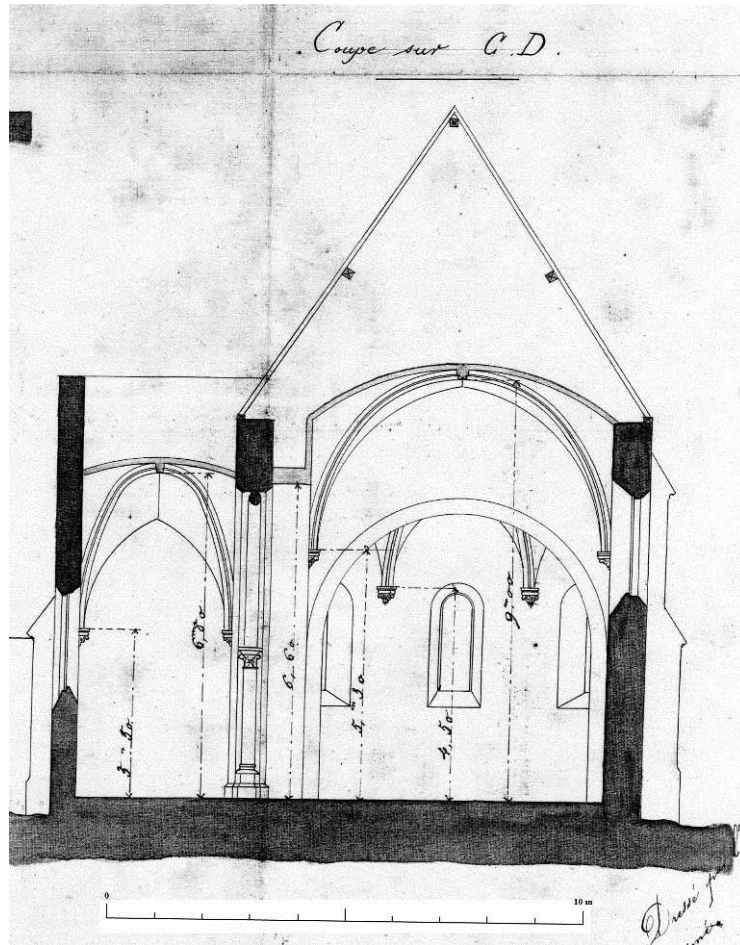
Fig. 9 : Coupe transversale.
