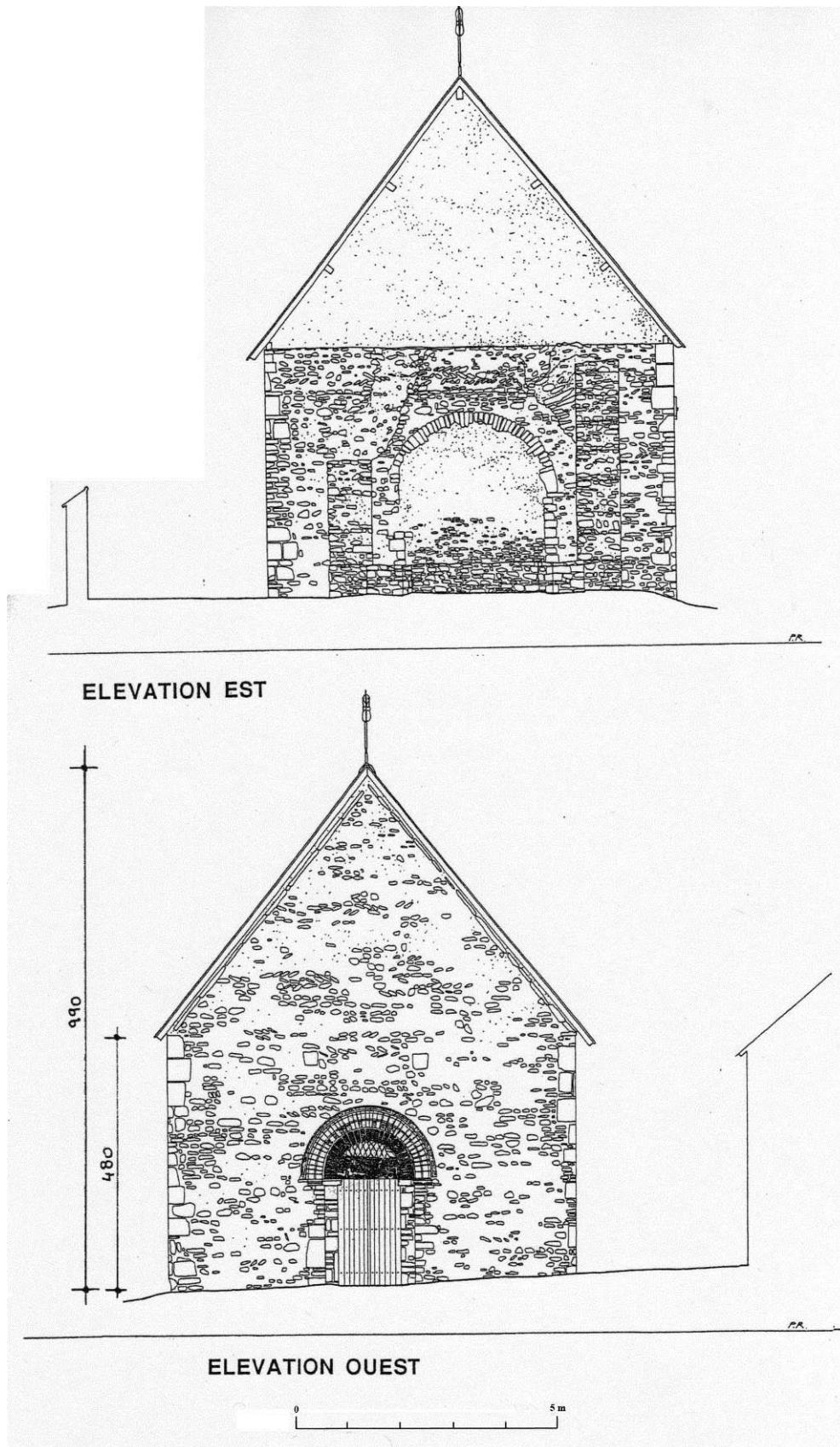
Fig. 10-11 : Relevés des élévations est et ouest de l'église. Leriche A., Cortrat (45) – Église Saint-Martin. Restauration de l'église (tranche 1). Élévations extérieures, Échelle 1/100 e , décembre 2005.
