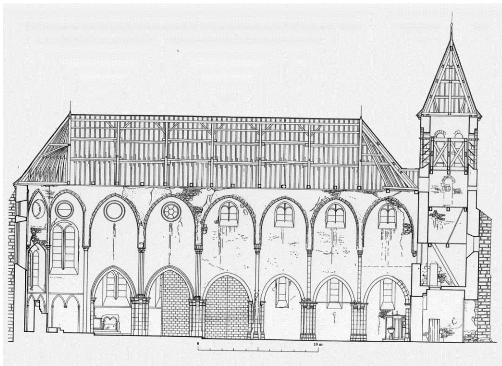
Fig. 8 : Coupe longitudinale sur l'église.
