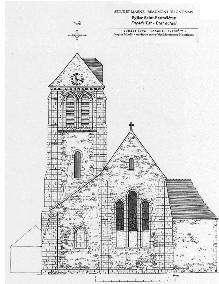
Fig. 10 : Relevé de la façade est. Moulin J., Seine-et-Marne. Beaumont-du-Gâtinais. Église Saint-Barthélémy. Façade est. État actuel , Échelle 1/100 e , juillet 1996.
