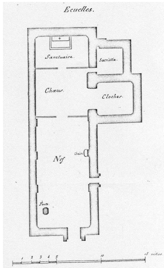
Fig. 7 : Plan anonyme de l'église, daté de 1865. In : Délivré J., Teyssot J., Fiche de pré-inventaire de l'église d'Écuelles , ministère de la Culture, 8 janvier 1975 (Région Ile-de-France – Service régional de l'Inventaire – dossier de la commune d'Écuelles).
