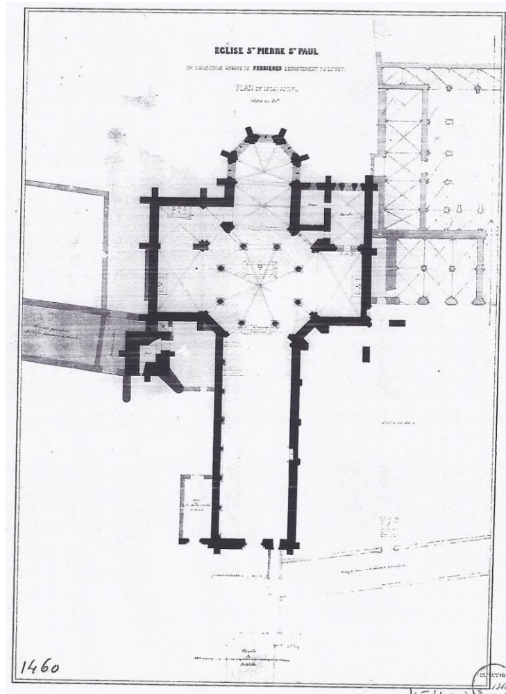
Fig. 3 : Plan de l'église au XIX e siècle. Église Saint-Pierre et Saint-Paul de l'ancienne abbaye de Ferrières. Département du Loiret. Plan de l'état actuel, anonyme, 1847, Échelle 1/184 e .
