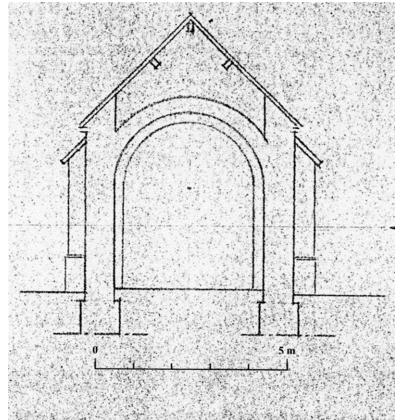
Fig. 11 : Coupe transversale sur le chevet (BB).
