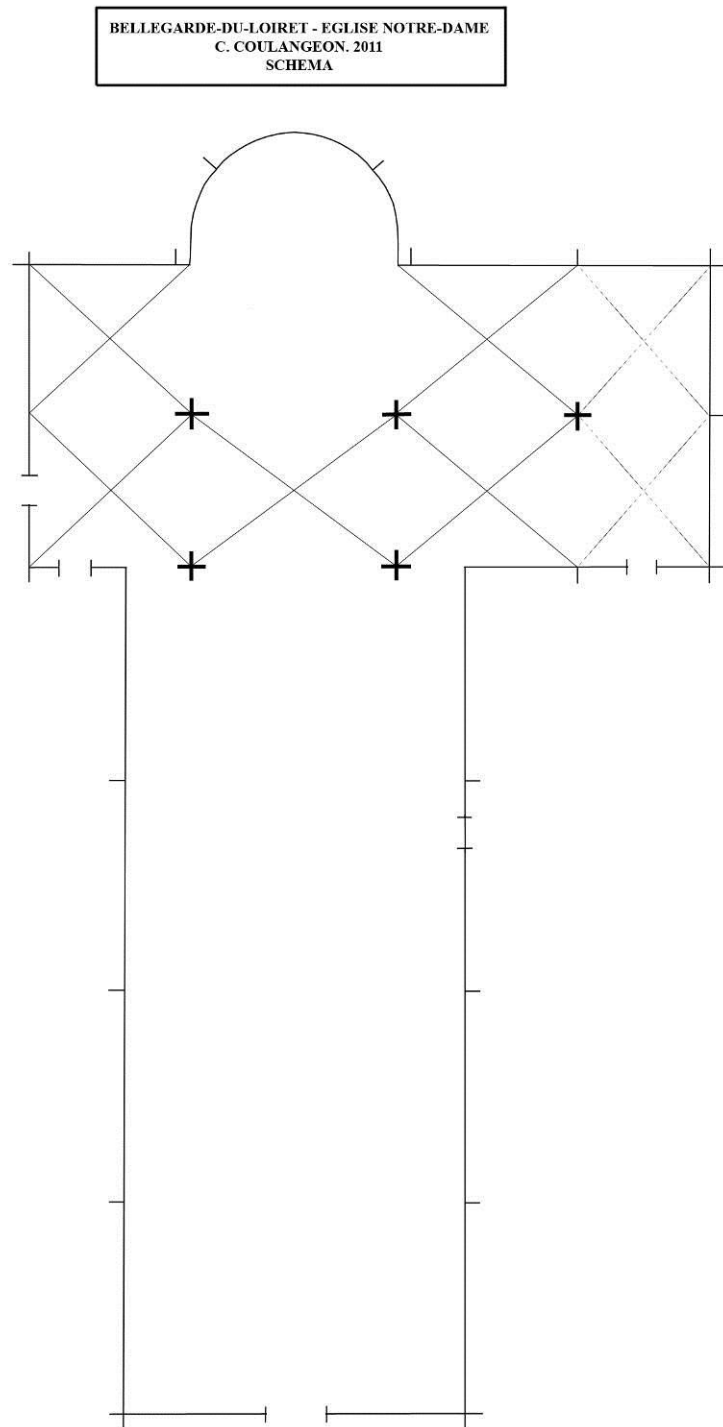
Fig. 5 : Schéma de l'église de Bellegarde.
