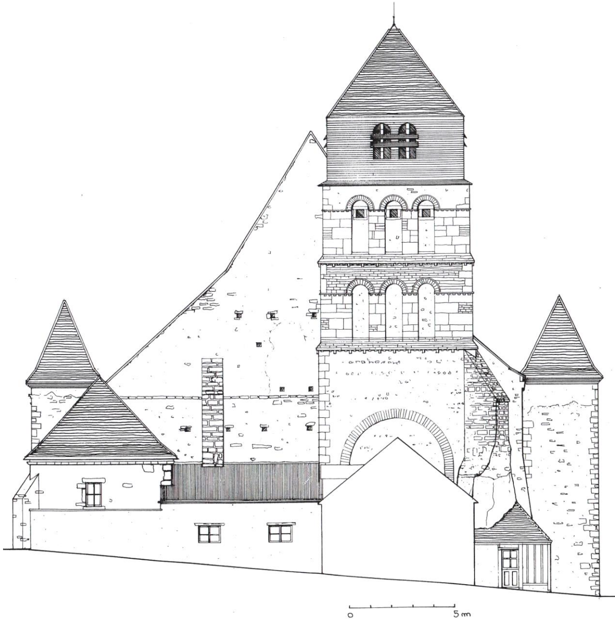
Fig. 9 : Relevé de la façade est du clocher, avant restauration, par Jacques Moulin. Moulin J., Loiret. Courtenay. Église. Façade est , Échelle de 1 cm pour 1 m, 1989 (CRMH, DRAC Centre, Orléans, dossiers sur la commune de Courtenay, 45115-1 G1).
