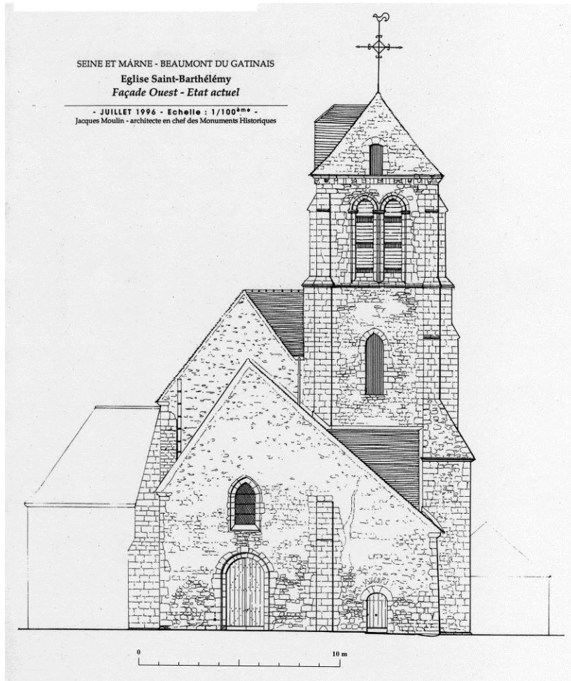
Fig. 9 : Relevé de la façade ouest. Moulin J., Seine-et-Marne. Beaumont-du-Gâtinais. Église Saint-Barthélémy. Façade ouest. État actuel , Échelle 1/100 e , juillet 1996.
