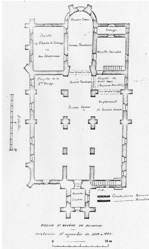
Fig. 7 : Plan de l'église de Bourron-Marlotte, en 1865. Plan de l'église de Bourron restaurée et agrandie de 1858 à 1861, s. é., 1865, Inventaire général, DRAC Ile-de-France, Dossiers de la commune de Bourron-Marlotte.
