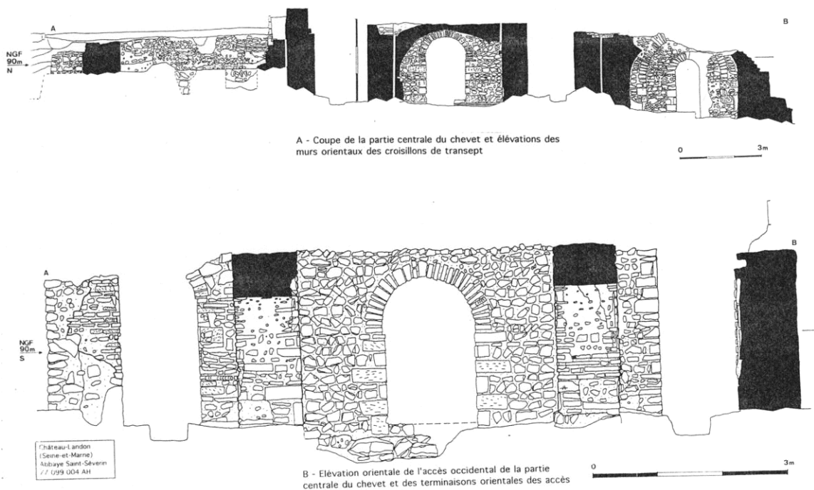
Fig. 26 : Relevés des élévations du mur oriental de la crypte.
