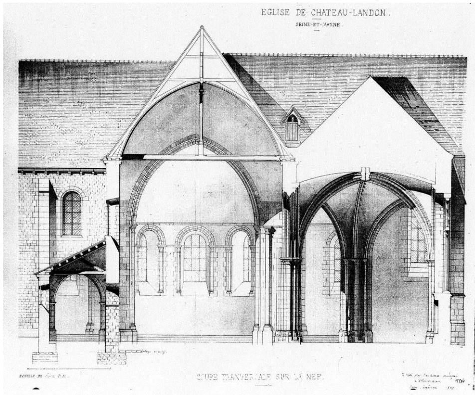
Fig. 14 : Coupe transversale sur l'église.
