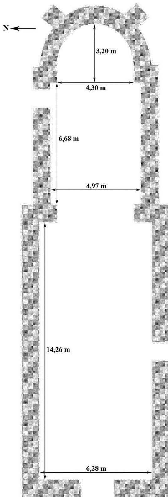
Fig. 5 : Plan schématique de l'église.
