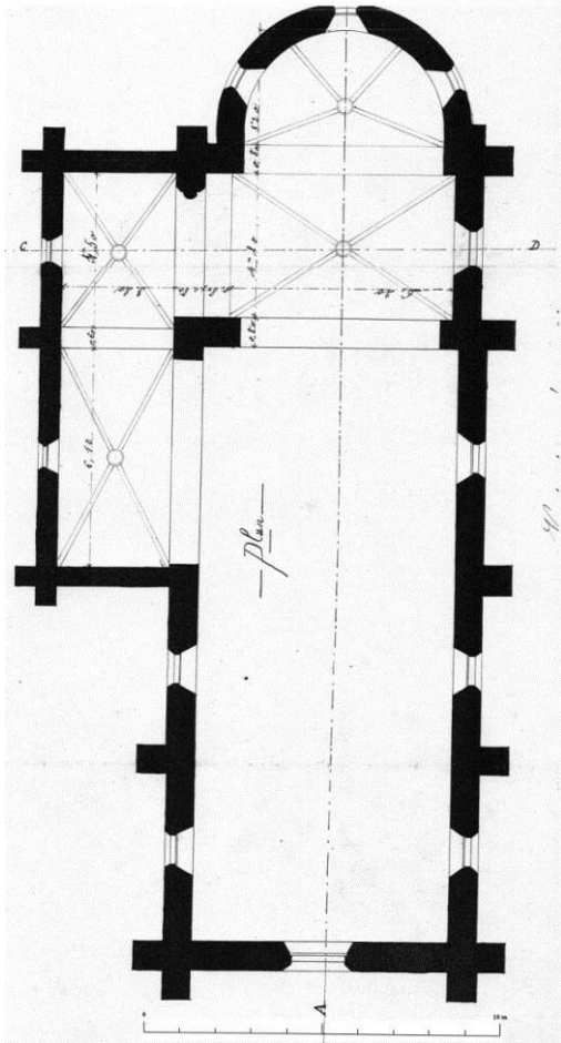
Fig. 5 : Plan de l'église, par l'architecte Heurteau.
