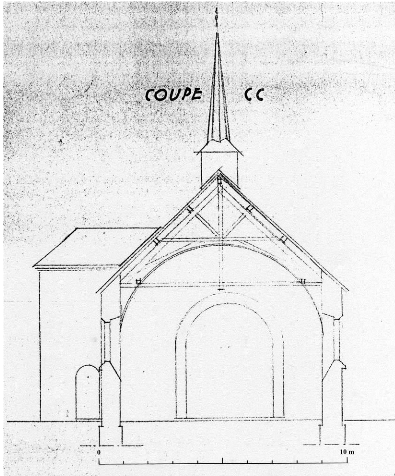
Fig. 10 : Coupe transversale sur la nef.
