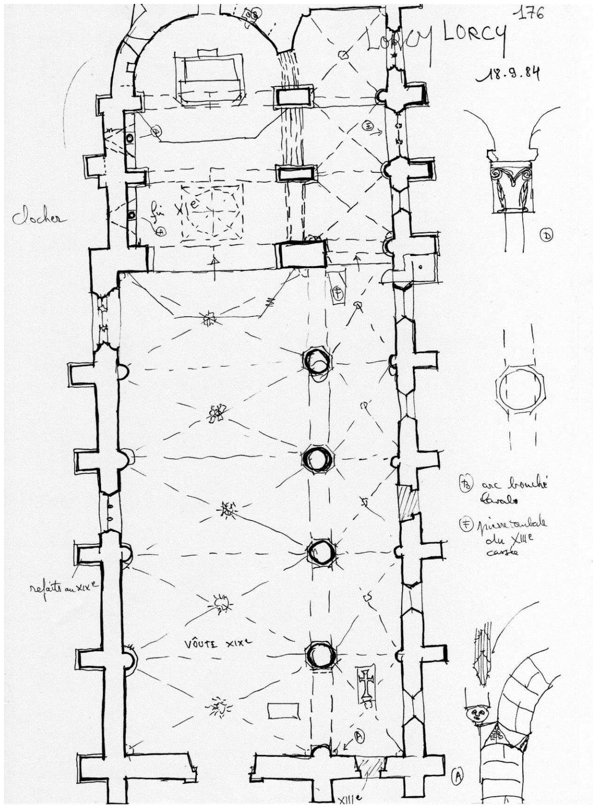
Fig. 5 : Croquis de l'église par un architecte des Bâtiments de France en 1984. In : Lorcy : dossier travaux (Orléans – Service départemental de l'architecture et du patrimoine – Dossier de la commune de Lorcy).
