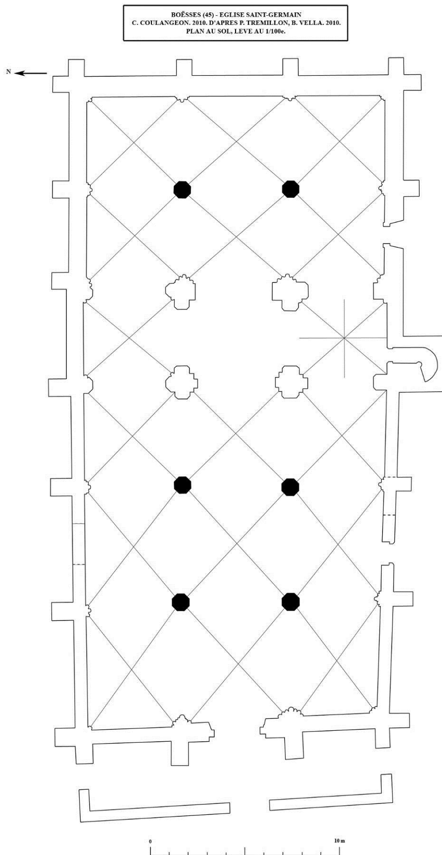
Fig. 5 : Plan de l'église de Boësses.
