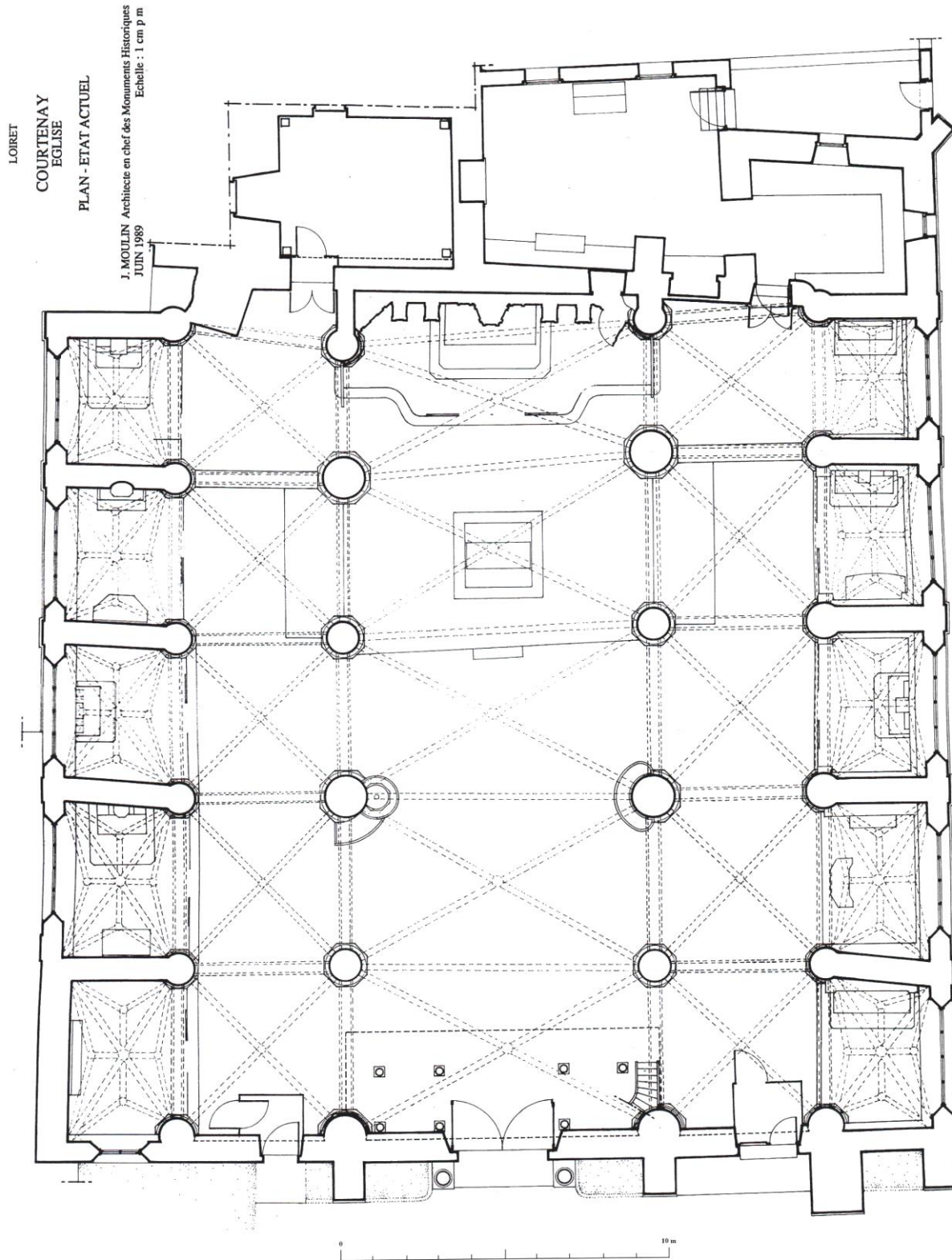
Fig. 6 : Plan de l'église par Jacques Moulin en 1989. Moulin J., Loiret. Courtenay. Église. Plan – État actuel , Échelle de 1 cm pour 1 m, 1989 (CRMH, DRAC Centre, Orléans, dossiers sur la commune de Courtenay, 45115-1 G1). Les numéros 1, 2 et 3 renvoient à la localisation des inscriptions.
