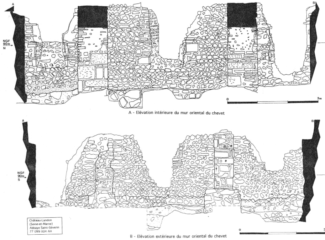
Fig. 25 : Relevés des élévations du mur oriental de la crypte.
