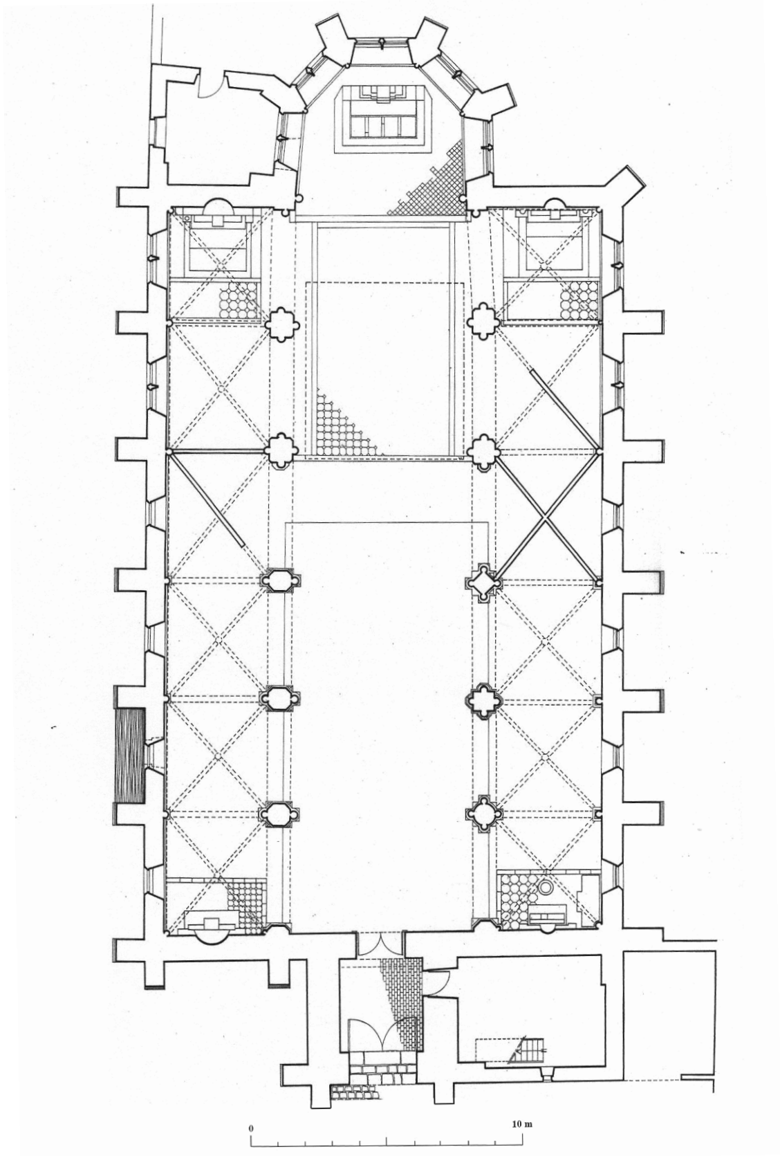
Fig. 6 : Plan de l'église par Jacques Moulin en 1997. Moulin J., Seine-et-Marne. Donnemarie-Dontilly. Église Saint-Pierre et Saint-Paul de Dontilly. État actuel. Plan, Échelle 1/100 e , 1997.
