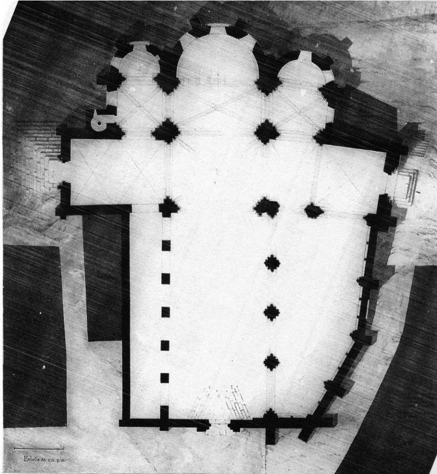
Fig. 5 : Plan de l'église levé en 1850.
