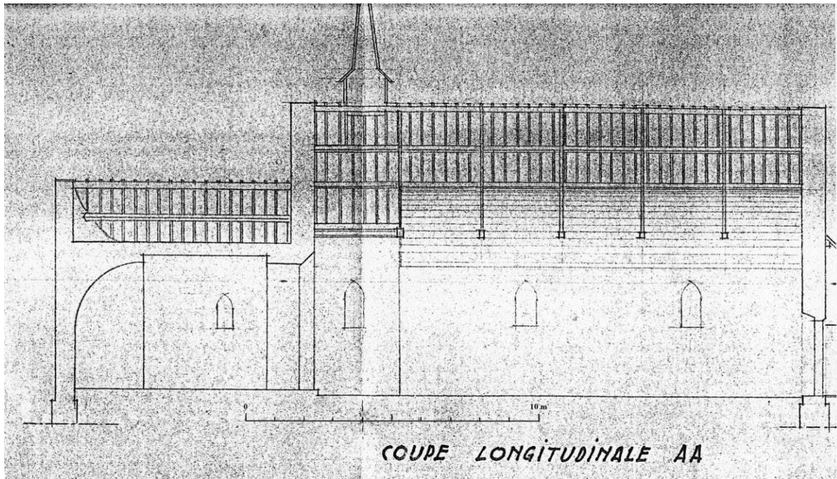
Fig. 8 : Coupe longitudinale de l'église.
