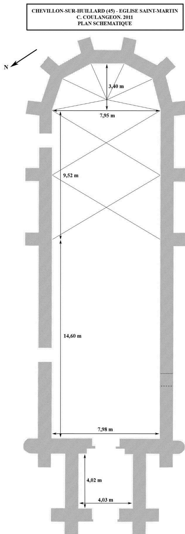
Fig. 4 : Plan schématique de l'église de Chevillon-sur-Huillard.
