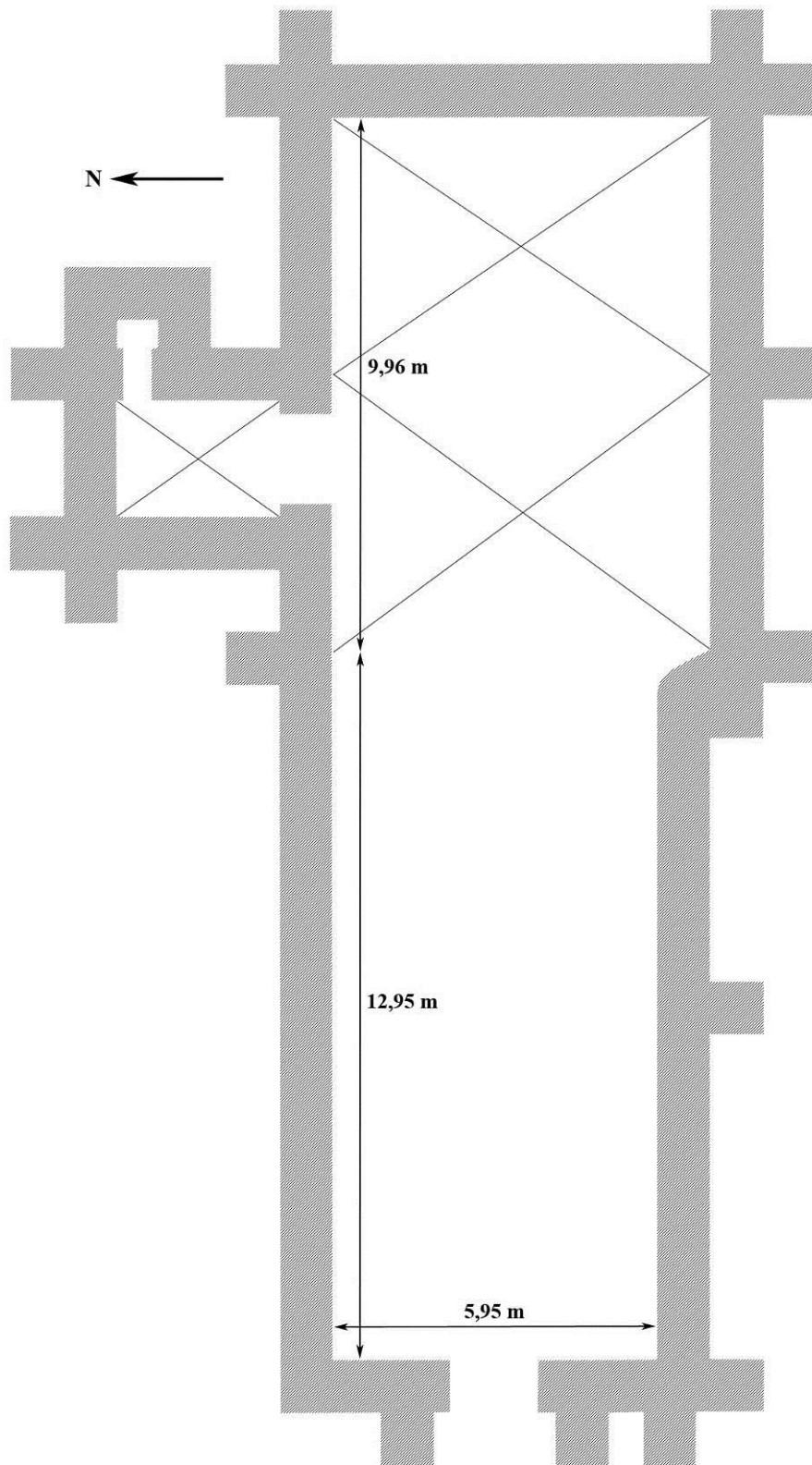
Fig. 4 : Plan schématique de l'église.
