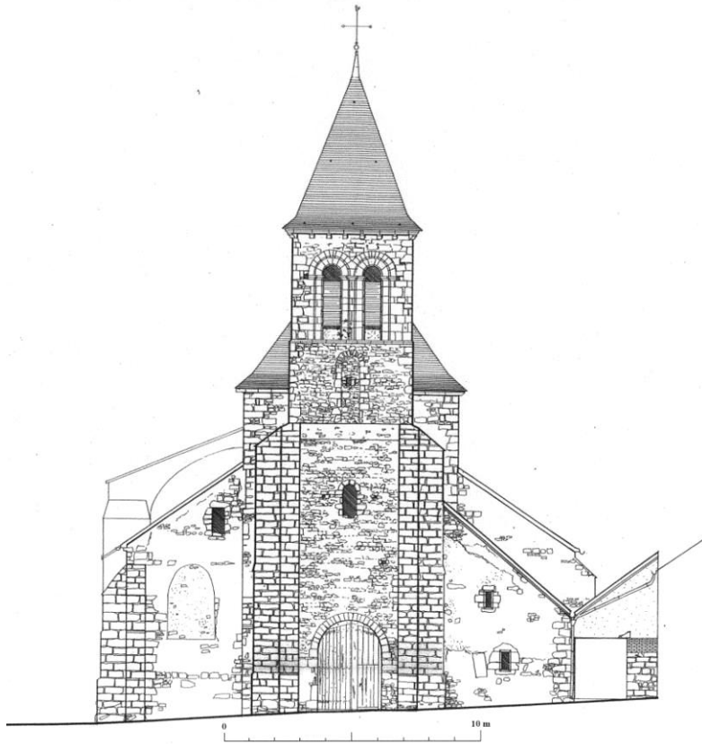
Fig. 9 : Façade occidentale.
