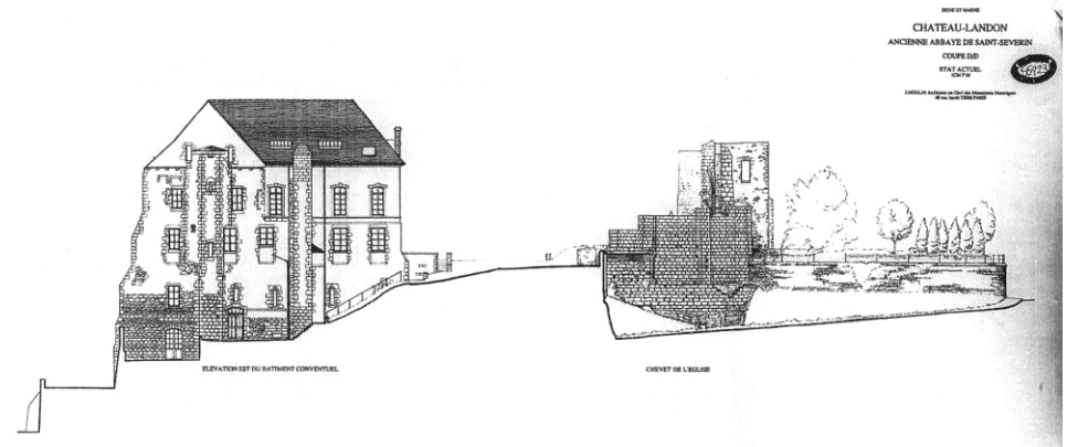
Fig. 10 : Élévation orientale de l'abbaye avant restauration. Moulin J., État actuel, Élévation est du bâtiment conventuel. Coupe du chevet de l'église , Échelle 0,01, s. d., Médiathèque de l'architecture et du patrimoine, 0082/077/2006.
