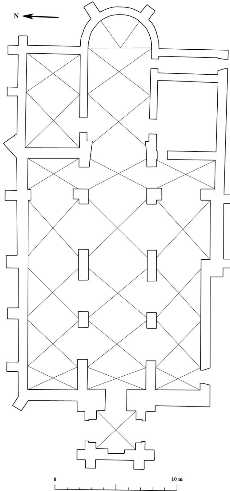
Fig. 4 : Plan de l'église.
