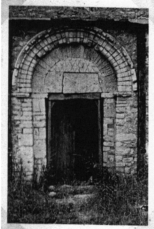
Fig. 57 : Le portail ouest en août 1953. Cortrat : dossier travaux (Orléans – Service départemental de l'architecture et du patrimoine – Dossier de la commune de Cortrat) [photographie n°MIIa].
