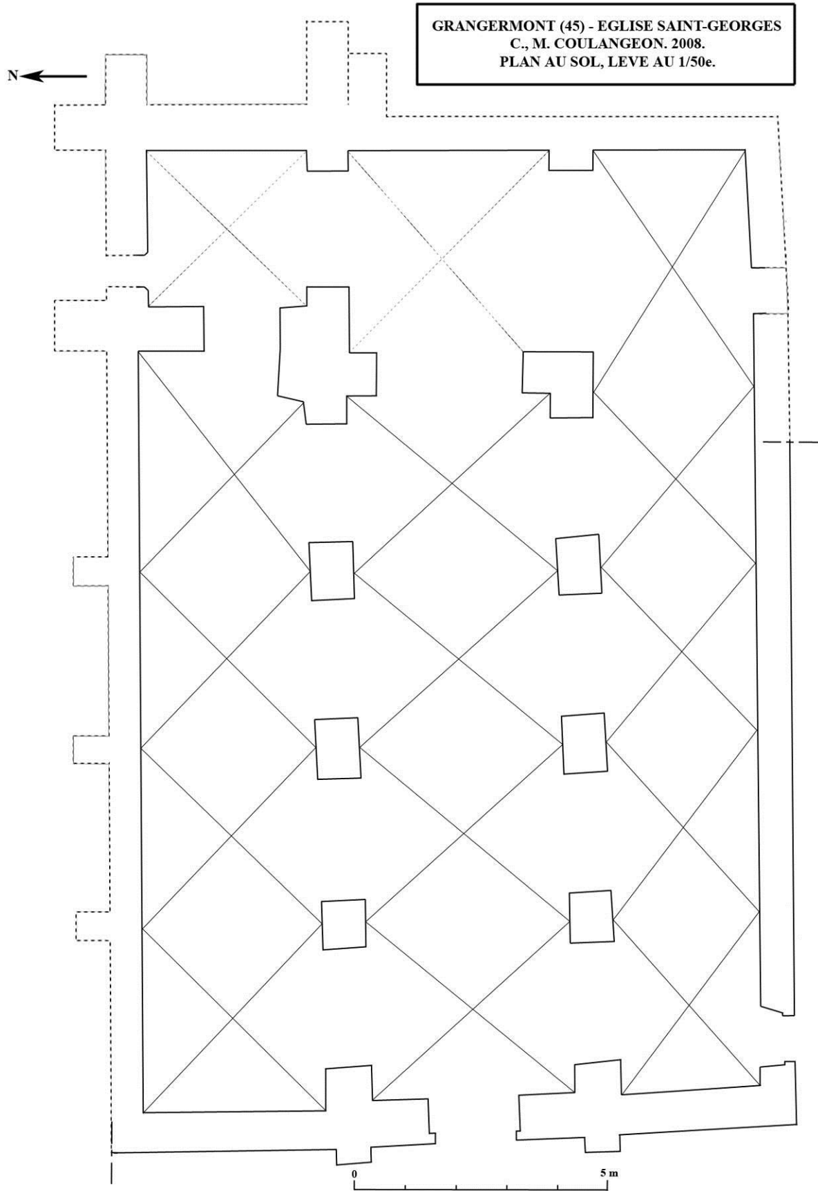
Fig. 5 : Plan de l'église.
