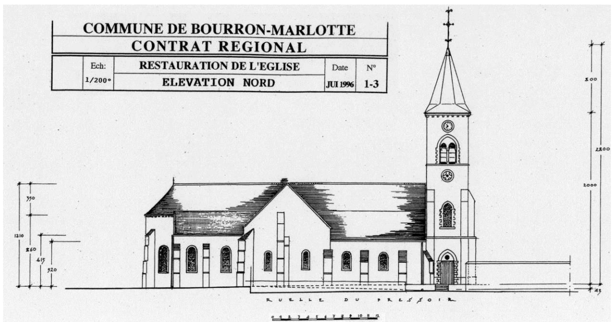
Fig. 10 : Élévation de la façade nord. Bergevin O. de, Commune de Bourron-Marlotte. Contrat régional. Restauration de l'église, juillet 1996, Cahier de plans, fig. 1-3.
