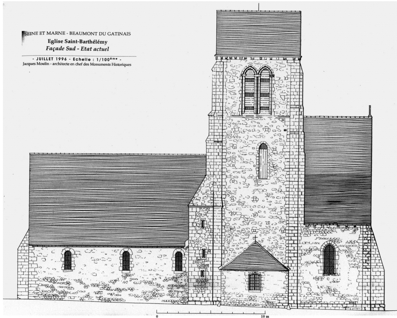
Fig. 12 : Relevé de la façade sud.
