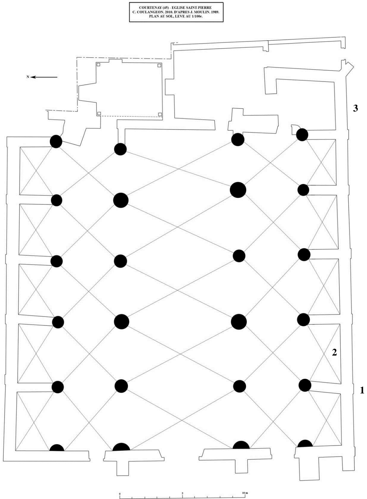
Fig. 4 : Plan de l'église de Courtenay, d'après Jacques Moulin. Les numéros indiquent la localisation des inscriptions.
