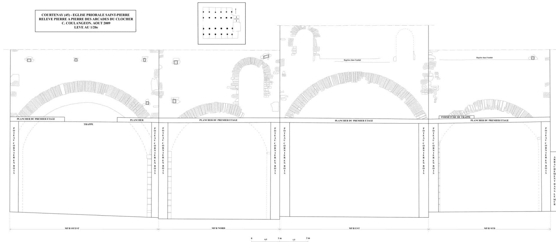
Fig. 11 : Relevé pierre à pierre des arcades du clocher. Voir planche A3 : volume VI.
