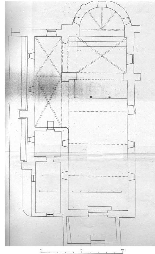
Fig. 6 : Plan de l'église par l'architecte Merceron.
