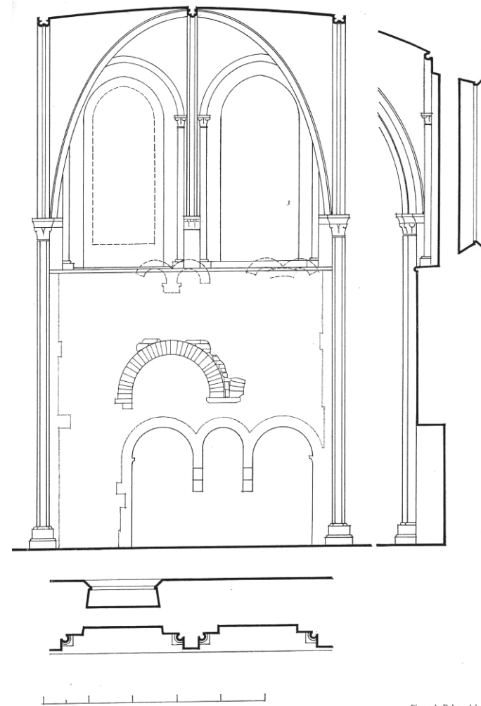
Fig. 15 : Relevé des traces de baies dans le mur sud du chevet par Saulnier.
