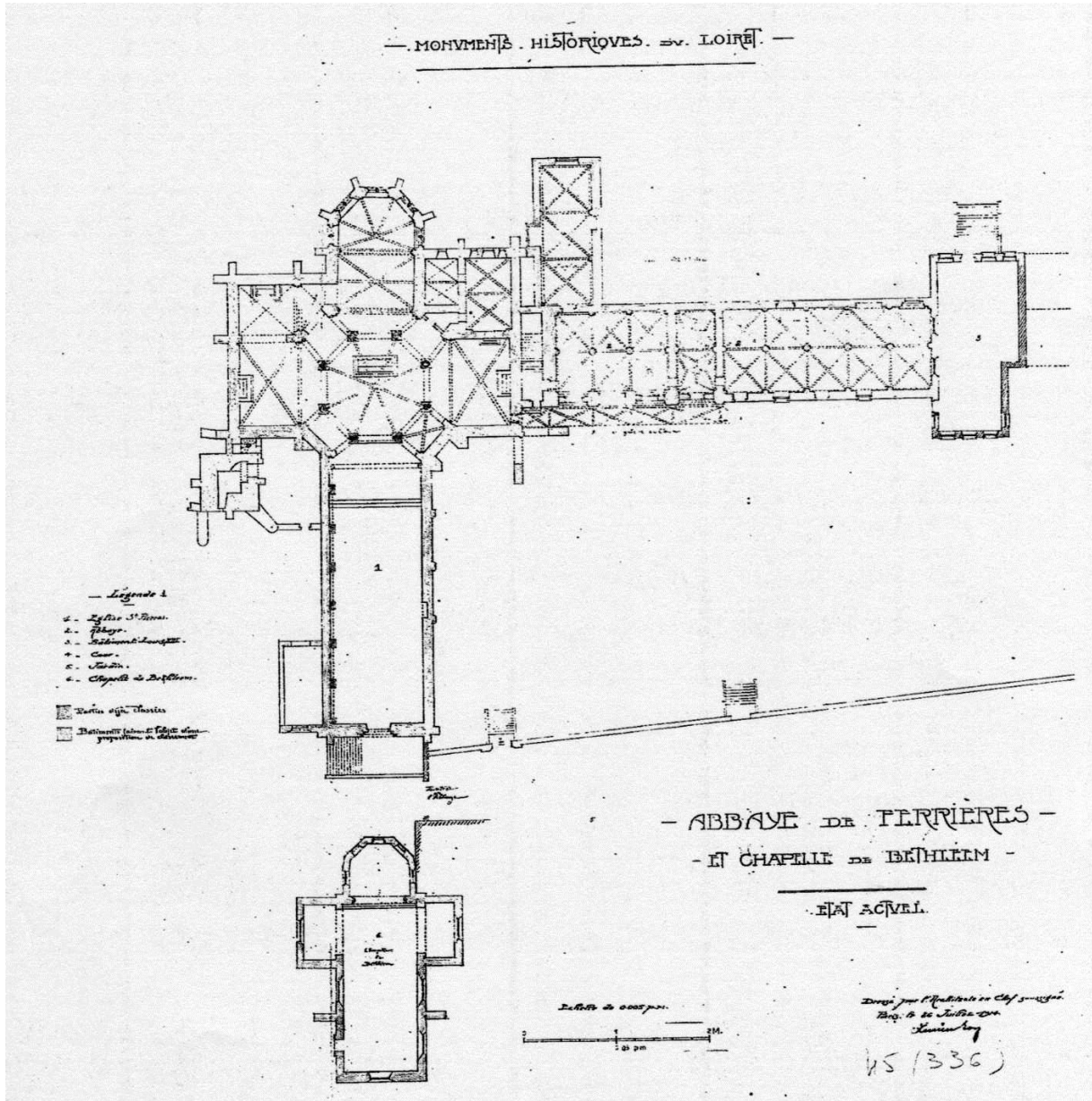
Fig. 5 : Plan des vestiges de l'abbaye en 1914. Roy L., Monuments historiques du Loiret. Abbaye de Ferrières et chapelle de Bethléem. État actuel , 26 juillet 1914, Échelle de 0,005 m pour 1 m.
