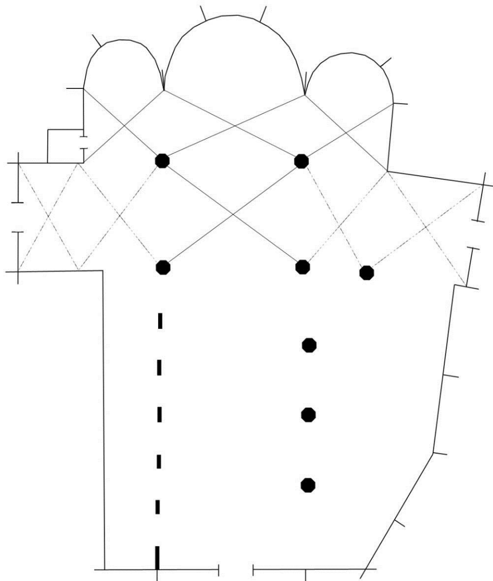
Fig. 3 Schéma de l'église Notre-Dame.
