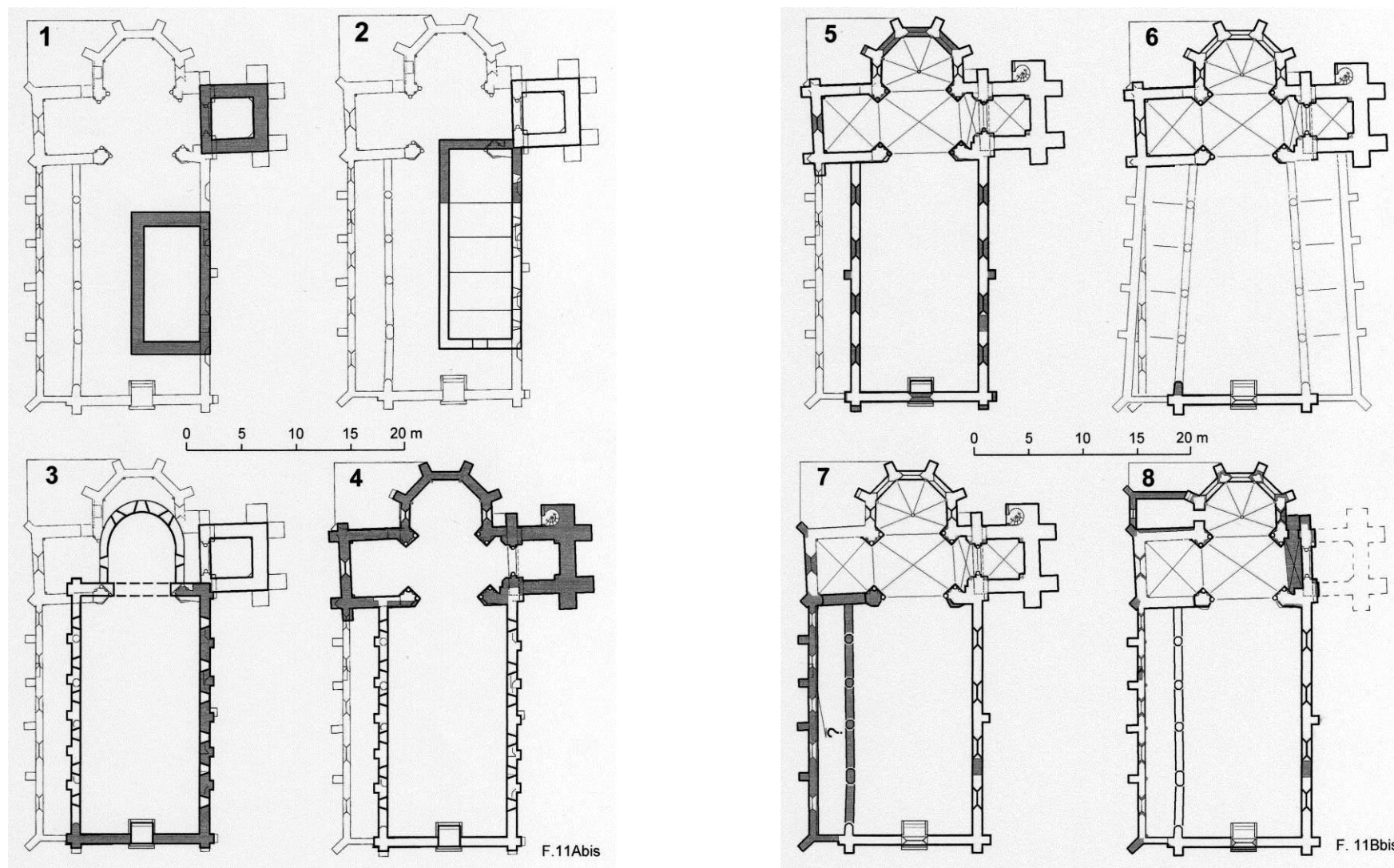
Fig. 7-8 : Hypothèses de Dominique Bureau pour la chronologie de l'édifice. In : Bureau D., Éléments et corps architecturaux de l'église St-Bon et St-Dulcide à Loury (Loiret), fig. 11 A et 11 B.
