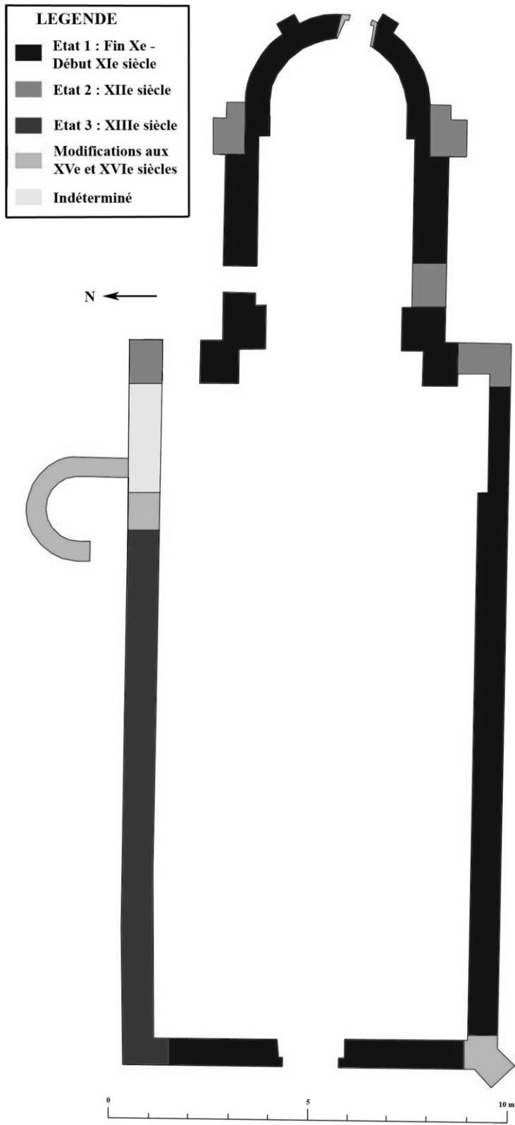
Fig. 14 : Plan phasé de l'église de Bondaroy. Voir planche couleur : volume VI.
