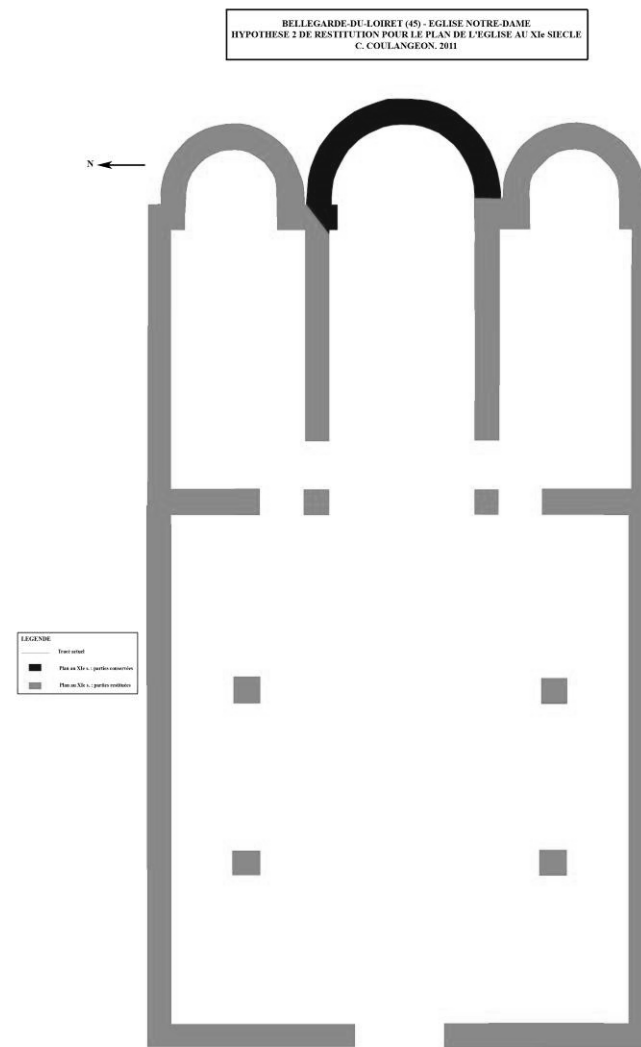
Fig. 11 : Restitution du plan de l'église pour le XI e siècle : hypothèse 2.
