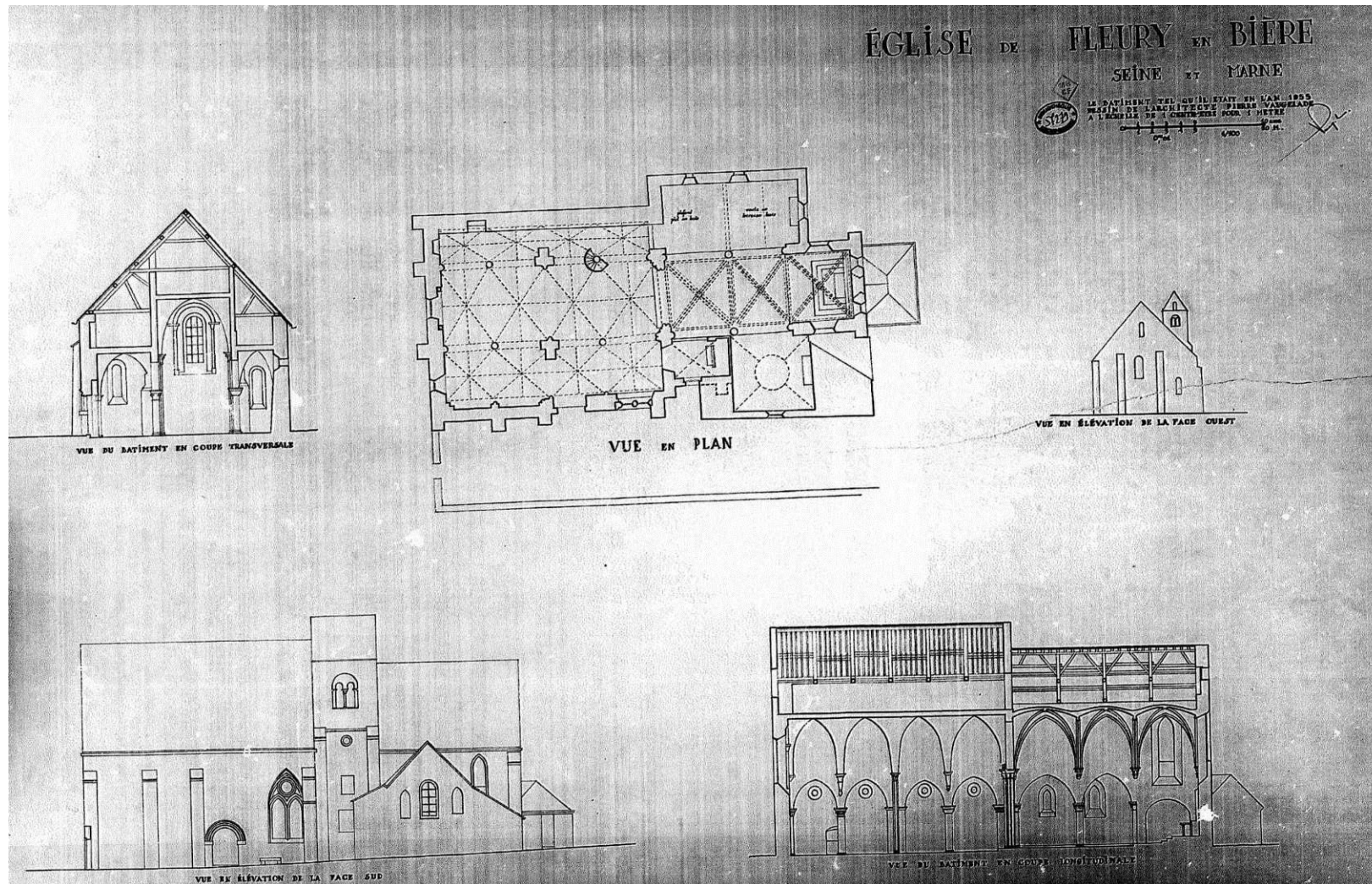
Fig. 6 : Plan, coupes et relevés des façades par Pierre Vaugelade en 1955.
