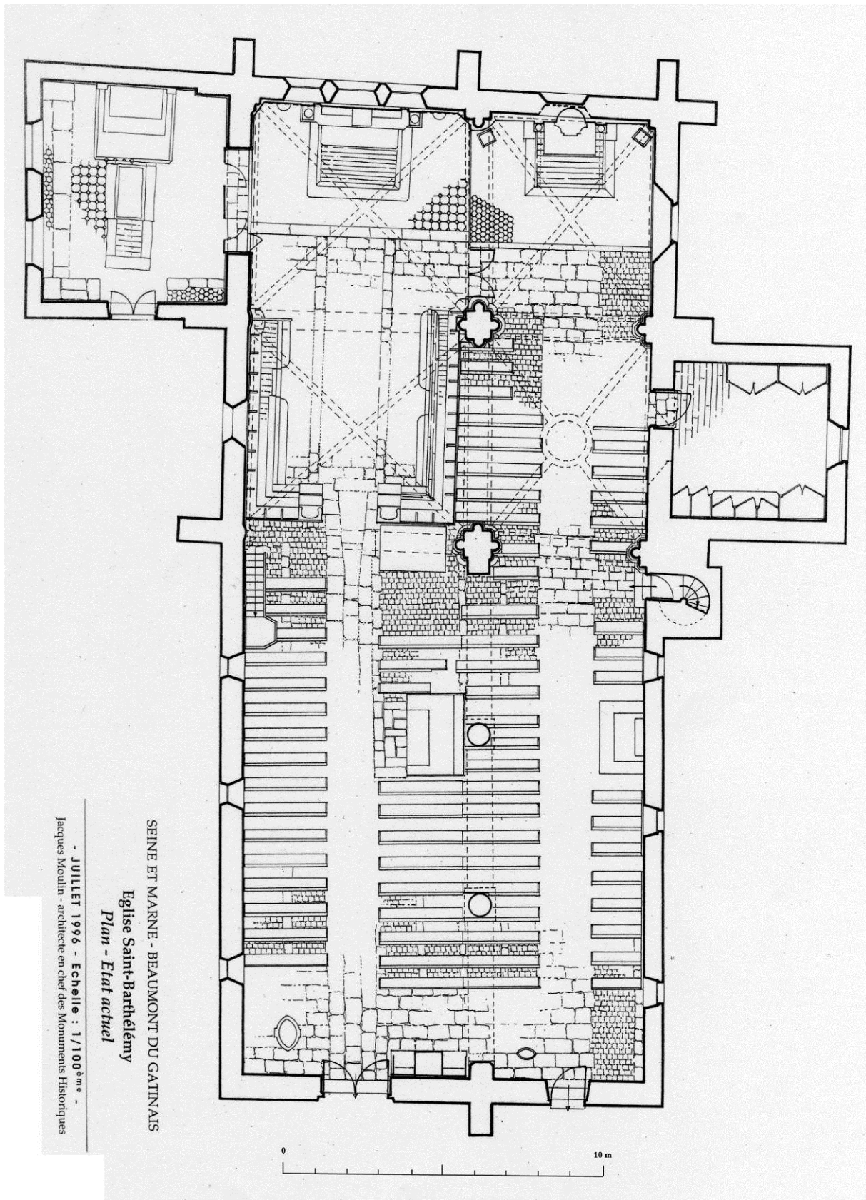
Fig. 8 : Plan de l'église de Beaumont-du-Gâtinais, par Jacques Moulin en 1996. Moulin J., Seine-et-Marne. Beaumont-du-Gâtinais. Église Saint-Barthélémy. Plan. État actuel , Échelle 1/100 e , juillet 1996.
