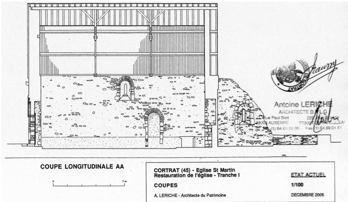
Fig. 12 : Coupe longitudinale, montrant l'élévation intérieure nord. Leriche A., Cortrat (45) – Église Saint-Martin. Restauration de l'église (tranche 1). Coupes , Échelle 1/100 e , décembre 2005.
