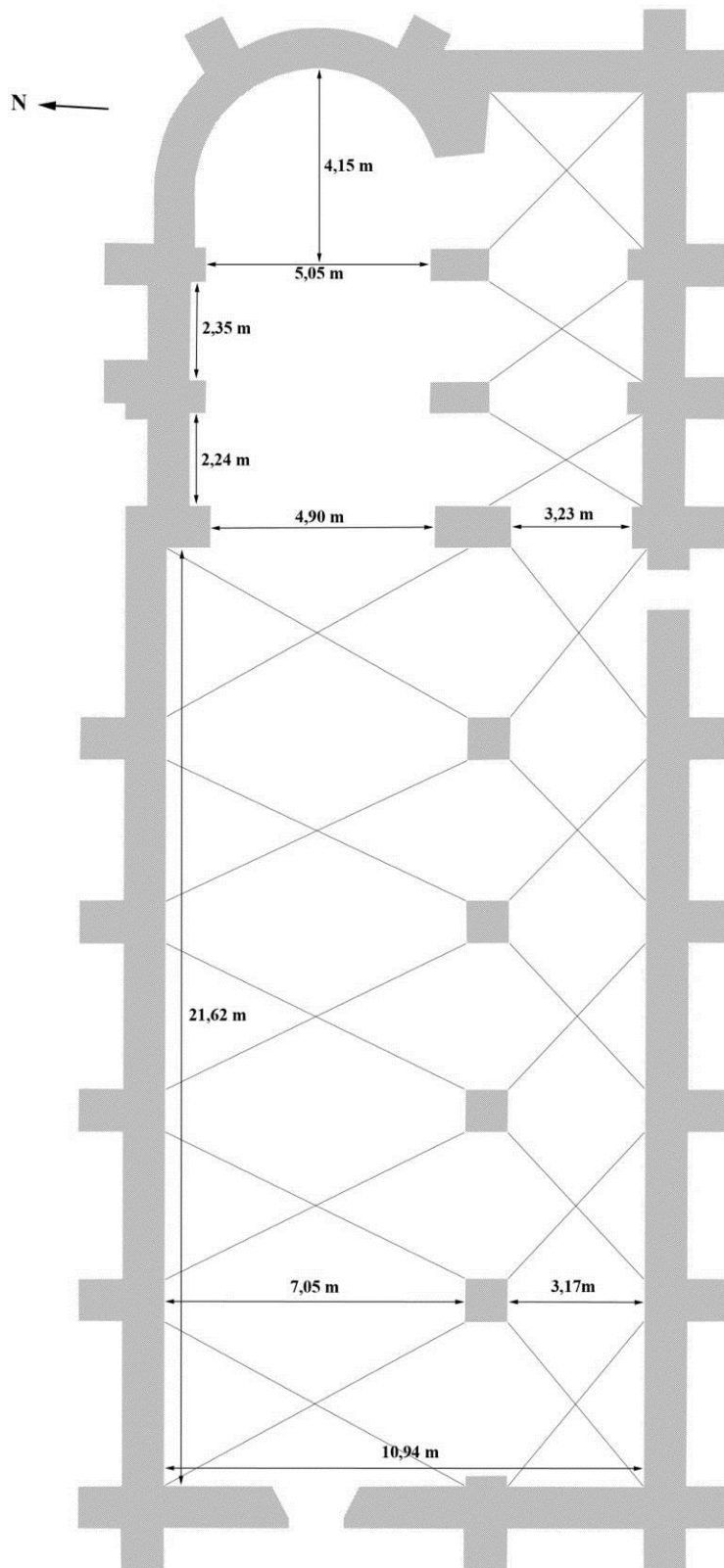
Fig. 4 : Plan schématique de l'église.
