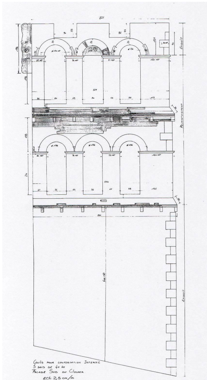
Fig. 8 : Schéma des travaux réalisés sur la face sud du clocher, par Jacques Moulin. Échelle de 2,5 cm pour 1 m.
