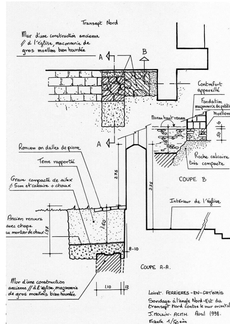
Fig. 8-9 : Plan de localisation et relevés du sondage réalisé en 1998 au nord-est du transept. In : Goubet R., Ferrières-en-Gâtinais (45). Église Saint-Pierre et Saint-Paul. Études de sols. Rapport , 3 juillet 1998, 14 p. (Annexe de l'étude préalable de Jacques Moulin de 1998).
