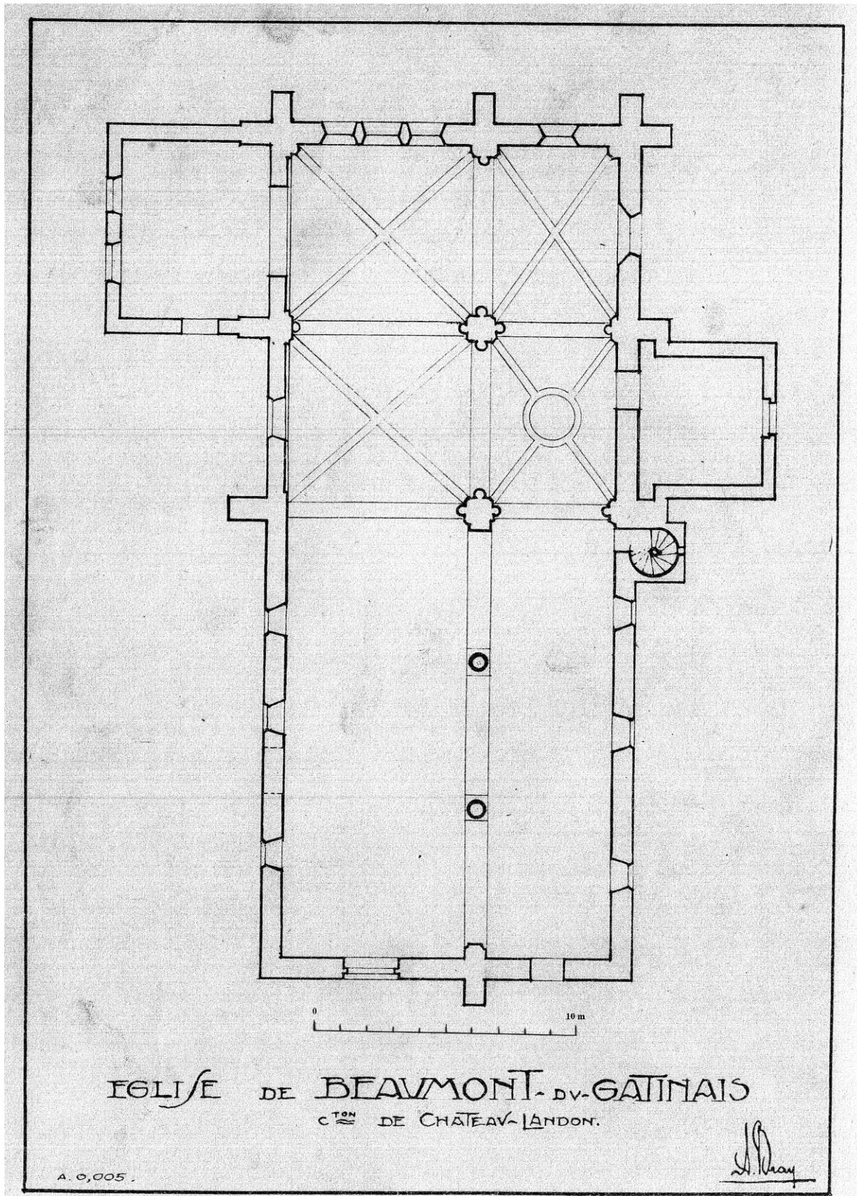
Fig. 7 : Plan de l'église de Beaumont-du-Gâtinais, par Albert Bray dans les années 1950. Bray A., Église de Beaumont-du-Gâtinais . Canton de Château-Landon, Plan, Échelle 1/200 e , s. d.
