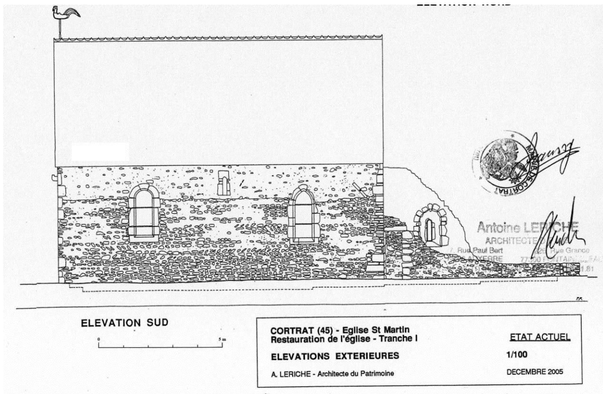
Fig. 9 : Relevé de l'élévation sud de l'église. Leriche A., Cortrat (45) – Église Saint-Martin. Restauration de l'église (tranche 1). Élévations extérieures, Échelle 1/100 e , décembre 2005.
