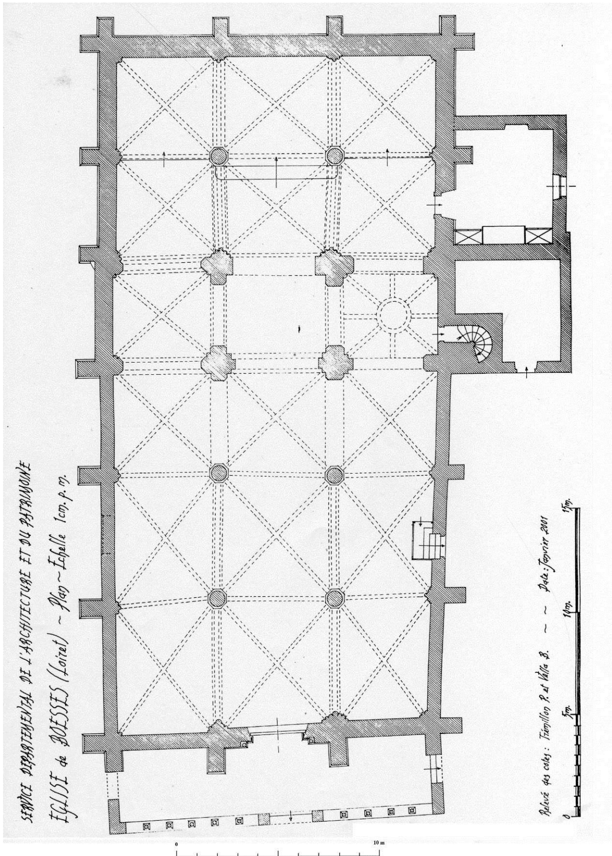
Fig. 6 : Plan de l'église de Boësses levé en 2001.
