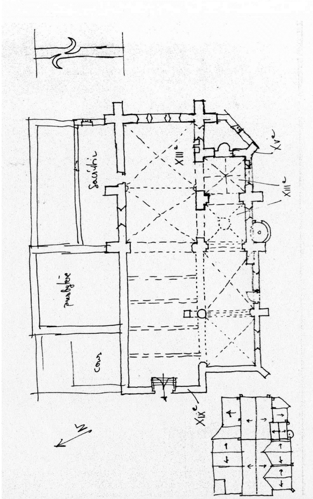
Fig. 5 : Croquis de l'église par un architecte des Bâtiments de France. In : Donnery : dossier travaux (Orléans – Service départemental de l'architecture et du patrimoine – Dossier de la commune de Donnery).
