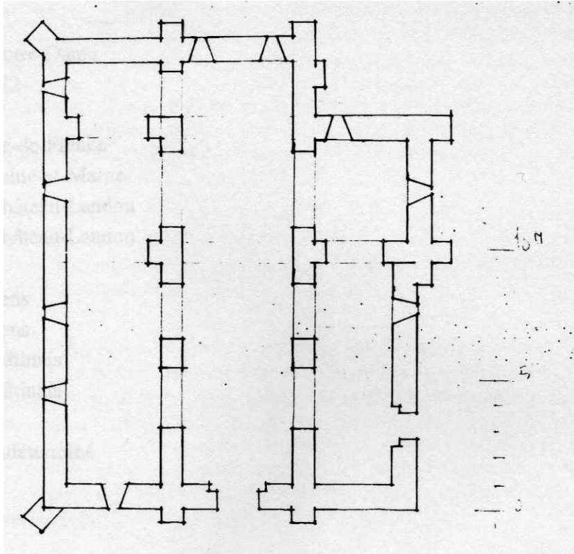
Fig. 11 : Reconstitution de l'état du XI e siècle par Jean-Louis Bernard.
