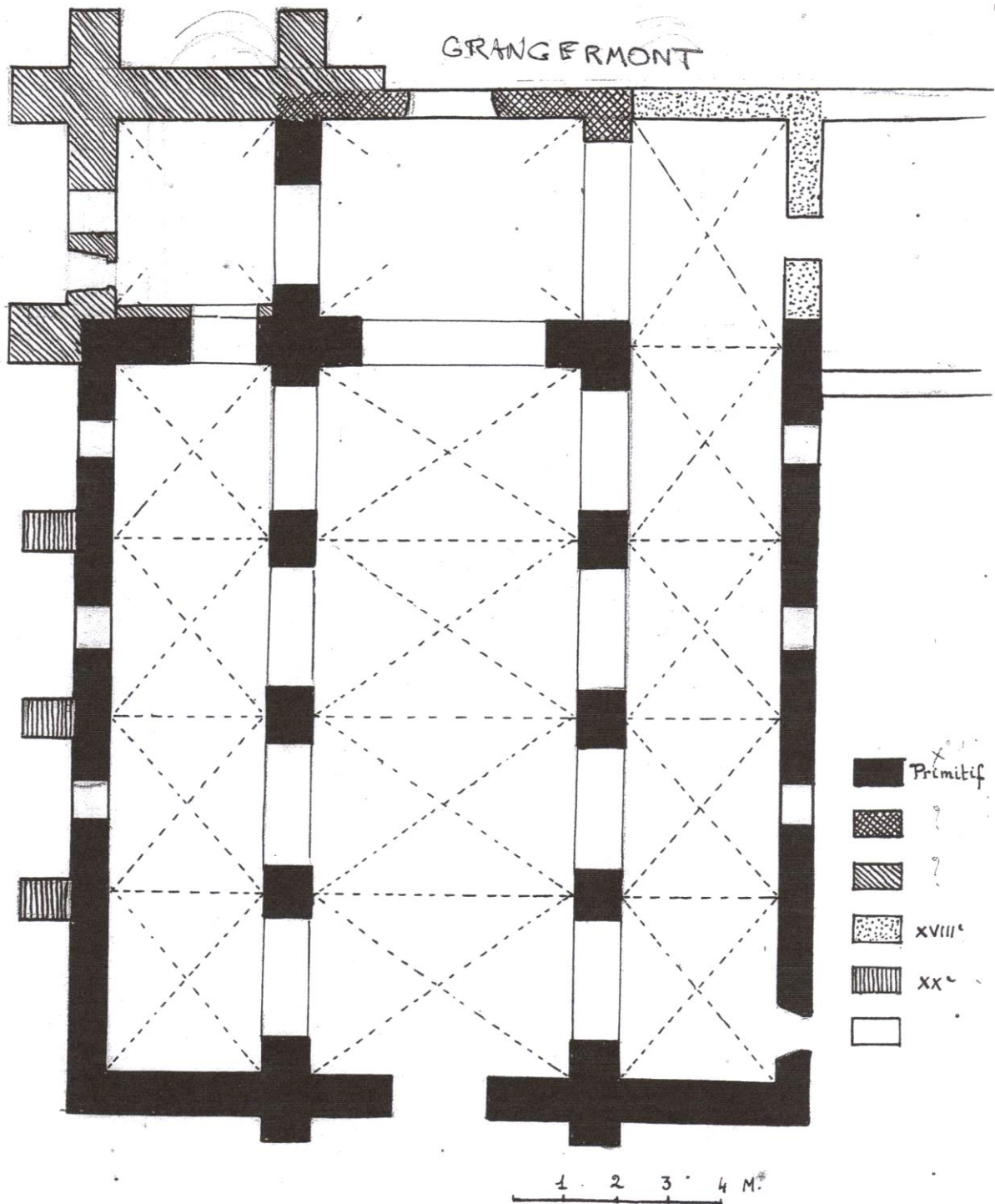
Fig. 6 : Plan de l'église par l'abbé Moufflet.
