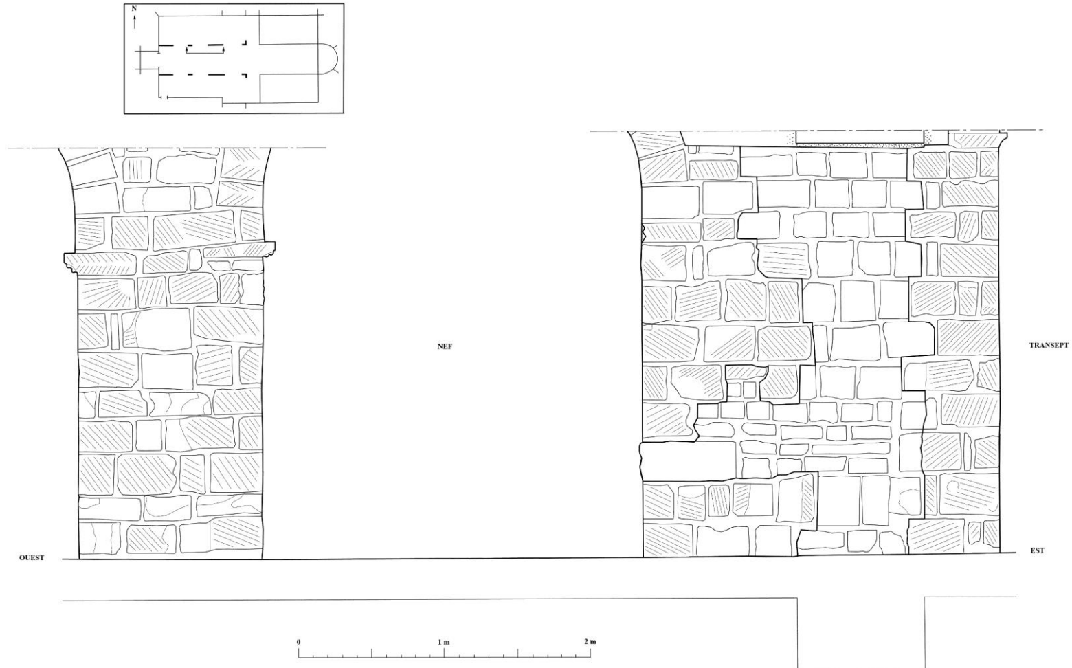
Fig. 13 : Relevé pierre à pierre de l'arcade orientale du mur gouttereau nord de la nef.
