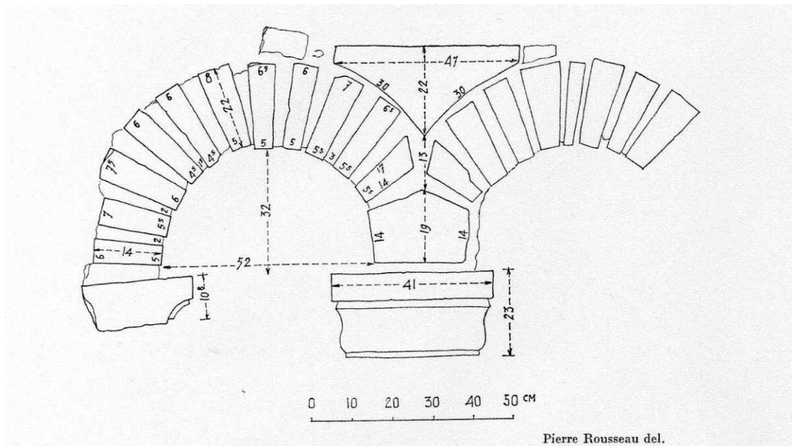
Fig. 17 : Relevé d'une des arcades du mur sud de la travée droite. In : Saulnier L., Ferrières-en-Gâtinais, Bulletin Monumental 130-IV, Paris, éd. de la Société française d'archéologie, 1972, fig. 4.
