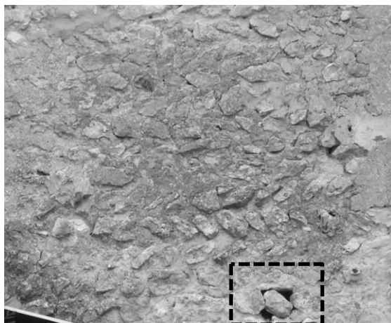
Fig. 28 : Détail du parement en opus spicatum du mur sud avec le trou de boulin (détail de la fig. 26).
