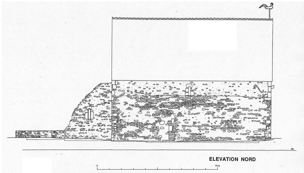
Fig. 8 : Relevé de l'élévation nord de l'église. Leriche A., Cortrat (45) – Église Saint-Martin. Restauration de l'église (tranche 1). Élévations extérieures, Échelle 1/100 e , décembre 2005.
