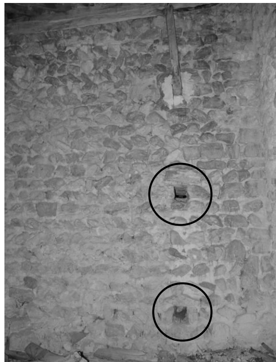
Fig. 66 : Combles au-dessus de la partie centrale du chœur : revers du pignon oriental de la nef : angle nord. Deux trous de boulins sont entourés.
