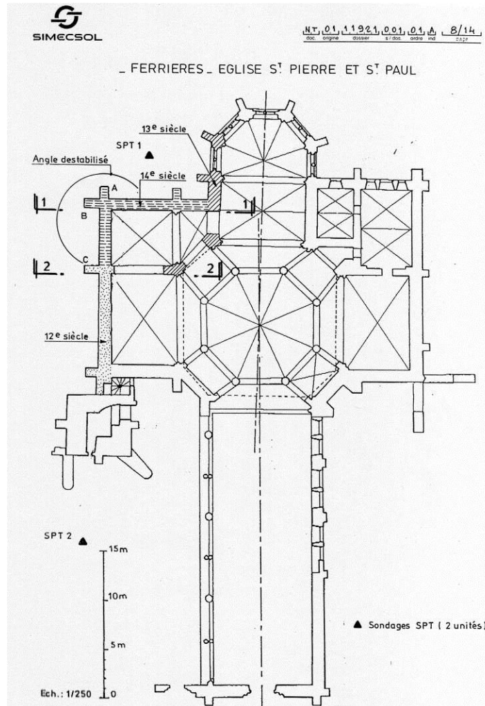
Fig. 8-9 : Plan de localisation et relevés du sondage réalisé en 1998 au nord-est du transept. In : Goubet R., Ferrières-en-Gâtinais (45). Église Saint-Pierre et Saint-Paul. Études de sols. Rapport , 3 juillet 1998, 14 p. (Annexe de l'étude préalable de Jacques Moulin de 1998).
