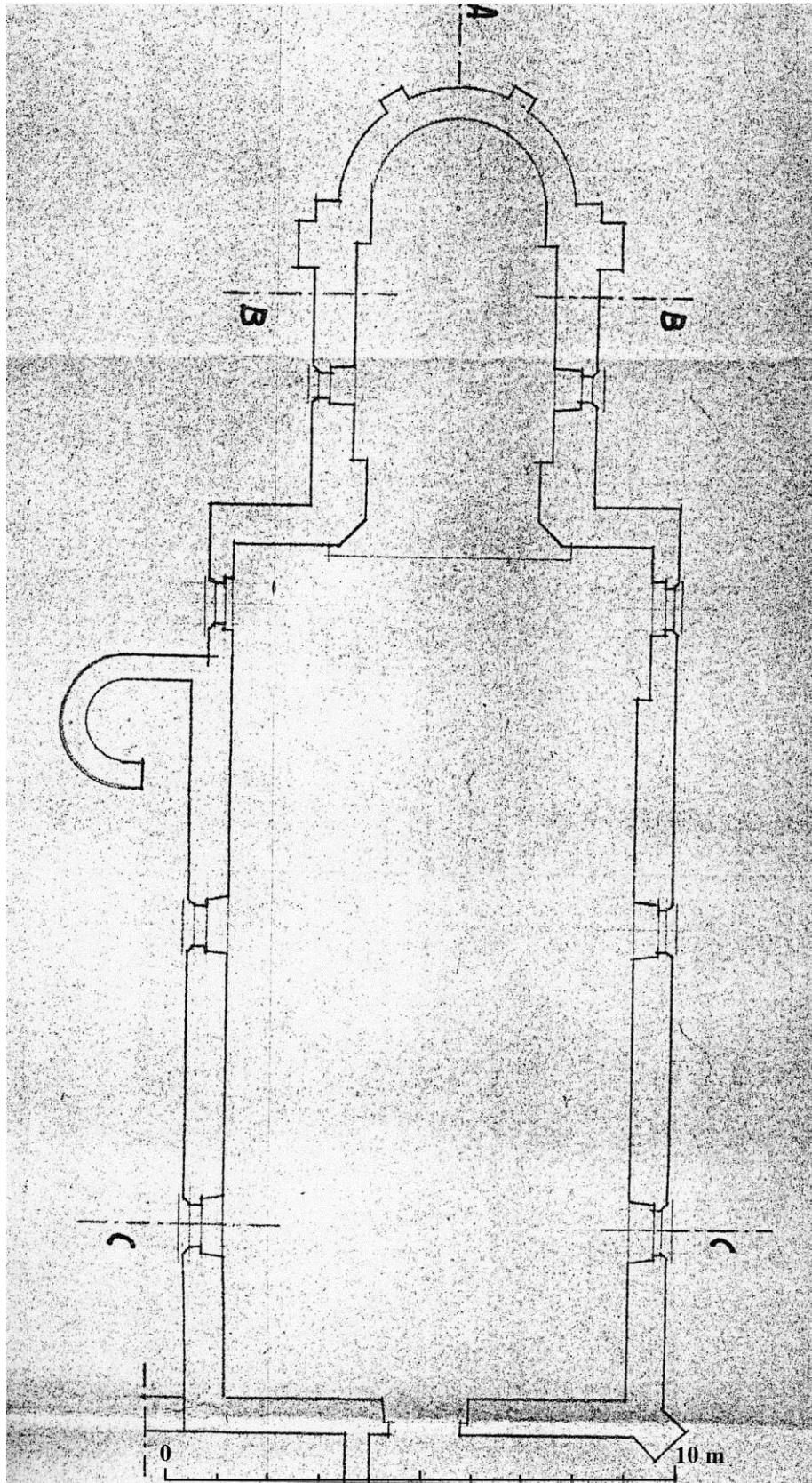
Fig. 7 : Plan de l'église de Saint-Martin-le-Seul.
