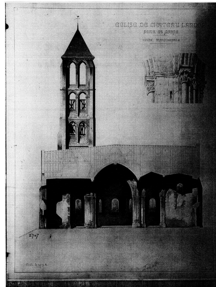
Fig.11 : Coupe transversale. Sauvageot L., Église de Château-Landon. Seine-et-Marne, Coupe transversale , Échelle 0,02, 1890.
