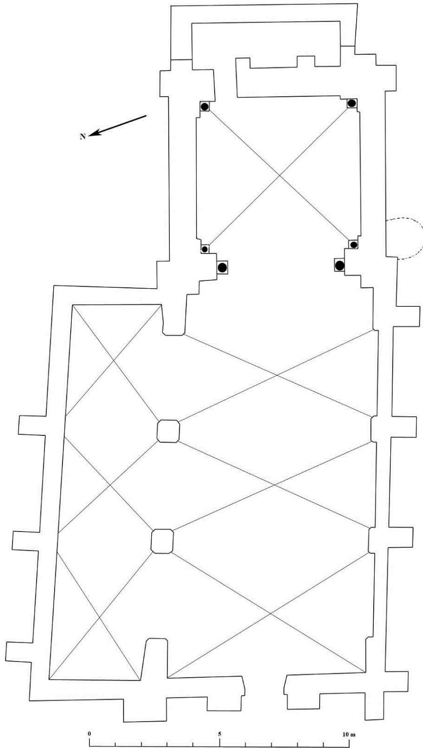
Fig. 4 : Plan de l'église de Charmont-en-Beauce.
