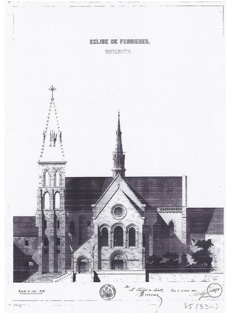
Fig. 11 : Vue de la façade occidentale de l'abbatiale après restauration. Lisch M., Église de Ferrières. Restauration , août 1865, Échelle 1/100 e .
