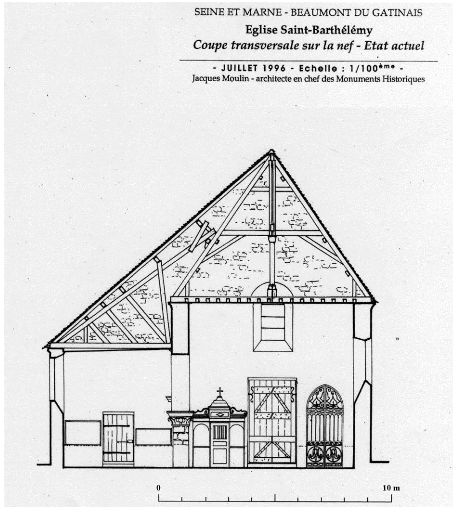
Fig. 14 : Coupe transversale sur la nef. Moulin J., Seine-et-Marne. Beaumont-du-Gâtinais. Église Saint-Barthélémy. Coupe transversale sur la nef. État actuel , Échelle 1/100 e , juillet 1996.
