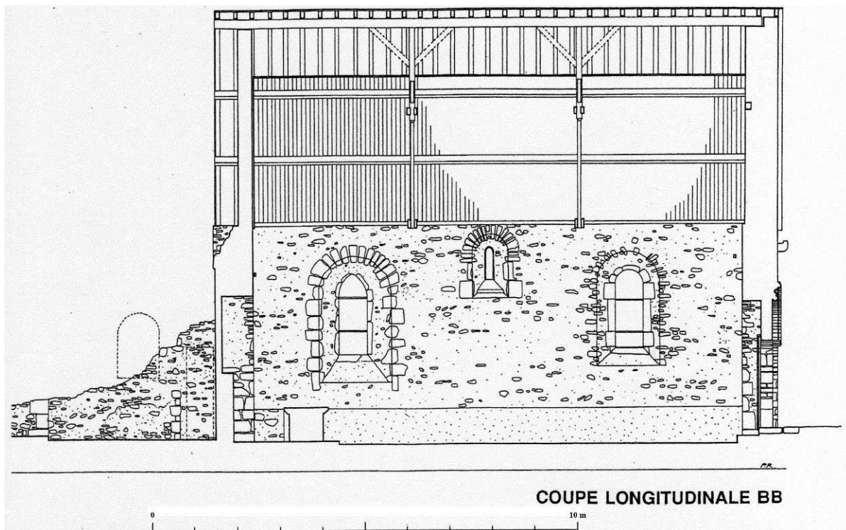
Fig. 13 : Coupe longitudinale, montrant l'élévation intérieure sud. Leriche A., Cortrat (45) – Église Saint-Martin. Restauration de l'église (tranche 1). Coupes , Échelle 1/100 e , décembre 2005.
