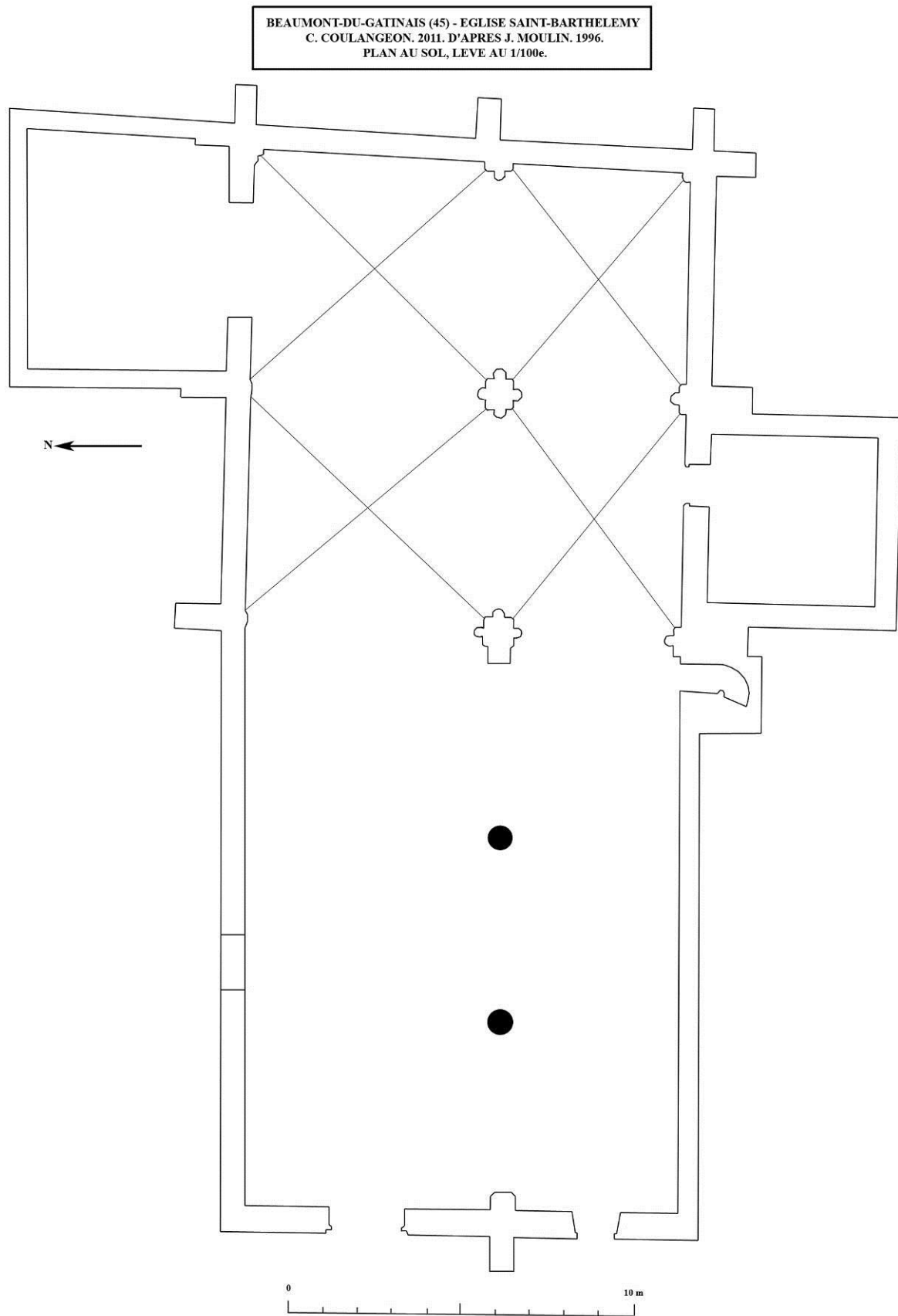
Fig. 5 : Plan de l'église de Beaumont-du-Gâtinais.
