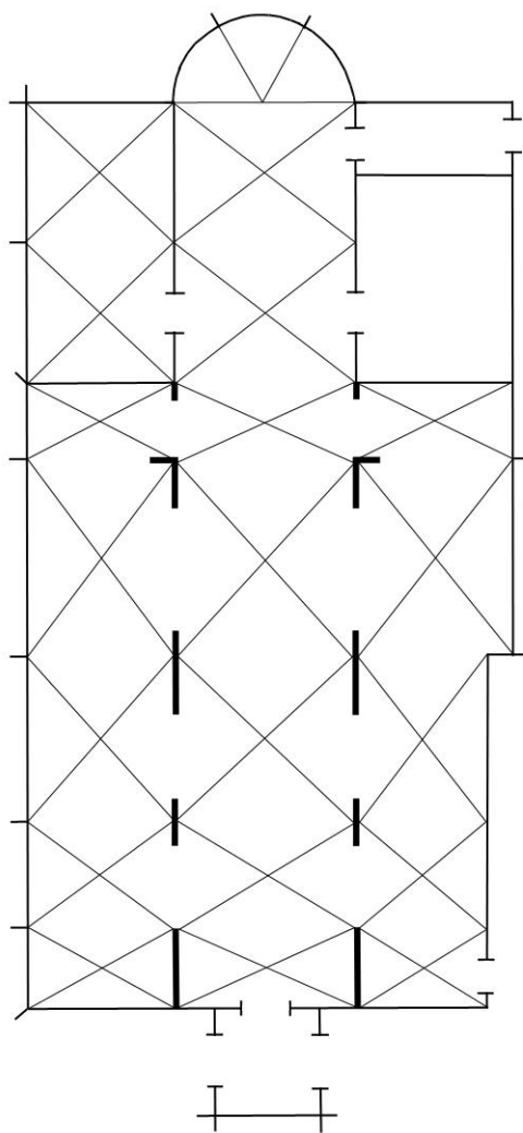
Fig. 3 : Schéma de l'église de Bourron-Marlotte.
