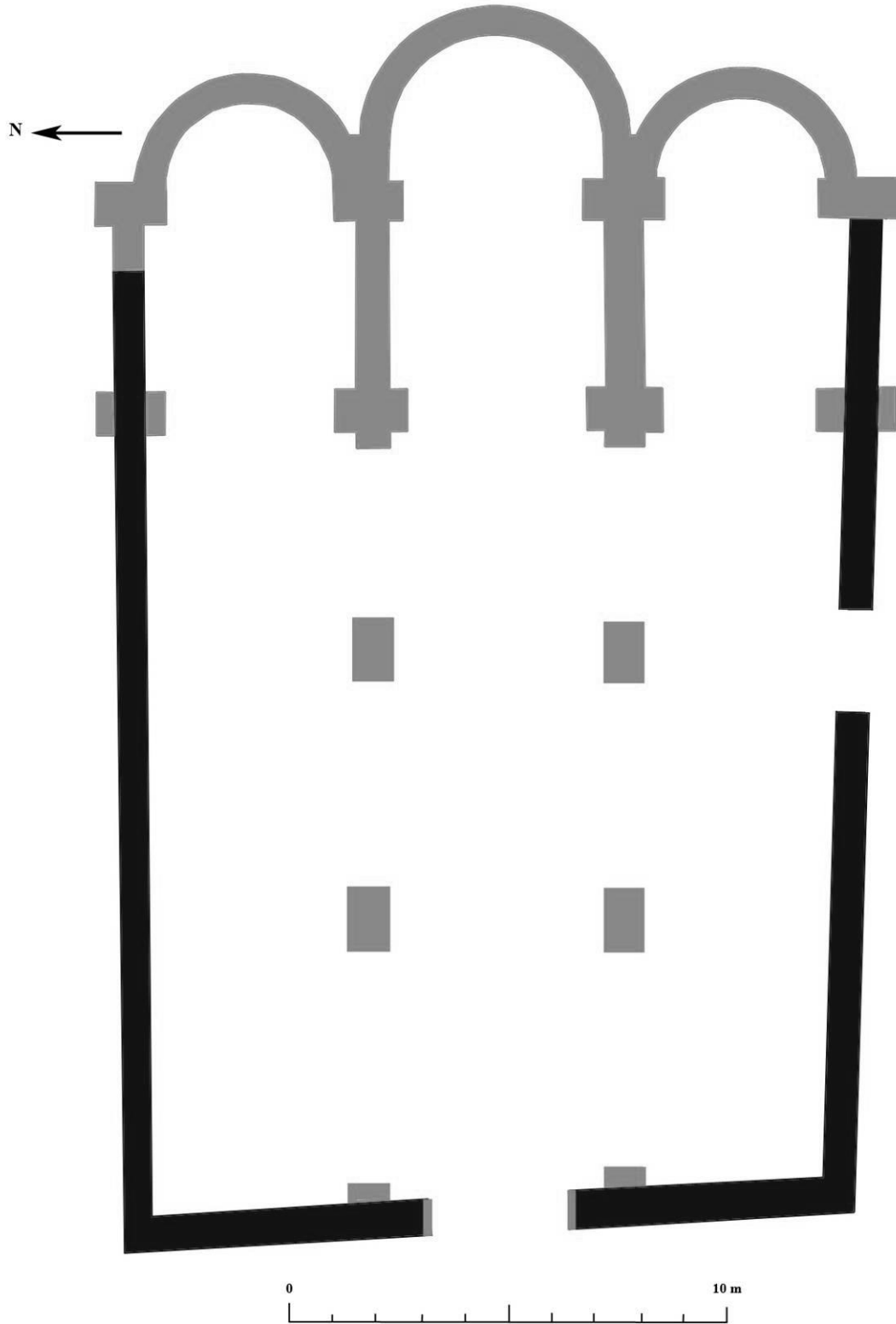
Fig. 7 : Hypothèse pour la restitution du plan de l'église au XI e siècle.
