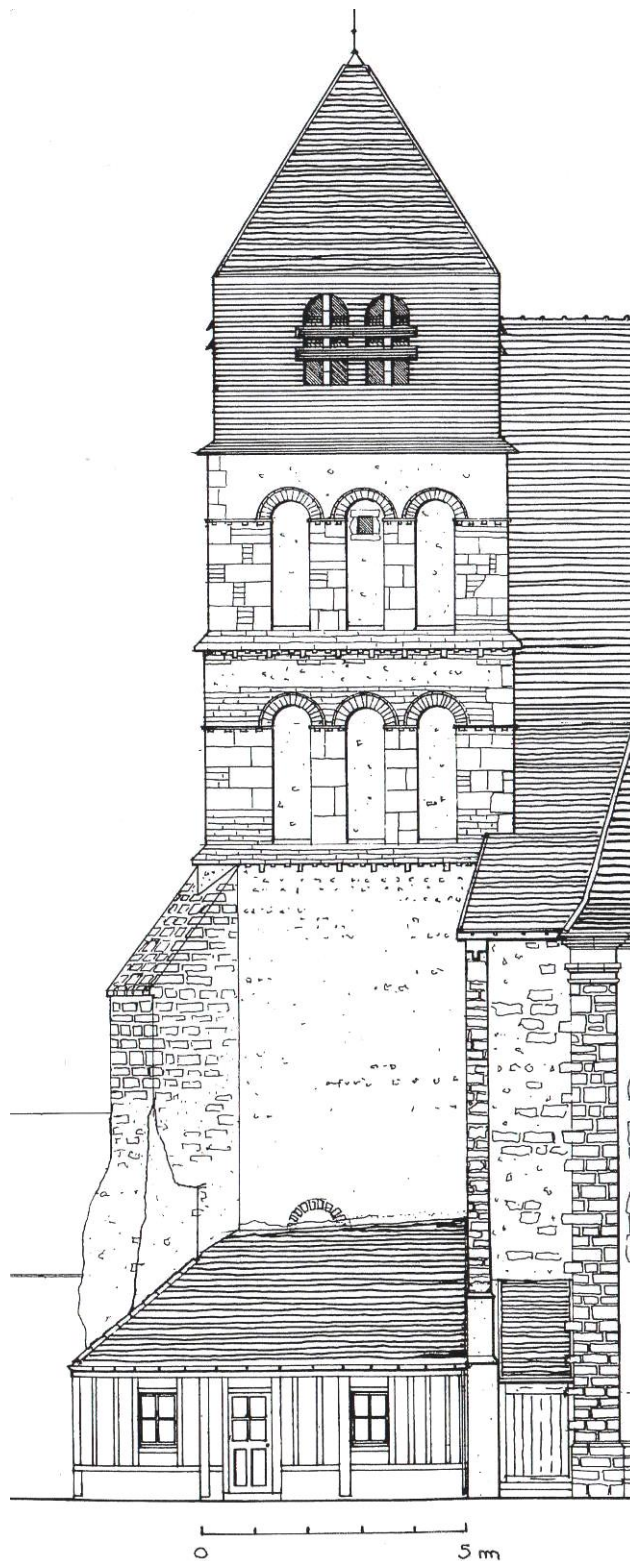
Fig. 10 : Relevé de la façade nord du clocher, avant restauration, par Jacques Moulin. Moulin J., Loiret. Courtenay. Église. Façade nord , Échelle de 1 cm pour 1 m, 1989 (CRMH, DRAC Centre, Orléans, dossiers sur la commune de Courtenay, 45115-1 G1).
