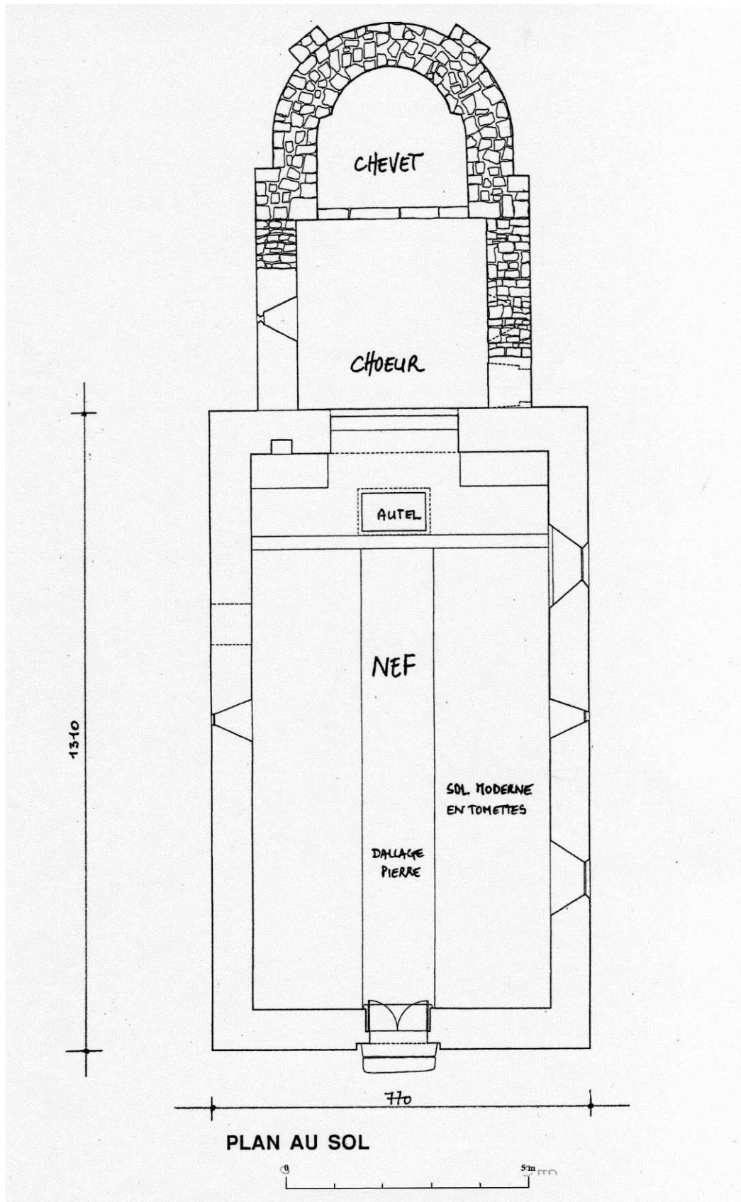
Fig. 7 : Plan de l'église en 2005 par l'architecte Leriche. Leriche A., Contrat (45) – Église Saint-Martin. Restauration de l'église (tranche 1). Plans. État actuel , Échelle 1/100 e , décembre 2005.
