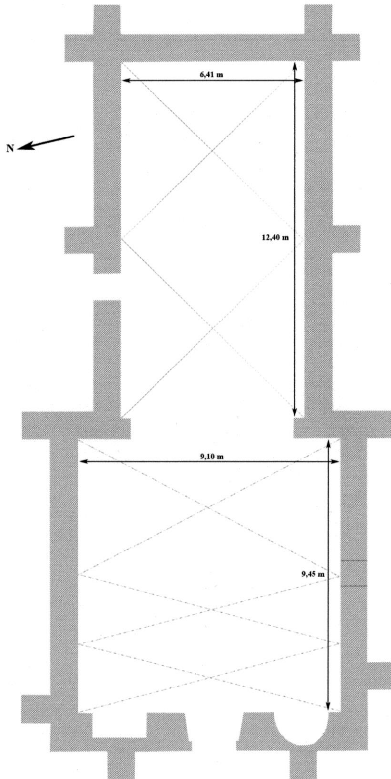
Fig. 3 : Plan schématique de l'église d'Adon.
