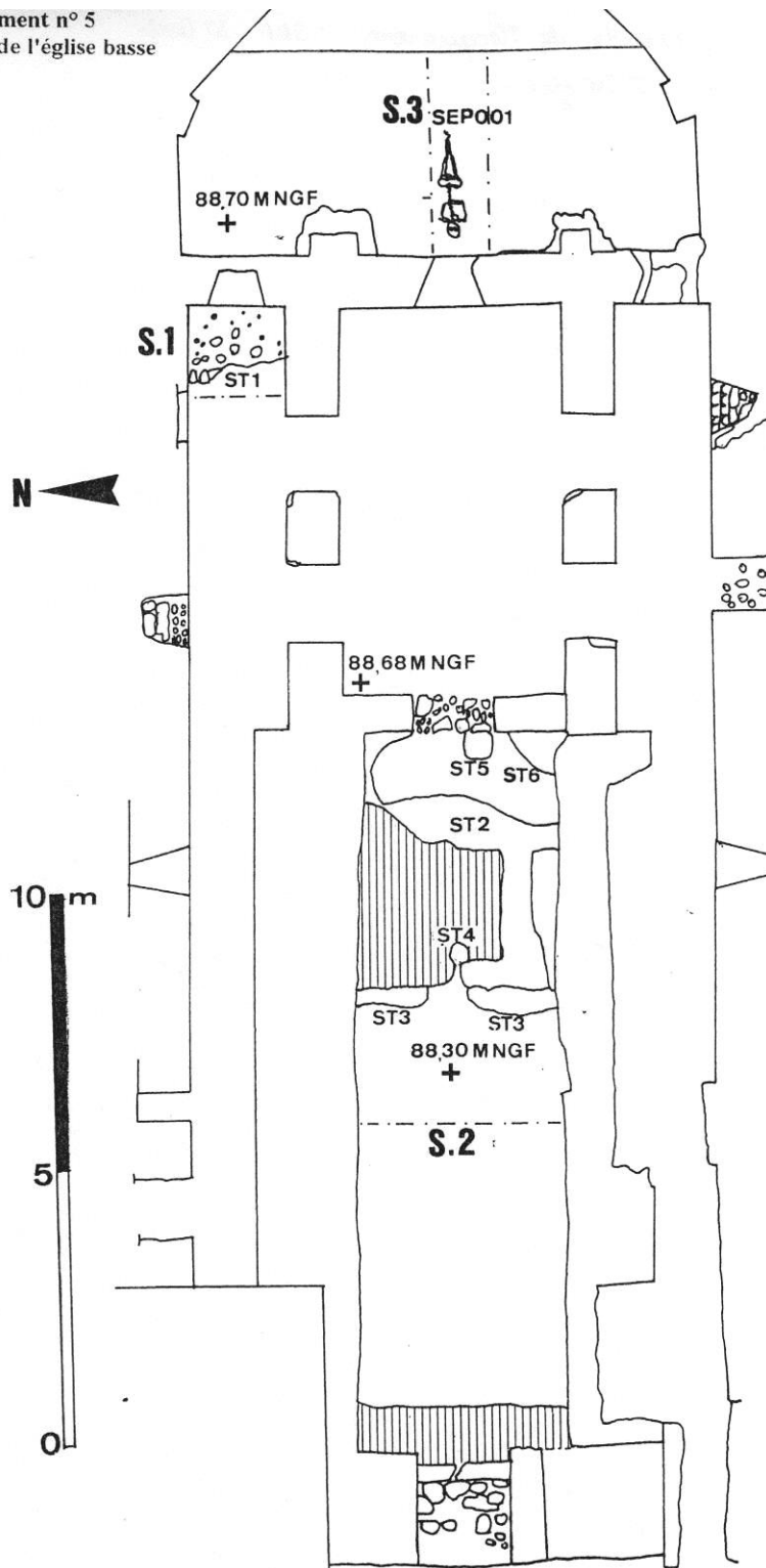
Fig. 16 : Plan de la crypte, levé à l'occasion des fouilles de 1997. In : Mecquenem C. de, Château-Landon (Seine-et-Marne) : D. F. S. Diagnostic archéologique. Ancienne abbaye de Saint-Séverin , 1996, doc. 5.
