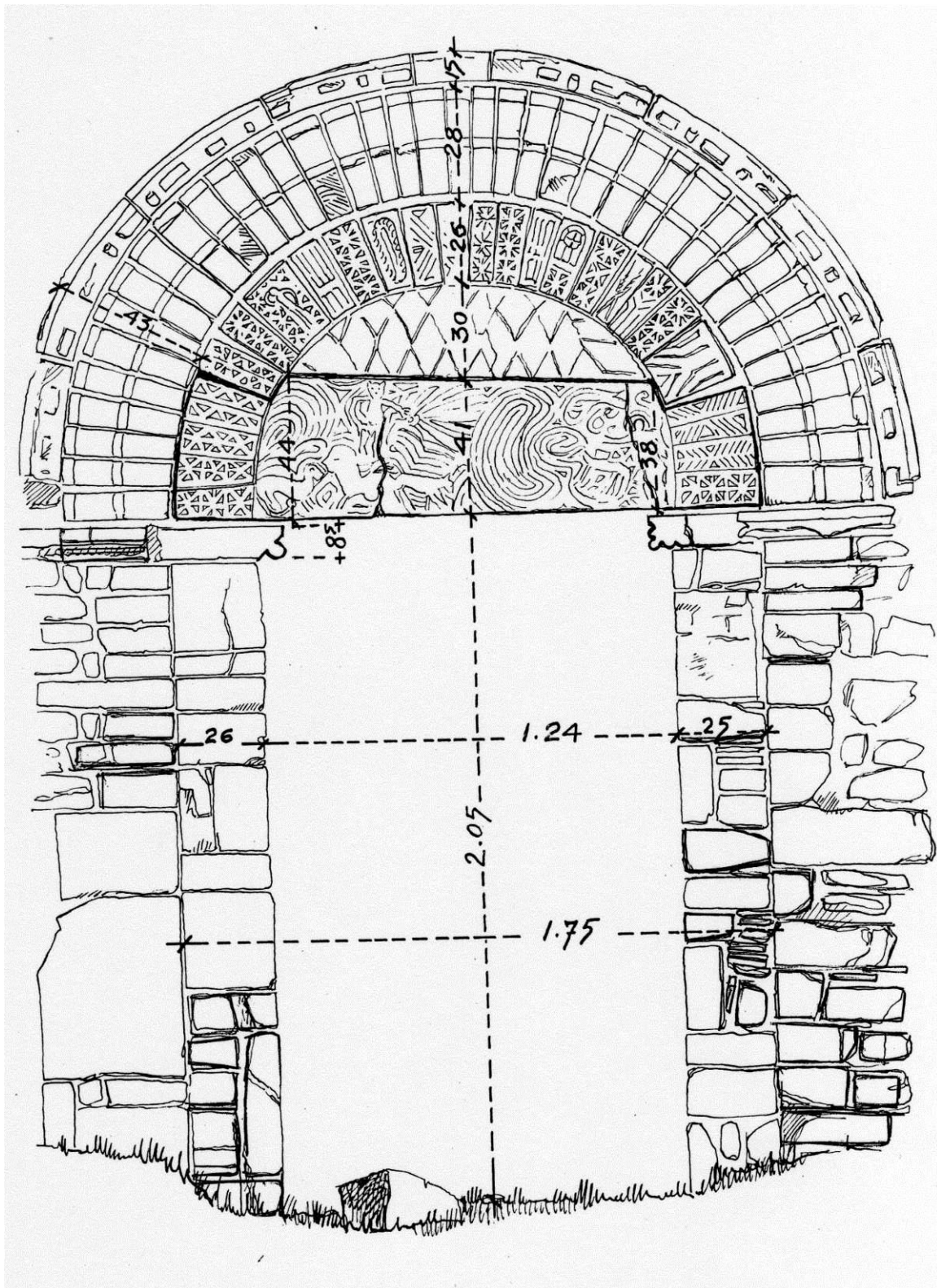
Fig. 16 : Relevé du portail ouest, par Pierre Rousseau.
