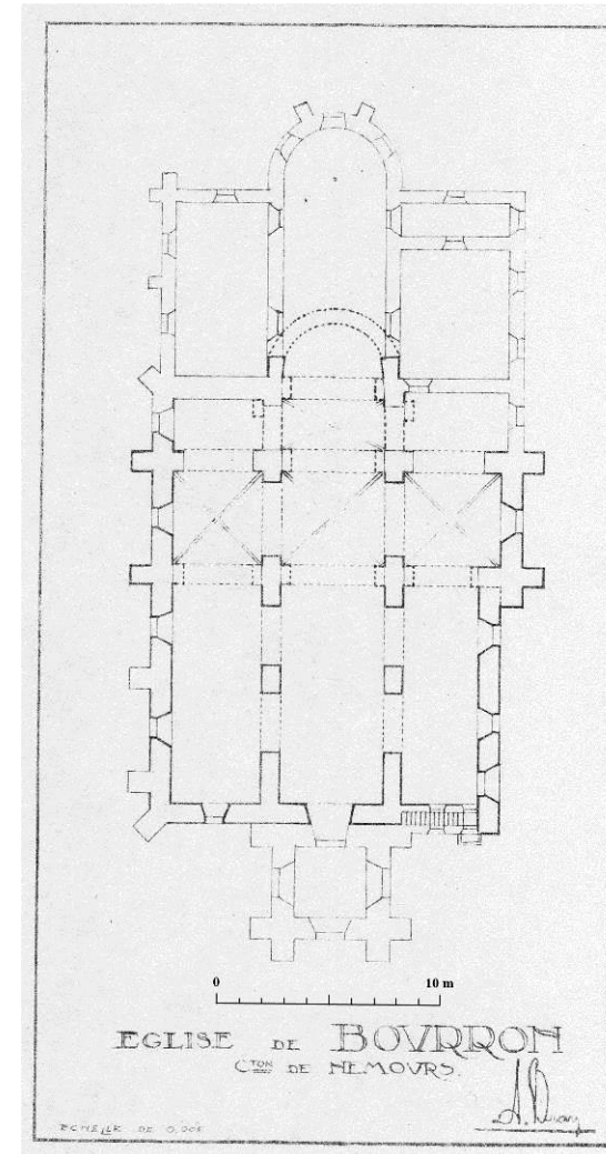
Fig. 8 : Plan de l'église par Albert Bray. Bray A., Église de Bourron. Canton de Nemours, Plan, Échelle au 1/200 e , s. d.
