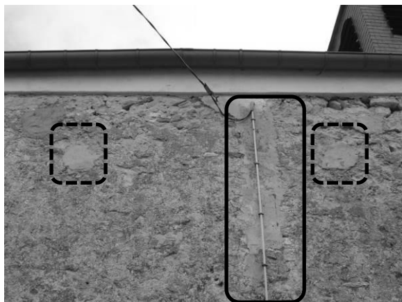
Fig. 25 : Vestiges d'une baie et de trous de boulins bouchés (entourés).
