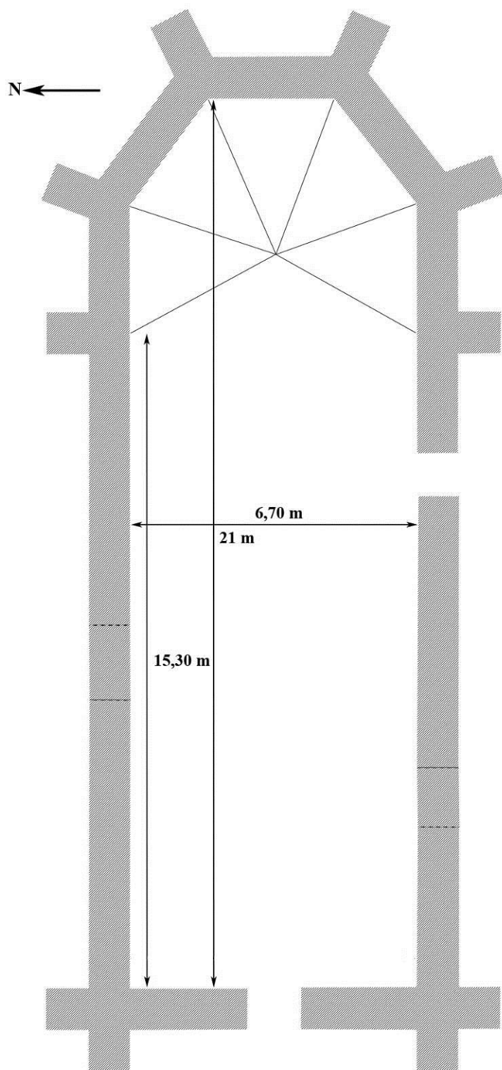
Fig. 4 : Plan schématique de l'église.
