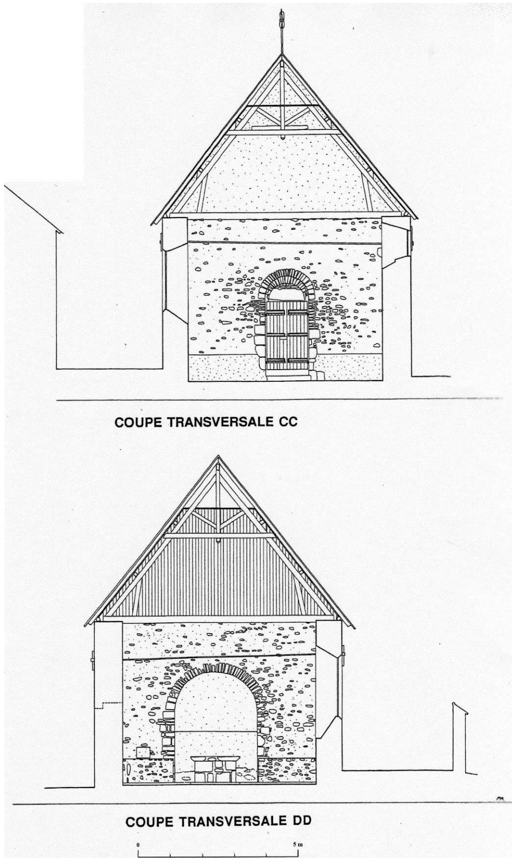
Fig. 14-15 : Coupes transversales, montrant les élévations intérieures ouest et est. Leriche A., Cortrat (45) – Église Saint-Martin. Restauration de l'église (tranche 1). Coupes, Échelle 1/100 e , décembre 2005.
