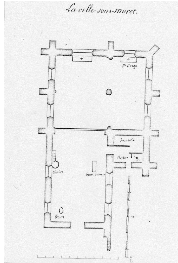
Fig. 6 : Plan de l'église au XIX e siècle.
