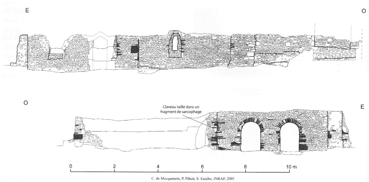
Fig. 23 : Relevés des élévations du couloir d'accès sud de la crypte.
