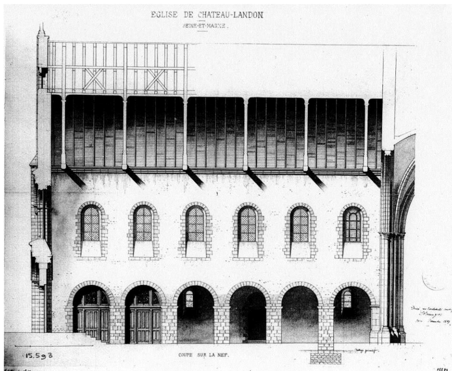
Fig. 13 : Élévation du mur gouttereau nord de la nef.
