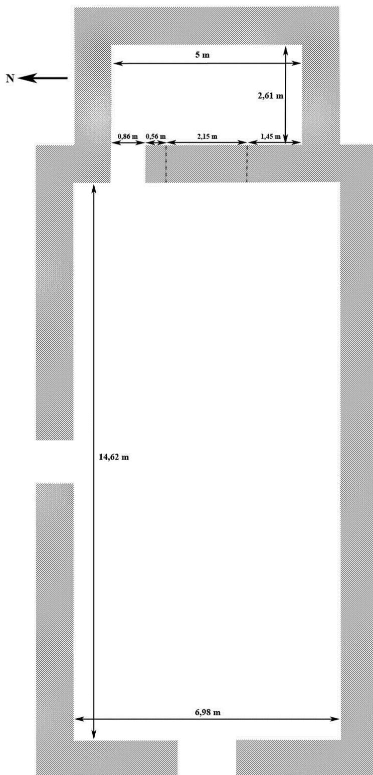
Fig. 4 : Plan schématique de l'église.
