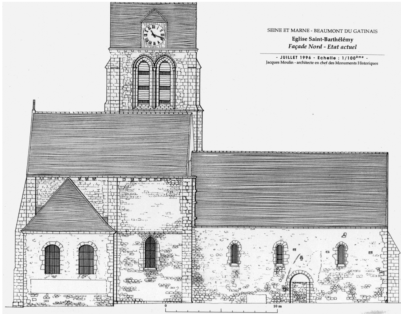
Fig. 11 : Relevé de la façade nord.
