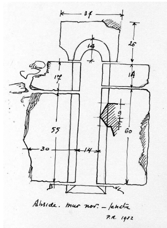
Fig. 17 : Relevé de la baie nord du chevet, par Pierre Rousseau. Rousseau P., Notes, relevés, articles de P. Rousseau et alii , 1957-1971, Médiathèque de l'architecture et du patrimoine, 1999/045/0010.
