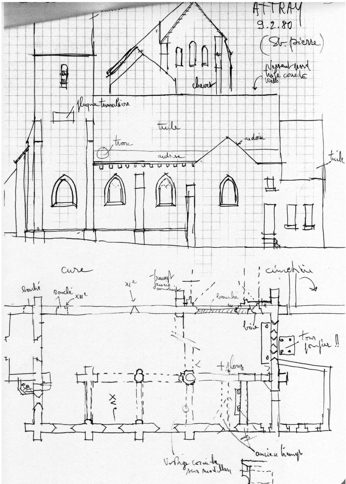
Fig. 5 : Plan et élévation de l'église d'Adon, à main levée. Dessin anonyme du 9 février 1980.
