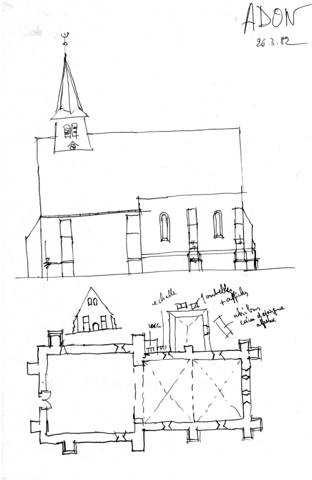
Fig. 4 : Plan et élévation de l'église d'Adon, à main levée. Dessin anonyme du 26 mars 1982.
