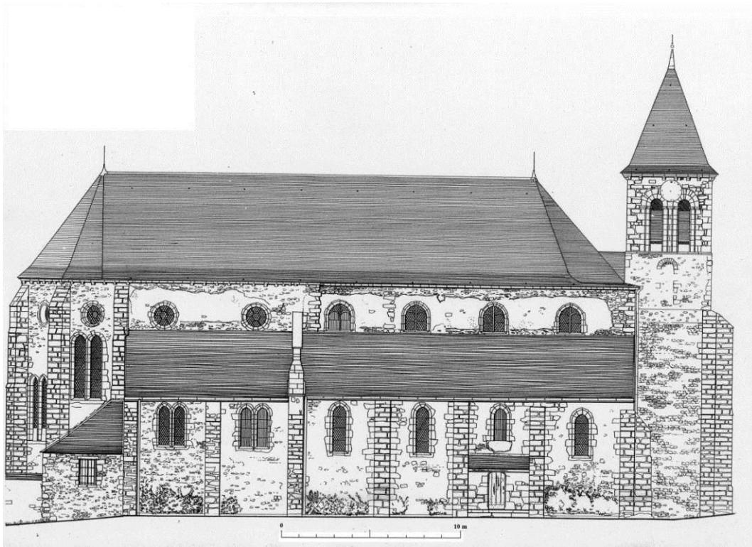
Fig. 7 : La façade nord de l'église.
