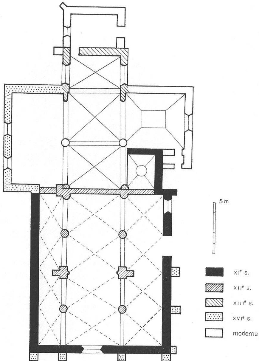
Fig. 9 : Plan phasé de l'église par Anne Prache. In : Prache A., Fleury-en-Bière, Ile-de-France Romane , La Pierre-qui-Vire, éd. du Zodiaque, 1983, p. 399 (La Nuit des Temps 60).
