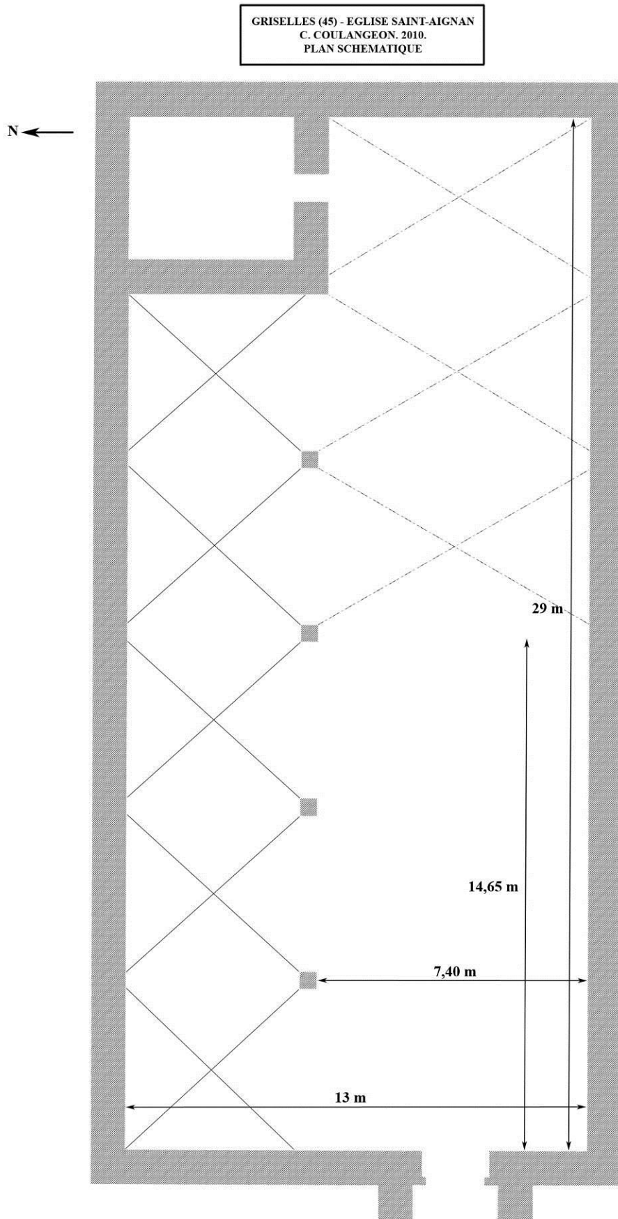
Fig. 5 : Plan schématique de l'église.
