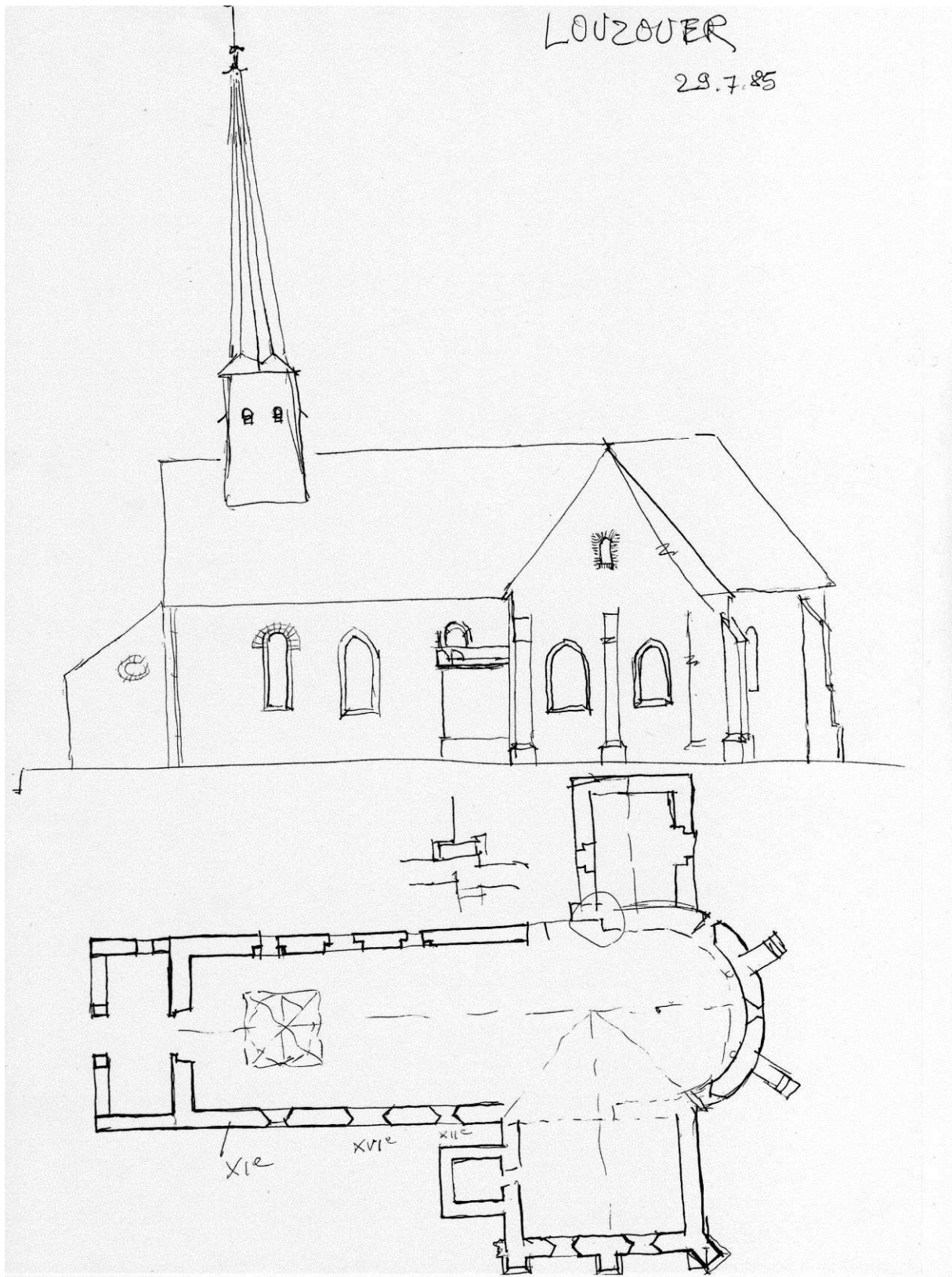
Fig. 5 : Croquis de l'église par un architecte des Bâtiments de France en 1985. In : Louzouer : dossier travaux (Orléans – Service départemental de l'architecture et du patrimoine – Dossier de la commune de Louzouer).
