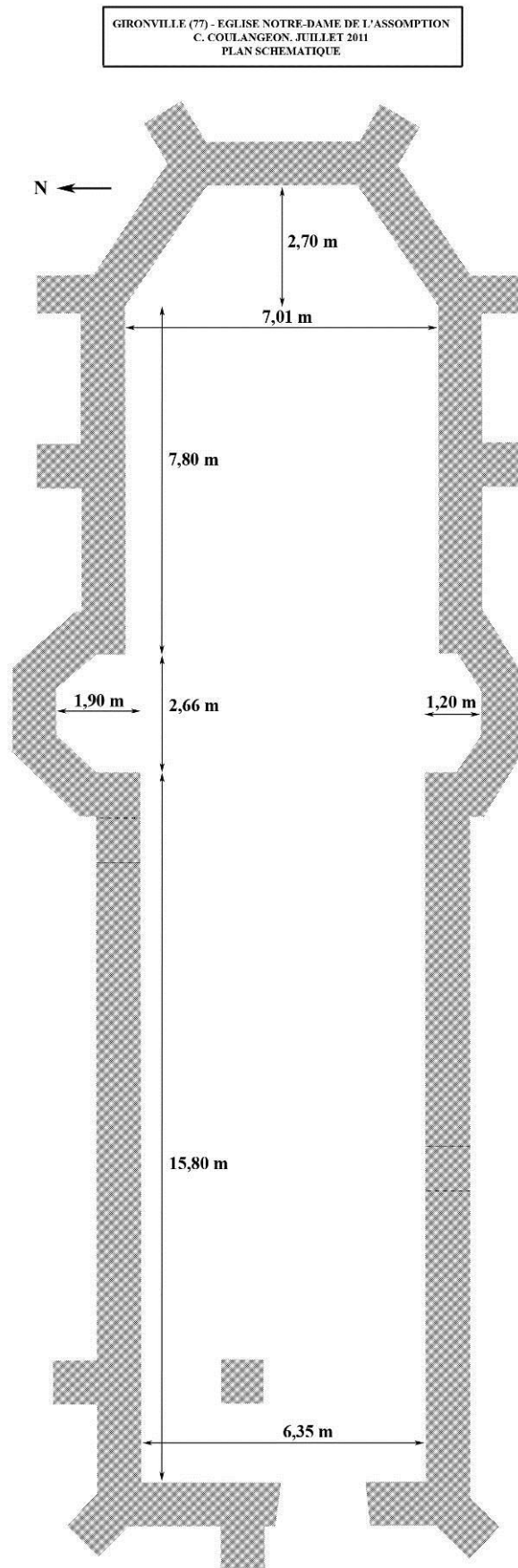
Fig. 4 : Plan schématique de l'église de Gironville.
