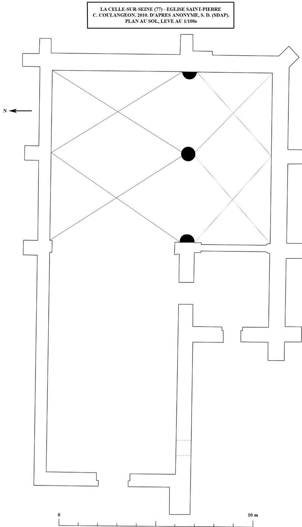
Fig. 4 : Plan de l'église de La Celle-sur-Seine.
