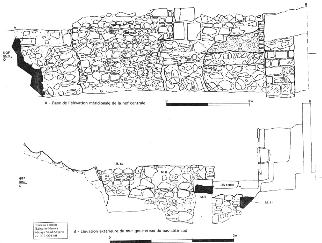
Fig. 28 : Relevés des élévations dans le collatéral sud de la nef. In : Bauchet O., Celly P., Delattre V., Mecquenem C. de, Paccard N., Simonin D., L'abbaye Saint-Séverin, Château-Landon (Seine-et-Marne), D. F. S. de fouille préventive, 1997, pl. XX.
