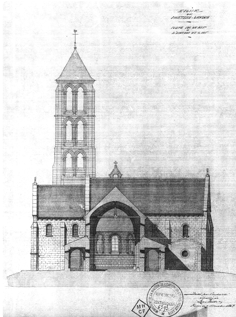
Fig. 8 : Coupe transversale sur la nef, par Millet, en 1863 (projet ?). Millet E., Coupe transversale sur la nef , Échelle 0,005, 1863, Médiathèque de l'architecture et du patrimoine, 0082/077/2007.
