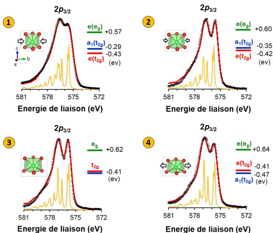
Figure A3. XPS Cr- 2p_{3/2} (cercles noirs évidés) et calculs réalisés par CFM (ligne rouge) pour des films minces de \alpha -Cr 2 O 3 (0001) soumis à une contrainte dans le plan : (1) compression élevée, (2) compression modérée, (3) relaxation complète et (4) tension. Pour chaque spectre, les raies calculées (FWHM = 0,1 eV) sont montrées (ligne jaune), qui ont été convoluées avec une fonction Lorentzienne (FWHM = 0,3 eV) et une fonction Gaussienne (FWHM = 0,7 eV) pour reproduire l'élargissement des raies expérimentales. En regard, la dégénérescence des niveaux 3d est montrée pour chaque cas. Une représentation schématique des distorsions de l'octaèdre CrO 6 est également indiquée.
