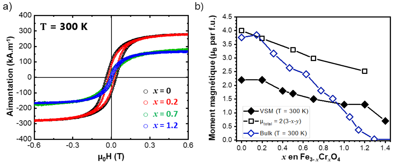
Figure A7. Magnétisme dans les films minces de \text{Fe}_{3-x}\text{Cr}_x\text{O}_4 . (a) Cycles d'hystérésis dans le plan, mesurés par VSM à T = 300 K. (b) Évolution du moment magnétique local en fonction de la composition pour les films minces à T = 300 K en comparaison avec les échantillons massifs (losanges bleus, P. Wasilewski et al. 1975). Les résultats VSM sont représentés par des losanges noirs, tandis que les valeurs déduites de la distribution des sites cationiques (XMCD) sont représentées par des carrés noirs ouverts.
