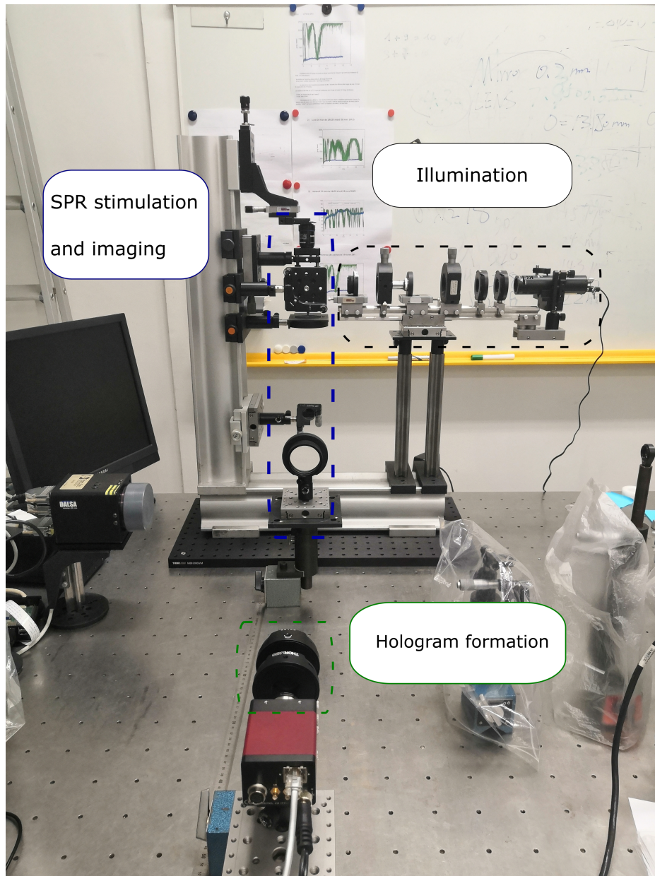
Fig. 3.5 SPR-DHM setup
