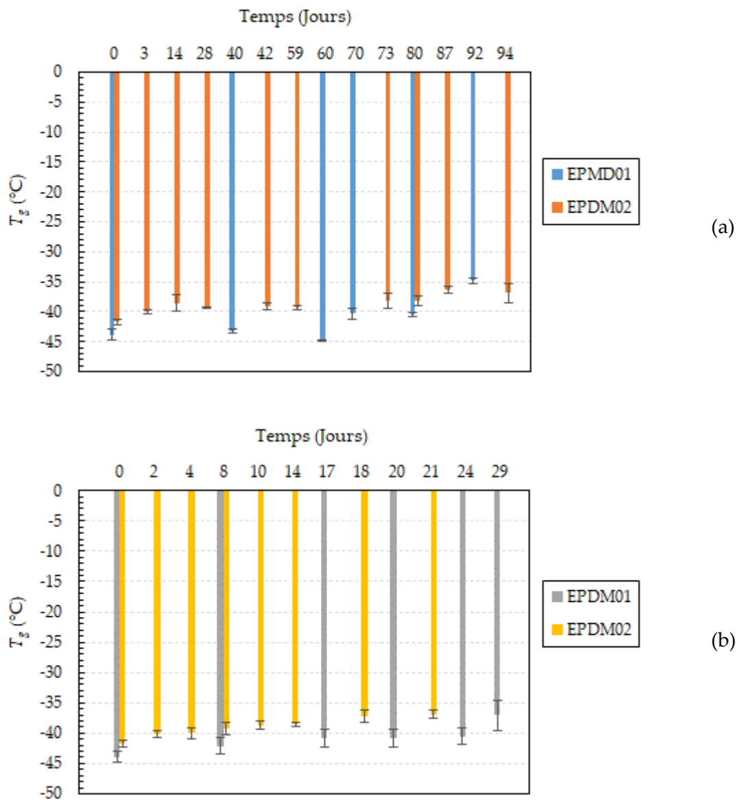
Figure III-17. Évolution de la température de transition vitreuse au cours du vieillissement thermique à 130°C (a) et à 150°C (b).
