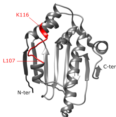
Figure 2.2 : Ci-dessus : séquence de HSP90α-NTD. Les résidus pour lesquels les déplacements chimiques ^{15}\text{N} et H_N ont été attribués sont représentés par un trait vert pour chacune des deux attributions reportées (7003 et 19560). Ceux non attribués sont représentés par un segment rouge. A gauche : structure cristallographique de HSP90-NTD (PDB : 1YES). Le segment rouge correspond aux signaux du squelette invisibles par RMN en raison de la dynamique dans la gamme de temps \mu\text{-ms} et appartenant au segment [L107-K116], localisé à proximité du site de fixation de l'ATP.
