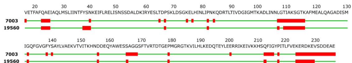
Figure 2.2 : Ci-dessus : séquence de HSP90α-NTD. Les résidus pour lesquels les déplacements chimiques ^{15}\text{N} et H_N ont été attribués sont représentés par un trait vert pour chacune des deux attributions reportées (7003 et 19560). Ceux non attribués sont représentés par un segment rouge. A gauche : structure cristallographique de HSP90-NTD (PDB : 1YES). Le segment rouge correspond aux signaux du squelette invisibles par RMN en raison de la dynamique dans la gamme de temps \mu\text{-ms} et appartenant au segment [L107-K116], localisé à proximité du site de fixation de l'ATP.
