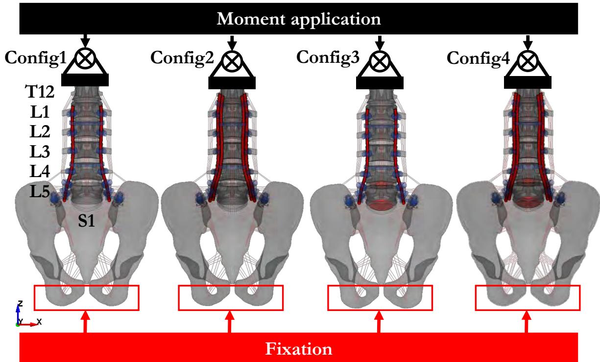
Figure 71 : Schématisation des conditions aux limites appliquées au MEF de la partie lombaire instrumentée. Le bassin a été encasté tandis qu'un moment pur de 7.5 N.m a été appliqué au niveau de T12 en accord avec les expérimentations de Ntilikina et al., 2019a, 2019b lors d'une inflexion latérale.
