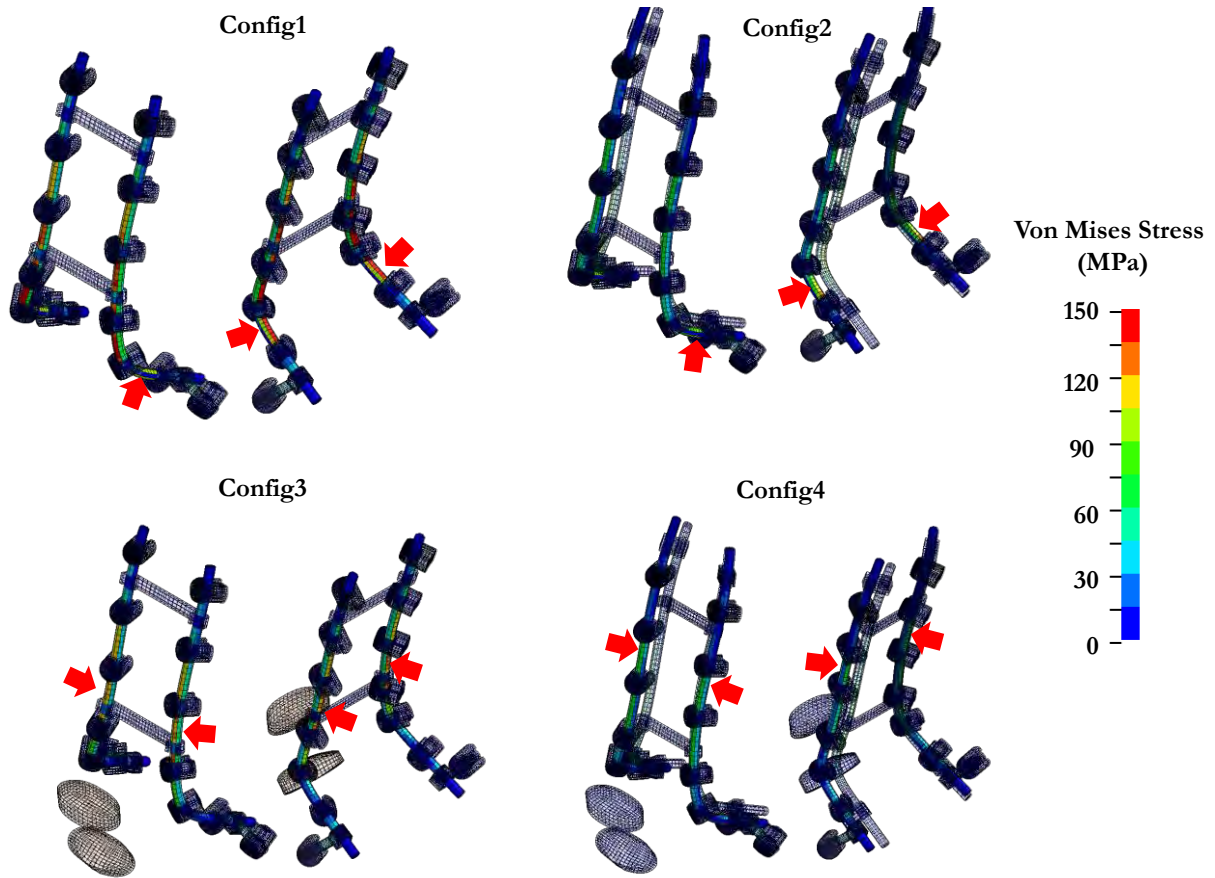
Figure 69 : Illustration de la distribution des contraintes de type von Mises dans la tige principale, lors d'une sollicitation de 7.5 N.m en extension, pour les quatre instrumentations étudiées. Les flèches rouges indiquent la localisation des maxima de contrainte de von Mises.
