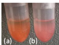
Figure 63 : (a) CPG-NP-ADIBO/NH 2 et (b) CPG-NP-ADIBO/DOTA-NHS en suspension ayant réagi avec la FITC-NCS.
