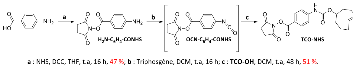
Schéma 16 : Synthèse du TCO-NHS.
