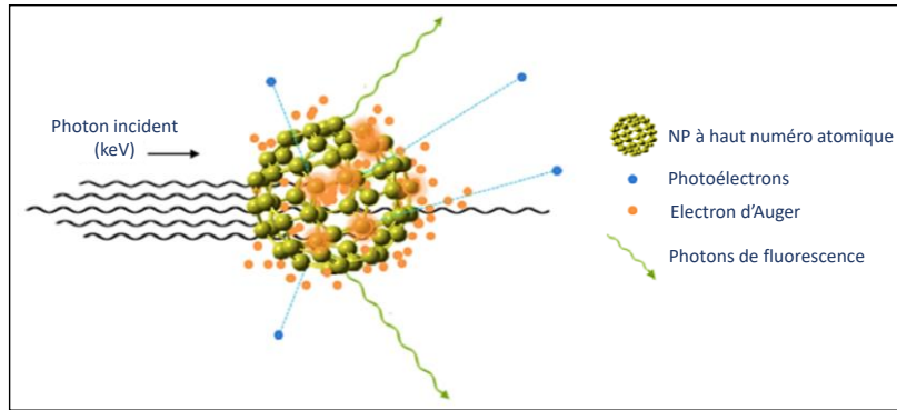
Figure 22 : Processus d'interaction des photons (KeV) avec des NP à haut numéro atomique. Adaptée de Kuncic et Lacombe, 2018 [178].
