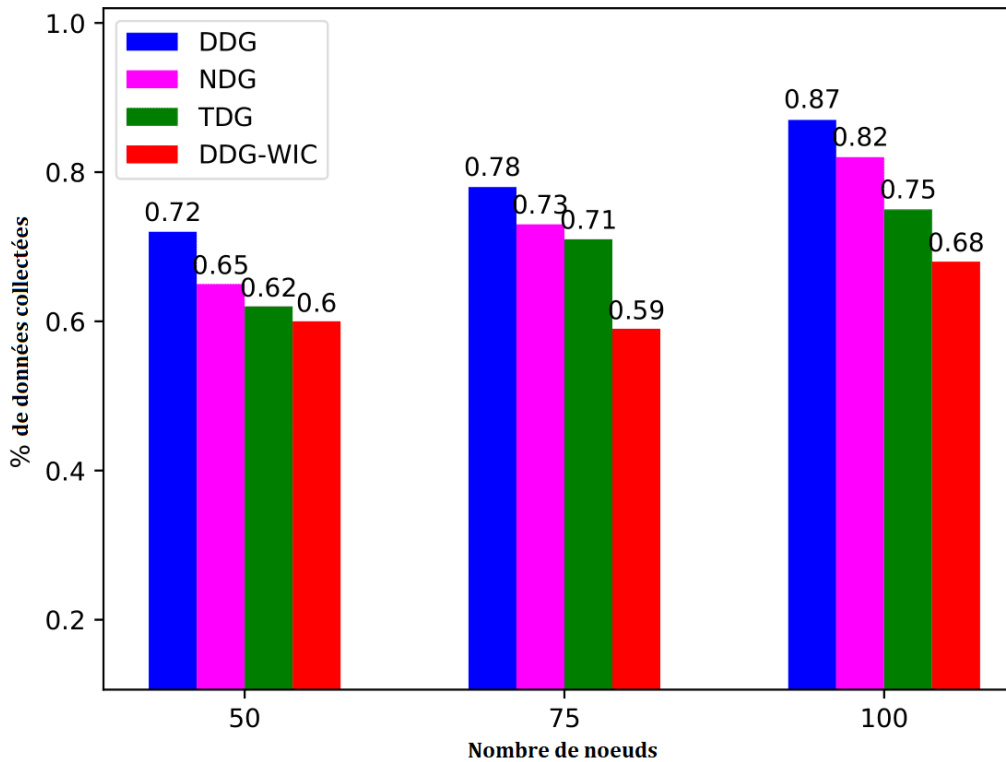
FIGURE 5.8 – Quantité de données récoltée VS nombre de noeuds capteurs
