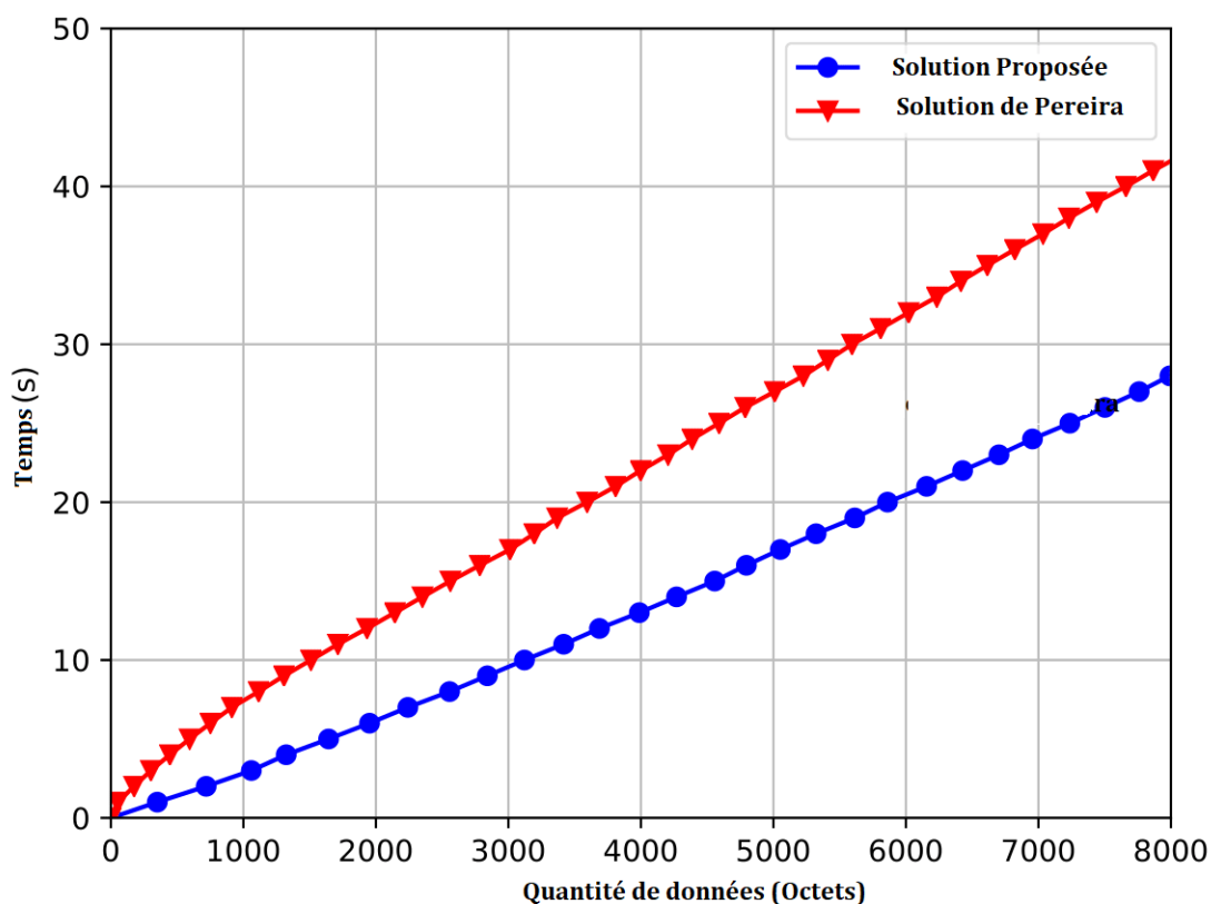
FIGURE 4.2 – Temps Vs Quantité de données
