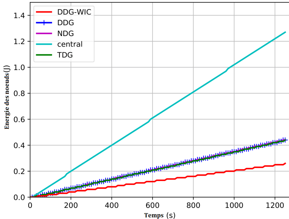
FIGURE 5.11 – Consommation d’énergie des noeuds capteurs
