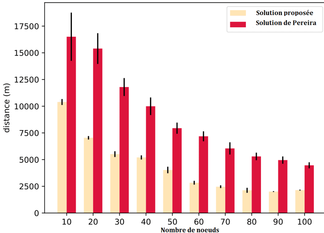
FIGURE 4.5 – Nombre de noeuds capteurs vs distance parcourue
