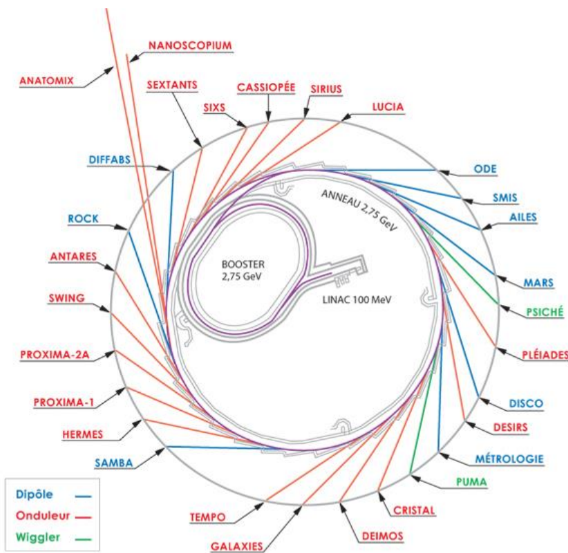
Figure II-11 : Schéma du synchrotron SOLEIL avec ses différentes lignes de lumière (SOLEIL, 2019b).
