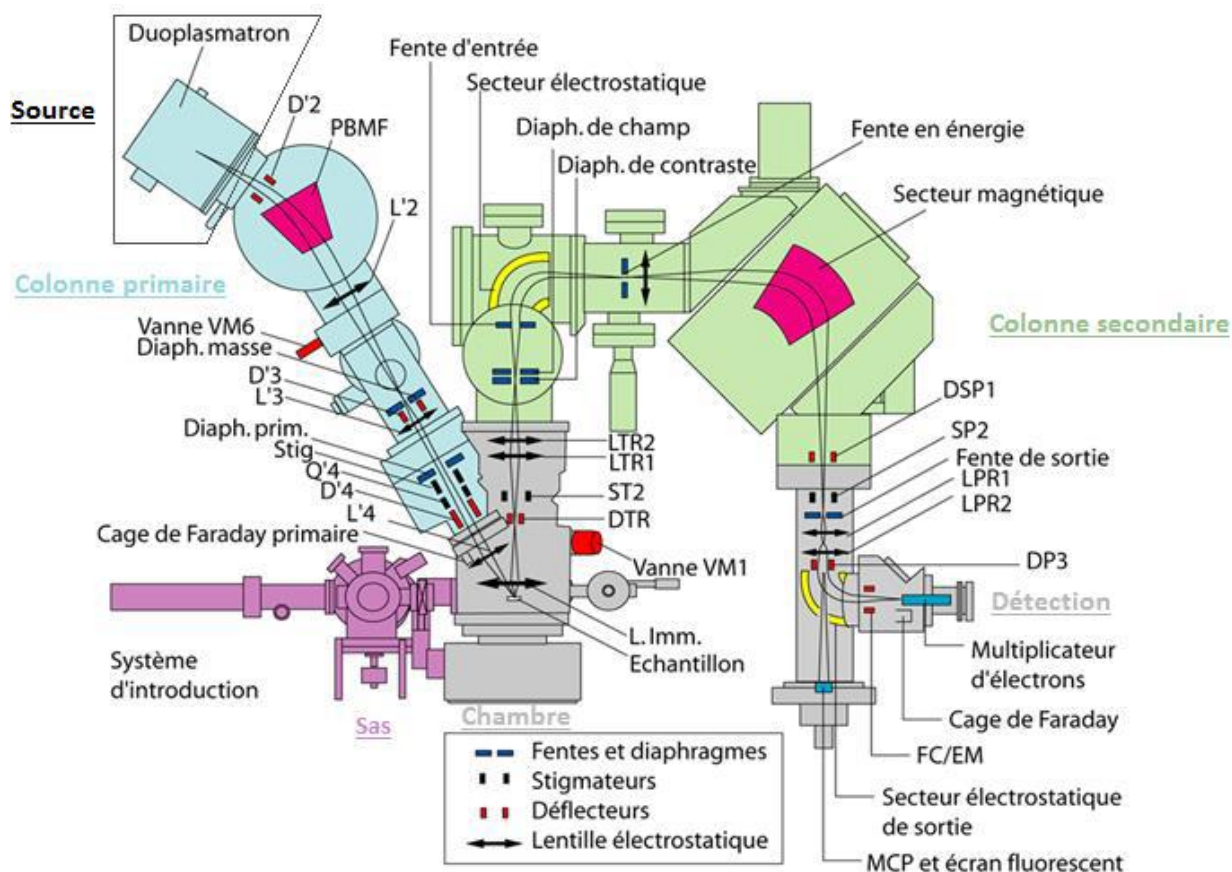
Figure II-12 : Schéma du SG-SIMS 7f de Cemea (d'après un document Cemea).
