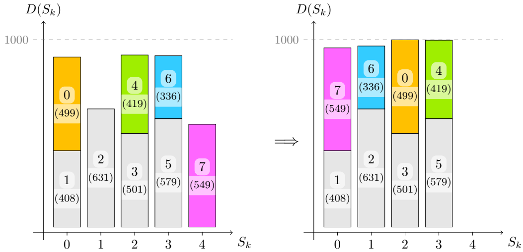
FIGURE 4.7 – Solution initiale (gauche) et solution obtenue après le mouvement \mathcal{M}_{chain} version « chaîne d'éjection » (droite)
