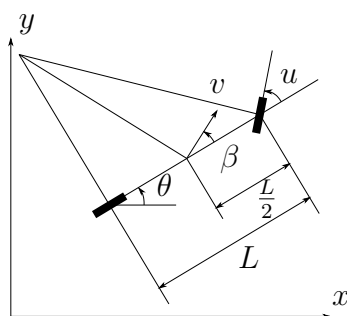
FIGURE 3.13 – Modèle bicyclette.
