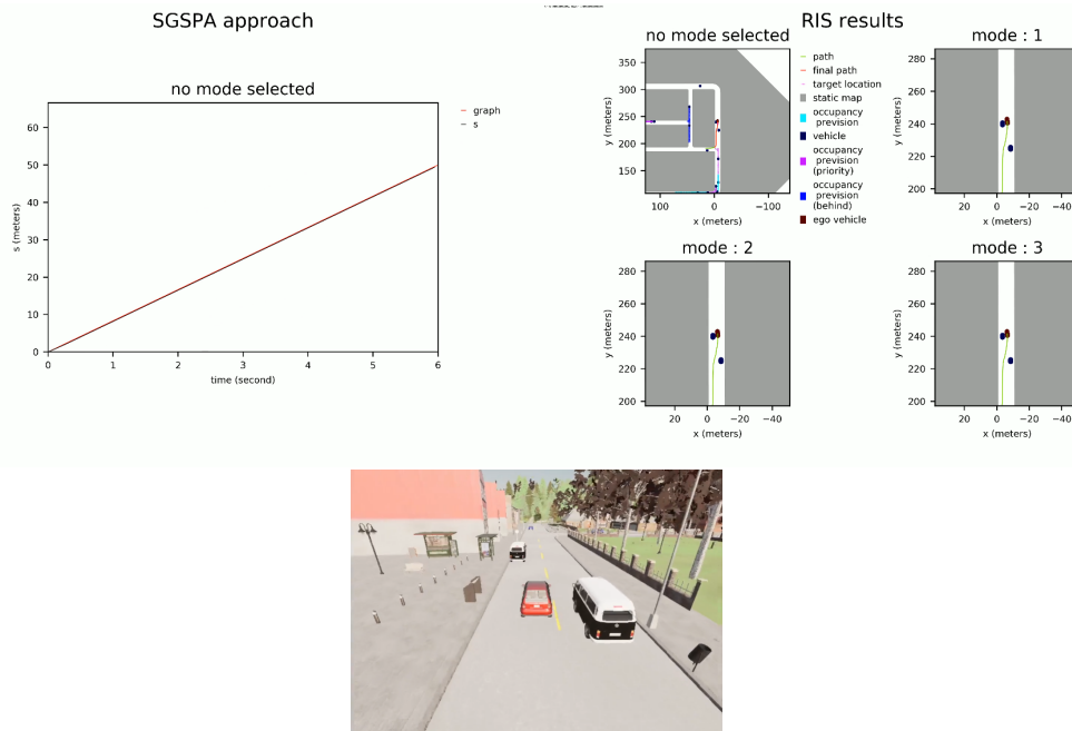
FIGURE 4.28 – Scénario avec deux véhicules arrêtés sur la voie. Fin du dépassement.
