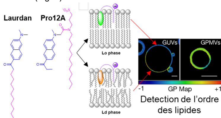
Fig. 4. Structure et mécanisme de détection de la sonde Pro12A.
