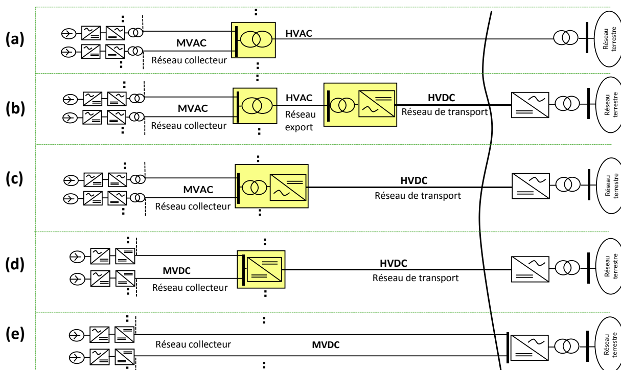
Figure 1: Principes d'architecture de raccordement sélectionnés dans la thèse
