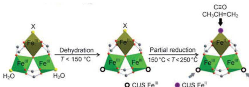
Figure 1.15 : Processus schématique de l'impact de la réduction du trimère de fer du MIL-100(Fe), pour la génération de sites acides au sens de Lewis. Reproduit à partir de [3].
