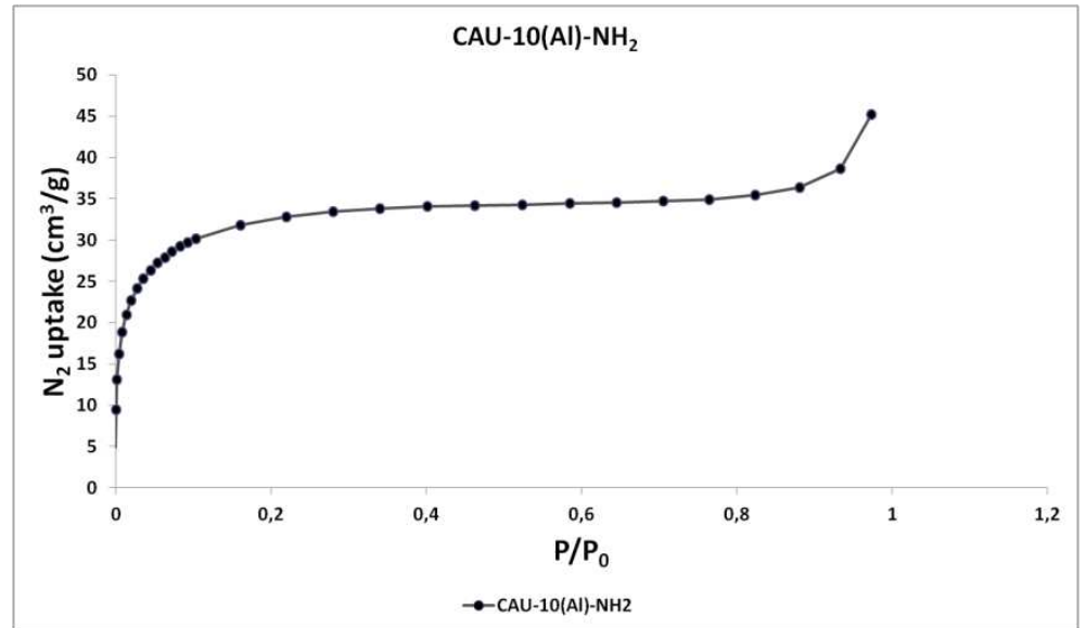
Figure A.42 : Adsorption/désorption de N 2 du CAU-10-NH 2 .
