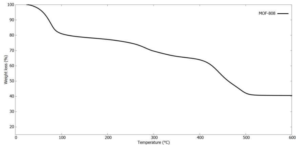
Figure A.17 : Analyse thermogravimétrique du MOF-808.
