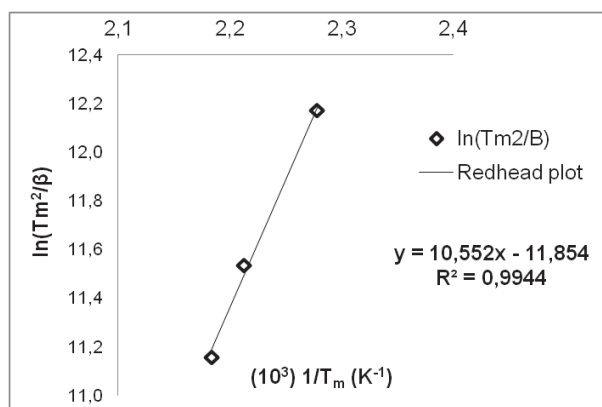
Figure A.64 : Tracé de Redhead (dans le cas d'une désorption d'ordre un, 1/T_m en fonction de \ln(T_m^2/\beta) ), pour la désorption du formaldéhyde ( D_2 ).
