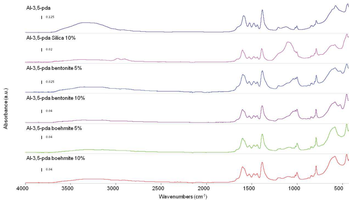
Figure A.51 : Spectres FTIR des échantillons Al-3.5-PDA mis en forme avec différents liants.
