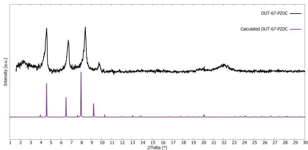
Figure A.34 : Analyse par diffraction des rayons X du Zr-DUT-67-PZDC.
