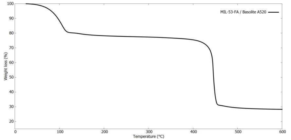
Figure A.11 : Analyse thermogravimétrique du MIL-53-FA.
