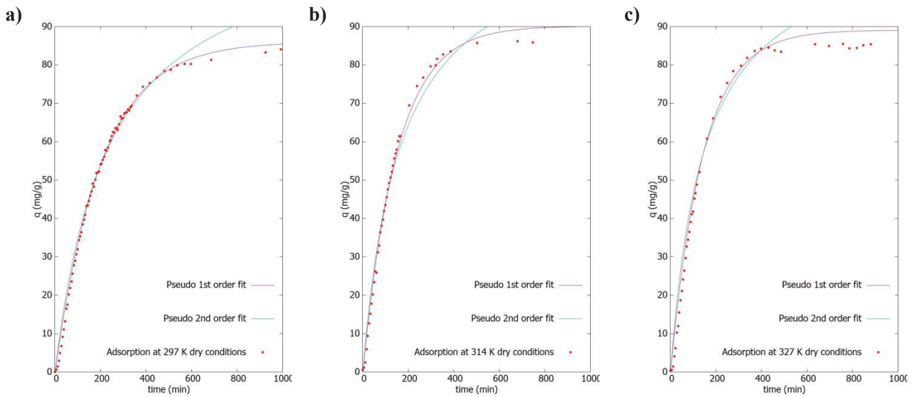
Figure 4.12 : Application des modèles du pseudo-1 er ordre et du pseudo-2 nd ordre pour l'adsorption du formaldéhyde par un échantillon Al-3.5-PDA dans un cas d'atmosphère anhydre a) à 297 K, b) à 314 K, c) 327 K. Réalisée en utilisant GNUPLLOT [10].
