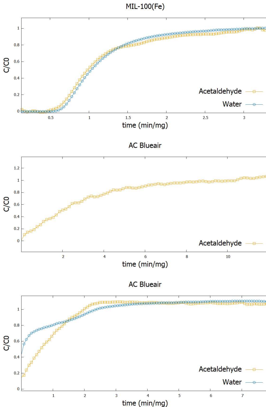
Figure 2.19 : Courbes de percée dans les cas d'adsorption d'acétaldéhyde et de co-adsorption d'eau et d'acétaldéhyde. Axe des abscisses : rapport temps par la quantité de matériau anhydre utilisée. Axe des ordonnées : rapport de la concentration du gaz efflué par la concentration de la charge.
