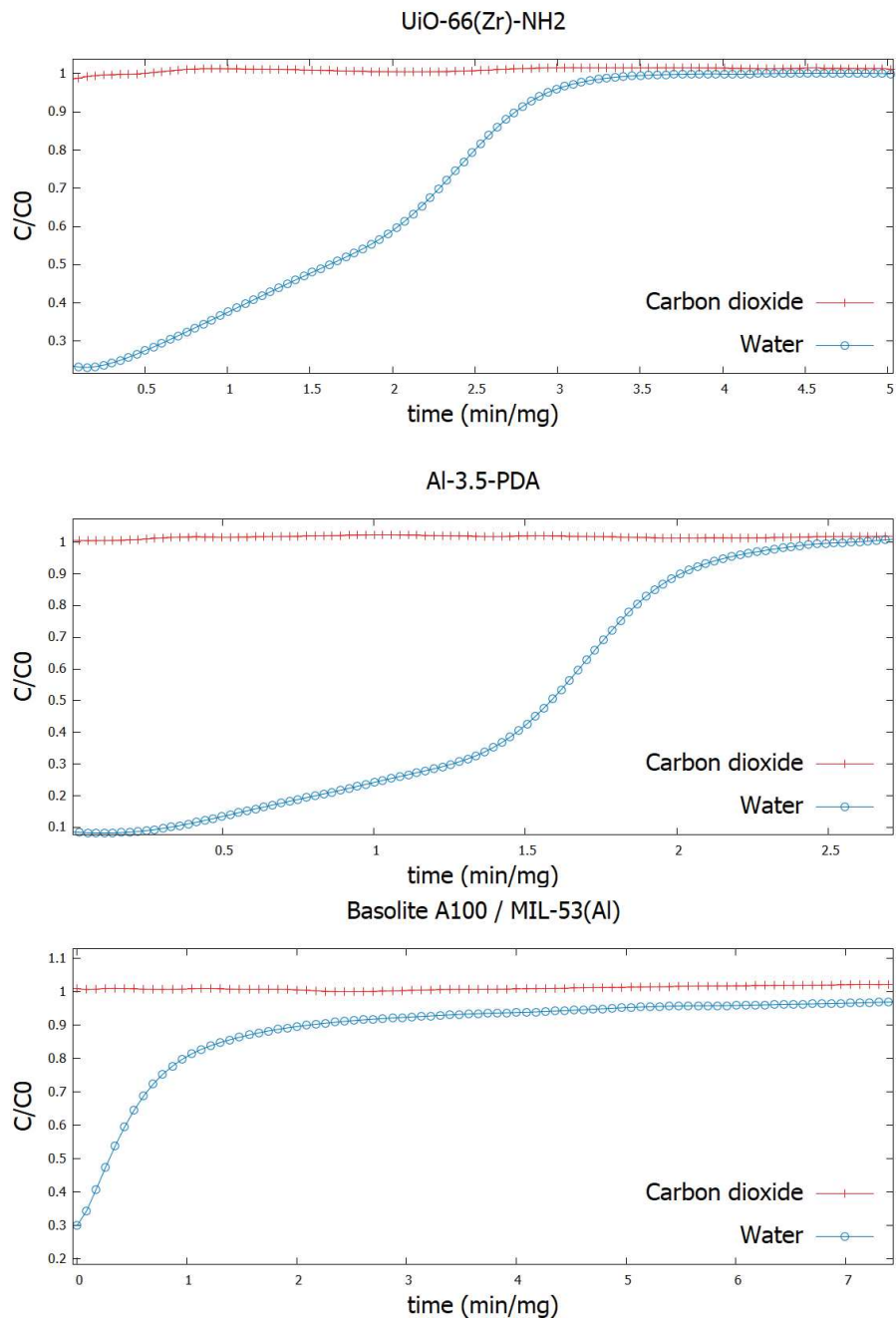
Figure 2.23 : Courbes de percée dans les cas de co-adsorption de dioxyde de carbone et d'eau. Axe des abscisses : rapport temps par la quantité de matériau anhydre utilisée. Axe des ordonnées : rapport de la concentration du gaz effluent par la concentration de la charge.
