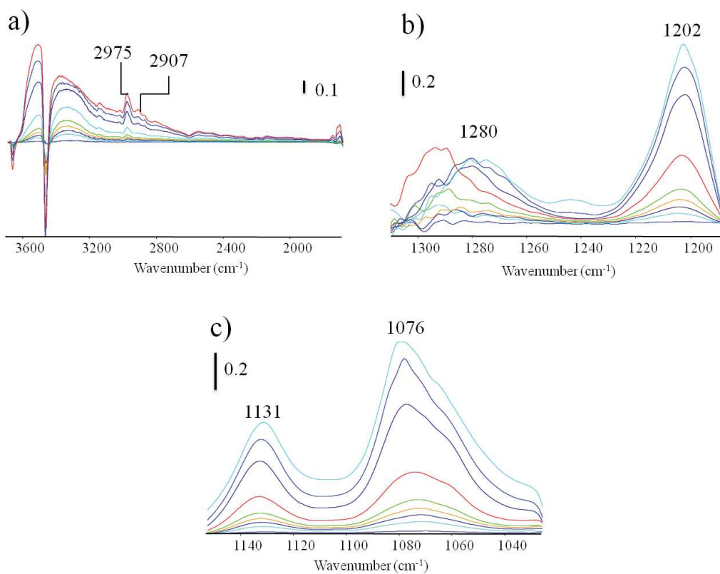
Figure 3.16 : Spectres FTIR lors de l'adsorption de formaldéhyde sur le solide DUT-67(Zr)-PZDC (avec soustraction du spectre de l'échantillon activé) a) dans la région spectrale 3675-1700 \text{cm}^{-1} , b) 1350-1180 \text{cm}^{-1} , c) 1160-1020 \text{cm}^{-1} .
