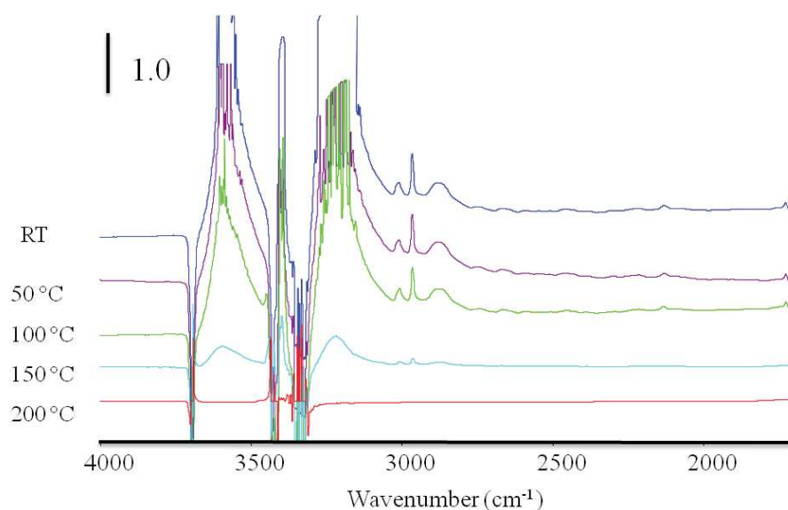
Figure A.62 : Spectres FTIR obtenus lors de la régénération thermique de l'Al-3.5-PDA dans la région spectrale 4000-1700\text{ cm}^{-1} ; de haut en bas : spectres de référence après saturation du formaldéhyde (à RT °C), 50 °C, 100 °C, 150 °C, 200 °C (en évacuation) (avec soustraction du spectre de l'échantillon).
