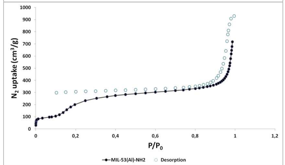
Figure A.27 : Adsorption/désorption de N 2 du MIL-53 et MIL-53- NH 2 .
