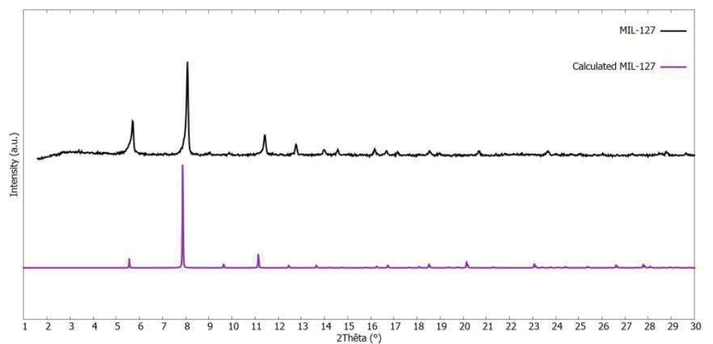
Figure A.4 : Analyse par diffraction des rayons X du MIL-127(Fe).
