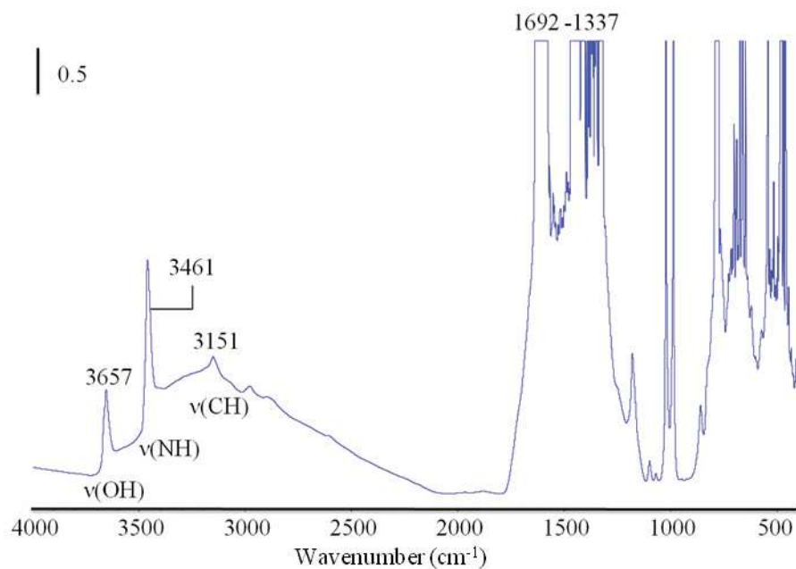
Figure 3.15 : Spectre FTIR du DUT-67(Zr)-PZDC après activation thermique.
