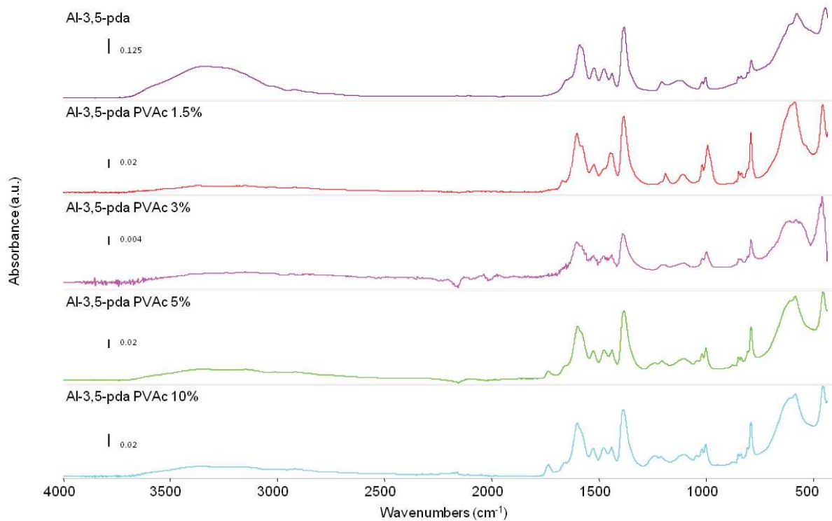
Figure A.50 : Spectres FTIR des échantillons Al-3.5-PDA mis en forme avec différents liants.
