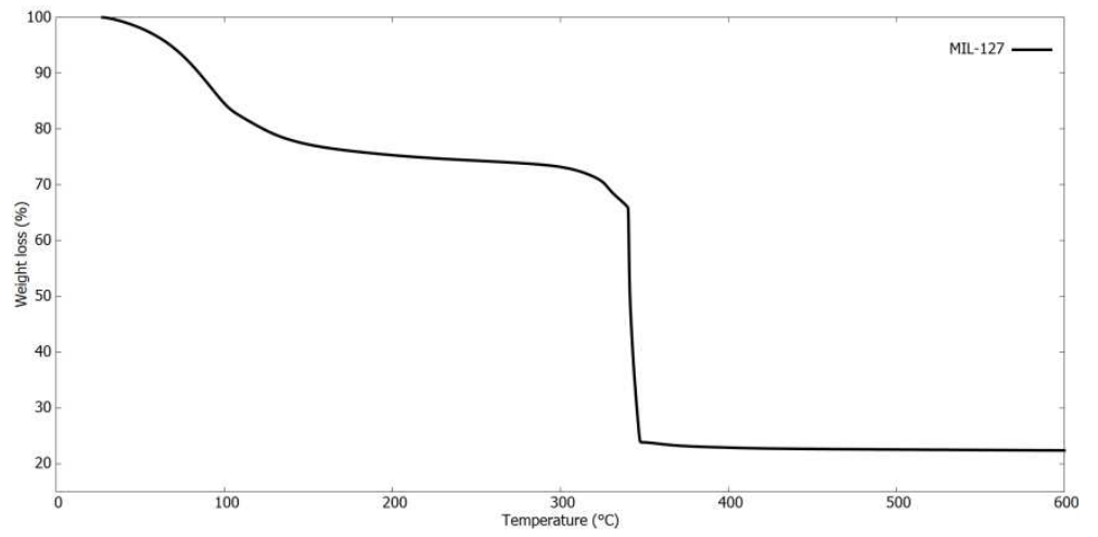
Figure A.5 : Analyse thermogravimétrique du MIL-127(Fe).
