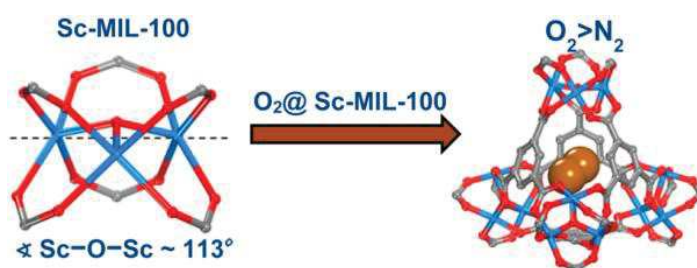
Figure 1.20 : L'adsorption du dioxygène par le Sc-MIL-100. Reproduit à partir de [204].
