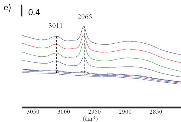
Figure A.61 : a) Spectres FTIR dans la région spectrale de 5500-700\text{ cm}^{-1} lors de l'adsorption du formaldéhyde par un échantillon Al-3.5-PDA présaturé avec du \text{CO}_2 , de bas en haut : augmentation progressive des bandes caractéristiques du formaldéhyde chimisorbé. b) Spectres FTIR dans la région spectrale de 2355-2320\text{ cm}^{-1} lors de l'adsorption du formaldéhyde par un échantillon Al-3.5-PDA présaturé avec du \text{CO}_2 , de haut en bas diminution de la bande caractéristique du \text{CO}_2 physisorbé (lors de l'augmentation des bandes caractéristique du formaldéhyde chimisorbé). c) Spectres décrits dans les sous-figures d) et e) dans la région spectrale 5500-700\text{ cm}^{-1} . d) Dans la région spectrale 2355-2320\text{ cm}^{-1} , (groupe de spectres dans la partie basse) spectres FTIR obtenus lors de l'adsorption du formaldéhyde par un échantillon AL-3.5-PDA saturé avec du \text{CO}_2 ; (groupe de spectres dans la partie haute) adsorption de \text{CO}_2 sur un échantillon saturé en formaldéhyde (spectre bleu dans la partie haute) suivie de l'évacuation sous vide dynamique (spectre rouge dans la partie haute). e) De bas en haut : Adsorption du formaldéhyde par un échantillon Al-3.5-PDA saturé avec du \text{CO}_2 (spectre vert) suivie de l'adsorption de \text{CO}_2 par un échantillon Al-3.5-PDA saturé avec du formaldéhyde (spectre bleu dans la partie haute) suivie par l'évacuation sous vide dynamique (spectre rouge dans la partie haute). Dans la région spectrale 3100-2800\text{ cm}^{-1} (échelle offset).
