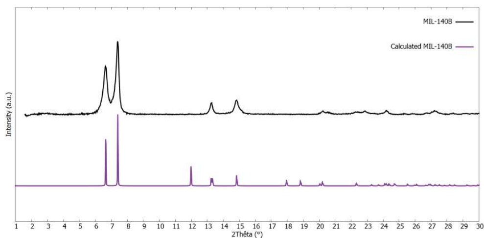
Figure A.13 : Analyse par diffraction des rayons X du MIL-140B.
