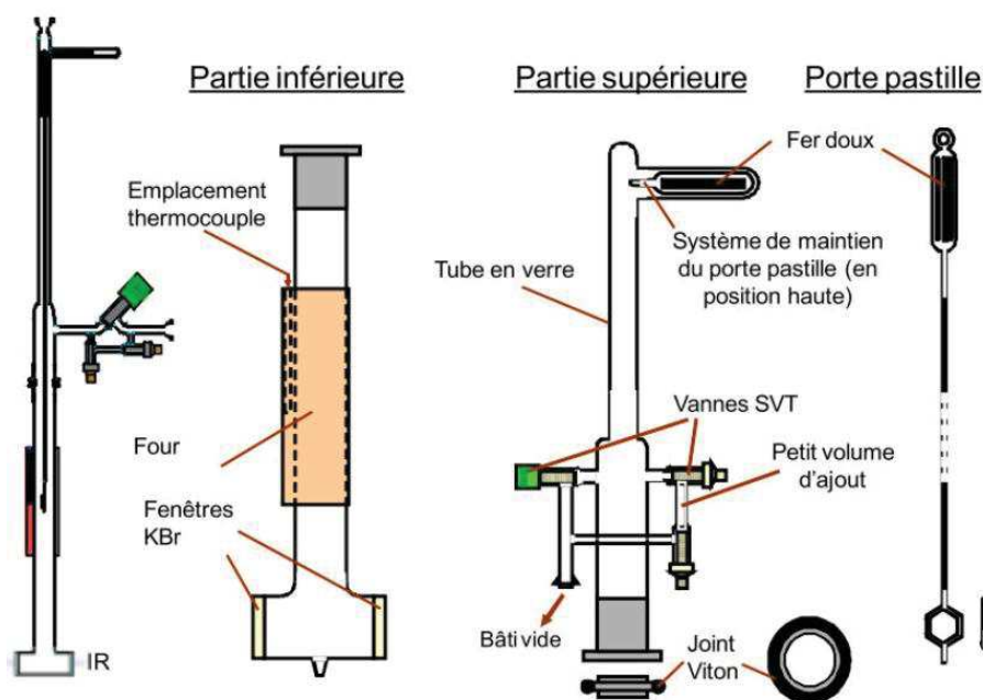
Figure A.60 : Cellule FTIR pour l'adsorption à température ambiante.
