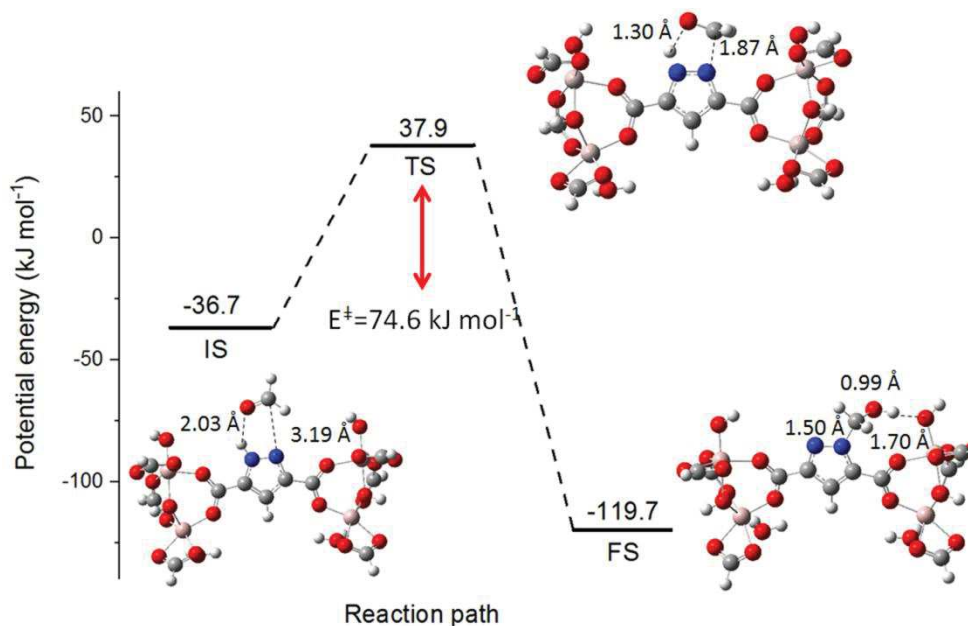
Figure 4.28 : Mécanisme réactionnel théorique de la formation des groupements oxyméthyles avec le modèle étendu.
