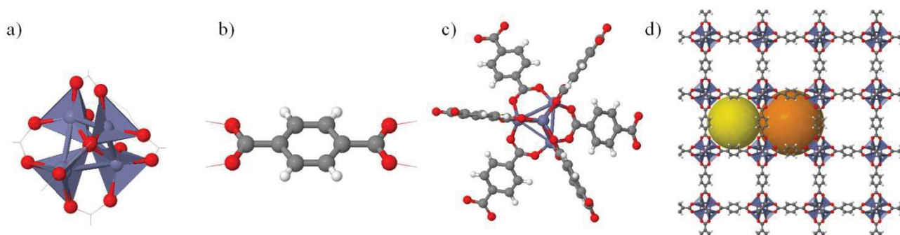
Figure 1.12 : Représentation selon le modèle « ball and sticks » de la reconstruction du MOF-5 (ou IRMOF-1) de formule \text{Zn}_4(\text{O}(\text{BDC}))_3 (BDC = benzène-1,4-dicarboxylique acide), formé de tétramères de \text{ZnO}_4 [en a)] liés par six acides benzène-1,4-dicarboxyliques [en b) et c)] conduisant à une structure 3D présentant deux types de cavités alternés de 15.1 Å et 11.0 Å représentées par des sphères oranges et jaunes respectivement [en d)]. Réalisé en utilisant [117], à partir de [119].
