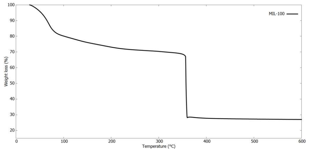
Figure A.2 : Analyse thermogravimétrique du MIL-100(Fe).
