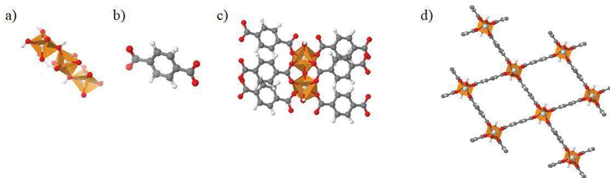
Figure 1.9 : Représentation selon le modèle « ball and sticks » de la reconstruction par étape du MIL-53(Al) ayant pour formule Al[OH][O_2C-C_6H_4-CO_2] , formé à partir de chaînes infinies d'aluminium et oxygènes ( AlO_6 ) _{\infty} [en a], reliées entre elles par l'acide benzène-1,4-dicarboxylique [en b) et c)] pour former une structure tunnel 1D. Réalisé en utilisant [117], reproduit à partir de [118].
