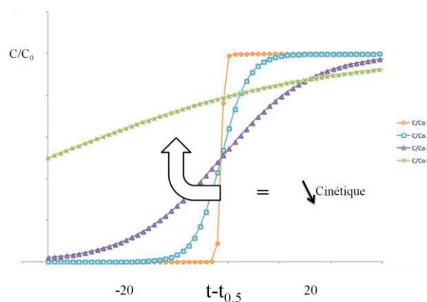
Figure 2.3 : Schématisation de la dépendance du transfert de masse avec la forme de la courbe de percée.
