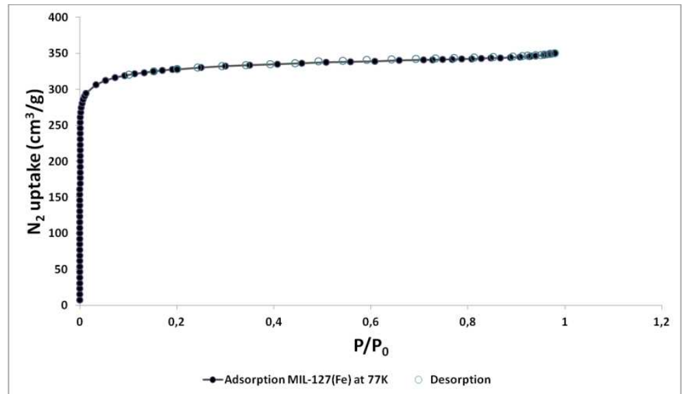
Figure A.6 : Adsorption/désorption de N 2 du MIL-127(Fe).
