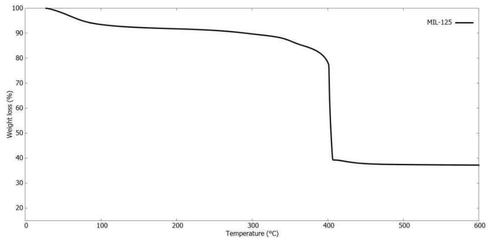
Figure A.20 : Analyse thermogravimétrique des MIL-125 / MIL-125-NH 2 .
