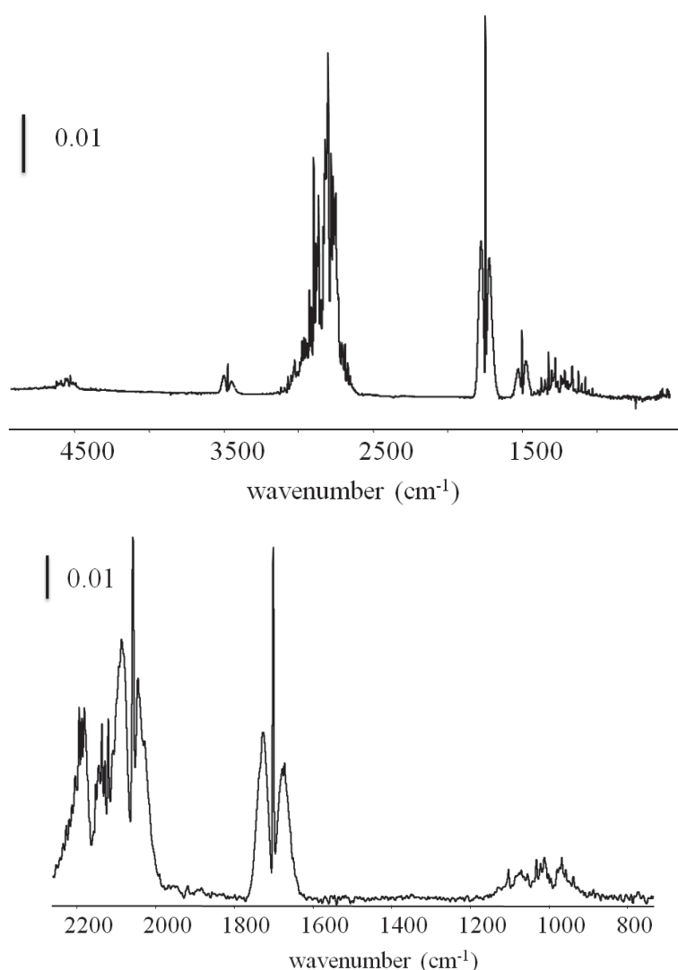
Figure 3.1 : Spectres FTIR obtenus à partir de la décomposition thermique du paraformaldéhyde et du paraformaldéhyde deutéré.
