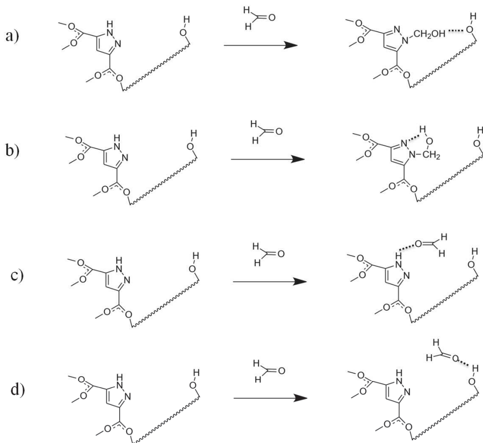
Figure 3.9 : Représentation schématique possible de l'interaction entre le formaldéhyde, le ligand pyrazole et les groupements \mu_2 -OH du MOF Al-3.5-PDA a) formation des groupements oxyméthyles après réaction du formaldéhyde sur le ligand pyrazole et stabilisation par liaison hydrogène sur les groupements \mu_2 -OH des chaînes inorganiques, b) formation des groupements oxyméthyles après réaction du formaldéhyde sur le ligand pyrazole et stabilisation par liaison hydrogène sur le doublet de l'azote pyridinique, c) interaction du formaldéhyde par liaison hydrogène avec l'azote pyrrolique, d) interaction du formaldéhyde par liaison hydrogène avec le groupement \mu_2 -OH.
