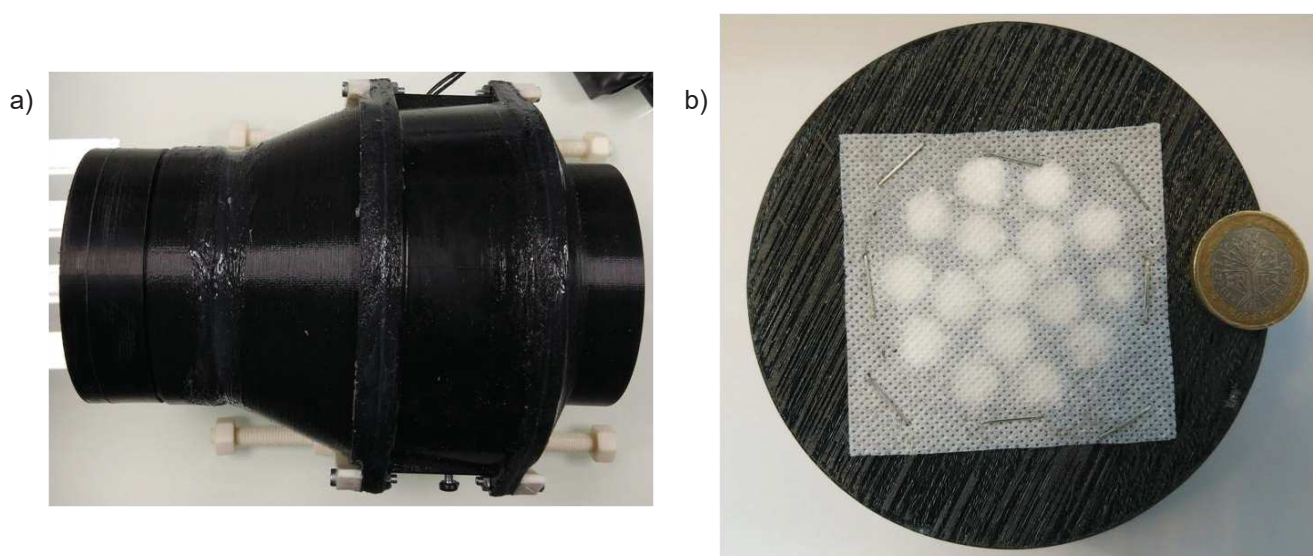
Figure 5.4 : a) Photographie du prototype de dépollution b) Photographie d'un filtre MOF.
