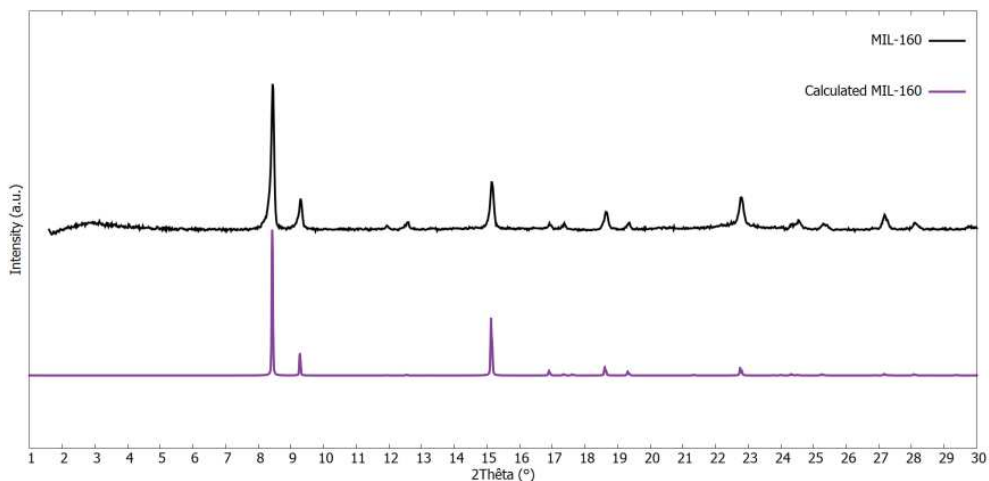
Figure A.22 : Analyse par diffraction des rayons X du MIL-160.
