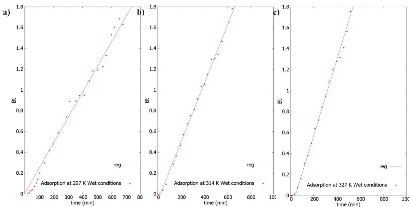
Figure A.66 : Application du modèle de Boyd-Reichenberg lors de l'adsorption du formaldéhyde par un échantillon Al-3.5-PDA, en condition d'atmosphère humide, à différentes températures : a) à 297 K, 314 K, 327 K. Réalisée en utilisant GNU PLOT [29].
