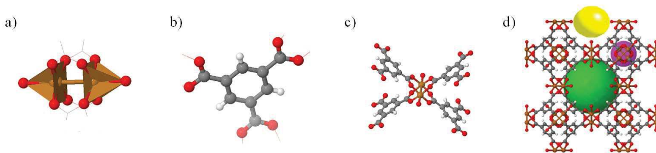
Figure 1.11 : Représentation selon le modèle « ball and sticks » de la reconstruction par étape du HKUST-1 de formule \text{Cu}_3(\text{BTC})_2 (BTC = acide 1,3,5-benzènetricarboxylique) sous sa forme déshydratée, formé à partir de dimères de \text{CuO}_4(\text{OH}) [en a)] liés par quatre BTC [en b) et c)] pour former une structure 3D présentant trois types de porosités d'un diamètre moyen de 14 Å, 11 Å, 5 Å, représentées respectivement sous forme de sphères verte, jaune et violette [en d)]. Réalisé en utilisant [117], à partir de [110].
