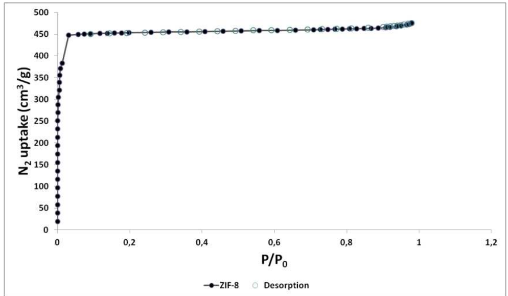
Figure A.39 : Adsorption/désorption de N 2 du ZIF-8.
