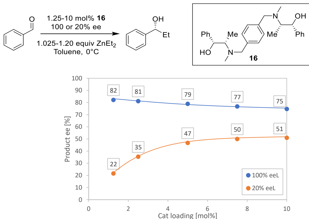
Figure 152: Variation de la charge en catalyseur dans l'addition énantiosélective de ZnEt_2 au benzaldéhyde catalysée par 16 à 100% ee_L (points bleus) et 20% ee_L (points oranges).
