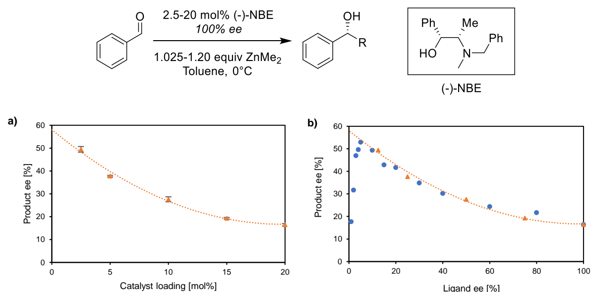
Figure 145: a) ee_P en fonction de la charge en catalyseur dans l'addition énantiosélective de ZnMe_2 au benzaldéhyde catalysée par (-)-NBE, b) superposition de a) avec l'effet non-linéaire hyperpositif.
