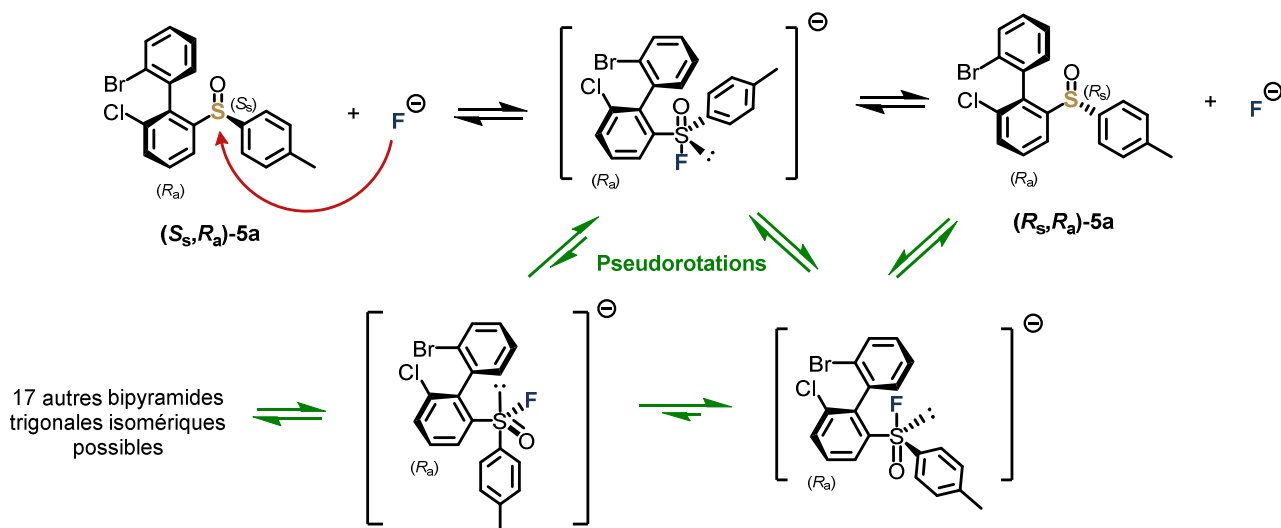
Schéma 53 Mécanisme supposé d'épimérisation du centre soufré de (S_s, R_a) -5a en présence d'ions fluorure
