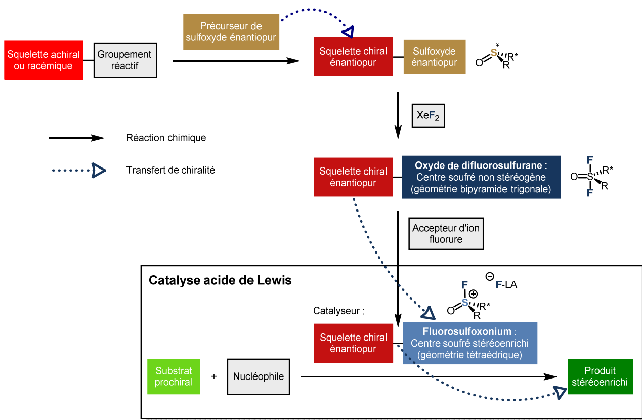
Figure 28 Schéma général du relais de chiralité possible entre le sulfoxyde à chiralité centrale et l'élément stéréogène supplémentaire
