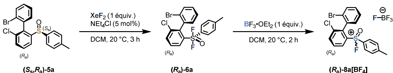
Schéma 50 Synthèse du sel de fluorosulfoxonium 8a [BF 4 ]
