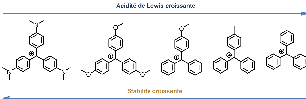
Figure 5 Classement de différents cations tritylium en fonction de leur acidité de Lewis et de leur stabilité thermodynamique
