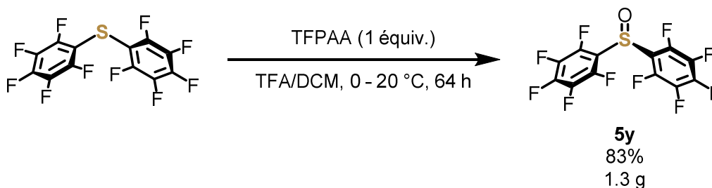
Schéma 143 Synthèse du sulfoxyde perfluoré 5y
