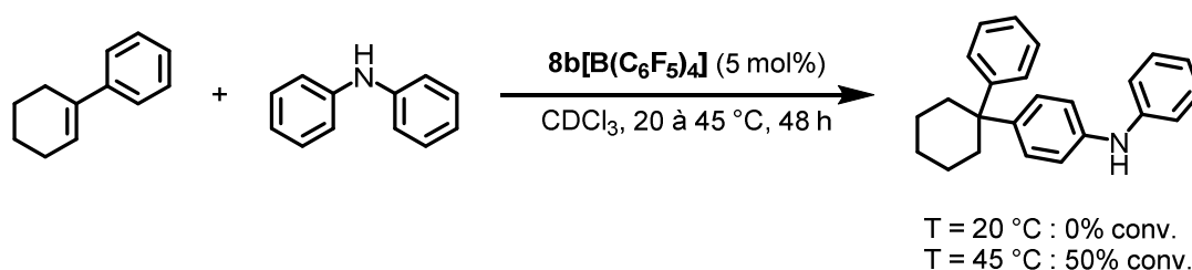
Schéma 60 Hydroarylation de dérivés de styrène par la diphenylamine
