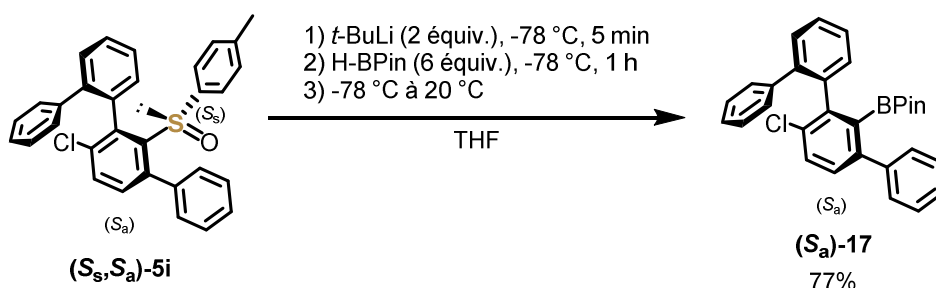
Schéma 78 Synthèse de l'ester boronique 17
