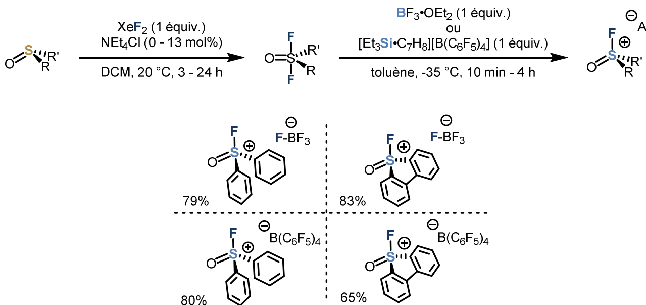
Figure 24 Synth\u00e8se et structure des sels de fluorosulfoxonium d\u00e9crits par Stephan et al.
