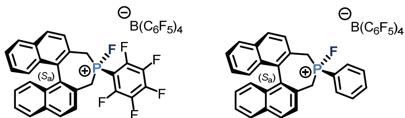
Figure 37 Structure des sels de fluorophosphonium à chiralité axiale de Stephan, Oestreich et al.
