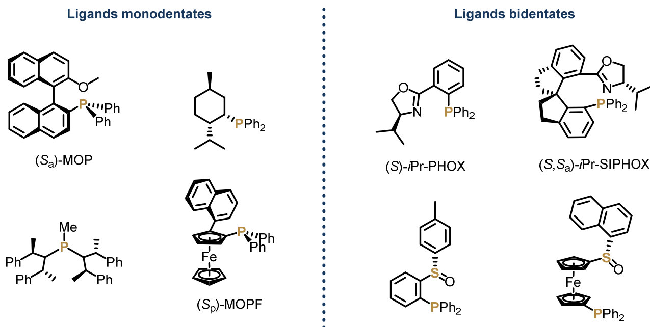
Figure 36 Exemples sélectionnés de quelques ligands monophosphines chirales mono- et bidentates non P -stéréogènes. Les noms génériques de ces ligands sont donnés lorsqu'ils existent
