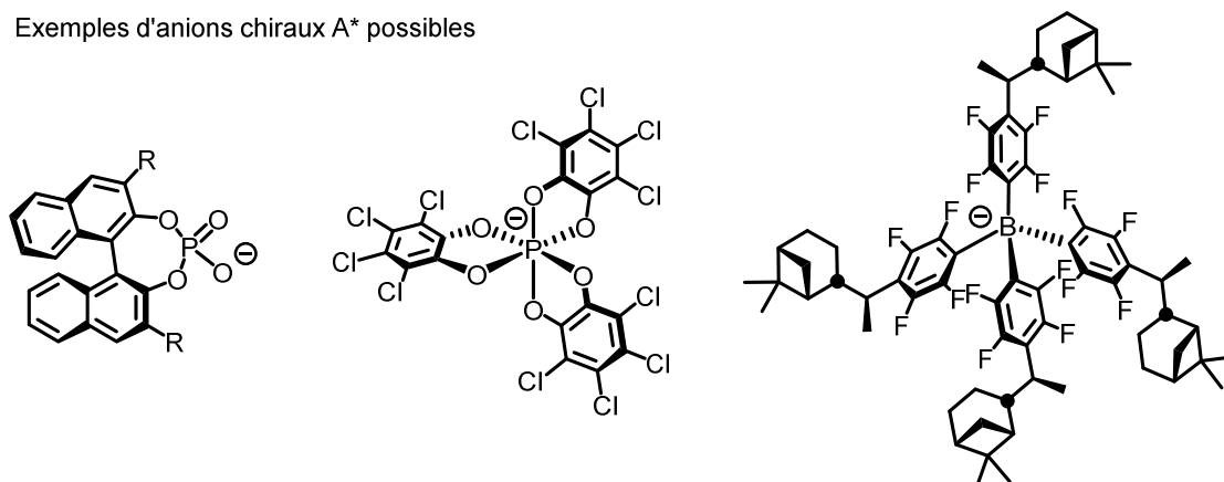
Schéma 162 Métathèse anionique pour l'installation d'anions chiraux sur des sels de fluorosulfonylium et exemples d'anions chiraux connus et potentiellement utilisables
