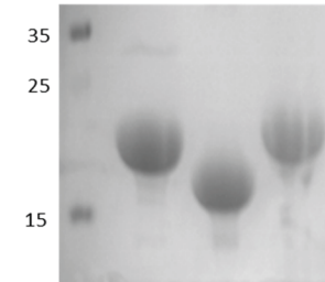
Figure 46 : Résultats de purification des différentes constructions d'ANP32E Gels SDS-PAGE et chromatogrammes des différentes étapes de purification, (Pd) : polydispersité
