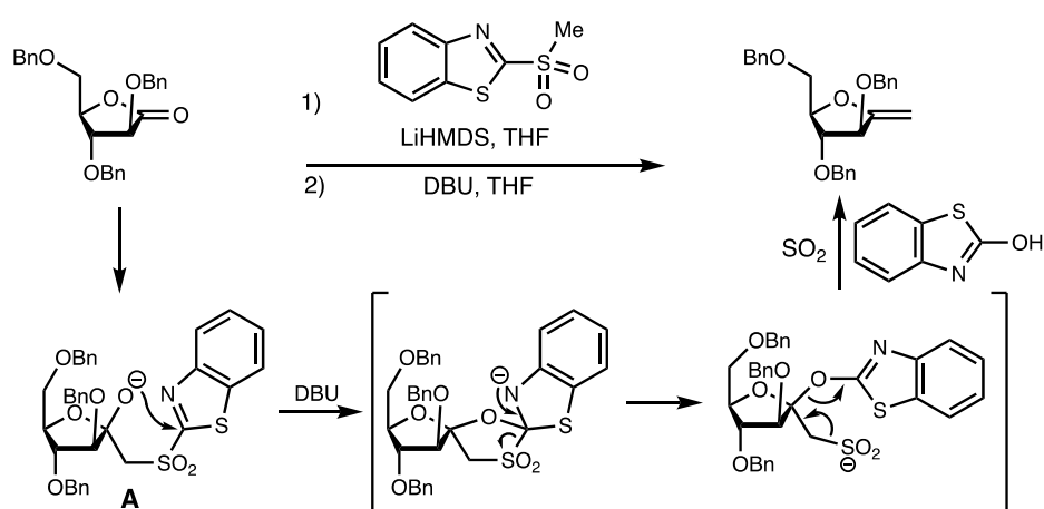
Schéma 107: Mécanisme de l'oléfin de Julia d'une lactone pour conduire à des exo -glycols
