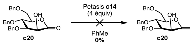
Schéma 204 : Tentative d'oléfination de la lactone c20 par le réactif de Petasis
