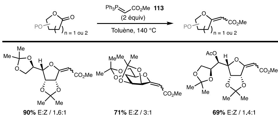
Sch\u00e9ma 101: Ol\u00e9fination de Wittig par l'ylure stabilis\u00e9 113
