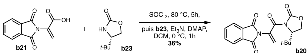
Schéma 166 : Couplage des fragments b21 et b23 pour fournir l'accepteur b20
