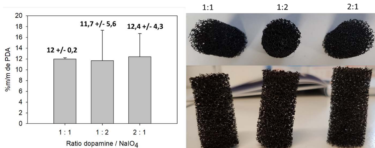
Figure 3.12. (gauche) Histogramme représentant l'augmentation de la masse des mousses polymères en fonction Du ratio DA / \text{NaIO}_4 ; (droite) Photographies des mousses modèles revêtues de PDA par pulvérisation en fonction des trois ratio différents
