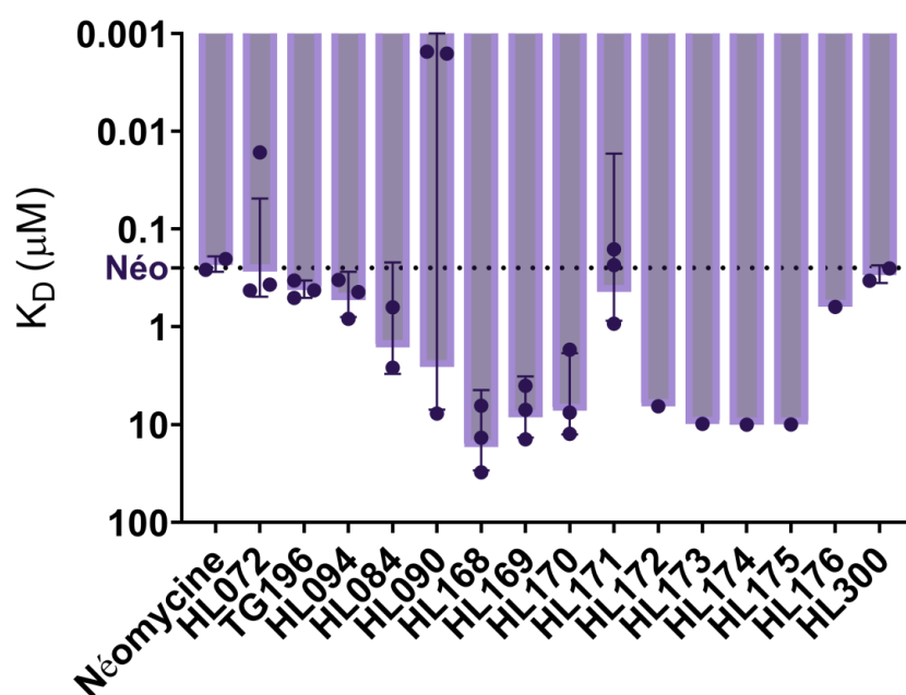
Figure 40 - Affinités des dérivés de néomycine pour le site A bactérien. Les valeurs de constante de dissociation ( K_D ) reflètent l'affinité des composés pour le site A, plus la valeur est faible, plus l'affinité est forte. La ligne pointillée représente la valeur de K_D pour la néomycine (Néo).
