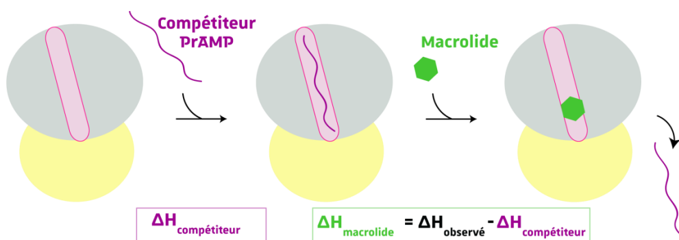
Figure 22 - Stratégie d'ITC par compétition
