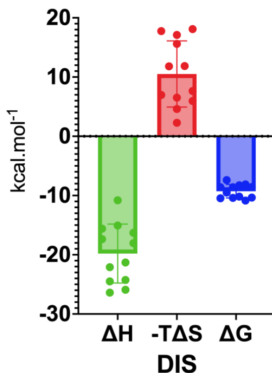
Figure 51 - Représentation de la distribution des profils thermodynamiques pour tous les dérivés de la néomycine en interaction avec DIS. Les valeurs moyennes de \Delta H , -T\Delta S et \Delta G pour chaque dérivé (Néomycine, HL072, TG196, HL094, HL084, HL090, HL168, HL169, HL170, HL171, HL172, HL173, HL300) sont représentées pour mettre en valeur la dispersion. Tous les résultats sont normalisés par un contrôle de titration de chaque dérivé dans du tampon seul.
