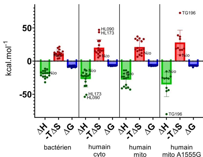
Figure 38 - Représentation de la distribution des profils thermodynamiques pour tous les dérivés de la néomycine en interaction avec les sites A humains cytoplasmique, mitochondrial et mitochondrial mutant. Humain cyto = Site A humain cytoplasmique. Humain mito = Site A humain mitochondrial WT. Humain mito A1555G = Site A humain mitochondrial mutant A1555G (numérotation ARNr 12 S, H. sapiens ). Les valeurs moyennes de \Delta H , -T\Delta S et \Delta G pour chaque dérivé (Néomycine, HL072, TG196, HL094, HL084, HL090, HL168, HL169, HL170, HL171, HL172, HL173, HL174, HL175, HL176, HL300) sont représentées pour mettre en valeur la dispersion. Les points correspondant à la néomycine (Néo) et aux dérivés avec les valeurs les plus éloignées de la moyenne sont indiqués. Tous les résultats sont normalisés par un contrôle de titration de chaque dérivé dans du tampon seul.
