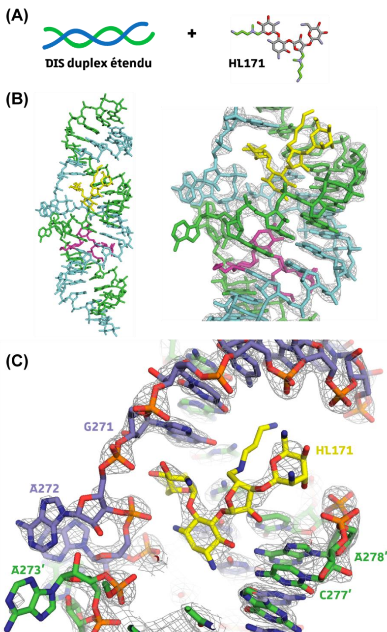
Figure 54 - Structure cristallographique du dérivé HL171 avec l'ARN DIS. (A) Schéma des du DISF et du composé ajouté pour la co-cristallisation. (B) Structure obtenue pour le co-cristal DISF-HL171. A gauche : vue globale du DISF en duplex étendu. A droite : zoom sur les deux molécules de dérivés HL171 observées au site d'interaction. (C) Carte de densité et reconstruction de la structure au niveau du site d'interaction de HL171 dans le DISF.
