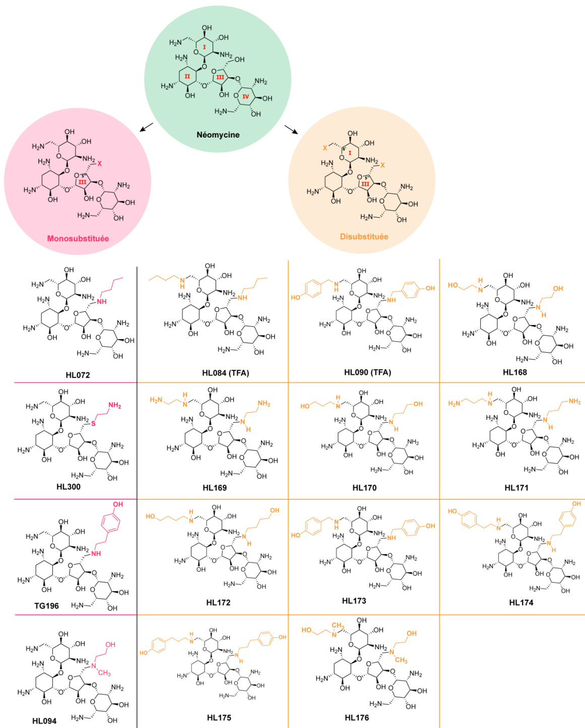
Figure 34 - Structures des dérivés de Néomycine. Les dérivés sont monosubstitués en position 5'' ou disubstitués aux positions 5'' et 6' du squelette de la Néomycine.
