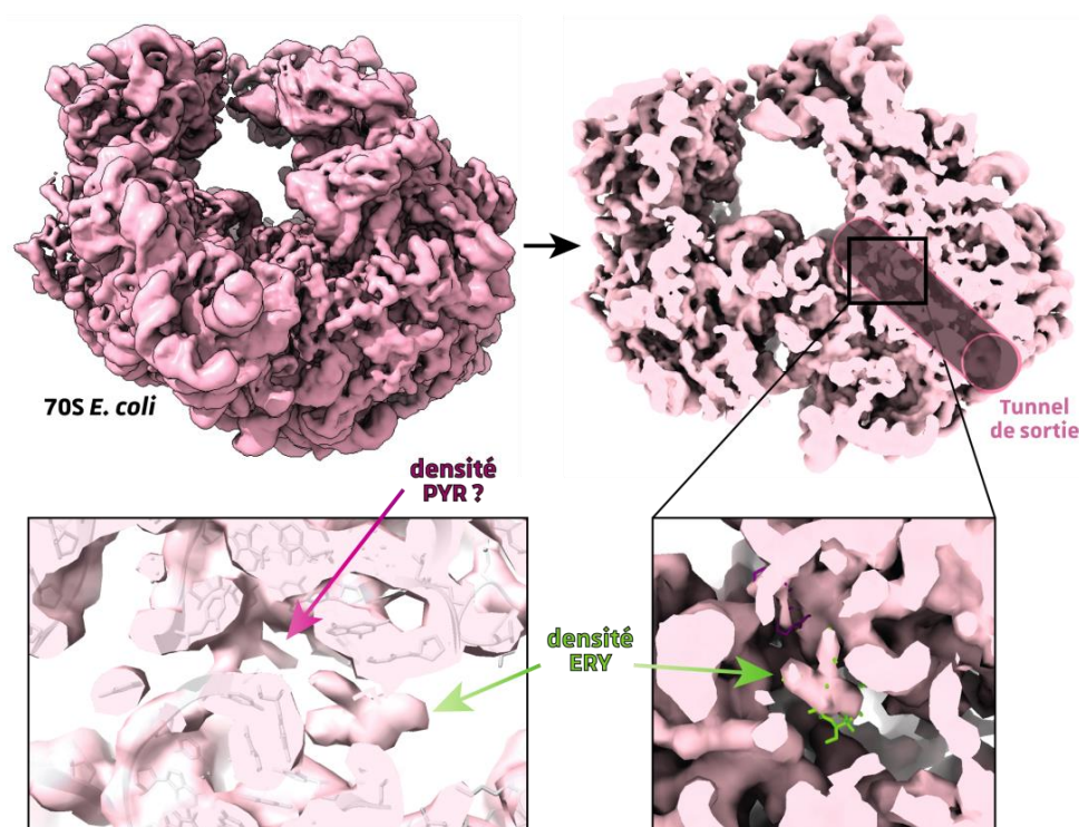
Figure 28 – Densités observées au site d'interaction dans le tunnel de sortie du ribosome. Le 70 S entier et en coupe sont représentés au-dessus. La position des densités est indiquée sur le 70 S. En dessous : zoom sur les densités observées au sein du site d'interaction des macrolides, la densité de droite correspondant très probablement à l'érythromycine, la densité à gauche de la première est moins résolue mais pourrait correspondre à la pyrrhocoricine.
