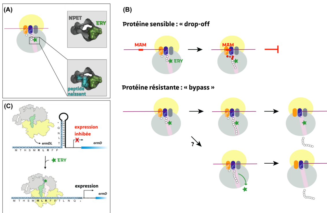
Figure 9 – Mécanisme d'action des macrolides, arrêt programmé de la traduction. (A) Vue de l'érythromycine au sein du tunnel de sortie. Le tunnel est assez large pour laisser passer un peptide (adapté de Vázquez-Laslop et Mankin 2018), NPET = « Native Peptide Exit Tunnel », tunnel de sortie des peptides naissants. (B) Mécanismes possibles de traduction lorsque le ribosome est lié à un macrolide. (C) Exemple de traduction de l'opéron ErmDL en présence d'un macrolide. L'expression du gène ermD est dépendante de la présence de l'érythromycine qui bloque la traduction du peptide leader qui comporte un motif MAM (de Beckert et al. 2021).
