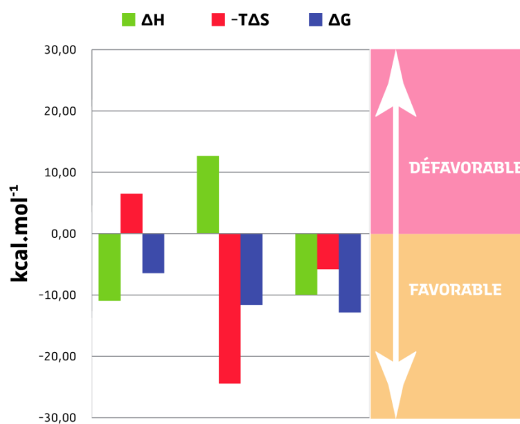
Figure 21 – Exemples de profils thermodynamiques. De gauche à droite : profil typique d'une interaction favorisée par la formation de liaisons et défavorisée par des changements conformationnels, profil typique d'une interaction dominée par des interactions hydrophobes, profil typique d'une interaction favorisée par la formation de liaisons hydrogènes et des interactions hydrophobes.
