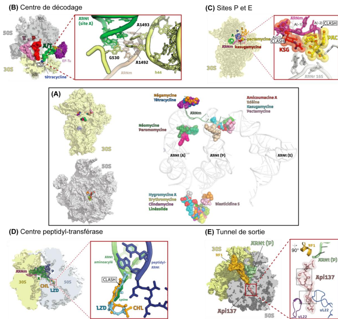
Figure 6 - Sites d'interaction d'antibiotiques ciblant le ribosome. (A) Sites d'interaction de différents antibiotiques au niveau des sites A, P et E du ribosome (adapté de Arenz et Wilson 2016a). (B) Site d'interaction au niveau du centre de codage (CD) des tétracyclines. Zoom sur les résidus impliqués dans l'interaction des antibiotiques ciblant le CD (adapté d'Arenz et Wilson 2016b). (C) Sites d'interaction de la kasugamycine (KSG) et de la pactamycine (PAC) au niveau des sites P/E (adapté de Vázquez-Laslop et Mankin 2018). (D) Interaction du linézolide (LZD) et du chloramphénicol (CHL) au niveau du centre peptidyle-transférase (adapté de Vázquez-Laslop et Mankin 2018). (E) Site d'interaction d'un PrAMP (Api137) dans le tunnel de sortie des peptides néosynthétisés (de Florin et al. 2017).
