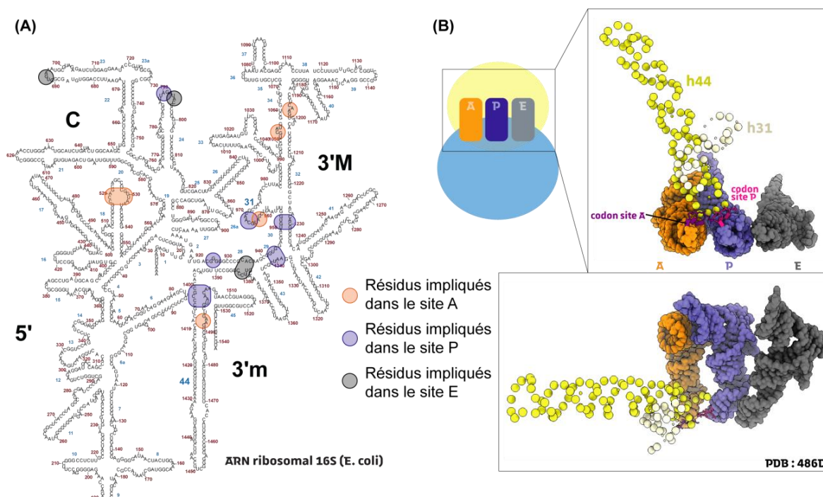
Figure 12 - Structure secondaire de l'ARN ribosomal 16S et position des sites A, P et E du ribosome. (A) Structure secondaire de l'ARNr 16 S (CC BY-SA, ©2013-2015 Georgia Institute of Technology). Les différents domaines de la structure sont indiqués (5', C, 3'M, 3'm), le numéro des hélices est indiqué en bleu, la numérotation des nucléotides est en bordeaux. Les nucléotides impliqués dans la liaison des ARNt dans les sites A, P et E sont cerclés en orange, bleu et gris, respectivement. (B) Représentation en 3D des ARNt positionnés dans les sites A (orange), P (bleu) et E (gris). PDB : 486D (Cate et al. 1999).
