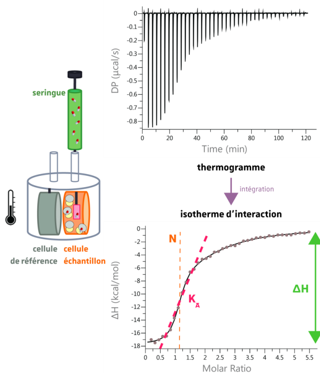
Figure 20 - Exemple de thermogramme obtenu lors d'une expérience d'ITC
