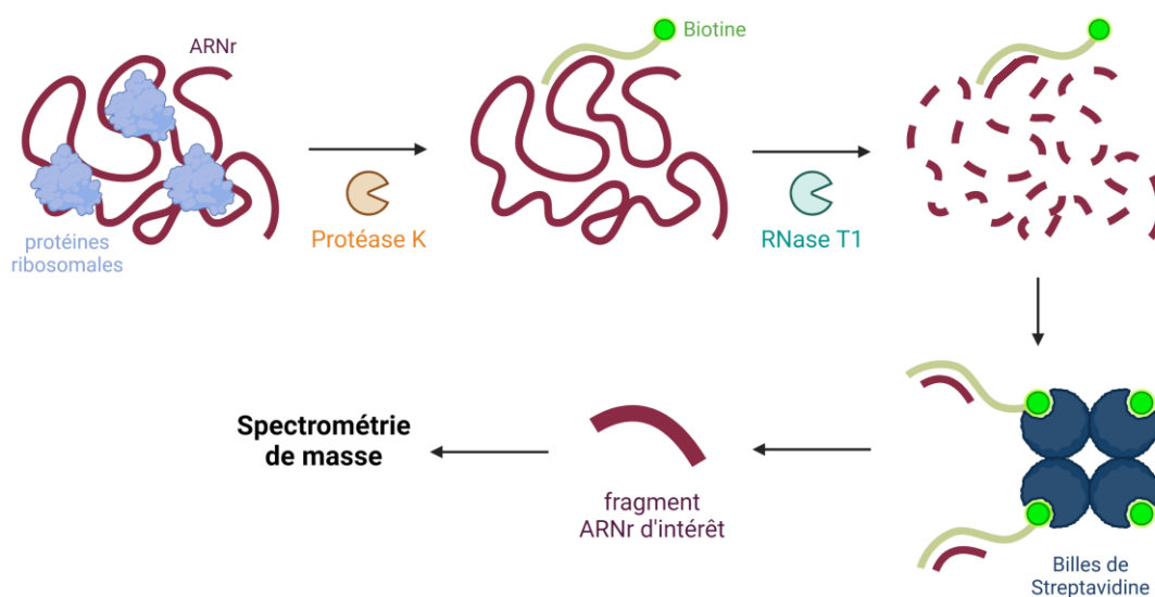
Figure 25 – Stratégie pour la mise en évidence de modifications sur l'ARNr.
