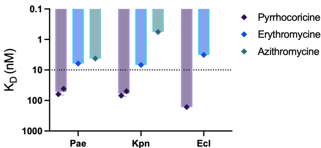
Figure 24 - Affinités des interactions de macrolides avec des ribosomes ESKAPE. Les valeurs des constantes de dissociation ( K_D ) en nM sont représentées pour chaque souche testée : Pseudomonas aeruginosa (Pae), Klebsiella pneumoniae (Kpn) et Enterobacter cloacae (Ecl).
