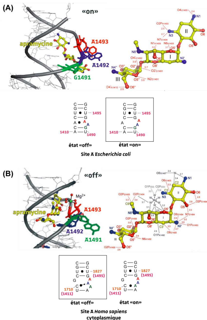
Figure 17 – Interaction de l'apramycine avec les sites A bactérien et humain cytoplasmique. (A) A gauche : Vue de la structure cristalline du complexe apramycine-site A bactérien (PDB : 1YRJ) (adapté de Kondo et al. 2006, SI). A droite : Contacts directs entre l'apramycine et les atomes du site A bactérien (numérotation E. coli ) représentés par des lignes pointillées rouges (adapté de Kondo et al. 2006, SI). En bas : représentation schématique des différents états du site A bactérien. L'état stabilisé en présence d'apramycine est encadré en noir. (B) A gauche : Vue de la structure cristalline du complexe apramycine-site A humain cytoplasmique (PDB : 2G5K) (adapté de Kondo et al. 2006). A droite : Contacts directs et indirects (via des molécules d'eau) entre l'apramycine et les atomes du site A humain cytoplasmique (numérotation E. coli ) représentés par des lignes pointillées rouges et noires, respectivement (adapté de Kondo et al. 2006). En bas : représentation schématique des différents états du site A humain cytoplasmique. L'état stabilisé en présence d'apramycine est encadré en noir.
