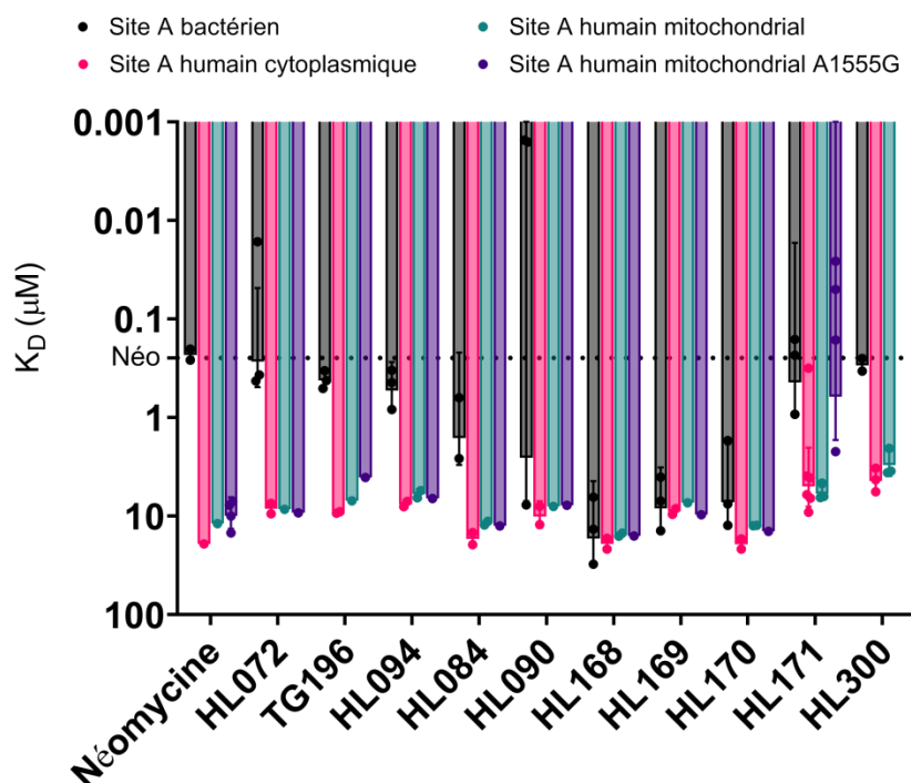
Figure 41 – Affinités des dérivés de néomycine pour les sites A bactérien, humain cytoplasmique, mitochondrial et mitochondrial mutant. Les valeurs de constante de dissociation ( K_D ) reflètent l'affinité des composés pour le site A, plus la valeur est faible, plus l'affinité est forte. La ligne pointillée représente la valeur de K_D pour la néomycine (Néo).
