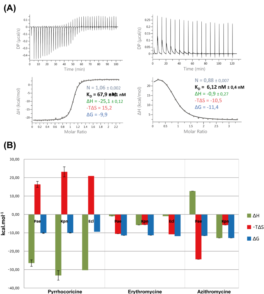
Figure 23 - ITC de compétition macrolides-ESKAPE. (A) Exemple d'isotherme d'interaction obtenu pour l'interaction du ribosome de Pseudomonas aeruginosa avec la pyrrhocoricine (à gauche) et du ribosome de Pae lié à la pyrrhocoricine (PYR) avec l'érythromycine (ERY) (à droite). Les paramètres indiqués correspondent à l'interaction de PYR seule ou du macrolide seul. (B) Signatures énergétiques des ITC de compétition macrolides-ESKAPE. Valeurs des paramètres thermodynamiques en kcal.mol -1 pour chaque souche testée : Pseudomonas aeruginosa (Pae), Klebsiella pneumoniae (Kpn) et Enterobacter cloacae (Ecl).
