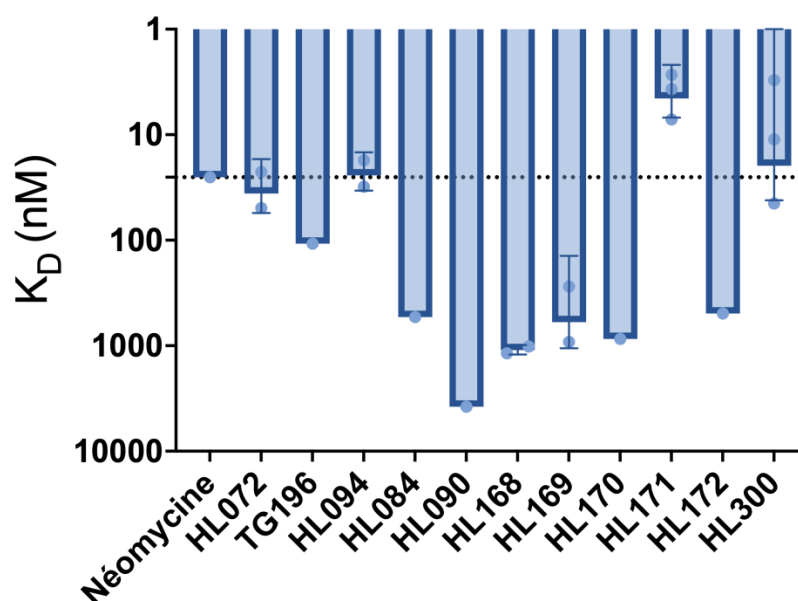
Figure 52 - Affinités des dérivés de néomycine pour l'ARN DIS. Les valeurs de constante de dissociation ( K_D ) reflètent l'affinité des composés pour le DIS, plus la valeur est faible, plus l'affinité est forte. La ligne pointillée représente la valeur de K_D pour la néomycine.
