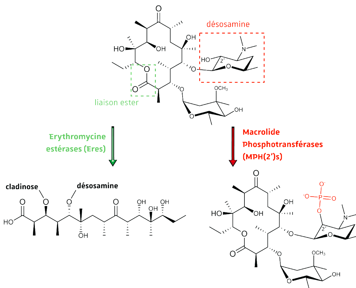
Figure 10 - Mode d'action des enzymes modificateurs de macrolides (adapté de Golkar et al. 2018, créé avec ChemDraw®). Modification de l'érythromycine A par une Macrolide Phosphotransférases (MPH (2')) qui phosphoryle la position 2' du désosamine et une Érythromycine estérases (Eres) qui linéarise le macrolactone.
