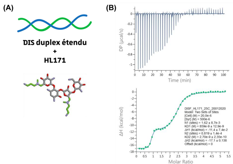
Figure 50 - Profil thermodynamique de l'interaction entre l'ARN DIS et le dérivé HL171
