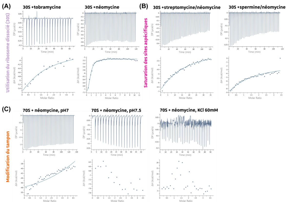
Figure 35 – Titration isotherme par calorimétrie d'un aminoglycoside avec le ribosome. (A) Thermogrammes et isothermes d'interaction d'aminoglycosides avec la sous-unité 30 S du ribosome d' E. coli . (B) Thermogrammes et isothermes d'interaction de compétition pour le 30 S entre une polyamine et la néomycine. (C) Thermogrammes et isothermes d'interaction de la néomycine avec le ribosome entier d' E. coli dans différents tampons. Tous les résultats sont normalisés par un contrôle de titration de chaque dérivé dans le tampon seul.
