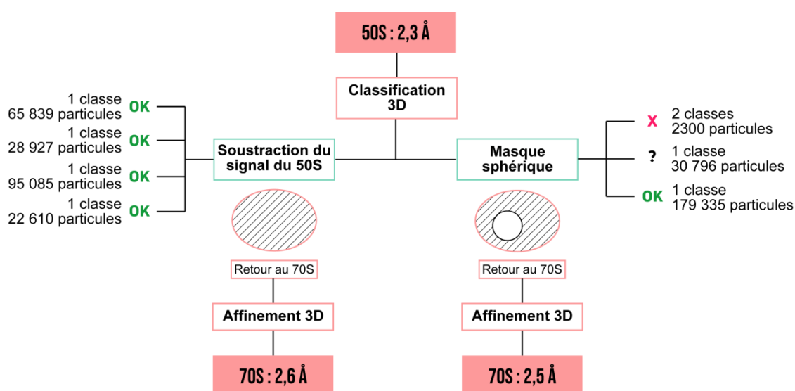
Figure 30 - Affinement à l'aide de masques focalisés sur la densité correspondant à l'érythromycine et une partie de la pyrrhocoricine.
