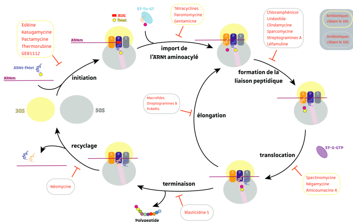
Figure 5 – Étapes de la traduction ciblées par les antibiotiques (adapté de Wilson et al. 2014). Les différentes étapes de la synthèse protéique procaryote et les antibiotiques les inhibant sont représentées. Les antibiotiques ciblant la petite sous-unité (30S) du ribosome sont encadrés en jaune, ceux ciblant la grande sous-unité (50S) sont encadrés en gris.
