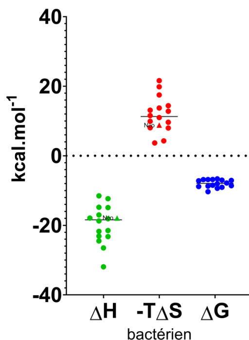
Figure 37 - Représentations de la distribution des profils thermodynamiques pour tous les dérivés de la néomycine en interaction avec le site A bactérien. Les valeurs moyennes de \Delta H , -T\Delta S et \Delta G pour chaque dérivé (Néomycine, HL072, TG196, HL094, HL084, HL090, HL168, HL169, HL170, HL171, HL172, HL173, HL174, HL175, HL176, HL300) sont représentées pour mettre en valeur la dispersion. Les points correspondant à la néomycine (Néo) et aux dérivés avec les valeurs les plus éloignées de la moyenne sont indiqués. Tous les résultats sont normalisés par un contrôle de titration de chaque dérivé dans du tampon seul.
