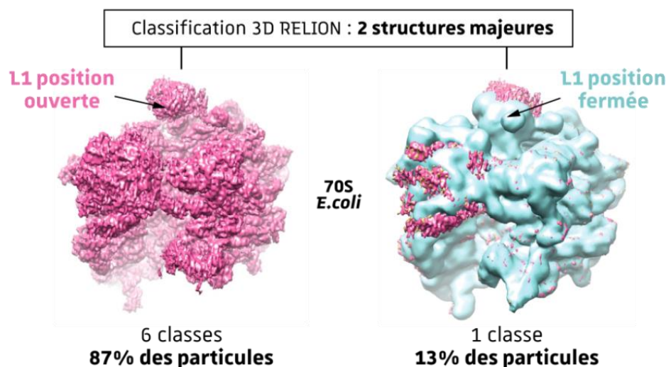
Figure 48 - Classes majeures du complexe E. coli-TG196 obtenues avec cryoSPARC™ et RELION. La reconstruction rose a été obtenue à une résolution de 4,66 Å, la bleue à une résolution de 7,47 Å.
