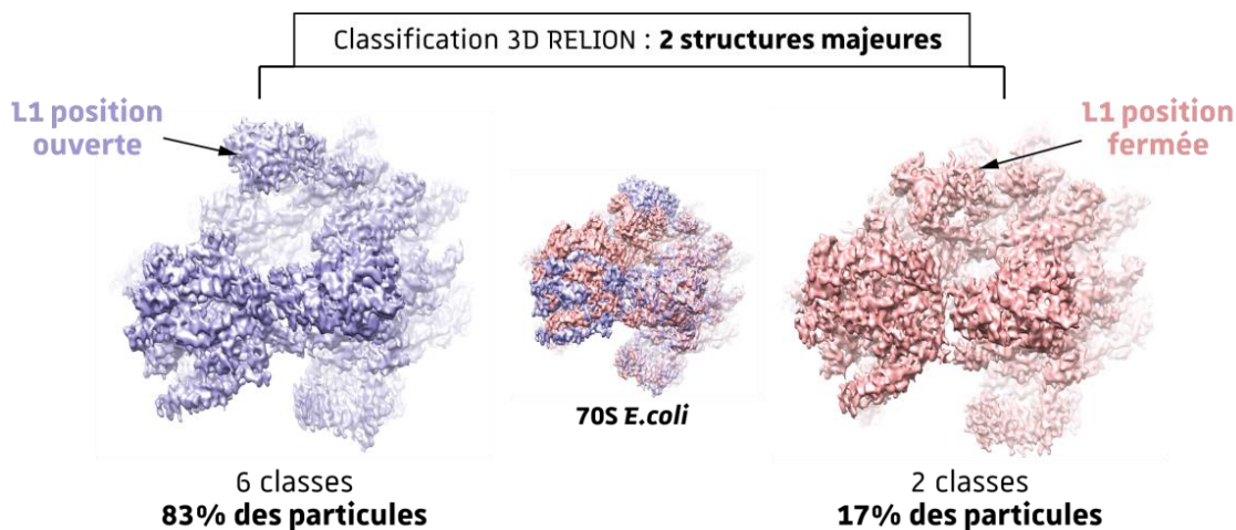
Figure 47 - Classes majeures du complexe E. coli -TG196 obtenues avec Scipion. La protéine L1 indiquée fait partie des protéines composant le 50 S. Les reconstructions ont été obtenues à des résolutions entre 4,9 et 5 Å.
