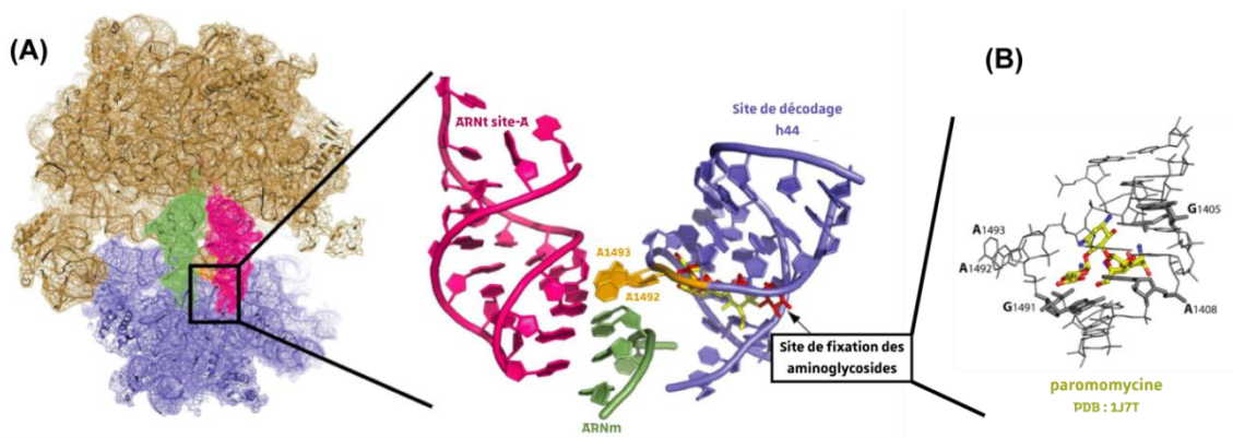
Figure 13 - Site d'interaction des aminoglycosides au niveau du site A (adapté de Feldman et al. 2010 et de Hobbie et al. 2006). (A) Les aminoglycosides fixent l'hélice 44 de l'ARNr 16 S de la petite sous-unité du ribosome et induisent la position ouverte des résidus A1492 et A1493. (B) Structure cristallographique de la paromomycine liée à un oligonucléotide correspondant au site de fixation dans l'hélice 44 (Vicens et Westhof 2001, PDB 1J7T).
