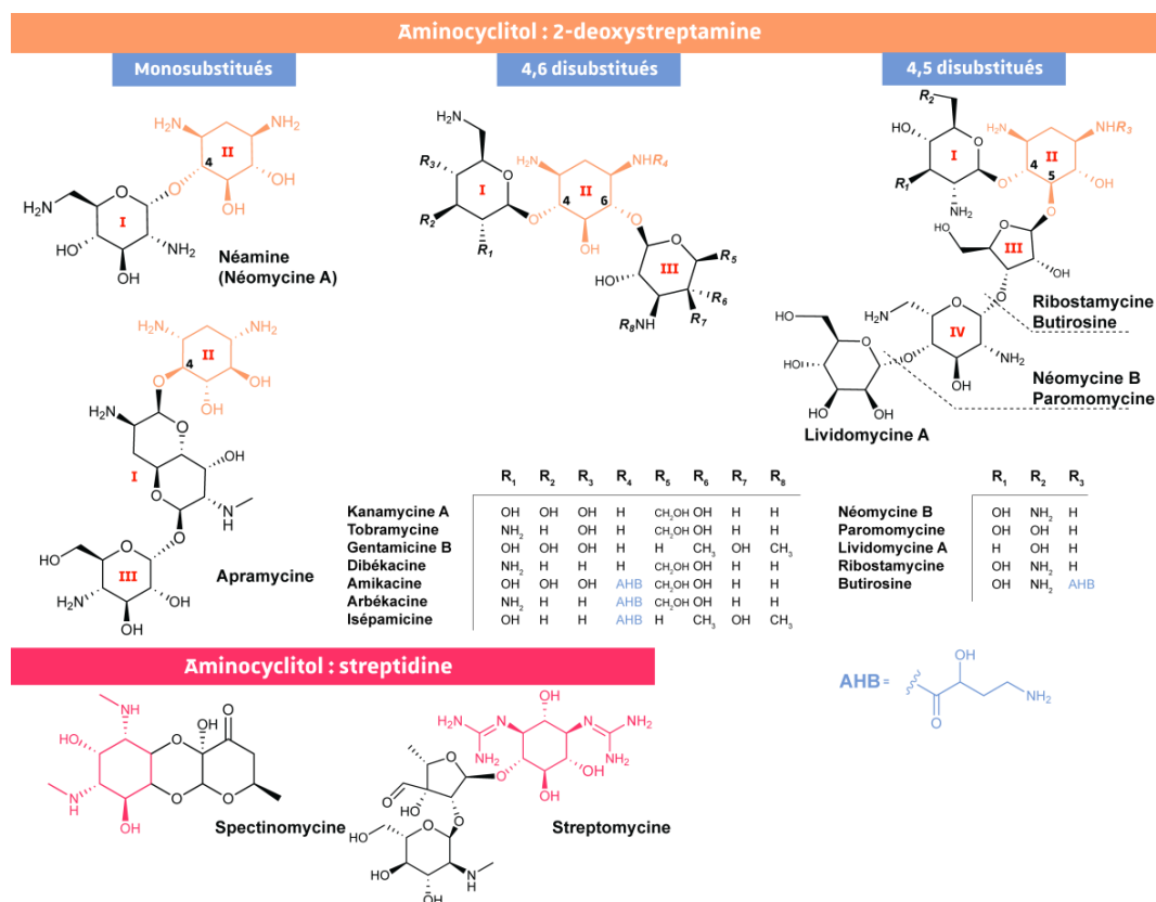
Figure 11 - Structures secondaires des principaux aminoglycosides (adapté de Shi et al. 2013, créé avec ChemDraw®). Le cycle 2-déoxystreptamine des aminoglycosides mono- et disubstitués est coloré en orange, le cycle streptidine est coloré en rose. Le numéro des cycles est indiqué en rouge.
