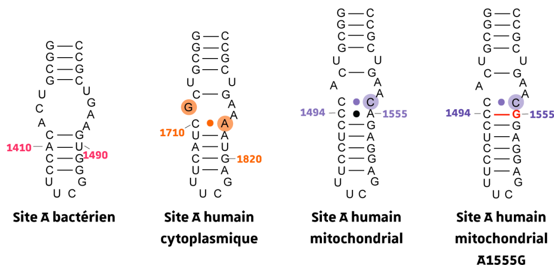
Figure 36 - Oligonucléotides mimant les sites A. Les séquences des oligonucléotides permettent de reproduire une partie de l'hélice 44, correspondant au site A de l'ARNr 16 S du ribosome bactérien ( E. coli ), de l'ARNr 18 S du ribosome humain ( H. sapiens ) ou de l'ARNr 12 S du ribosome mitochondrial ( H. sapiens ).
