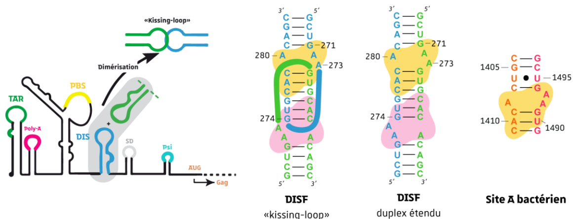
Figure 49 - Similarité entre le DIS et le site A bactérien (adapté de Ennifar 2006)
