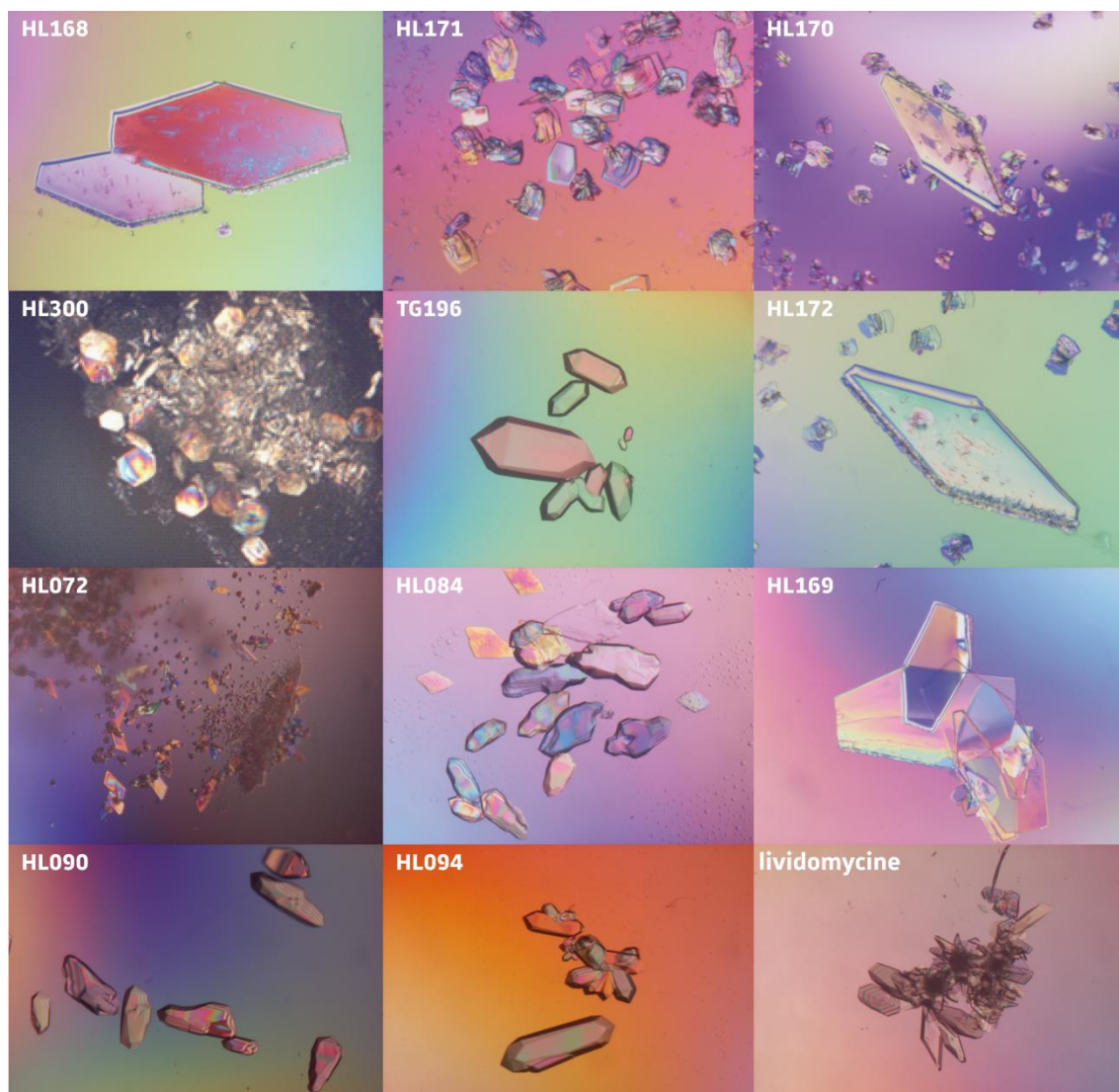
Figure 53 - Cristaux obtenus pour le DISF en présence de dérivés de néomycine ou de la lividomycine.
