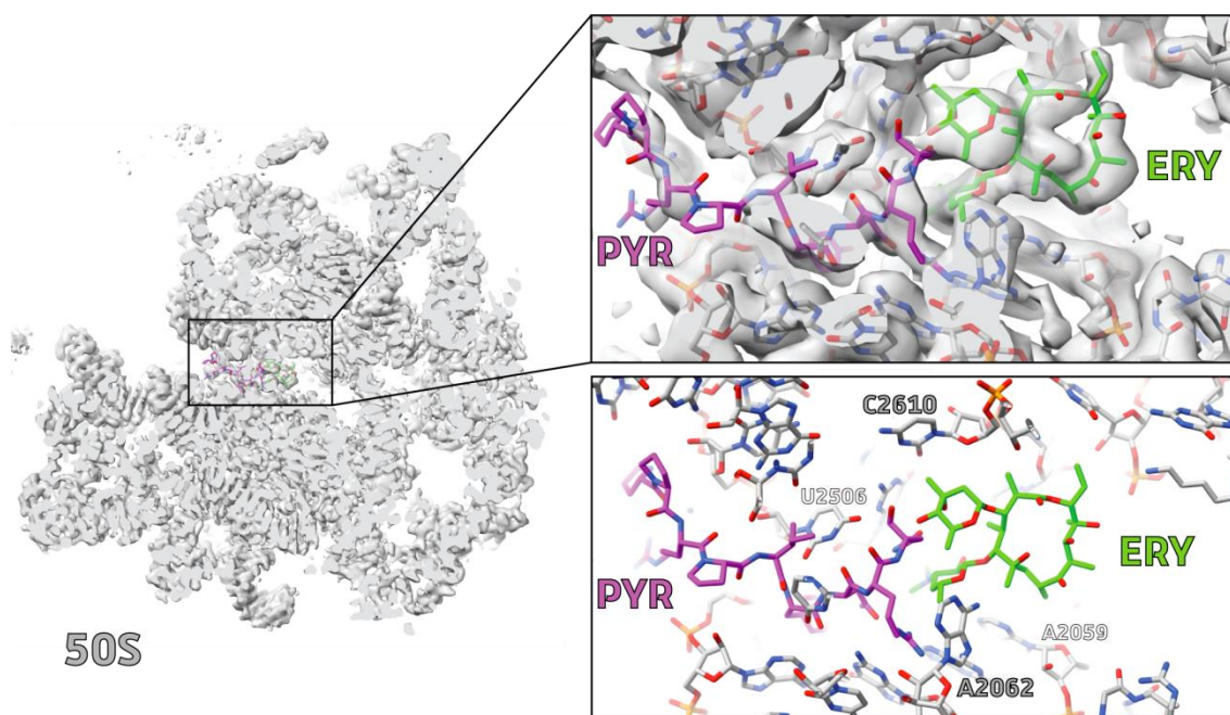
Figure 31 - Carte de densité et reconstruction du 50S, l'érythromycine et une partie de la pyrrhocoricine
