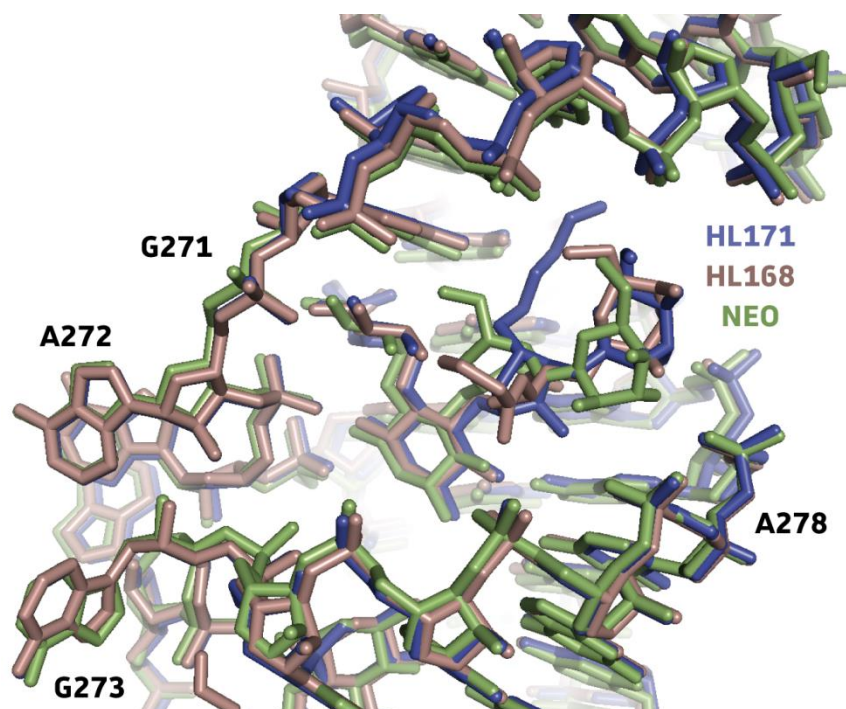
Figure 55 - Comparaison des structures obtenues pour HL168 (rose saumon), HL171 (violet) et la néomycine (vert, PDB = 3C7R)
