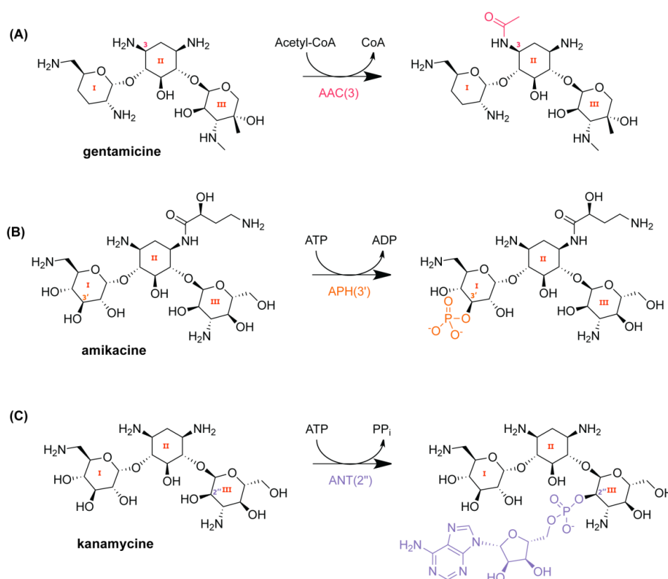
Figure 16 – Enzymes modifiant les aminoglycosides (adapté de Krause et al. 2016, créé avec ChemDraw®). (A) Exemple d'une acétyltransférase de sous-type AAC (3) modifiant la position 3 de l'aminocyclitol de la gentamicine. (B) Exemple d'une phosphotransférase de sous-type APH (3') modifiant la position 3' de l'aminoside (cycle I) de l'amikacine. (C) Exemple d'une adényltransférase de sous-type ANT (2'') modifiant la position 2'' du cycle III de la kanamycine.
