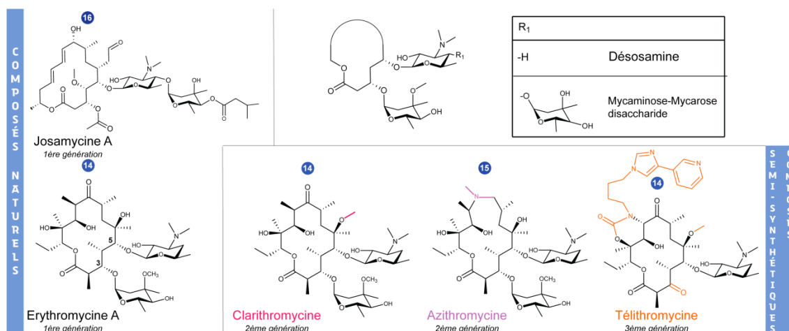
Figure 7 - Structures de macrolides de différentes générations (adapté de Golkar, Zieliński, et Berghuis 2018, créé avec ChemDraw®). La structure commune à tous les macrolides est représentée en haut à droite de la figure. Le nombre d'atomes du macrocycle lactone est indiqué par un cercle bleu. Les modifications apportées à l'érythromycine naturelle pour les composés semi-synthétiques sont colorées en rose, violet ou orange. La troisième génération correspond aux kétolides.
