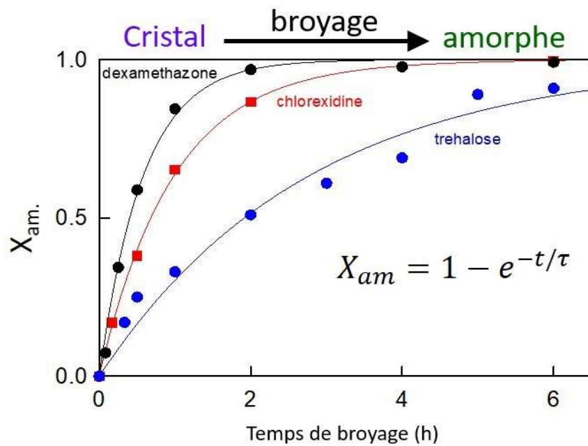
Figure 20: Exemples de cinétiques d'amorphisation sous broyage reportées dans la littérature pour la dexaméthazone, la chlorhexidine et le tréhalose pour des conditions de broyages identiques. Les symboles représentent les données expérimentales et les traits pleins représentent le meilleur ajustement obtenu dans chacun des cas avec la loi indiquée ci-dessus.
