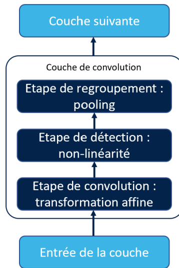
FIGURE 3.12 – Étapes d'une couche de convolution.
