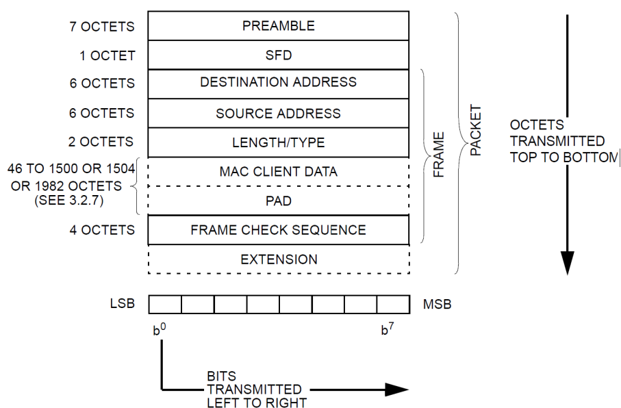
FIGURE 1.6 – Format de la trame Ethernet (« IEEE Standard for Ethernet », 2018).
