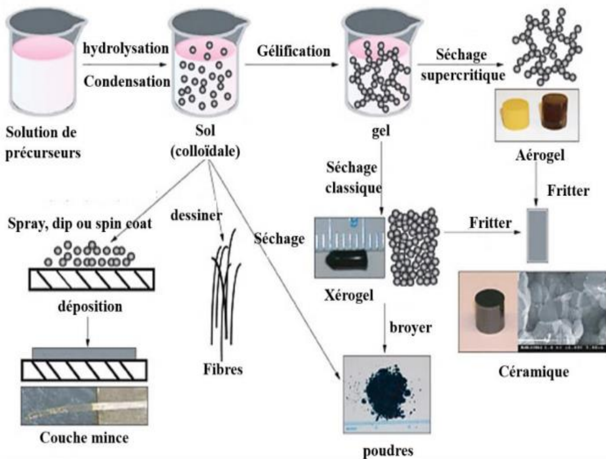
Fig.II.1 Synthèse d'un matériau par voie sol-gel [2]
