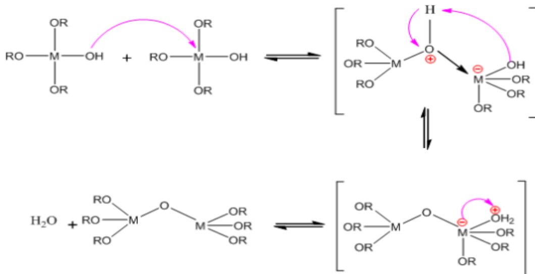
Fig.II.4 Mécanisme d'oxolation des alcoxydes métalliques M(OR)_n
