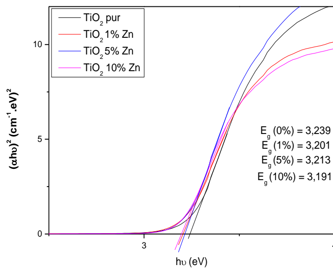
Fig.V.21 Energie de la bande interdite obtenue en extrapolant la partie linéaire de la courbe (\alpha h\nu)^2 en fonction de l'énergie des photons (eV) des nanoparticules de TiO 2 pur et de TiO 2 dopé au Zn
