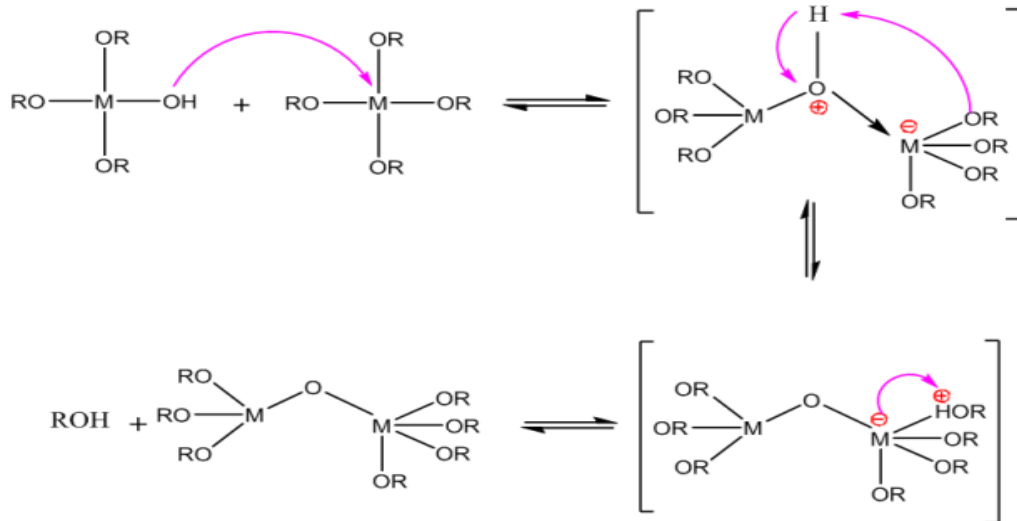
Fig.II.3 Mécanisme d'alcoylation des alcoxydes métalliques M(OR)_n [4]
