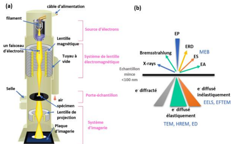
Fig.III.5 (a) : Schéma du principe de fonctionnement d'un Microscope Electronique à Transmission, (b) : Interactions électrons-matière dans une cible mince
