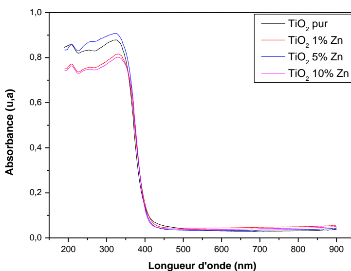
Fig.V.20 Spectres d'absorbance des nanopoudres de TiO 2 pur et dopé au Zn
