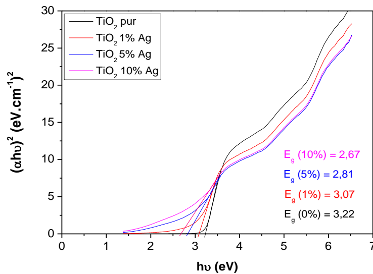
Fig.V.10 Bande interdite obtenue en extrapolant la partie linéaire de la courbe (\alpha h\nu)^2 en fonction de l'énergie des photons (eV) des nanoparticules de TiO 2 et de TiO 2 dopé à l'Ag
