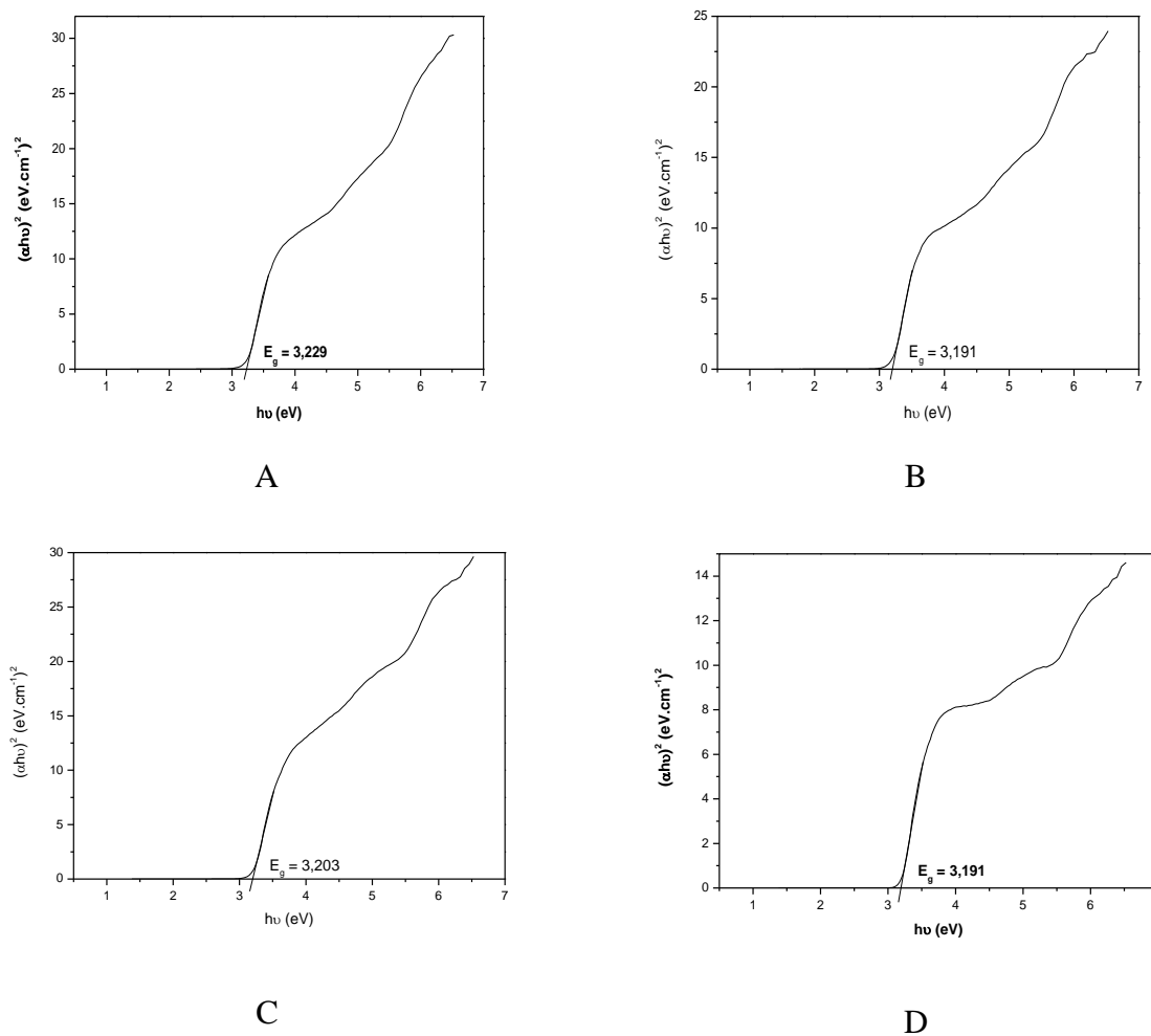
Fig.V.22 Détermination de l'énergie de la bande des nanoparticules de \text{TiO}_2 pur (A) et de \text{TiO}_2 dopé au Zn : 1% (B), 5% (C) et 10% (D)
