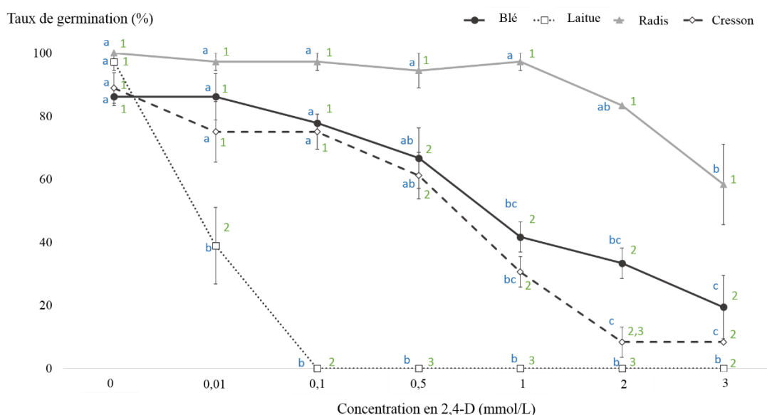
Figure II-22 – Taux de germination des graines de blé, laitue, radis, et cresson en fonction de la concentration en 2,4-D. Le taux de germination est exprimé comme la moyenne ± erreur type de la moyenne de 3 réplicats. Les lettres en bleu indiquent une différence significative (selon un test de Tukey au seuil \alpha = 0,05 %) entre les taux de germination des graines d'une espèce en fonction de la concentration en 2,4-D. Les chiffres en vert indiquent une différence significative (selon un test de Tukey au seuil \alpha = 0,05 ) entre les taux de germination obtenus pour les 4 espèces à une concentration donnée en 2,4-D.
