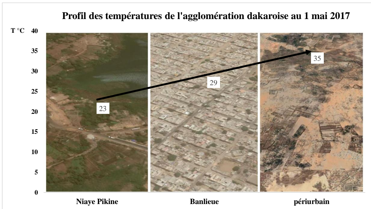
Figure 198 : Profil des températures de l'agglomération dakaraise au 1 mai 2017
