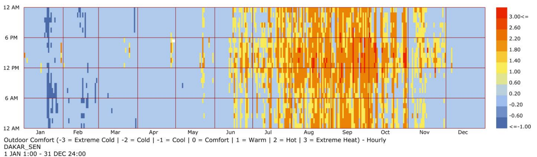
Figure 195 : Estimation du confort extérieur de la région de Dakar
