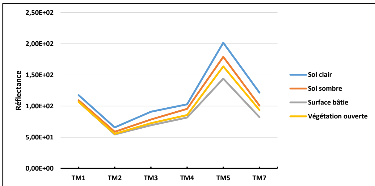
Figure 89 : Courbes radiométriques de la carte de l'occupation du sol de Touba, 1992
