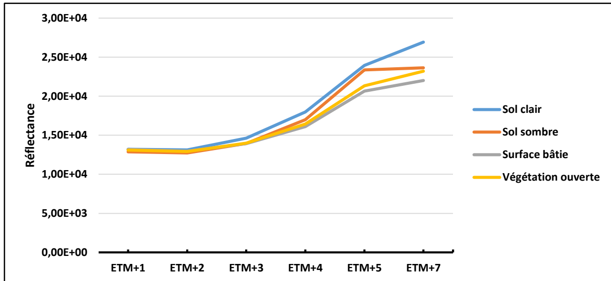
Figure 93 : Serpents radiométriques de la carte de l'occupation du sol de Touba, 2017
