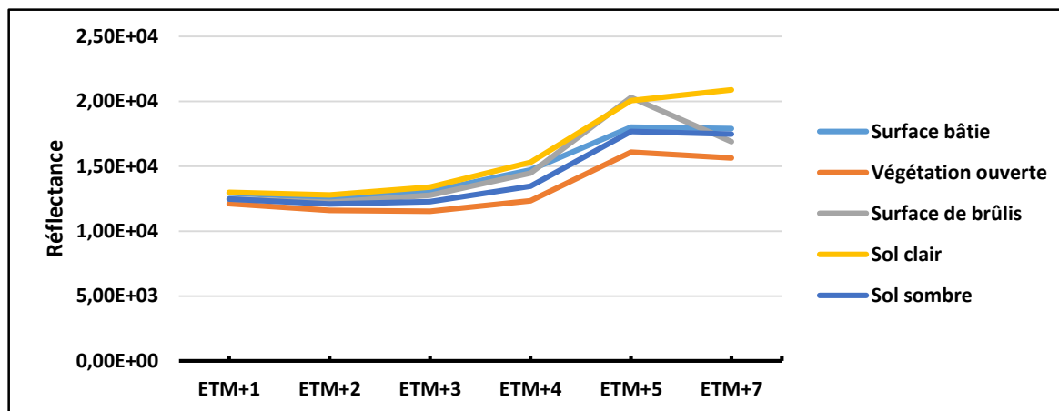
Figure 127 : Courbes radiométriques de la carte de l'occupation de Tambacounda, 2017
