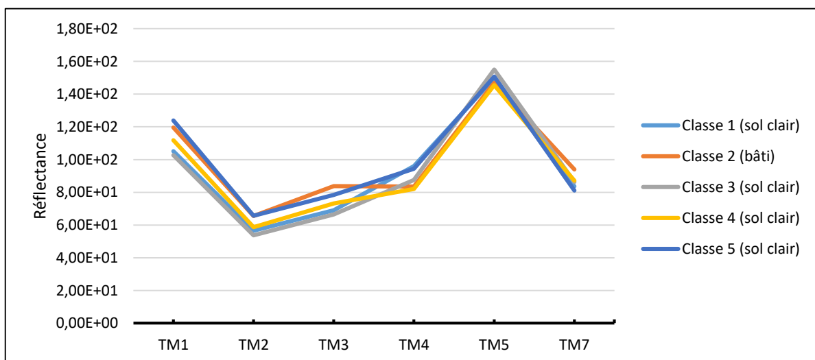
Figure 64 : Courbes radiométriques de la classification non dirigée de la sous-classe 2
