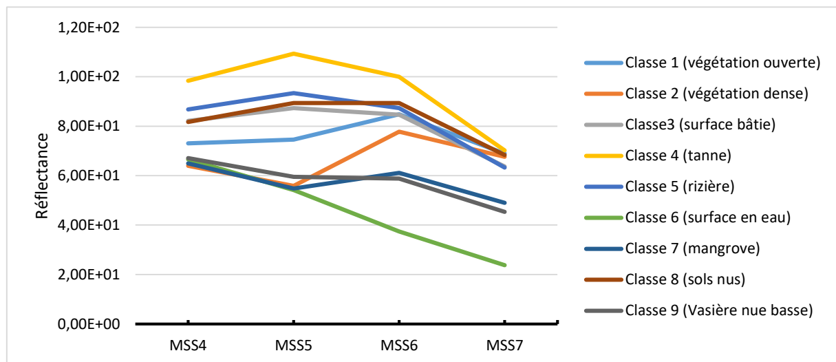
Figure 105 : Courbes radiométriques de la carte de l'occupation du sol de Ziguinchor, 1973
