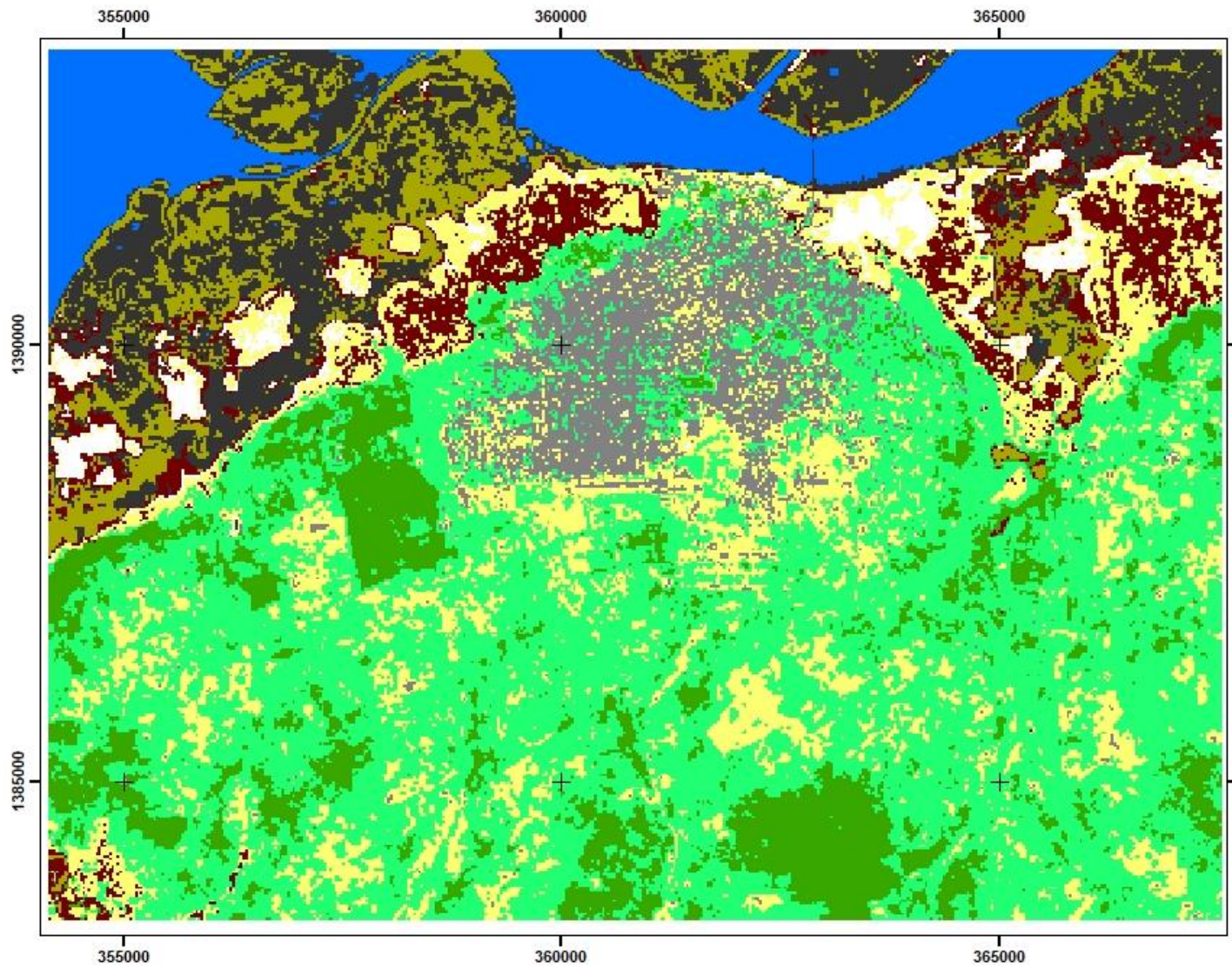
Figure 110 : Cartographie de l'occupation du sol de la ville de Ziguinchor et ses environs, 1990
