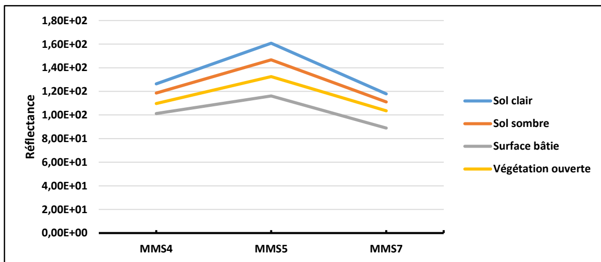
Figure 87 : Courbes radiométriques de la carte de la couverture du sol de Touba, 1973
