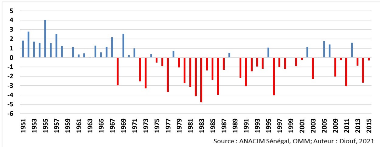
Figure 41 : Évolution de l'indice standardisé des précipitations entre 1951 et 2015 à Diourbel (Touba)
