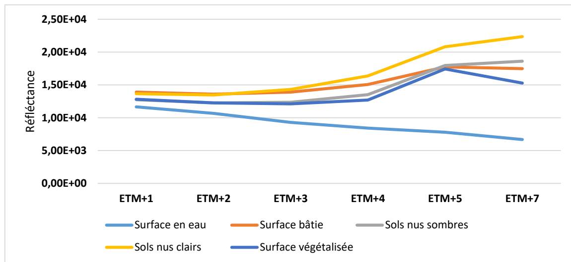
Figure 73 : Courbes radiométriques de la carte de l'occupation du sol de Dakar, 2017
