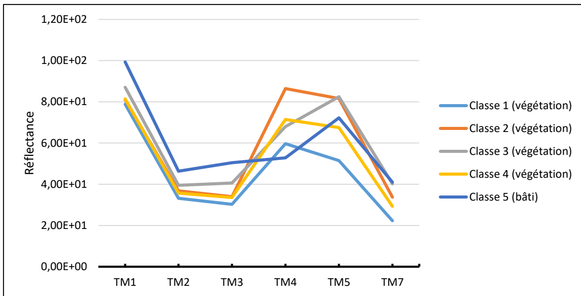
Figure 63 : Courbes radiométriques de la classification non dirigée du masque de la classe 9
