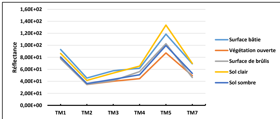
Figure 125 : : Courbes radiométriques de la carte de l'occupation de Tambacounda, 1990
