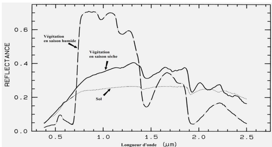
Figure 52 : Courbes de réflectance de la végétation et du sol. Source : Clark, in Rencz ed. 1999
