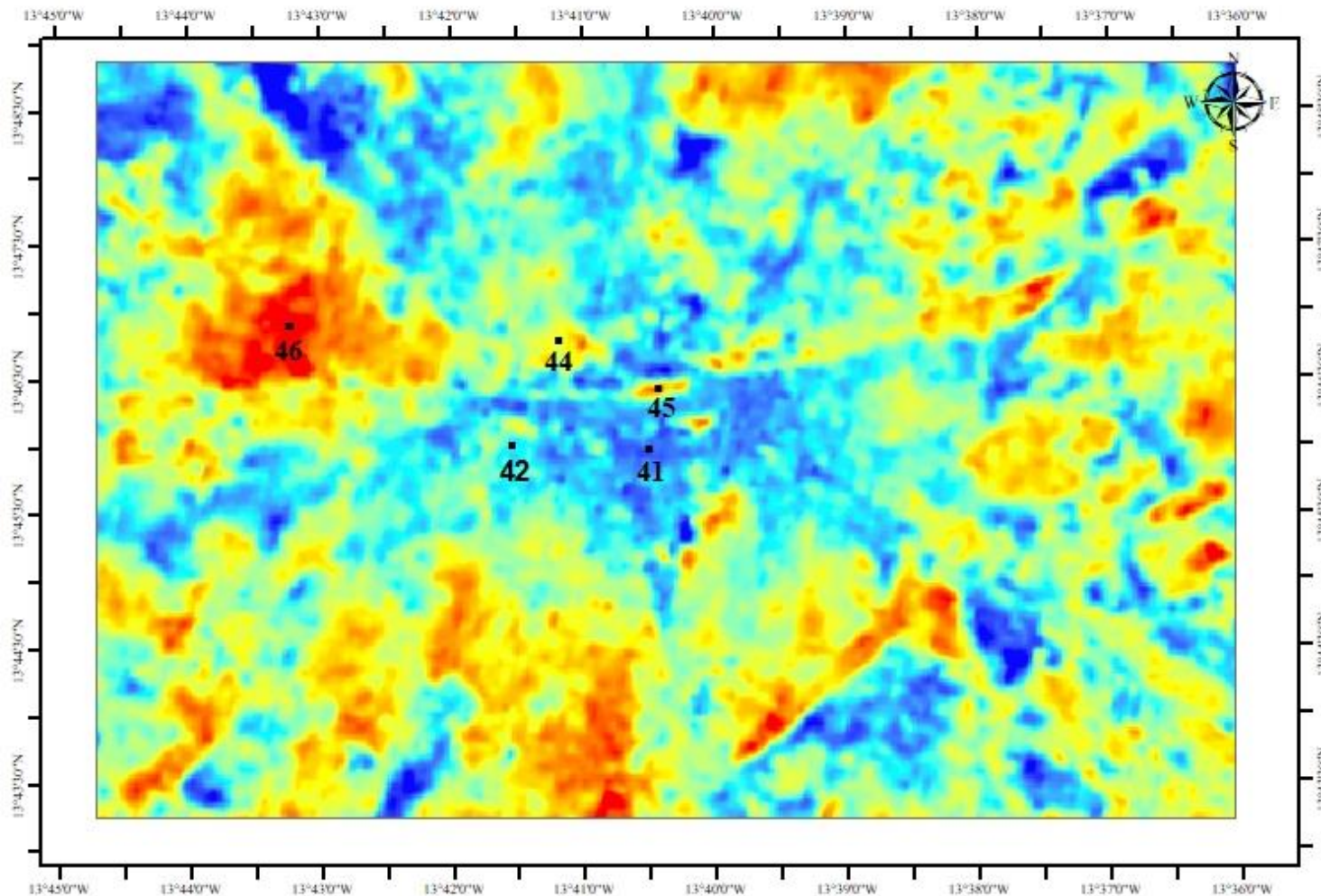
Figure 208 : Carte des températures de la ville de Tambacounda du 21 avril 2017
