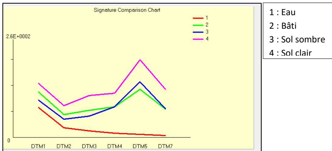
Figure 62 : Courbes radiométriques des quatre classes obtenues après regroupement des classes homogènes
