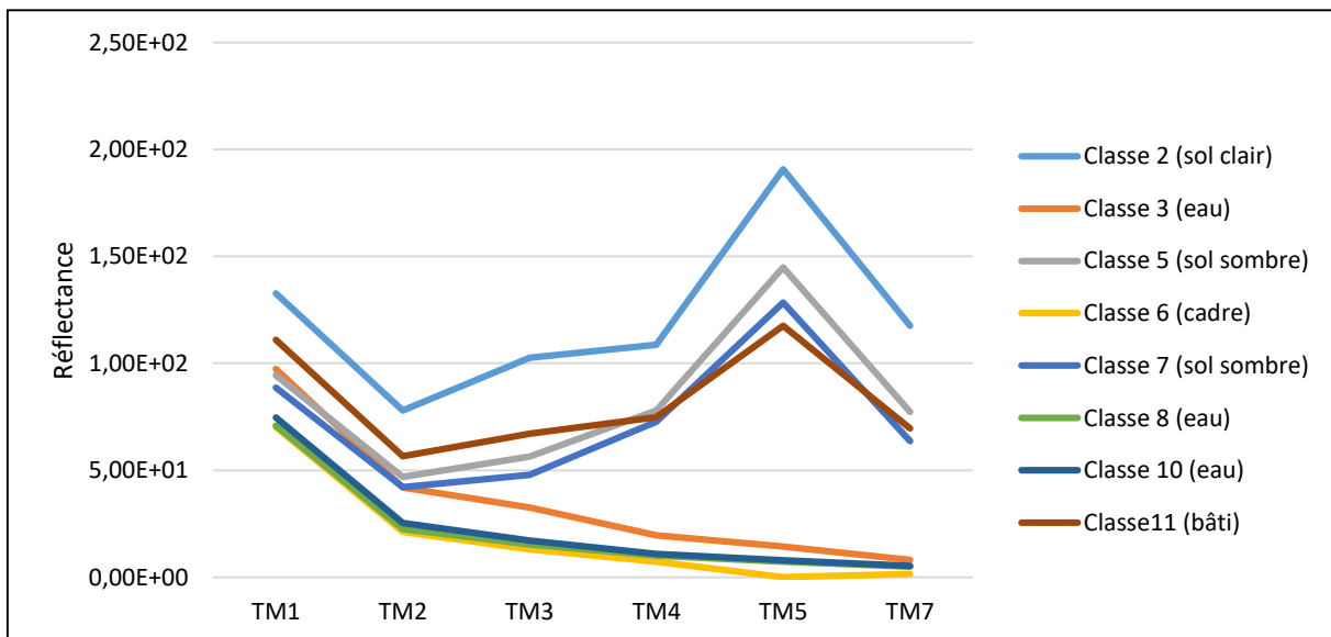
Figure 61 : Courbes radiométriques de la première classification (sans les classes hétérogènes)
