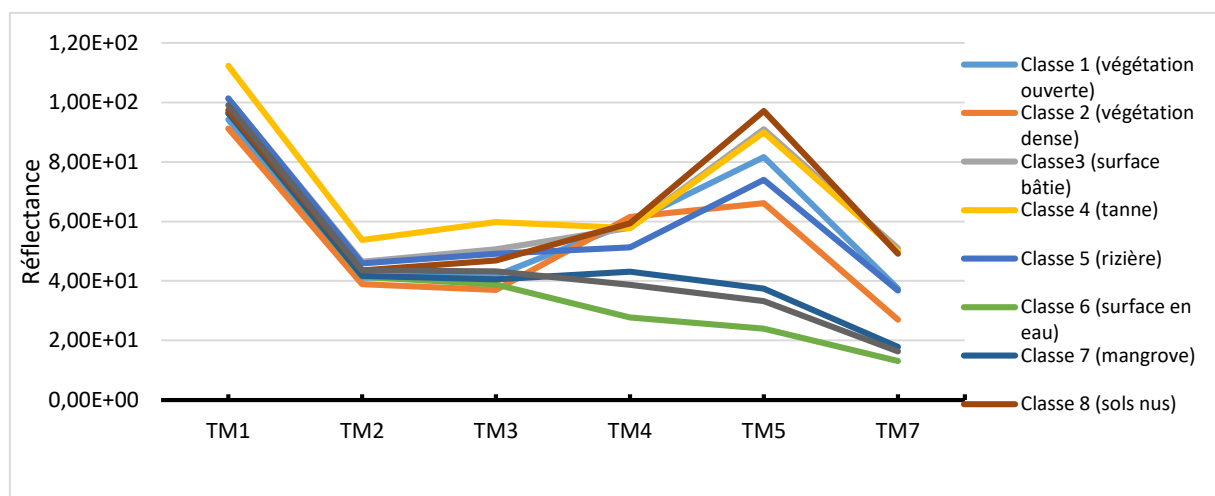
Figure 108 : Courbes radiométriques de la carte d'occupation du sol de Ziguinchor, 1990
