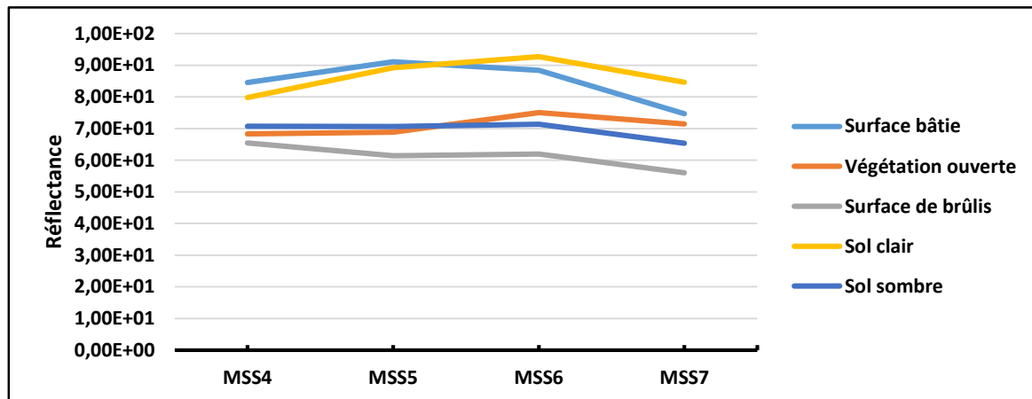
Figure 123 : : Courbes radiométriques de la carte de l'occupation du sol à Tambacounda, 1973
