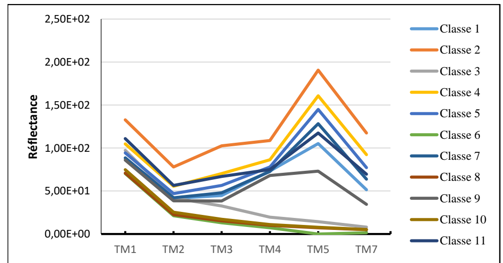
Figure 60 : Première classification en nuées dynamiques (K 15) et leurs réponses radiométriques
