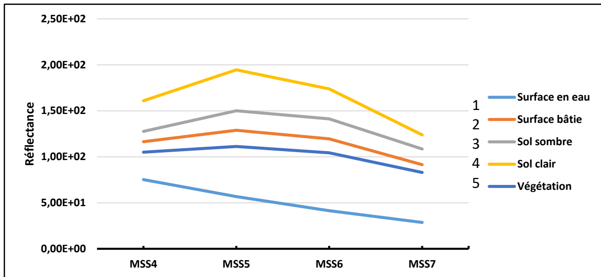
Figure 69 : Courbes radiométriques de la carte de l'occupation du sol de Dakar, 1973
