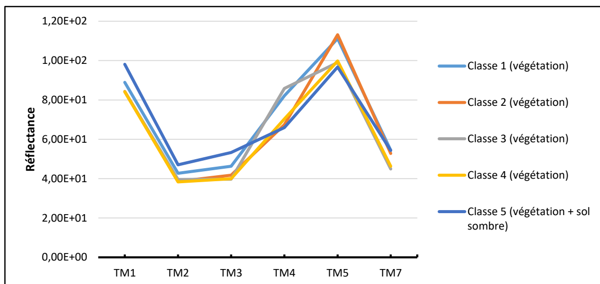
Figure 65 : Courbes radiométriques du masque de la classe 1
