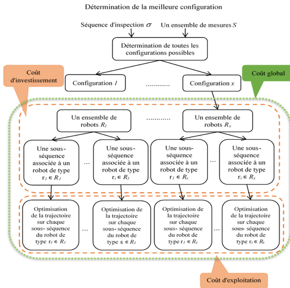
Figure 4. 4 : Une approche en 3 étapes pour optimiser la patrouille d'inspection
