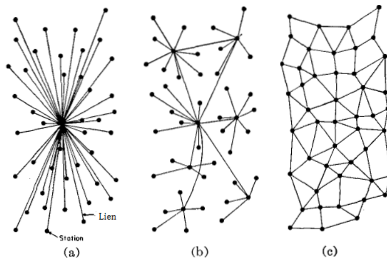
Figure 2. 12 : Types des approches : (a) centralisée (b) décentralisée (c) distribuée.
