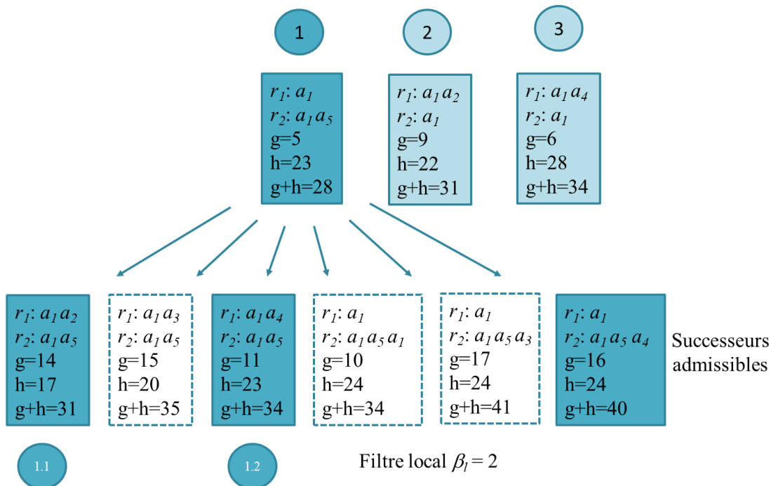
Figure 5. 8 : Méthode d'optimisation : deuxième étape
