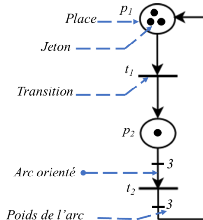
Figure 4. 2 : Réseau de Petri généralisé
