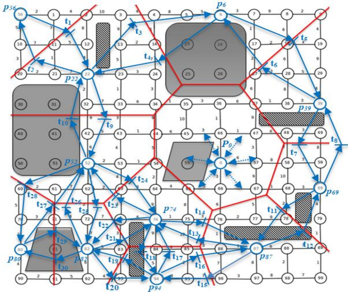
Figure 4. 6 : Décomposition de Voronoï et extraction du modèle par réseau de Petri
