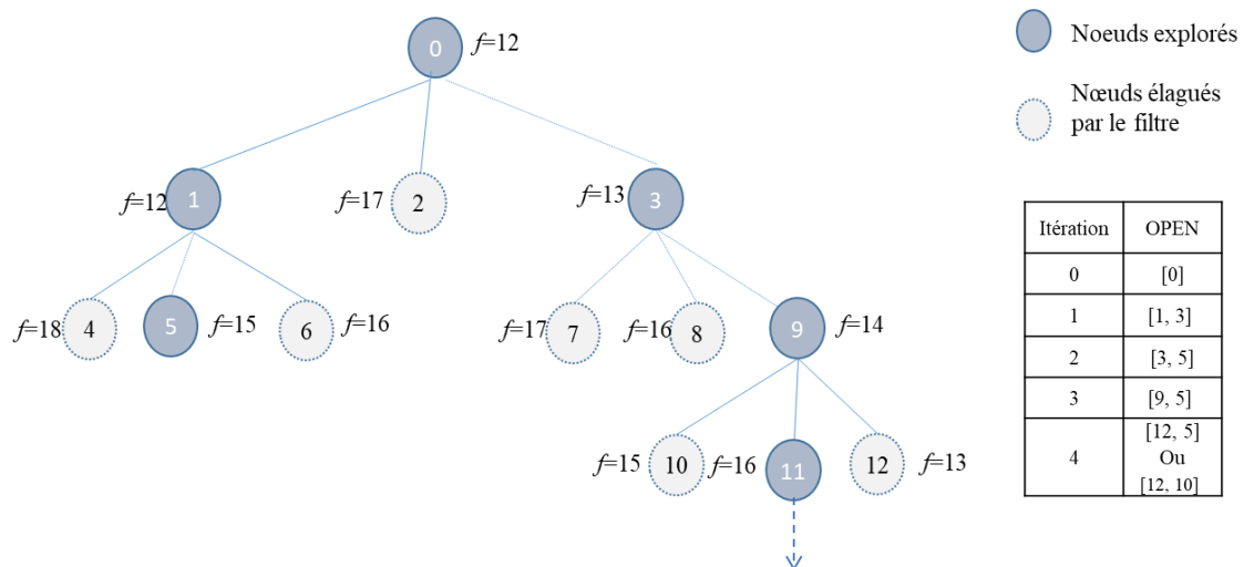
Figure 3. 5 : Exploration de l'arbre de recherche avec l'algorithme BS pour \beta = 2
