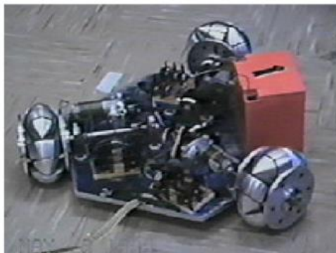
Figure 2. 9 : Exemple de plate-forme omnidirectionnelle à roues suédoises.
