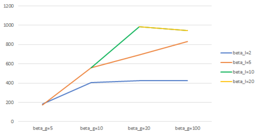
Figure 5.14 : Analyse de la complexité pour différentes valeurs des paramètres \beta_g et \beta_l .
