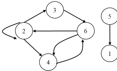
Figure 5. 3 : Un exemple de graphe orienté non élémentaire
