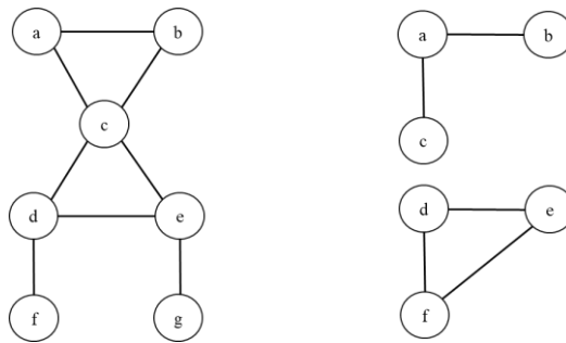
Figure 5. 4 : Exemples de graphe connexe (à gauche) et non connexe (à droite)
