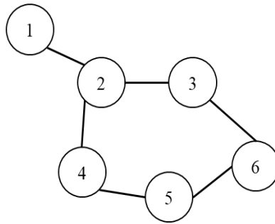
Figure 5. 2 : Un exemple de graphe simple non orienté
