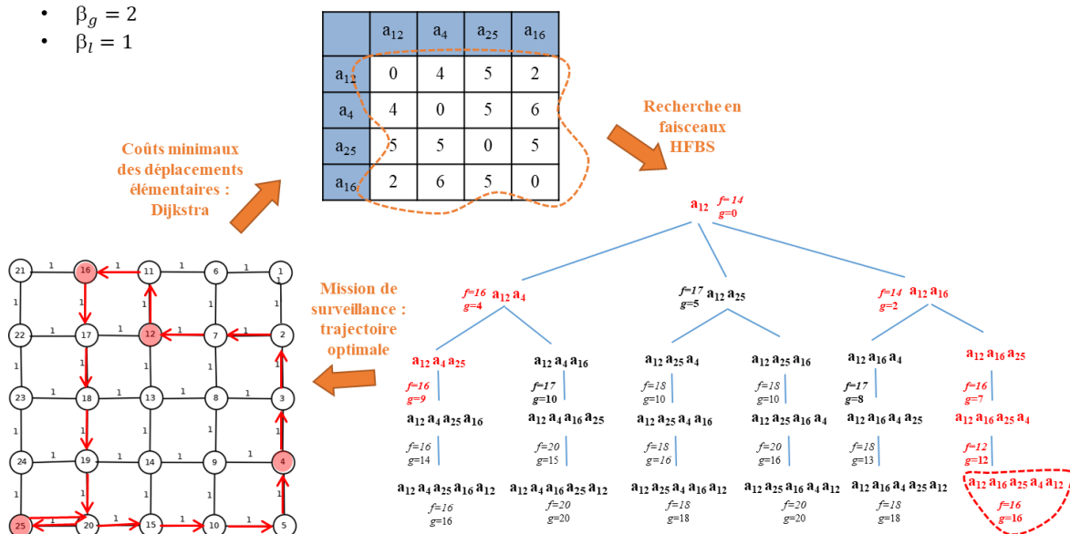
Figure 5. 1 : Graphe d'optimisation combinant les algorithmes HFBS et l'algorithme de Dijkstra.
