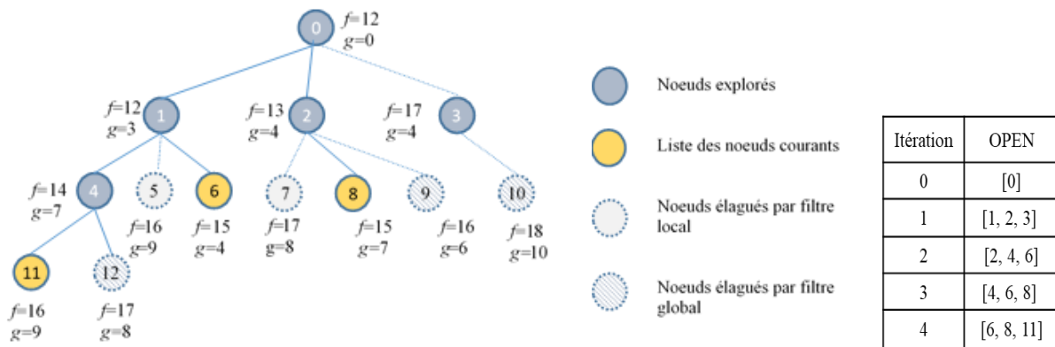
Figure 3. 6 : Exploration de l'arbre de recherche avec la méthode HFBS
