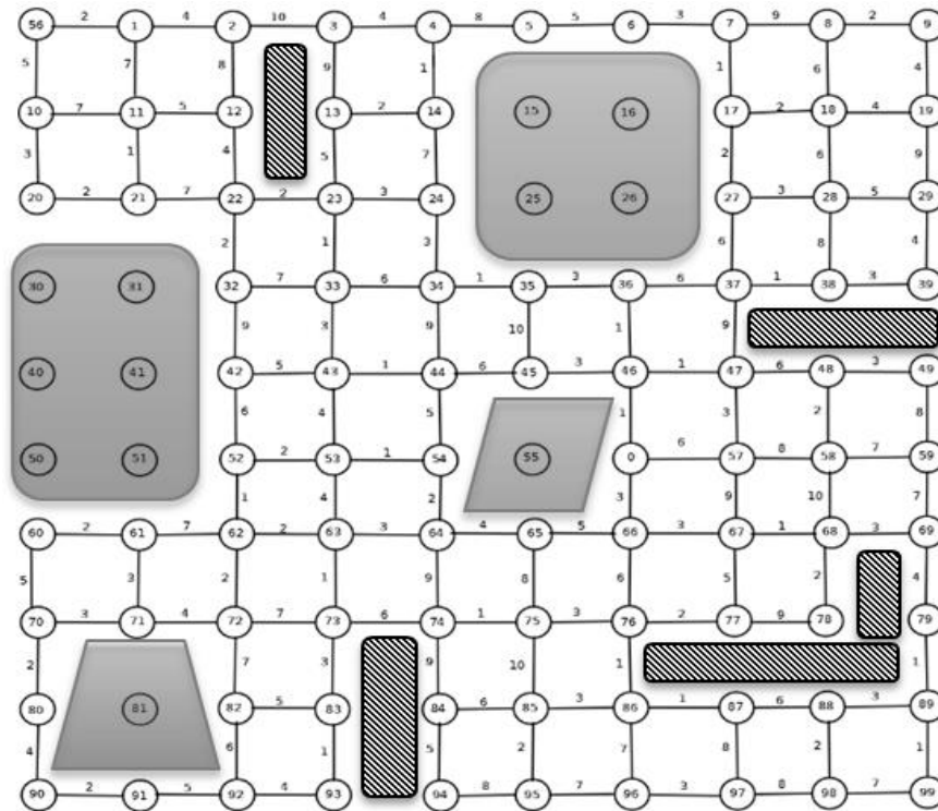
Figure 4. 3 : Un exemple d'environnement sous la forme d'un graphe d'états
