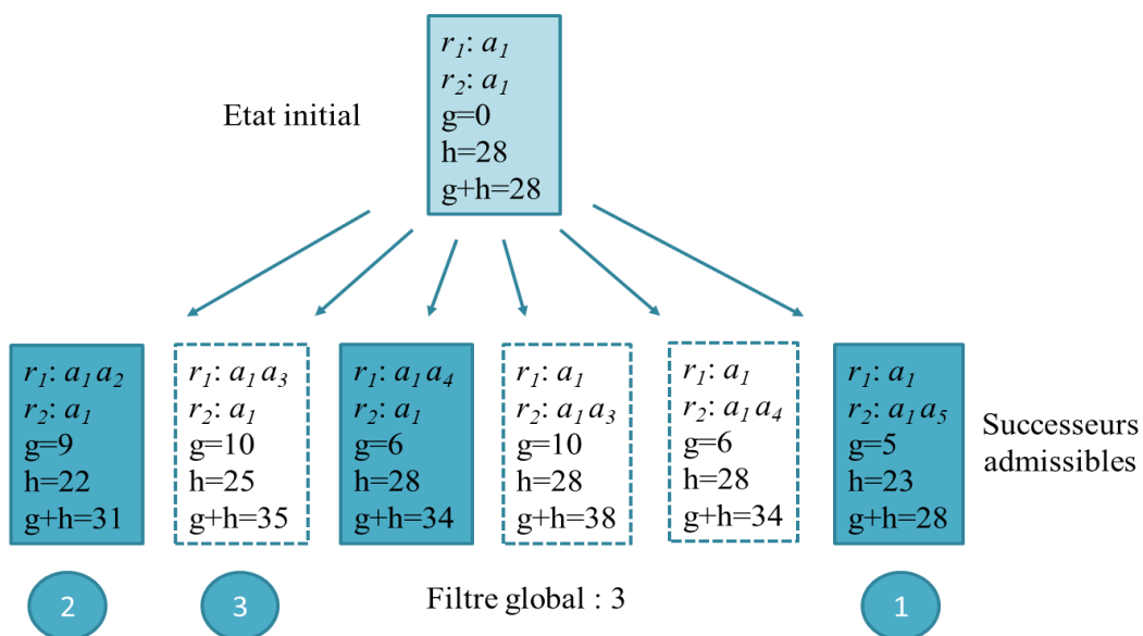
Figure 5. 7 : Méthode d'optimisation : première étape
