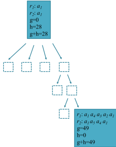
Figure 5. 9 : Méthode d’optimisation : vue d'ensemble
