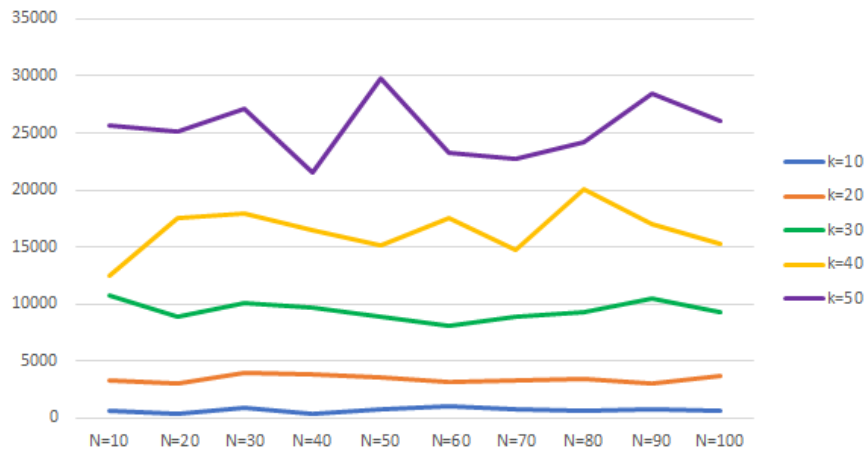
Figure 5.13 : Analyse de la complexité pour différentes valeurs des paramètres k et de N .
