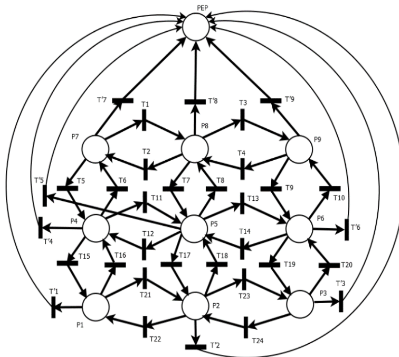
Figure 4. 8 : Modèle PN de l'environnement de la Fig. 4. 7
