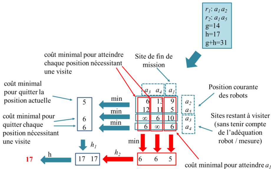
Figure 5. 10 : Détail de la fonction heuristique h(S)
