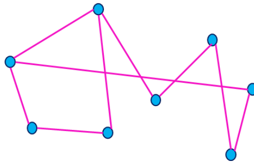
Figure 3. 1 : Exemple de solution du TSP
