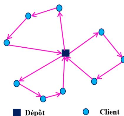
Figure 3. 2 : Exemple de solution du VRP
