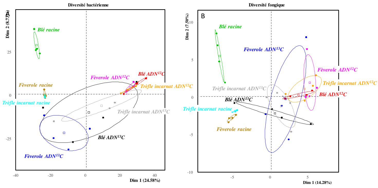
Figure 39 : Analyse en composantes principales de l'effet du couvert végétal sur la diversité bactérienne (A) et fongique (B) dans les fractions d'ADN 12 C et 13 C ainsi dans les racines.
