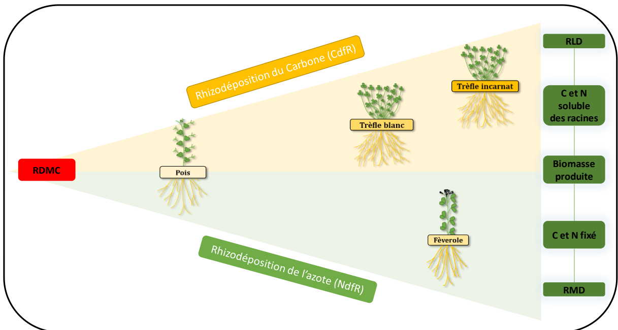
Figure 34 : Principales relations entre traits fonctionnels et la rhizodépôt de C et l’N.
