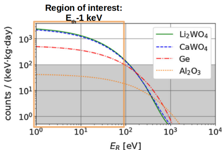
Figure 1: Taux de comptage différentiel \text{CE}\nu\text{NS} sur \text{Li}_2\text{WO}_4 (ligne verte), \text{CaWO}_4 (ligne bleue), germanium (ligne rouge) et \text{Al}_2\text{O}_3 (ligne orange pointillée), calculé avec le flux d'anti-neutrinos attendu sur le site expérimental. L'expérience NUCLEUS vise à atteindre un taux de comptage du bruit de fond de 100 coups/(keV kg jour) (bande grise) [1].
