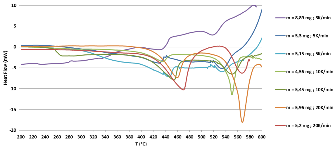
Figure 58 : Résultats des analyses DSC sur le SrO 2 sous argon à différentes rampes en température.
