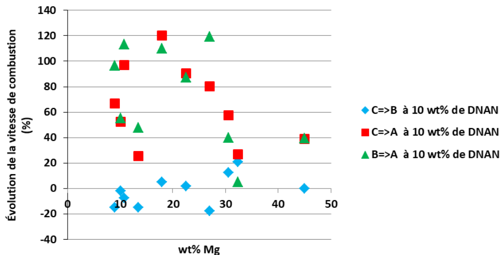
Figure 102 : Taux d'évolution de la vitesse de combustion d'une classe granulométrique à l'autre des compositions à 10 wt% de DNAN.
