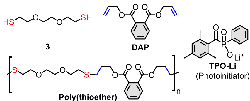
Schéme IV-1 Structure chimique des monomères diène et dithiol DAP et 3 , photoamorceur radicalaire hydrosoluble (TPO-Li) et poly(thioéther) dérivé de la polyaddition DAP-3 .
