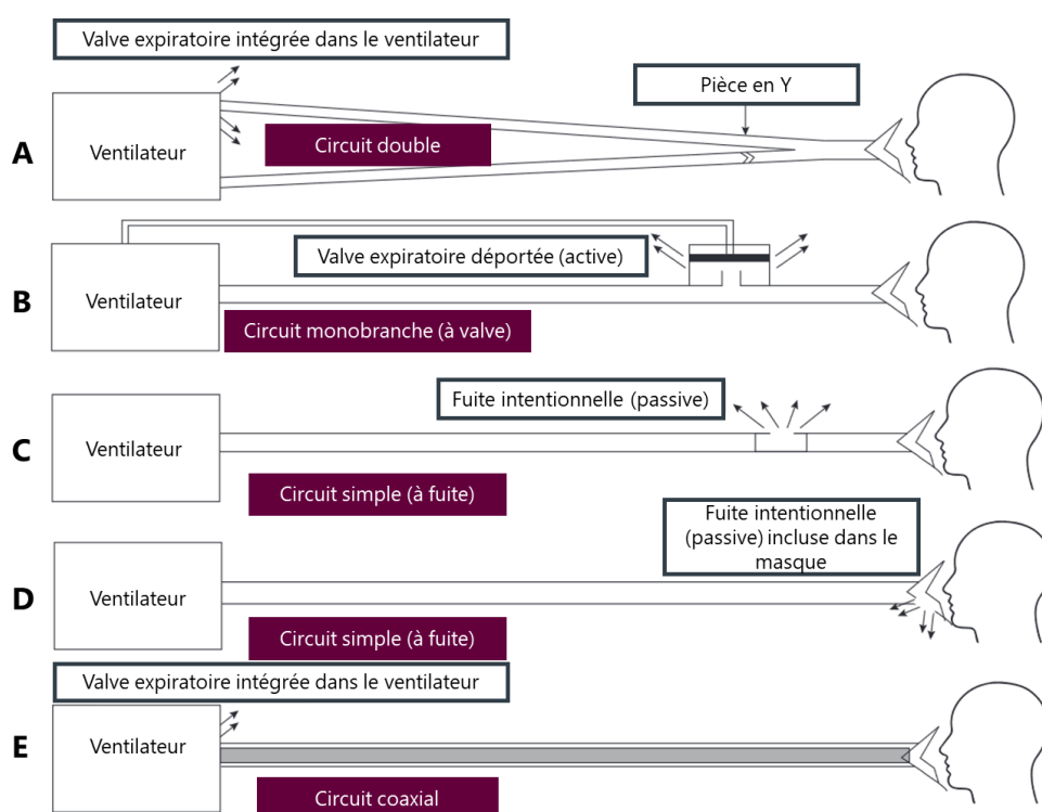
Figure 13. Principales configurations de circuits pour la ventilation non-invasive.
