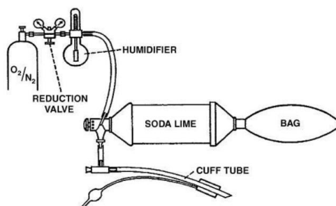
Figure 5. Dispositif de ventilation utilisé pendant l'épidémie de poliomyélite à Copenhague, 1952. Lassen HCA. Lancet, 1953 [13]
