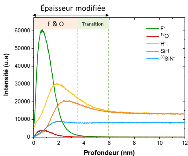
Figure V-11 – Profil de composition en profondeur d'une couche de SiN PECVD modifiée avec un plasma H 2 pendant 60s, obtenus par ToF-SIMS.
