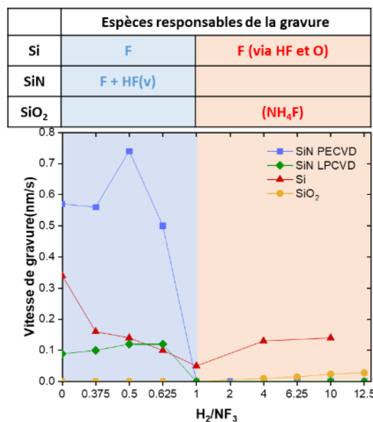
Figure IV-14 – Vitesses de gravure du SiN PECVD, LPCVD, SiO 2 et Si selon différents ratios H 2 /NF 3 à 60 °C et espèces supposées responsables de la gravure.
