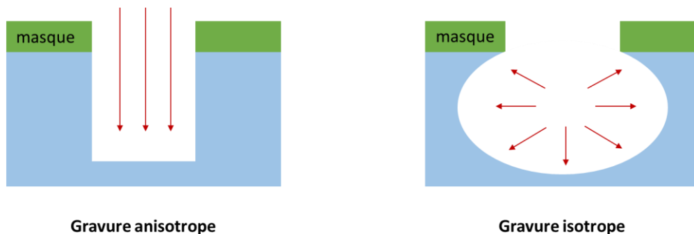
Figure I-3 – Différence entre la gravure anisotrope et isotrope.
