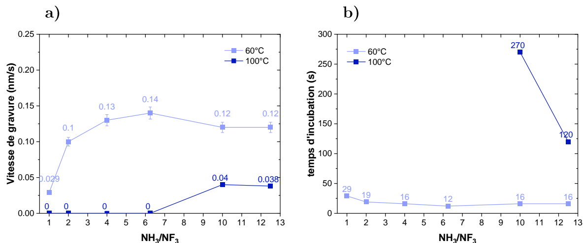
Figure IV-27 – a) Vitesse de gravure et b) temps d'incubation mesurés sur SiN PECVD à 60 et 100 °C dans un plasma délocalisé de type NF 3 /NH 3 /He (1 Torr, 250 W).
