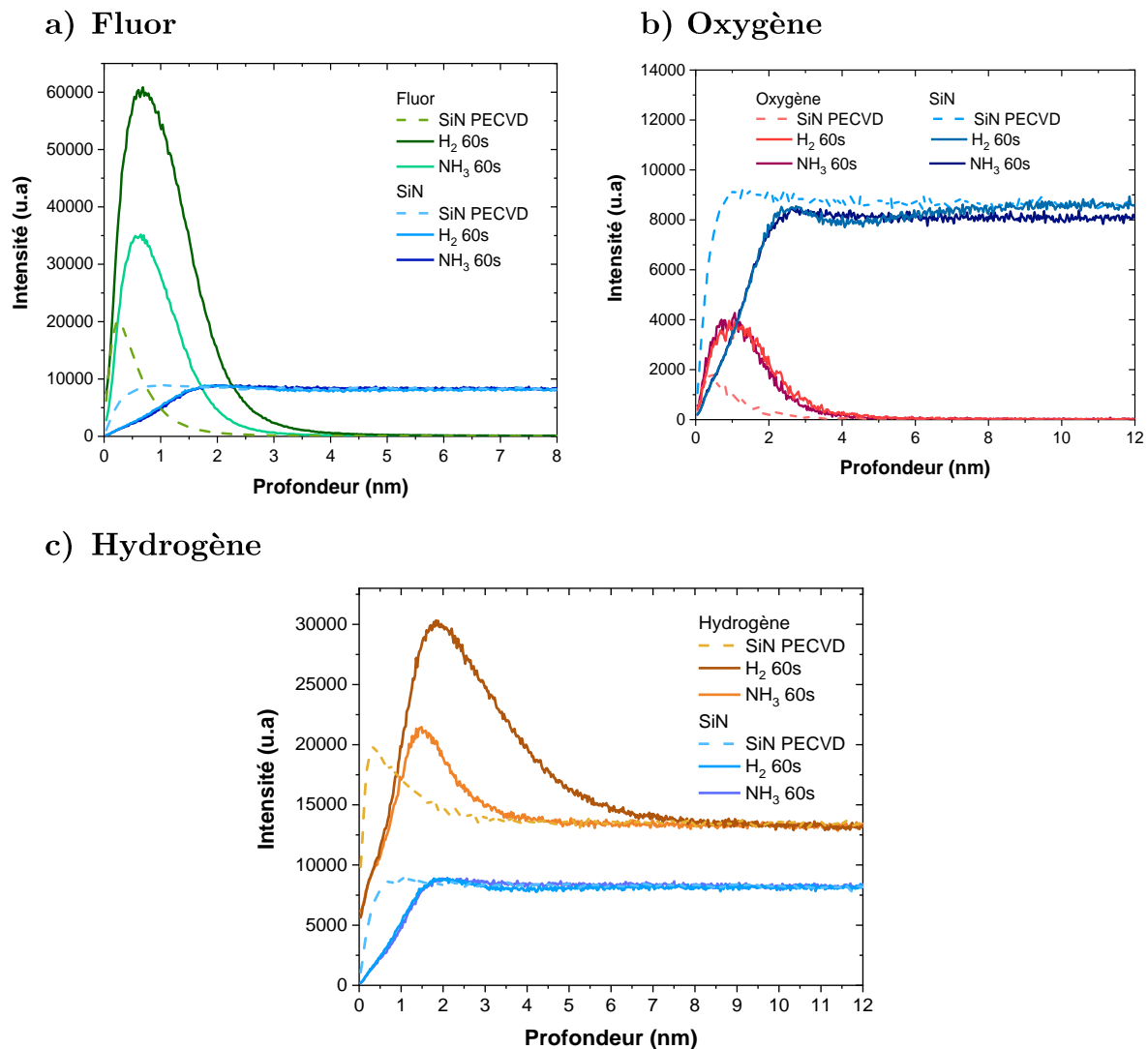
Figure V-19 – a) Profils de composition en profondeur en a) fluor, b) oxygène et c) hydrogène d'une couche de SiN PECVD modifiée avec un plasma H 2 ou NH 3 pendant 60 s, obtenus par ToF-SIMS.
