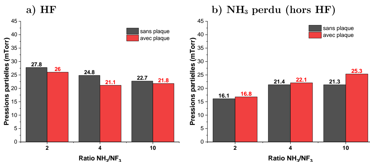
Figure IV-31 – Pressions partielles de a) HF et de b) NH 3 perdu avec ou sans plaque de SiN PECVD à 60 °C pour différents ratios.
