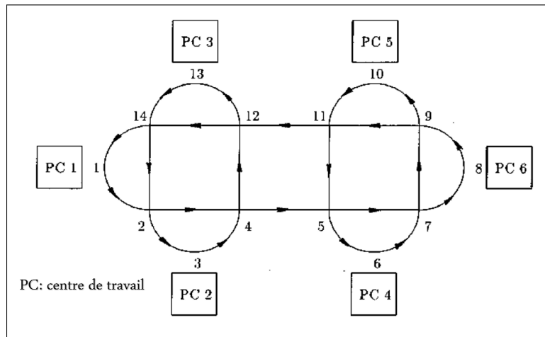
FIGURE 2.10 – Configuration du modèle traité par Rajotia et al. (1998)
