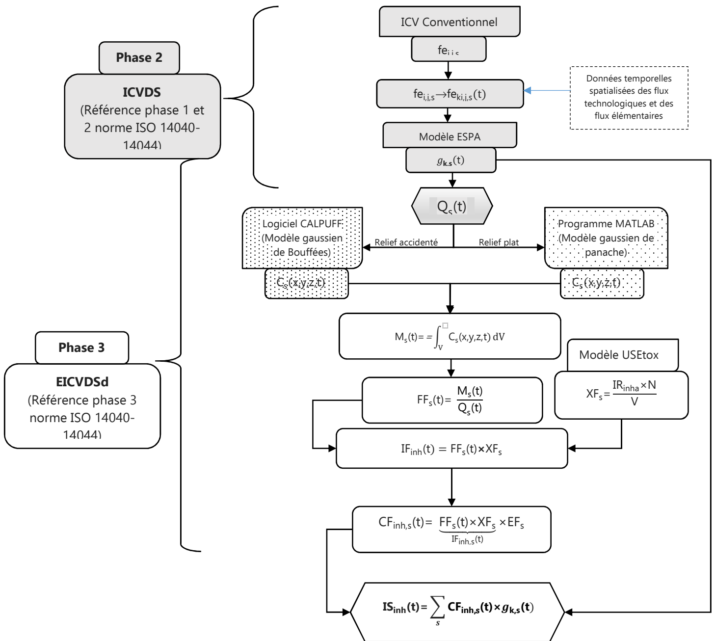
Figure II. 3 : Algorithme de l'ACVDSd
