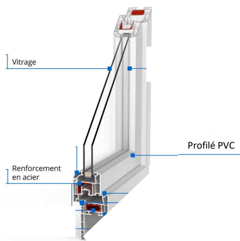
Figure III. 2 : Illustration d'une fenêtre double vitrage PVC (source : fenêtre24.com)
