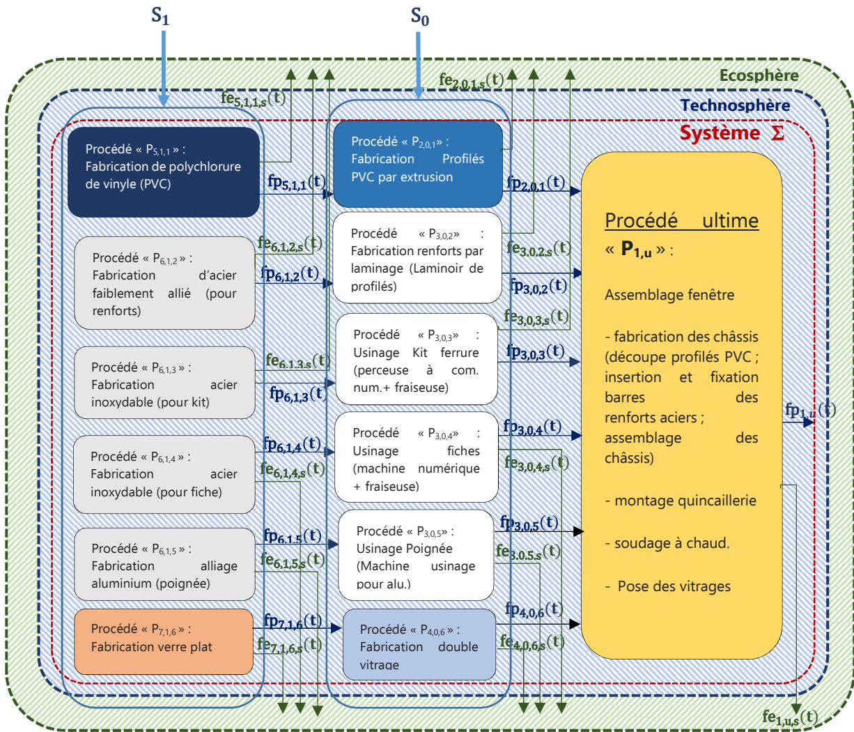
Figure III. 4 : Arbre de processus unitaire d'une baie PVC double vitrage d'1 m 2 de surface
