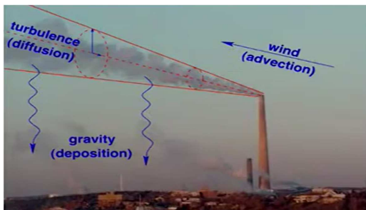
Figure I. 15 : Illustration des phénomènes physiques à modéliser lors d'une dispersion atmosphérique de polluants [Stockie, 2011]
