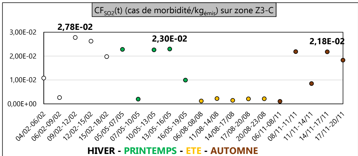
Figure III. 99 : CF SO 2 (t) (cas de morbidité/kg émis ) sur zone Z3-C
