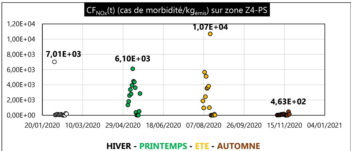
Figure III. 92 : CF NO x (t) (cas de morbidité/kg émis ) sur zone Z4-PS
