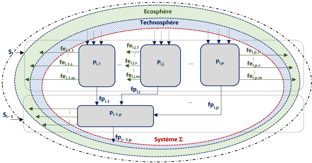
Figure I. 7 : Zoom sur un ensemble d'éléments de la chaîne des processus de la figure I. 6. Source : [Jolliet et al., 2005]
