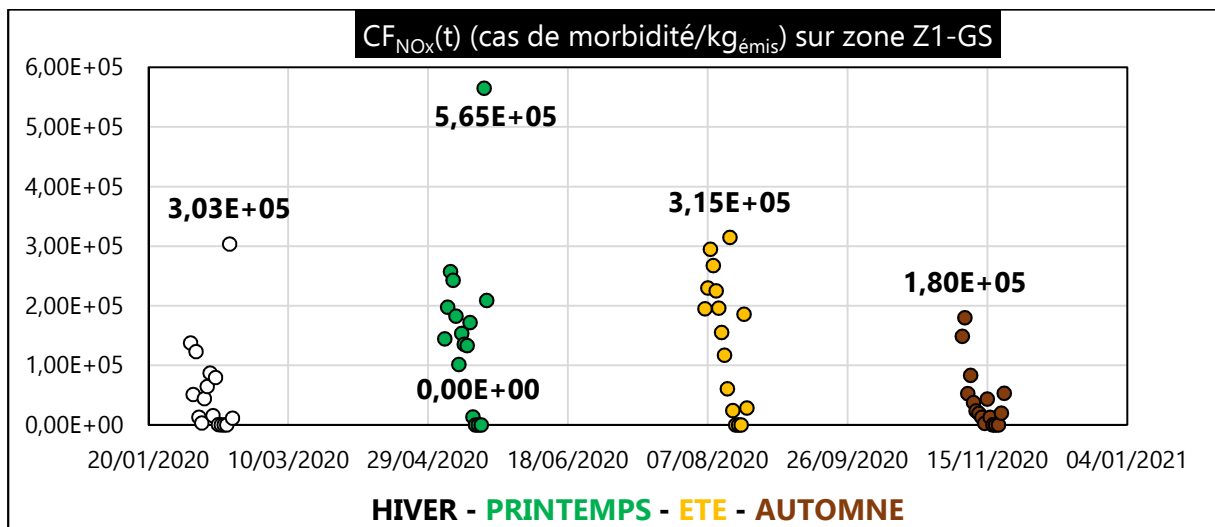
Figure III. 86 : CF_{NO_x}(t) (cas de morbidité/kg émis ) sur zone Z1-GS
