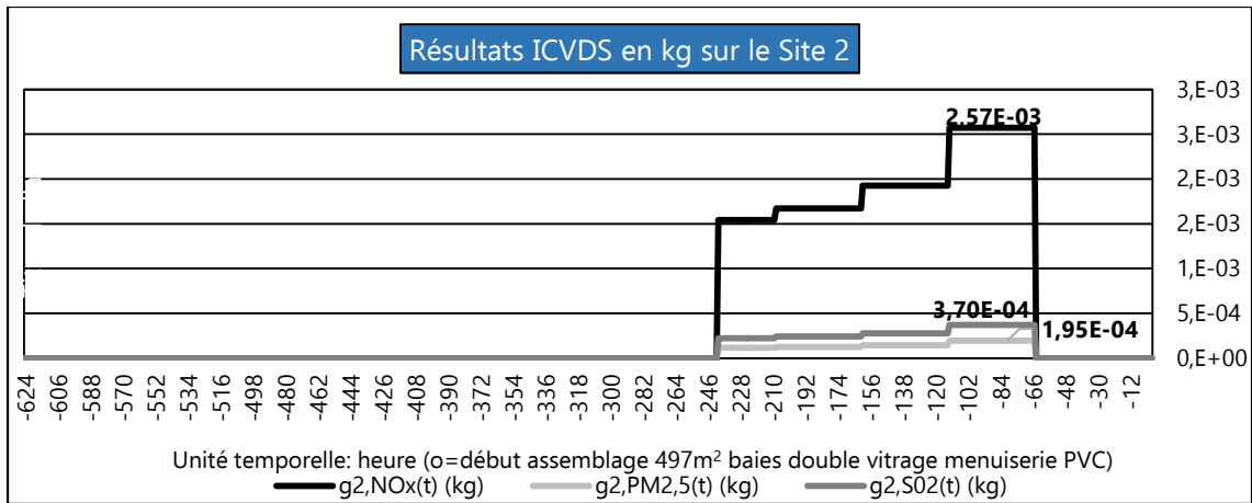
Figure III. 8 : Évolution temporelle g_{2,s}(t)
