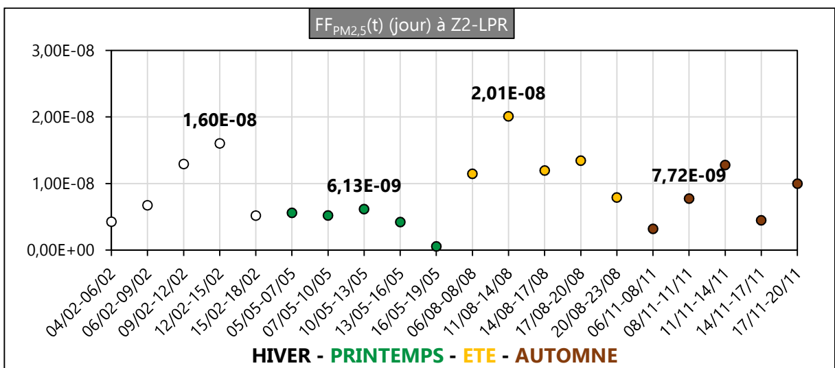
Figure III. 60 : FF PM2,5 (t) (jour) en zone Z2-LPR en 2020
