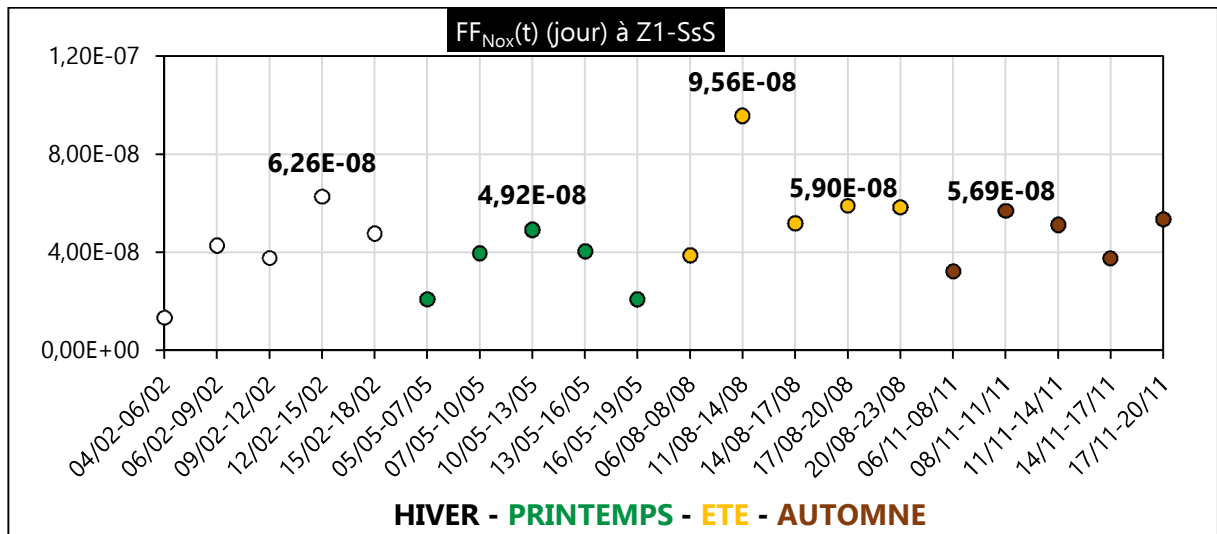
Figure III. 56 : \text{FF}_{\text{NO}_x}(t) (jour) en zone Z1-SsS en 2020
