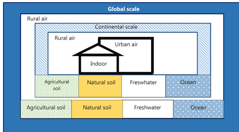
Figure I. 9 : Paramètres caractéristiques de certains compartiments. Source modèle USEtox [Henderson et al., 2011]
