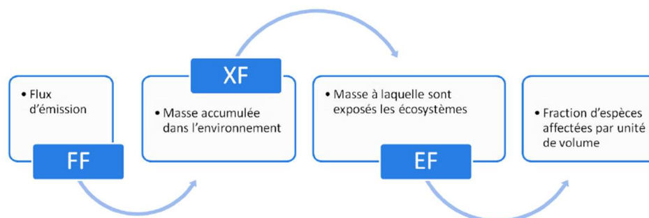
Figure I. 10 : Modélisation matricielle de la chaîne cause à effet dans USEtox [Rosenbaum et al., 2007]
