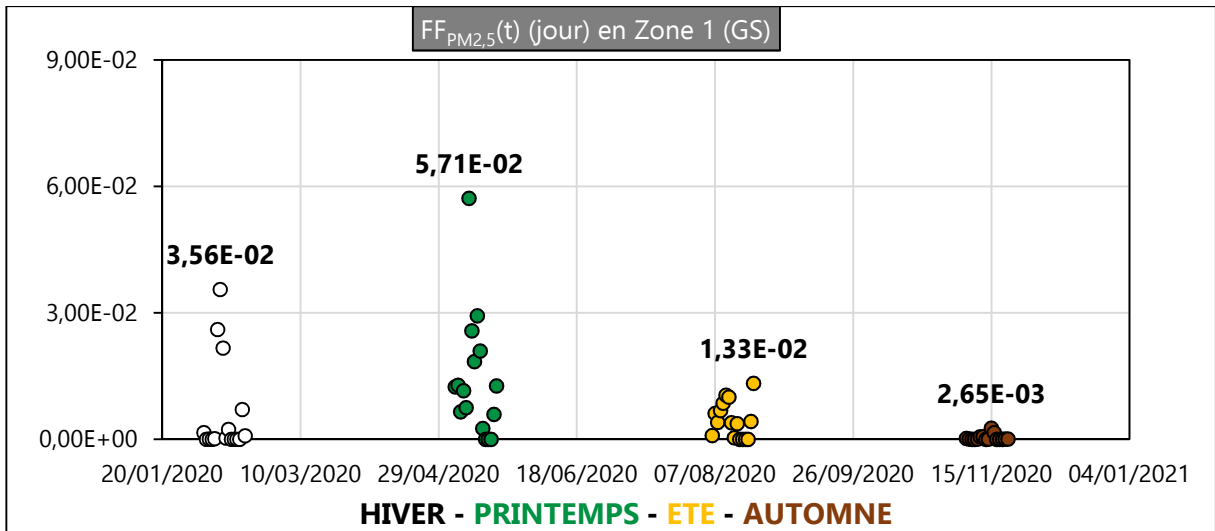
Figure III. 45 : FF PM 2,5 (t) (jour) en zone Z1-GS en 2020
