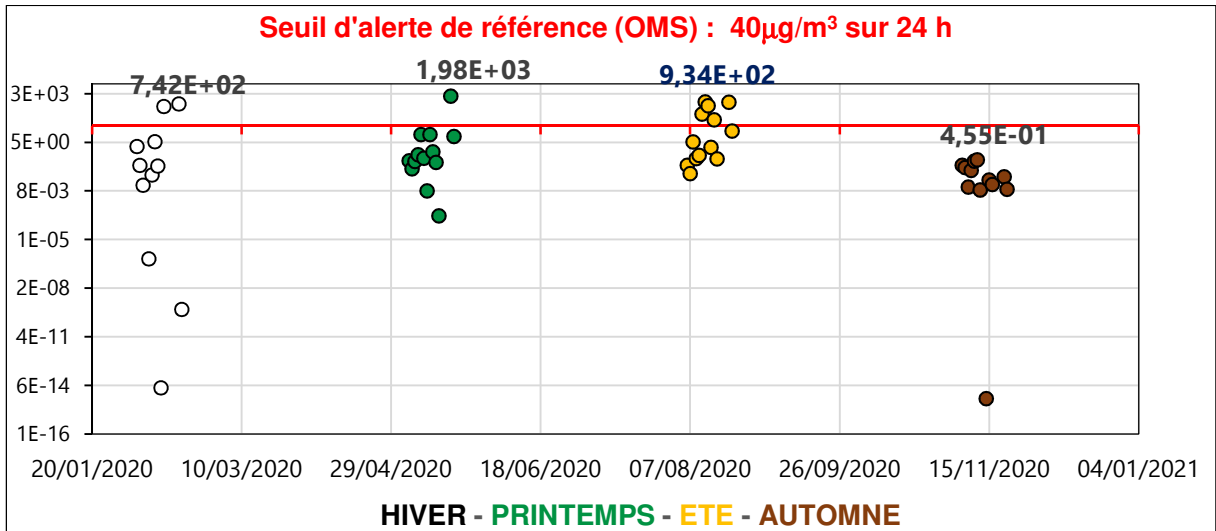
Figure III. 25 : Concentration potentielle moyenne/24h par saison de \text{SO}_2 ( \mu\text{g}/\text{m}^3 ) en zone Z2-FM en 2020
