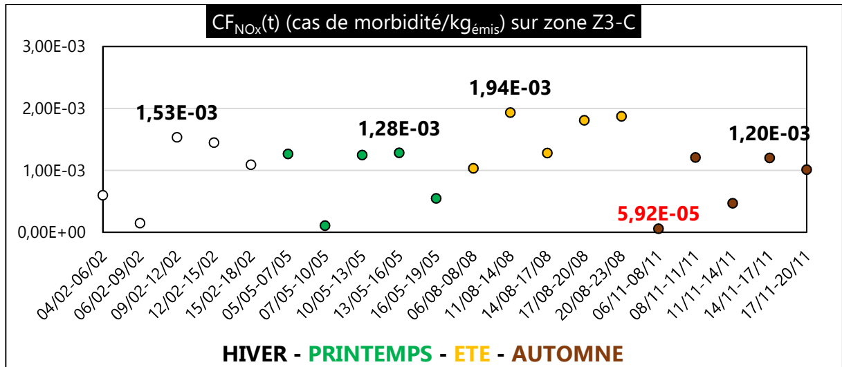
Figure III. 98 : CF NO x (t) (cas de morbidité/kg émis ) sur zone Z3-C
