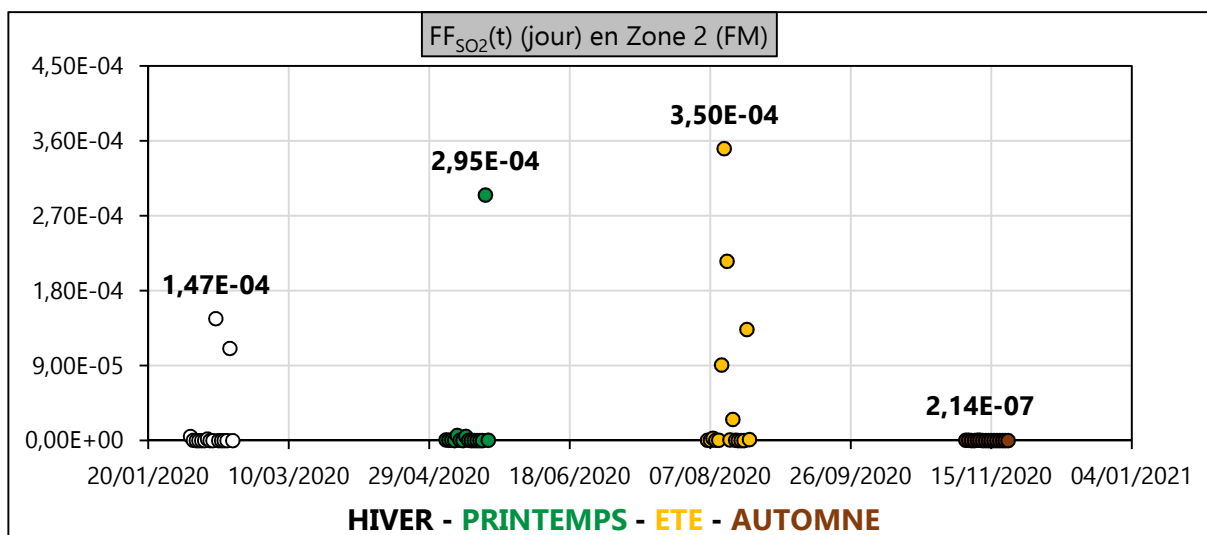
Figure III. 49 : FF SO2 (t) (jour) en zone Z2-FM en 2020
