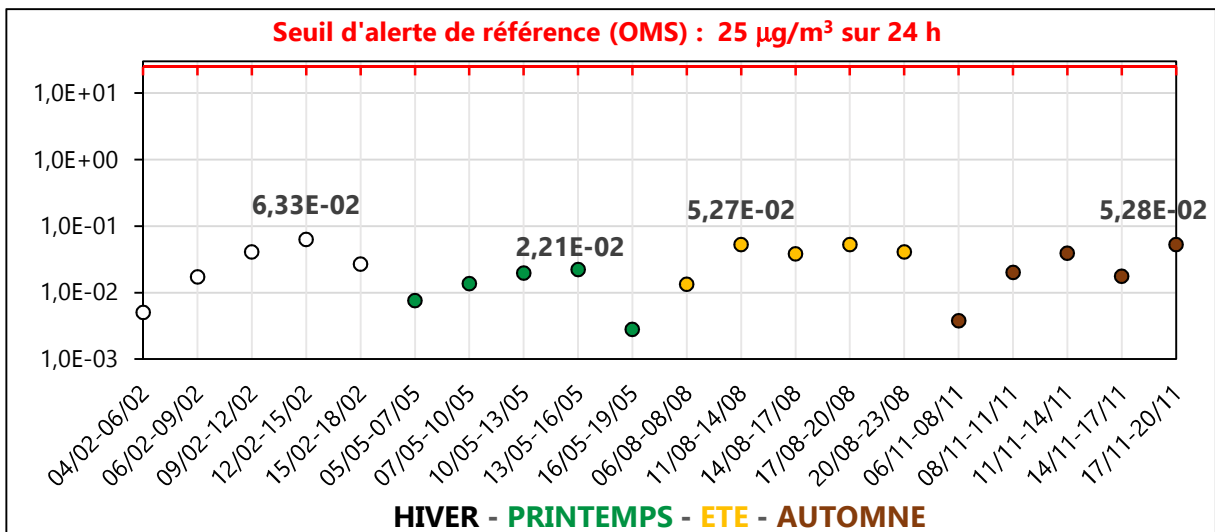
Figure III. 38 : Concentration potentielle moyenne/24h de NO x (µg/m 3 ) à Z2-LPR en 2020
