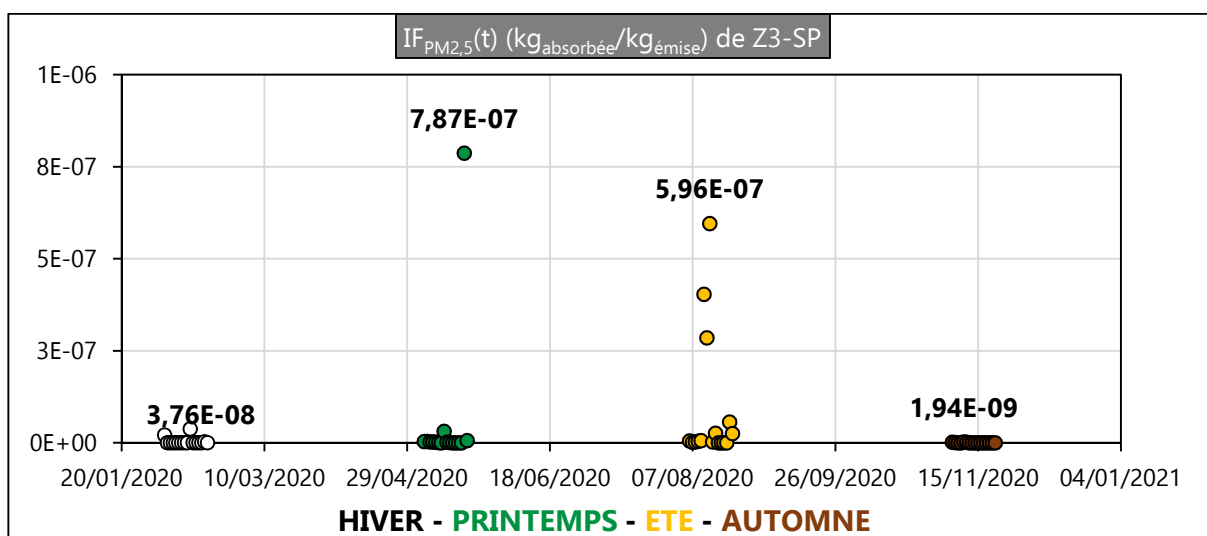
Figure III. 72 : IF PM2,5 (t) (kg absorbée /kg émise ) de Z3-SP en 2020
