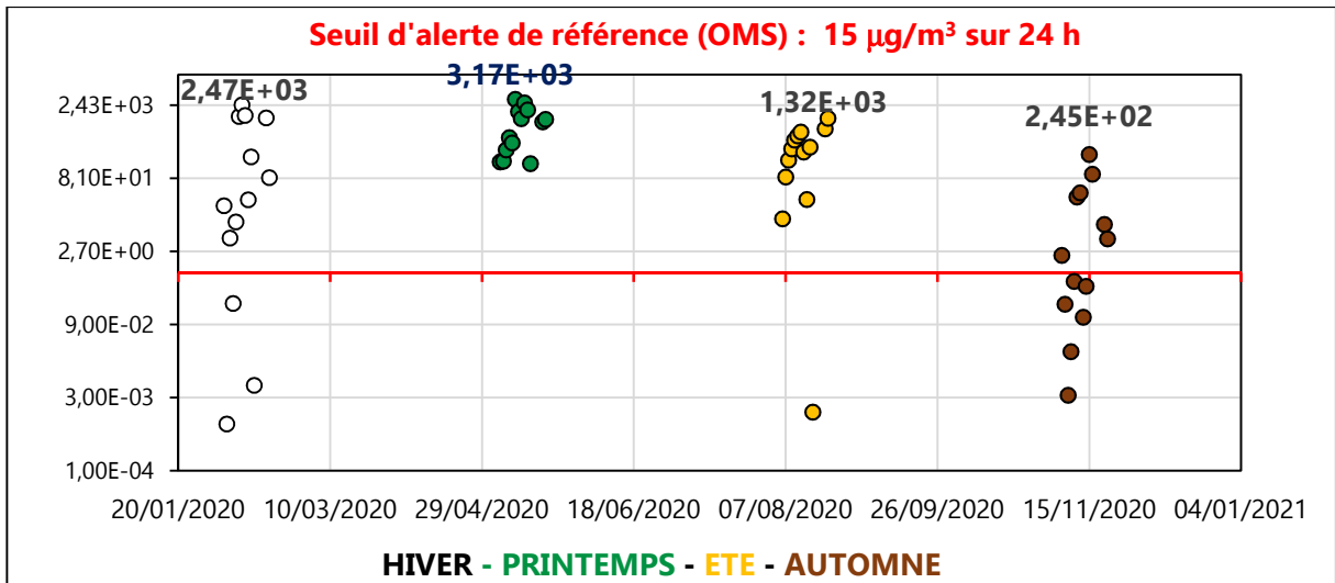
Figure III. 21 : Concentration potentielle moyenne/24h par saison de \text{PM}_{2,5} (Fe) ( \mu\text{g}/\text{m}^3 ) en zone Z1-GS en 2020
