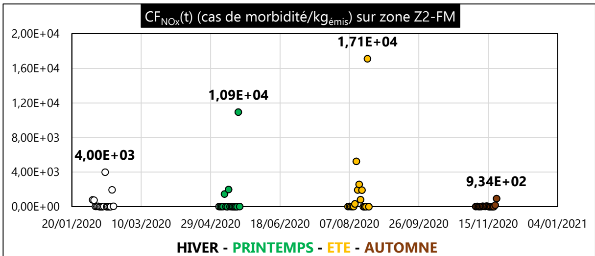
Figure III. 88 : CF NO x (t) (cas de morbidité/kg émis ) sur zone Z2-FM
