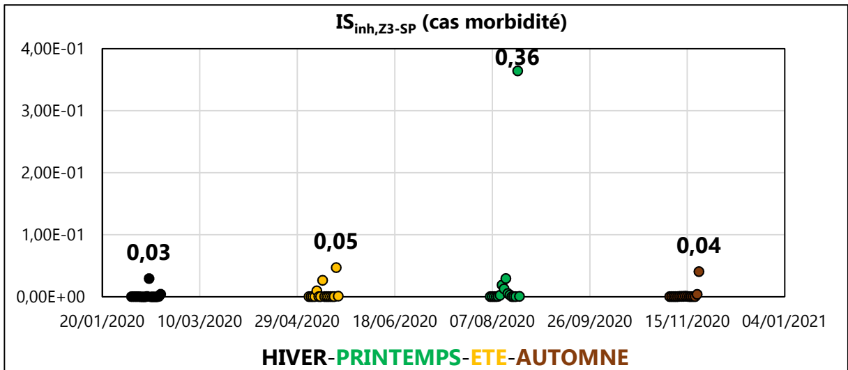
Figure III. 102 : Impact de toxicité humaine dans Z3-SP (cas de morbidité) hors PM 2,5
