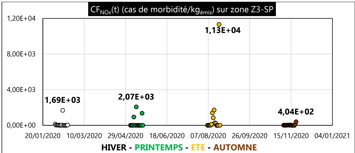
Figure III. 90 : CF NO x (t) (cas de morbidité/kg émis ) sur zone Z3-SP
