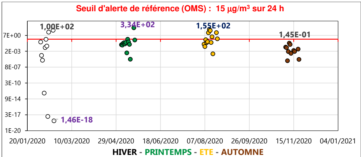
Figure III. 24 : Concentration potentielle moyenne/24h par saison de \text{PM}_{2,5} (Fe) ( \mu\text{g}/\text{m}^3 ) en zone Z2-FM en 2020
