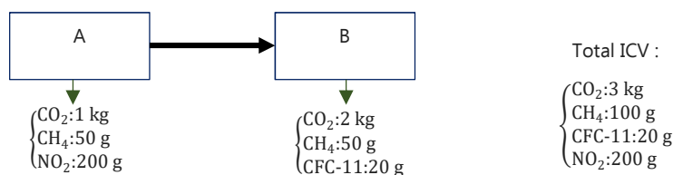
Figure I. 3 : Calcul d'un ICV pour un système fictif composé de deux étapes A et B. Source [Abrassart et al. 2011]
