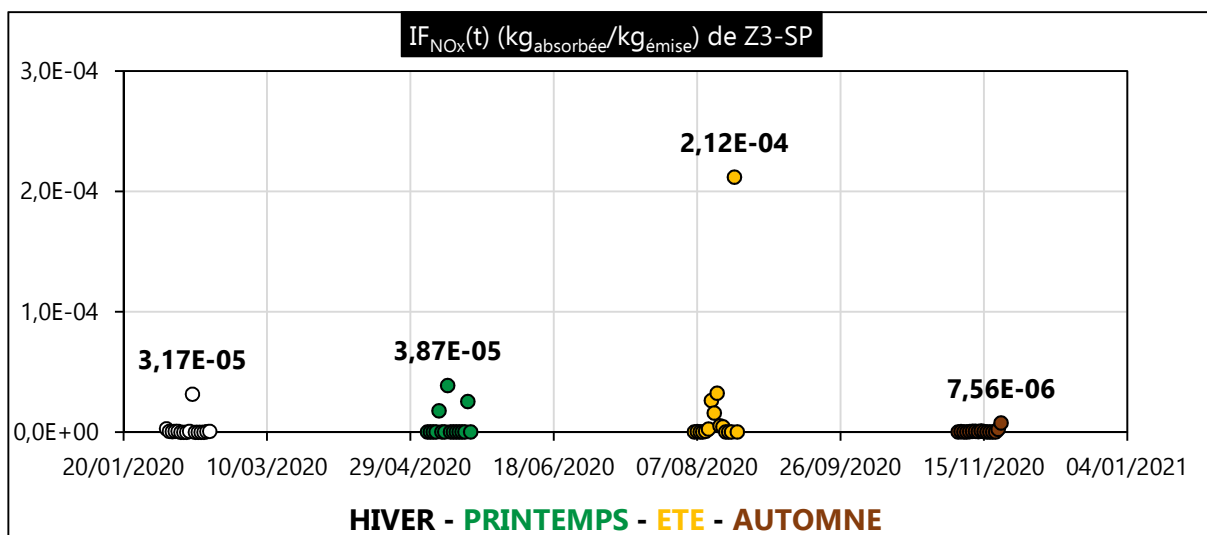
De ces Figure III. 71 : IF NOx (t) (kg absorbée /kg émise ) de Z3-SP en 2020
