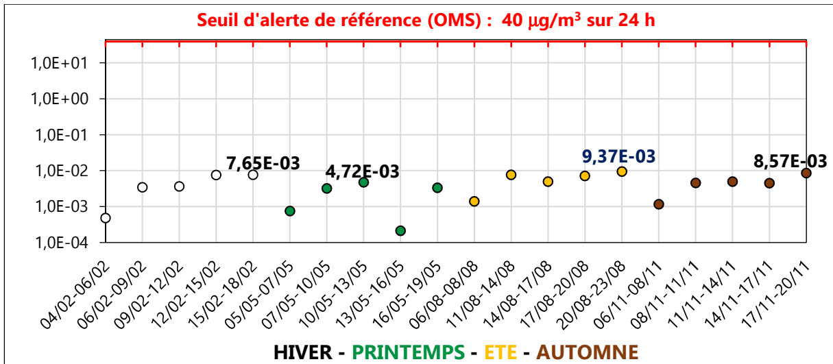
Figure III. 37 : Concentration potentielle moyenne/24h de SO 2 (µg/m 3 ) à Z1-SsS en 2020
