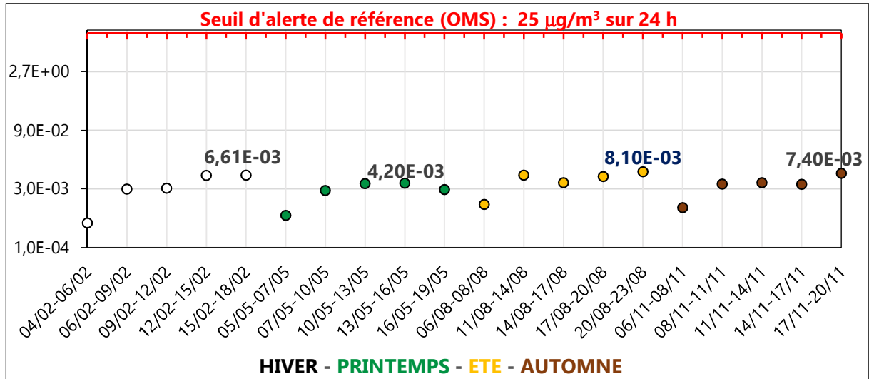
Figure III. 35 : Concentration potentielle moyenne/24h de NO x (µg/m 3 ) à Z1-SsS en 2020
