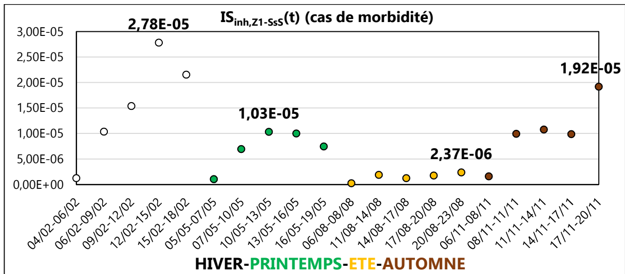
Figure III. 104 : Impact de toxicité humaine dans Z1-SsS (cas de morbidité) hors PM 2,5
