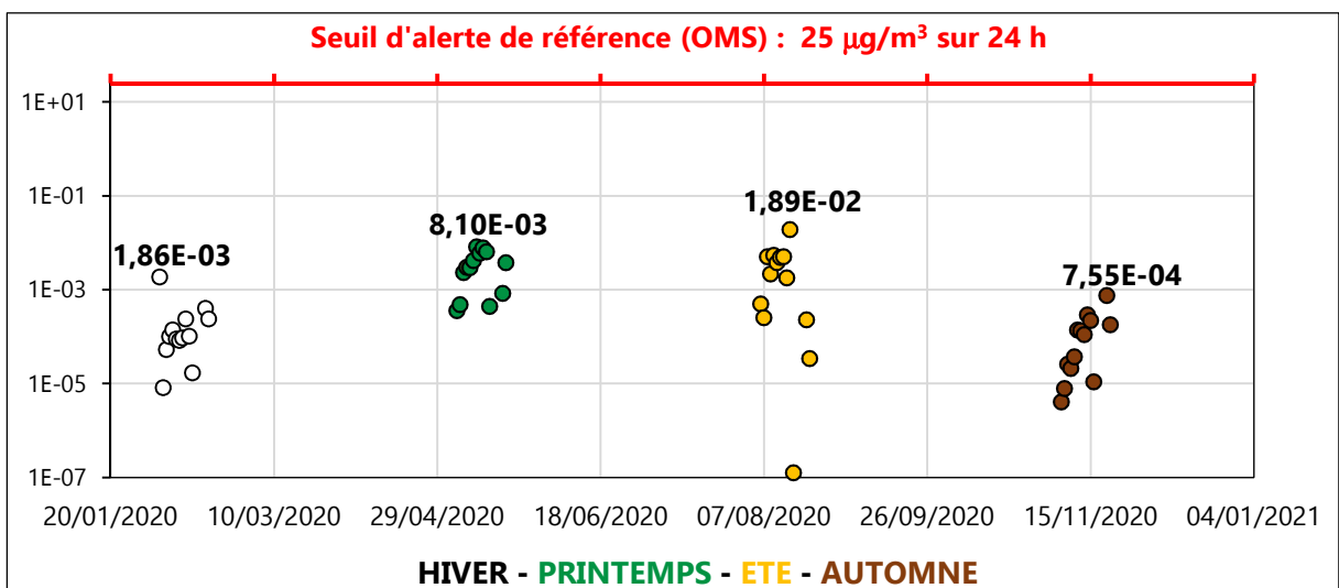
Figure III. 29 : Concentration potentielle moyenne/24h par saison de NO x (µg/m 3 ) en zone Z4-PS en 2020
