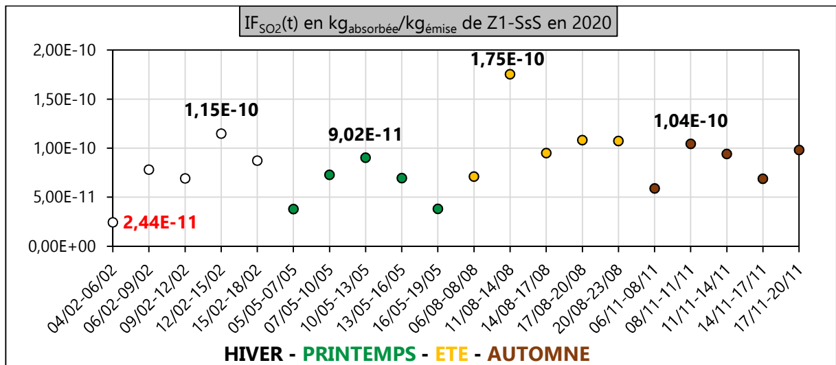
Figure III. 79 : IF SO2 (t) en kg absorbée /kg émise de Z1-SsS en 2020
