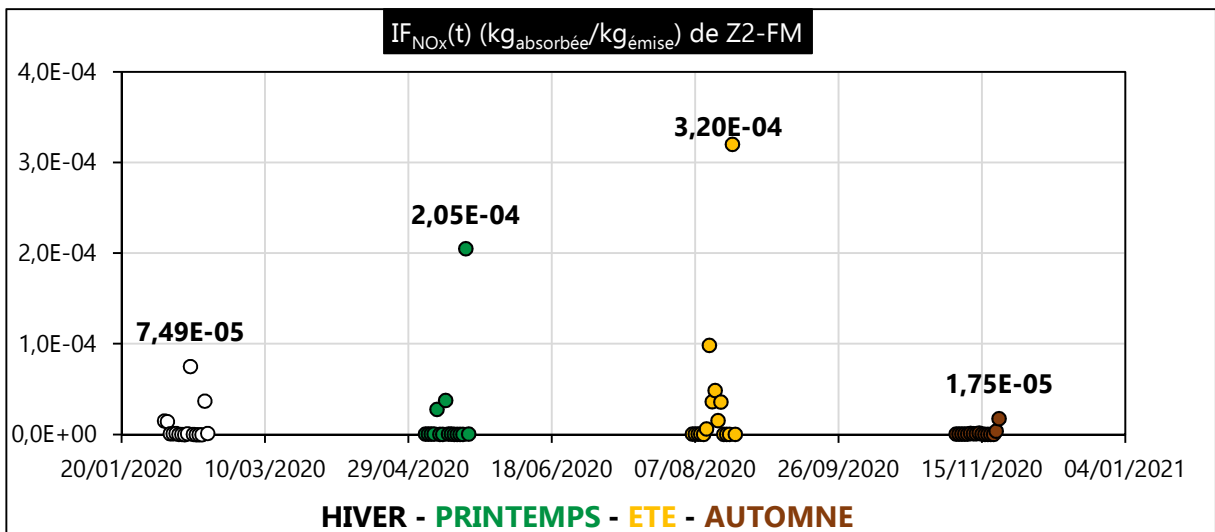
Figure III. 68 : IF NO x (t) (kg absorbée /kg émise ) de Z2-FM en 2020
