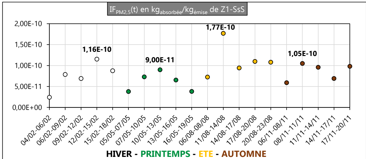
Figure III. 78 : IF PM2,5 (t) en kg absorbée /kg émise de Z1-SsS en 2020
