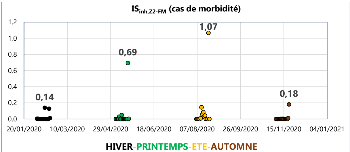
Figure III. 101 : Impact de toxicité humaine dans Z2-FM (cas de morbidité) hors PM 2,5
