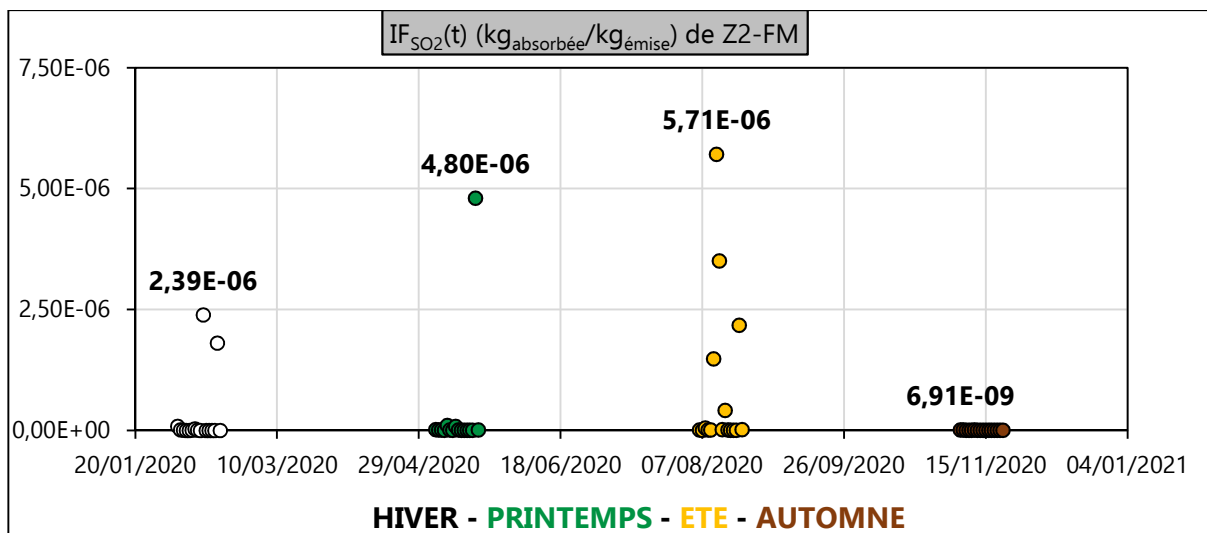
Figure III. 70 : IF SO2 (t) (kg absorbée /kg émise ) de Z2-FM en 2020
