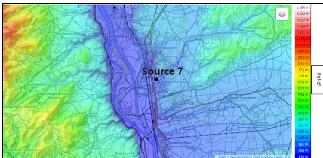
Figure III. 32 : Carte topographique de Salaise-sur-Sanne et des villes avoisinantes
