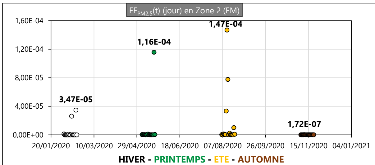
Figure III. 48 : FF PM2,5 (t) (jour) en zone Z2-FM en 2020
