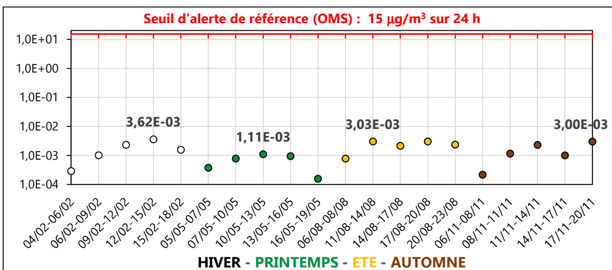
Figure III. 39 : Concentration potentielle moyenne/24h de PM 2,5 (µg/m 3 ) à Z2-LPR en 2020
