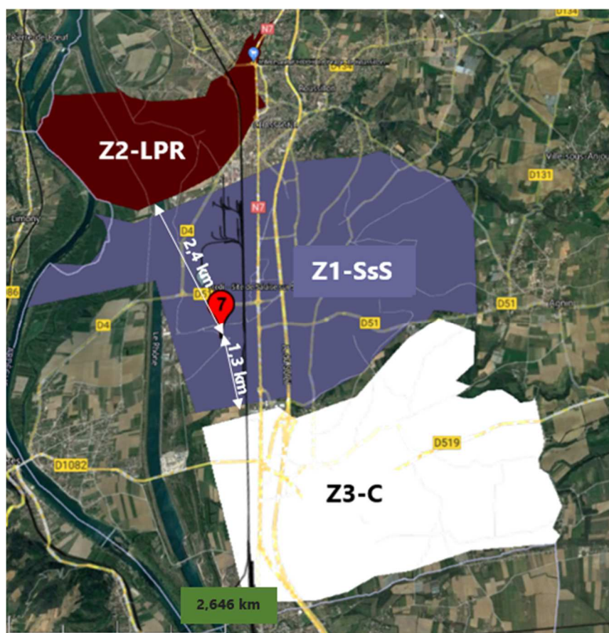
Figure III. 34 : Cartographie des 3 zones exposées à la source d'émission 7
