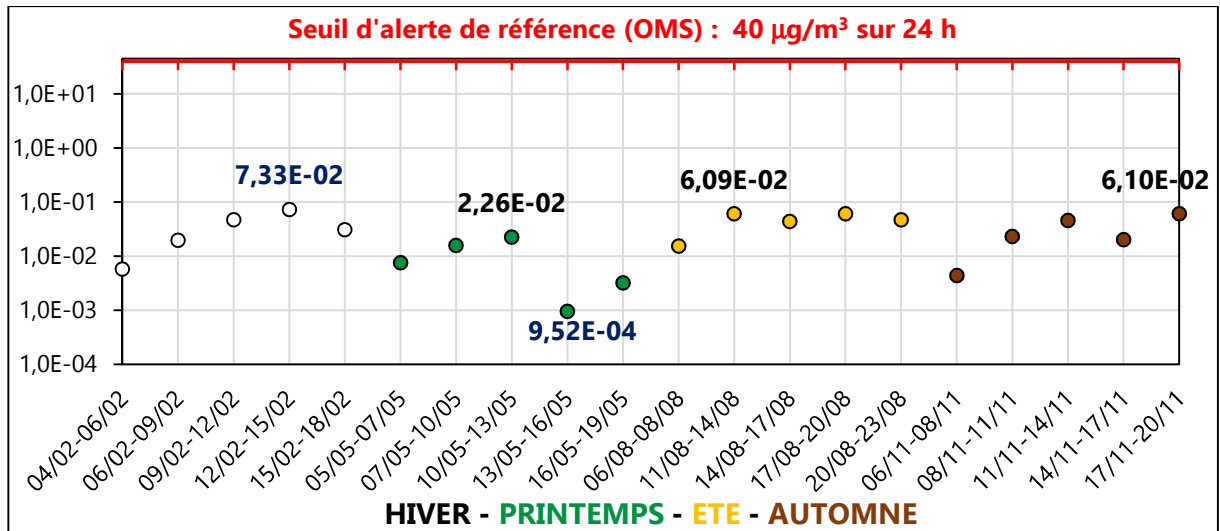
Figure III. 40 : Concentration potentielle moyenne/24h de SO 2 (µg/m 3 ) à Z2-LPR en 2020
