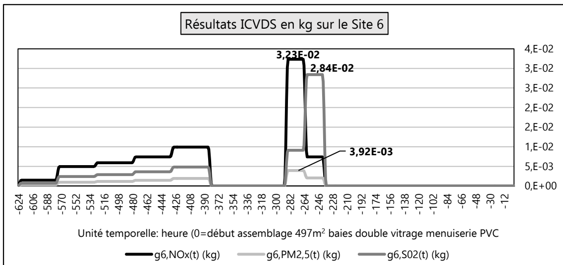
Figure III. 12 : Évolution temporelle g_{6,s}(t)
