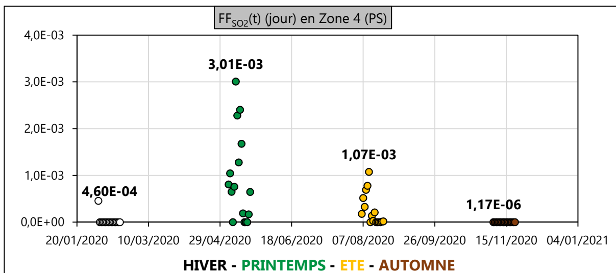
Figure III. 55 : FF_{SO_2}(t) (jour) en zone Z4-PS en 2020
