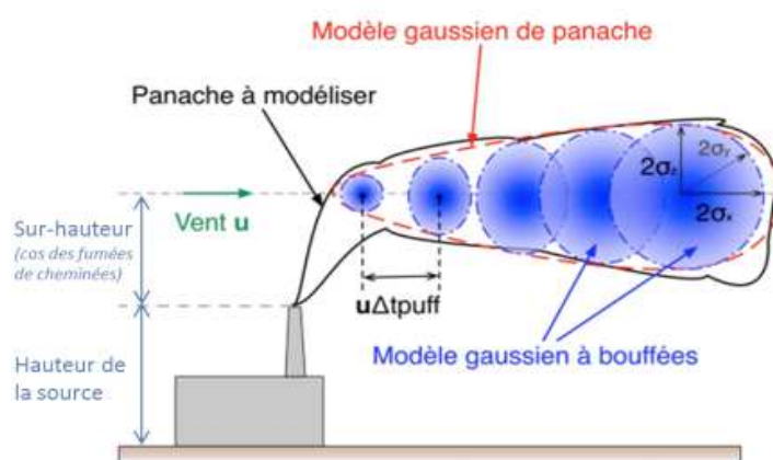
Figure I. 17 : Distinction schématique entre le modèle gaussien de panache et le modèle gaussien à bouffées [Foulet et al., 2017]
