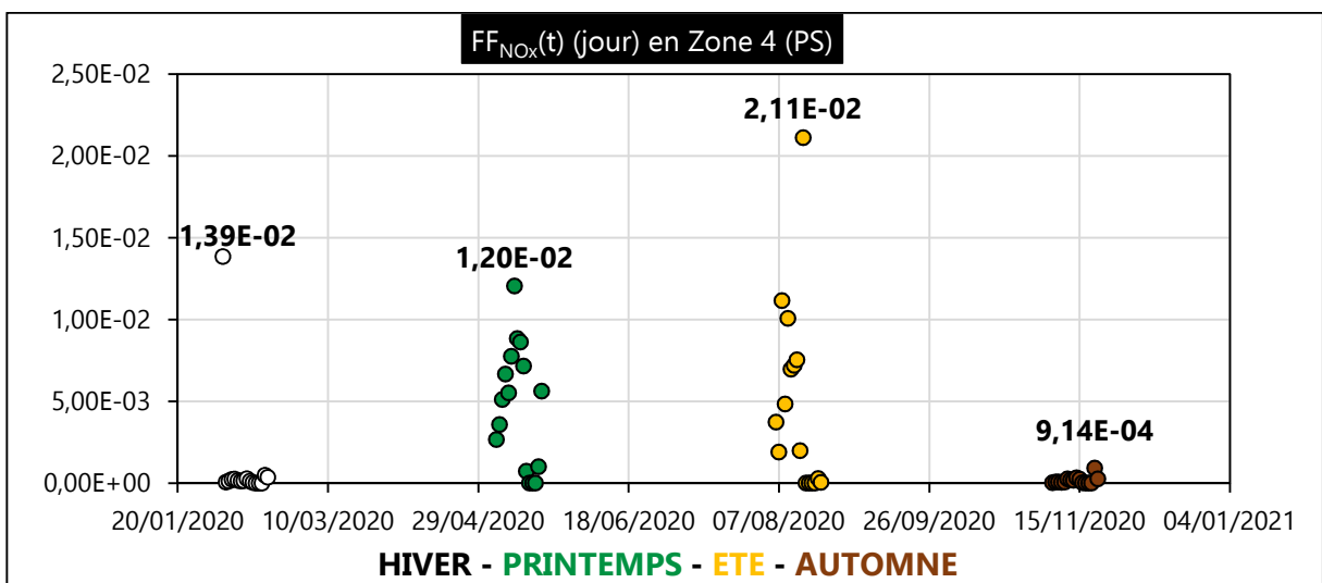
Figure III. 53 : FF NOx (t) (jour) en zone Z4-PS en 2020
