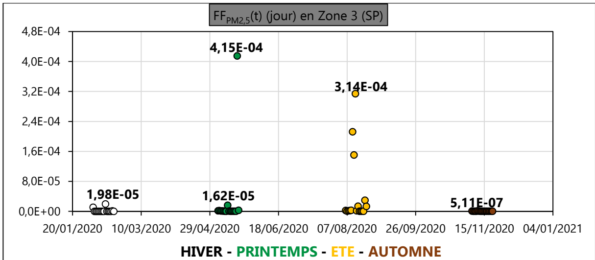
Figure III. 51 : FF PM2,5 (t) (jour) en zone Z3-SP en 2020
