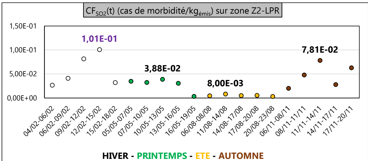
Figure III. 97 : CF SO2 (t) (cas de morbidité/kg émis ) sur zone Z2-LPR
