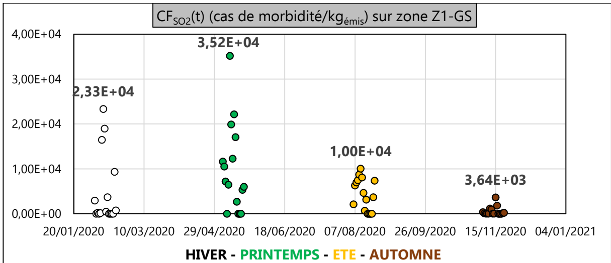
Figure III. 87 : CF SO 2 (t) (cas de morbidité/kg émis ) sur zone Z1-GS
