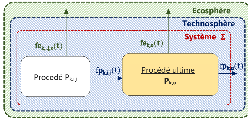
Figure II. 2 : Arbre de processus unitaire partiel d'un système lors d'une ACVDSd
