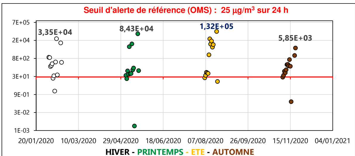
Figure III. 23 : Concentration potentielle moyenne/24h par saison de \text{NO}_x ( \mu\text{g}/\text{m}^3 ) en zone Z2-FM en 2020
