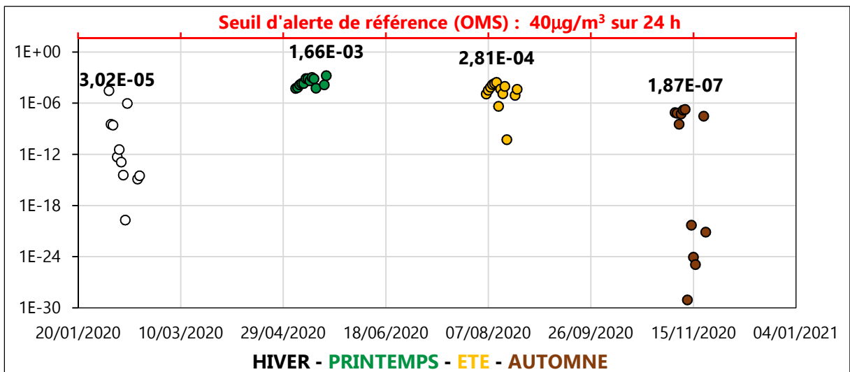
Figure III. 31 : Concentration potentielle moyenne/24h de SO 2 (µg/m 3 ) en zone Z4-PS en 2020
