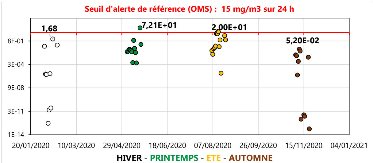
Figure III. 27 : Concentration potentielle moyenne/24h par saison de PM 2,5 (Fe) (µg/m 3 ) en zone Z3-SP en 2020
