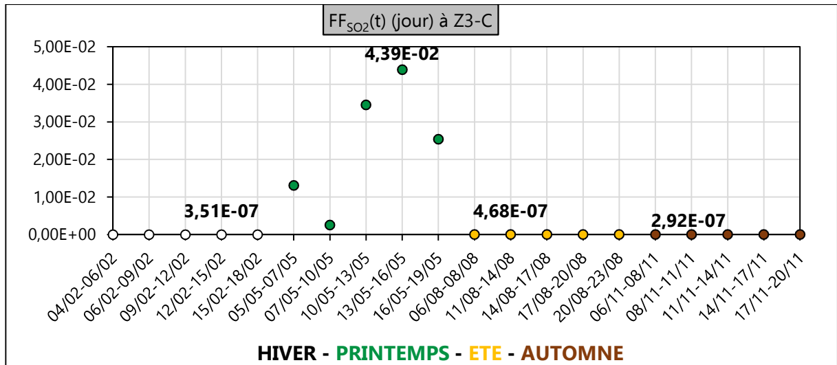
Figure III. 64 : FF SO2 (t) (jour) en zone Z3-C en 2020
