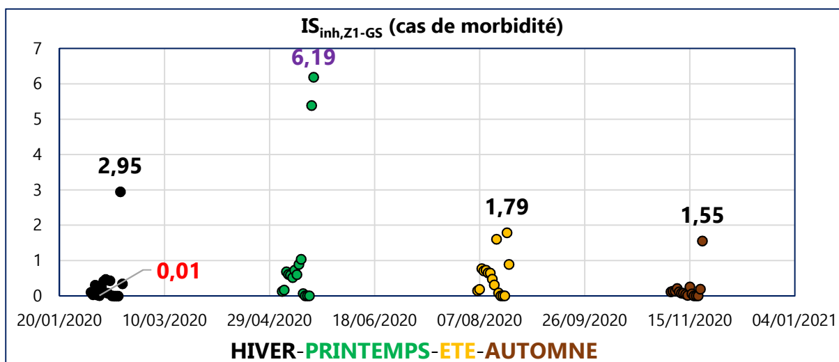
Figure III. 100 : Impact de toxicité humaine dans Z1-GS (cas de morbidité) hors PM 2,5
