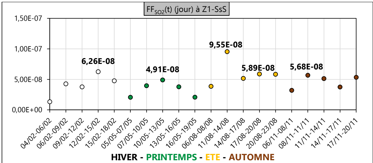
Figure III. 58 : FF SO2 (t) (jour) en zone Z1-SsS en 2020
