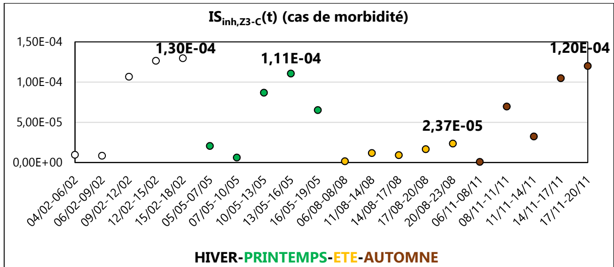
Figure III. 106 : Impact de toxicité humaine dans Z3-C (cas de morbidité) hors PM 2,5
