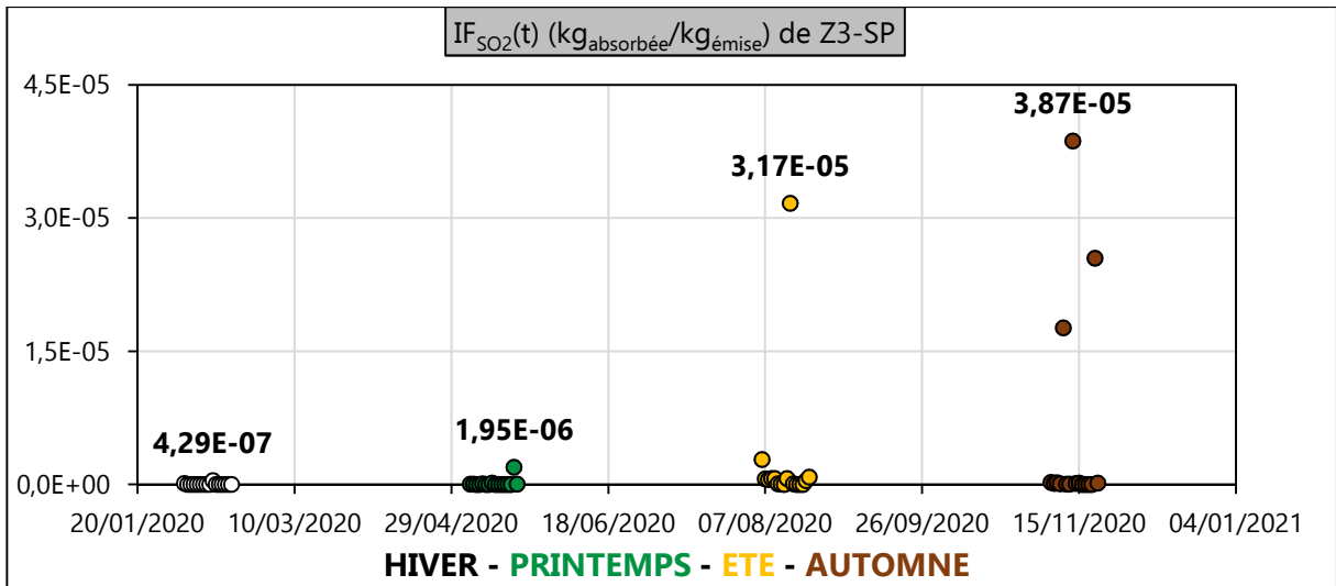
Figure III. 73 : IF SO 2 (t) (kg absorbée /kg émise ) de Z3-SP en 2020
