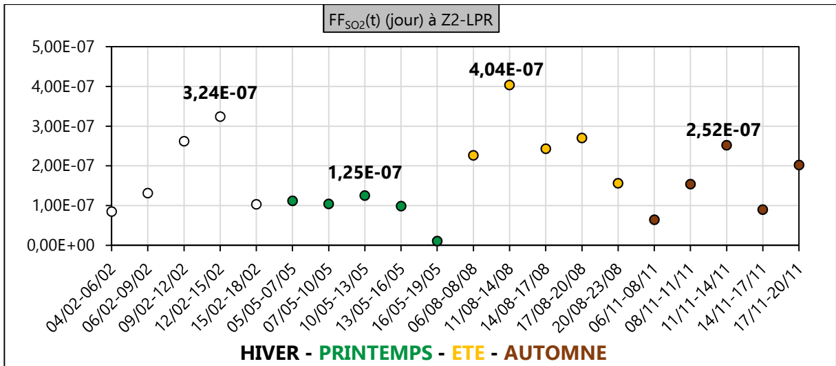
Figure III. 61 : FF SO2 (t) (jour) en zone Z2-LPR en 2020
