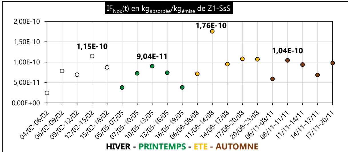
Figure III. 77 : IF Nox (t) en kg absorbée /kg émise de Z1-SsS en 2020
