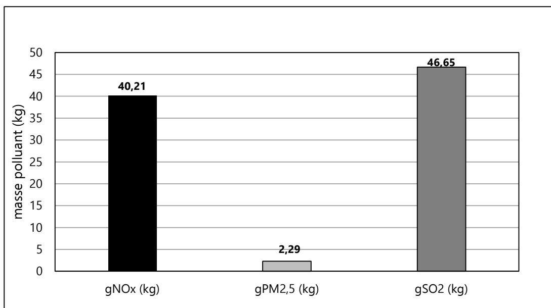
Figure III. 7 : ICV conventionnel du procédé P 7,1,6
