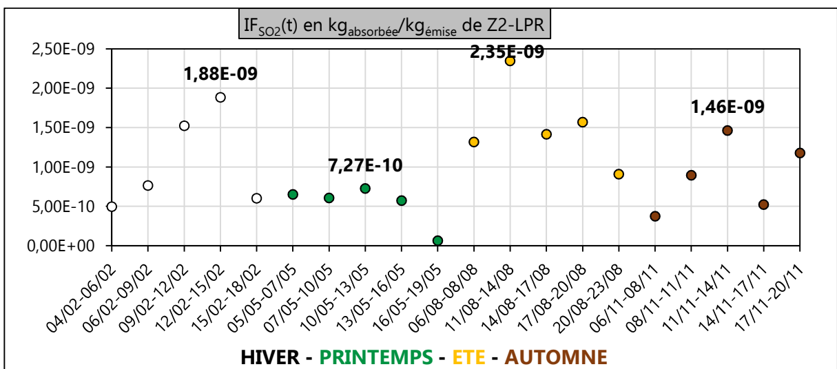
Figure III. 82 : IF SO2 (t) en kg absorbée /kg émise de Z2-LPR en 2020
