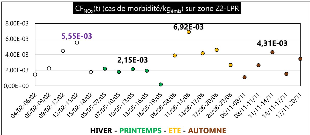
Figure III. 96 : CF NOx (t) (cas de morbidité/kg émis ) sur zone Z2-LPR
