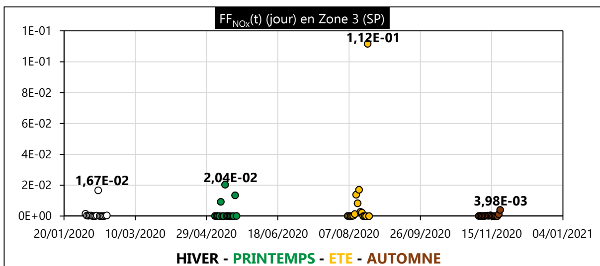
Figure III. 50 : FF NOx (t) (jour) en zone Z3-SP en 2020
