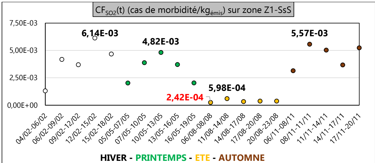
Figure III. 95 : CF SO2 (t) (cas de morbidité/kg émis ) sur zone Z1-SsS
