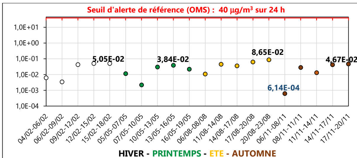
Figure III. 43 : Concentration potentielle moyenne/24h de SO 2 (µg/m 3 ) à Z3-C en 2020
