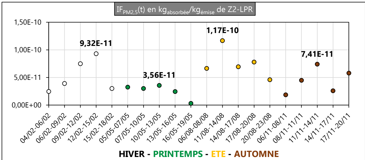
Figure III. 81 : IF PM2,5 (t) en kg absorbée /kg émise de Z2-LPR en 2020
