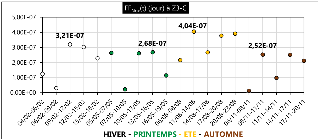
Figure III. 62 : FF NOx (t) (jour) en zone Z3-C en 2020
