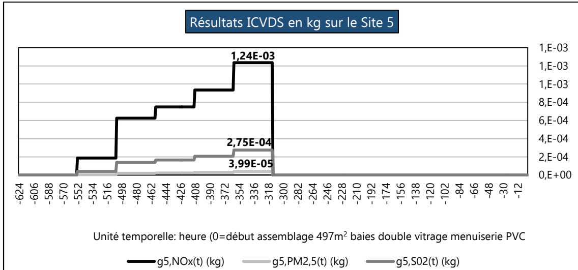
Figure III. 11 : Évolution temporelle g_{5,s}(t)
