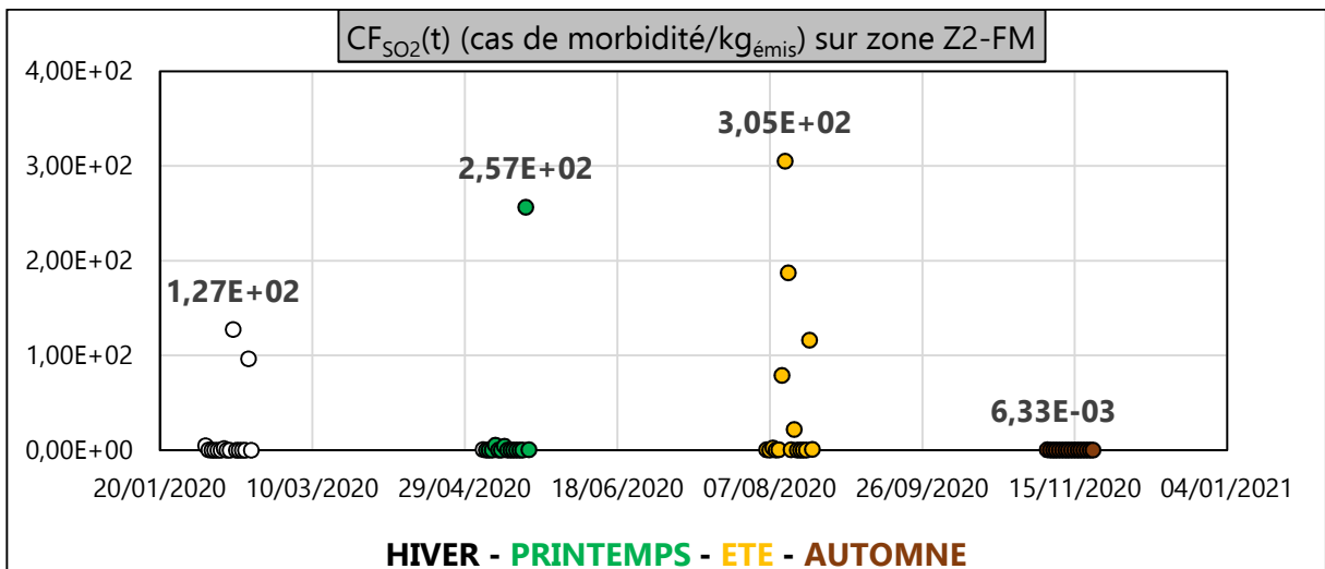
Figure III. 89 : CF SO 2 (t) (cas de morbidité/kg émis ) sur zone Z2-FM
