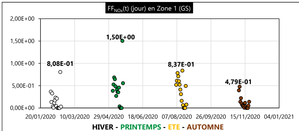
Figure III. 44 : FF_{NO_x}(t) (jour) en Z1-GS en 2020
