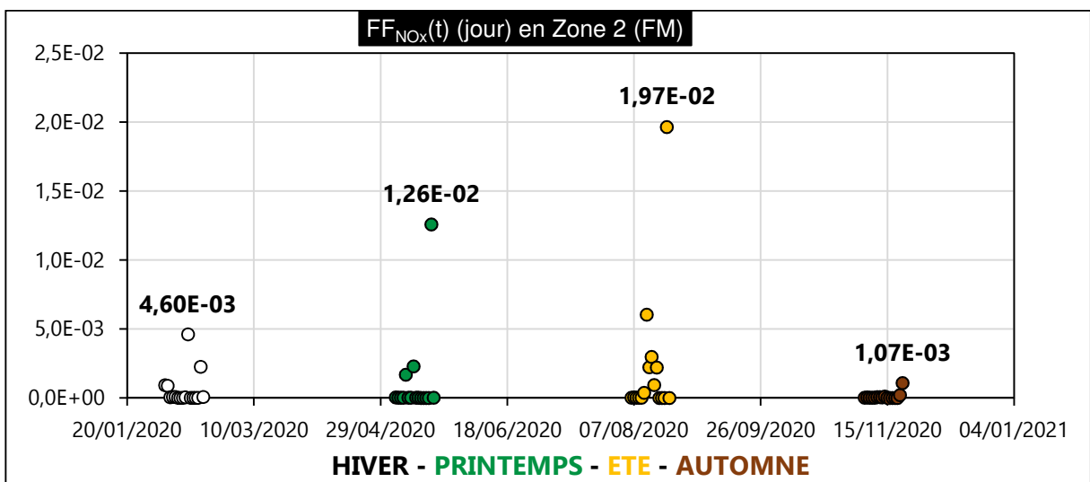
Figure III. 47 : FF NO x (t) (jour) en zone Z2-FM en 2020
