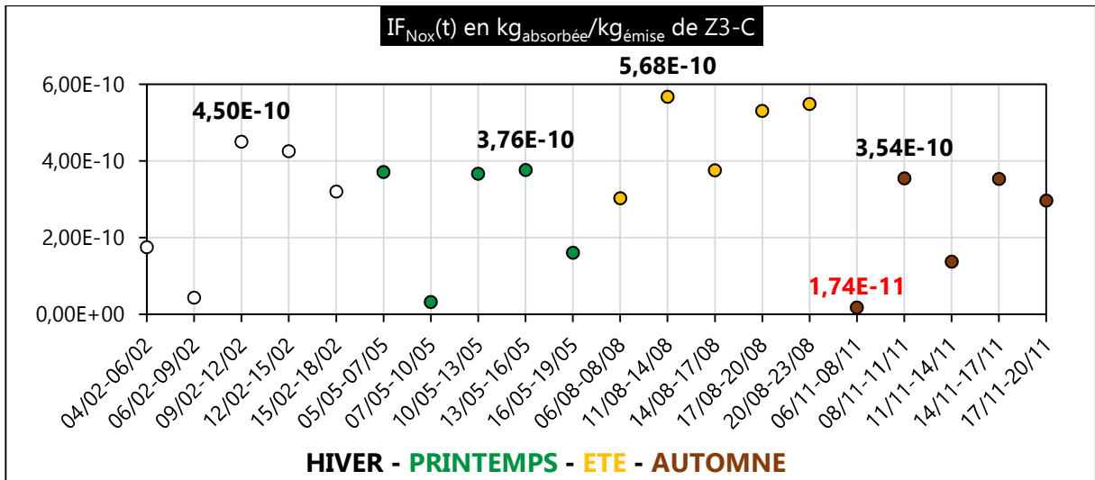
Figure III. 83 : IF NOx (t) en kg àbsorbée /kg émise de Z3-C en 2020
