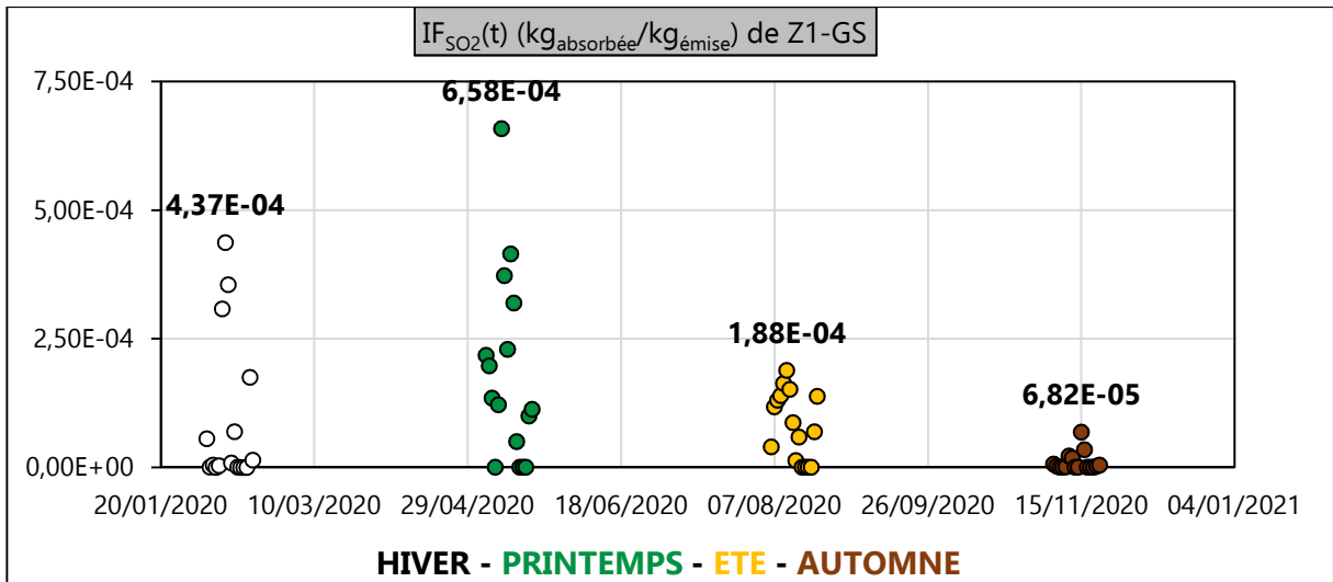
Figure III. 67 : IF SO 2 (t) (kg absorbée /kg émise ) de Z1-GS en 2020
