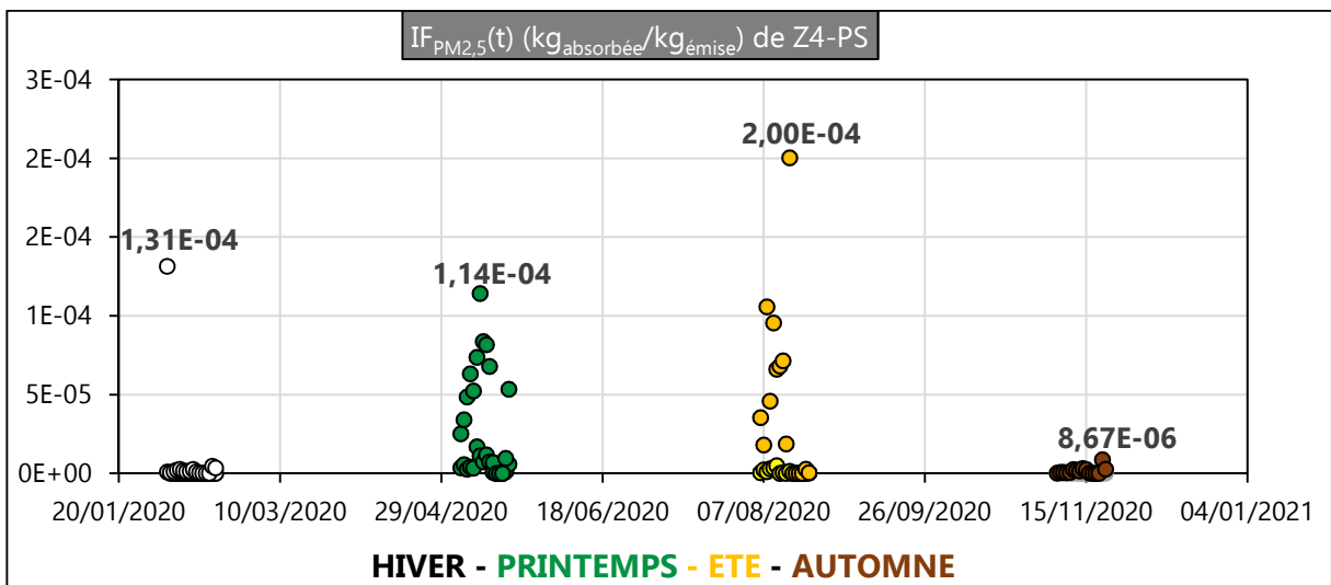
Figure III. 75 : IF PM 2,5 (t) (kg absorbée /kg émise ) de Z4-PS en 2020
