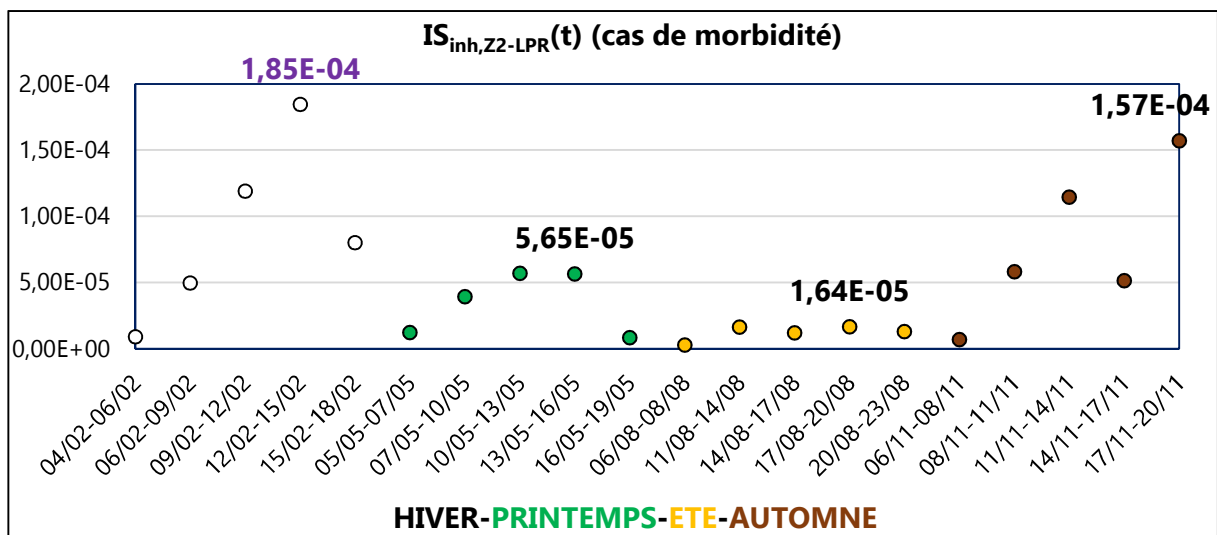
Figure III. 105 : Impact de toxicité humaine dans Z2-LPR (cas de morbidité) hors PM 2,5
