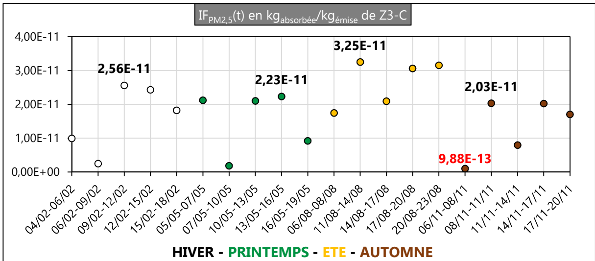
Figure III. 84 : IF PM2,5 (t) en kg àbsorbée /kg émise de Z3-C en 2020
