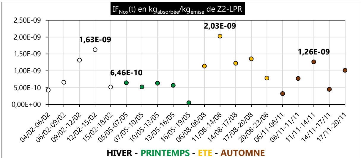
Figure III. 80 : IF Nox (t) en kg absorbée /kg émise de Z2-LPR en 2020
