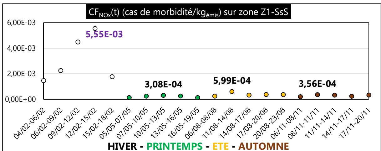
Figure III. 94 : CF NO x (t) (cas de morbidité/kg émis ) sur zone Z1-SsS
