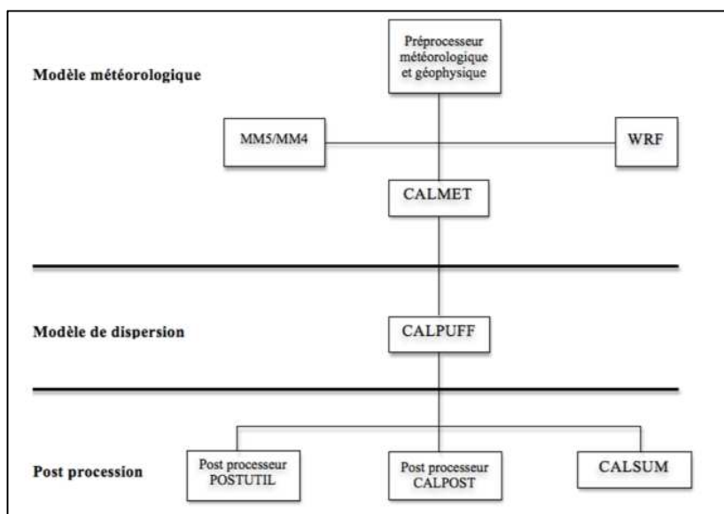
Figure I. 18 : Schématisation de CALPUFF
