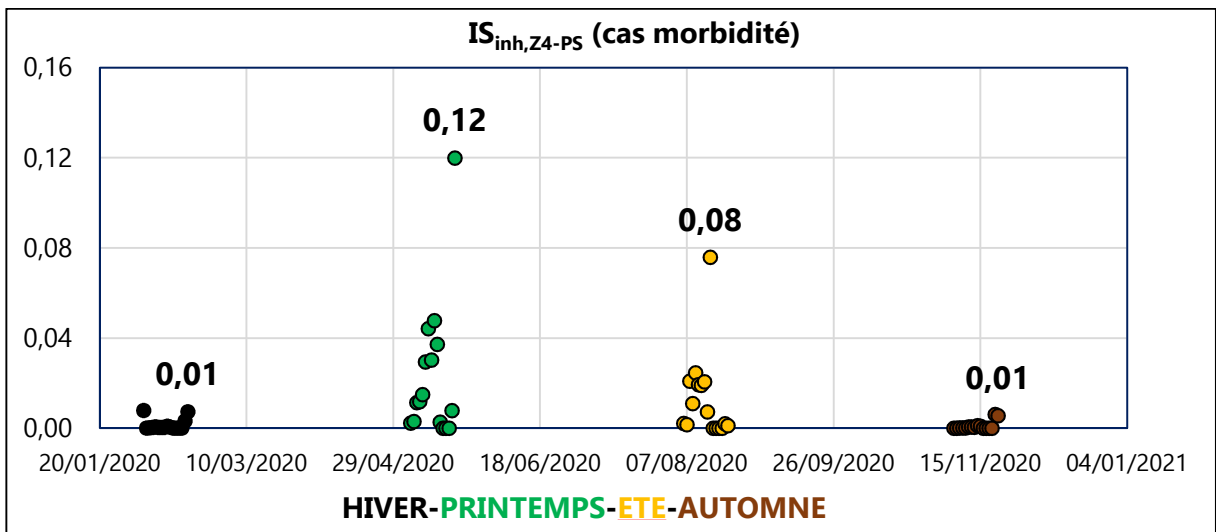
Figure III. 103 : Impact de toxicité humaine dans Z4-PS (cas de morbidité) hors PM 2,5
