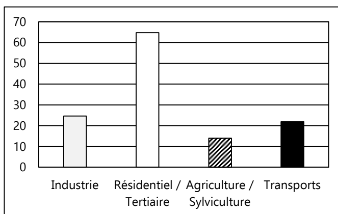
Figure I. 14 : Émission de PM 2,5 en France (en milliers de tonnes) en 2019, [Bilan de la qualité de l'air en France en 2019]
