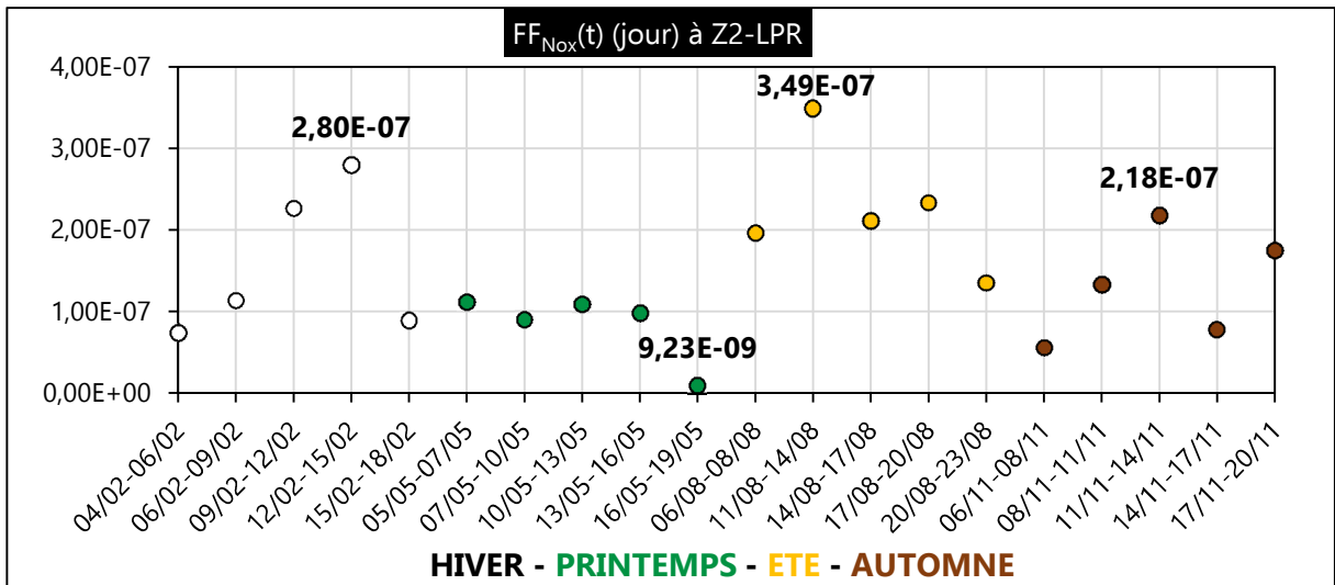
Figure III. 59 : FF NOx (t) (jour) en zone Z2-LPR en 2020
