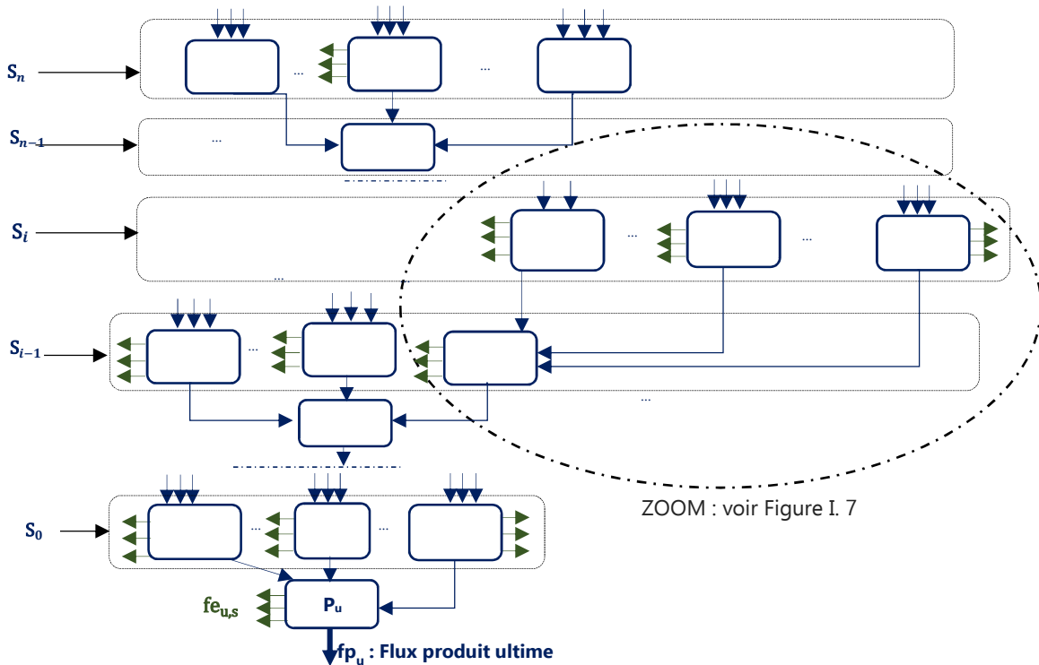
Figure I. 6 : Chaîne des procédés inspirée de l'arbre des processus [Joliet et al., 2005]
