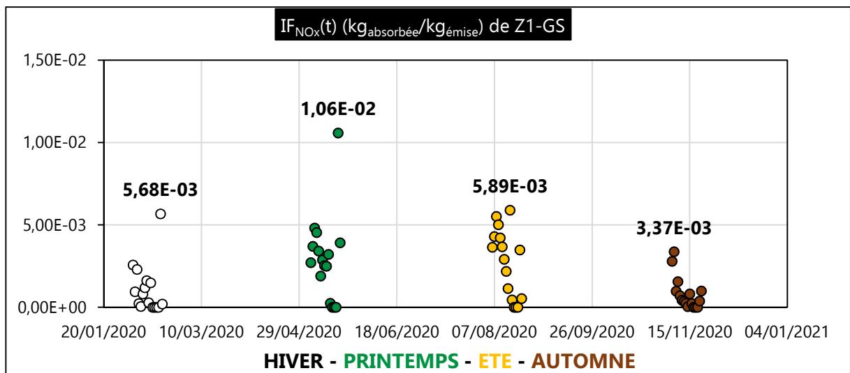
Figure III. 65 : IF_{NO_x}(t) ( kg_{\text{absorbée}}/kg_{\text{émise}} ) de Z1-GS en 2020
