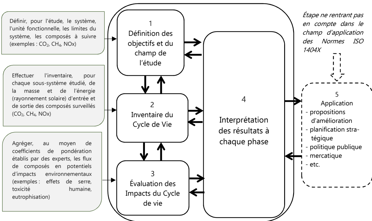
Figure I. 1: Méthodologie de l'ACV, inspirée de [ILCD Handbook, 2010]
