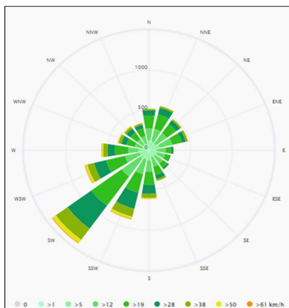
Figure III. 18 : Direction moyenne année 2020 Rose des vents ville de Grande-Synthe (Source : https://www.meteoblue.com/fr/meteo/historyclimate/climatemodelled/grande-synthe_france_3015160 )
