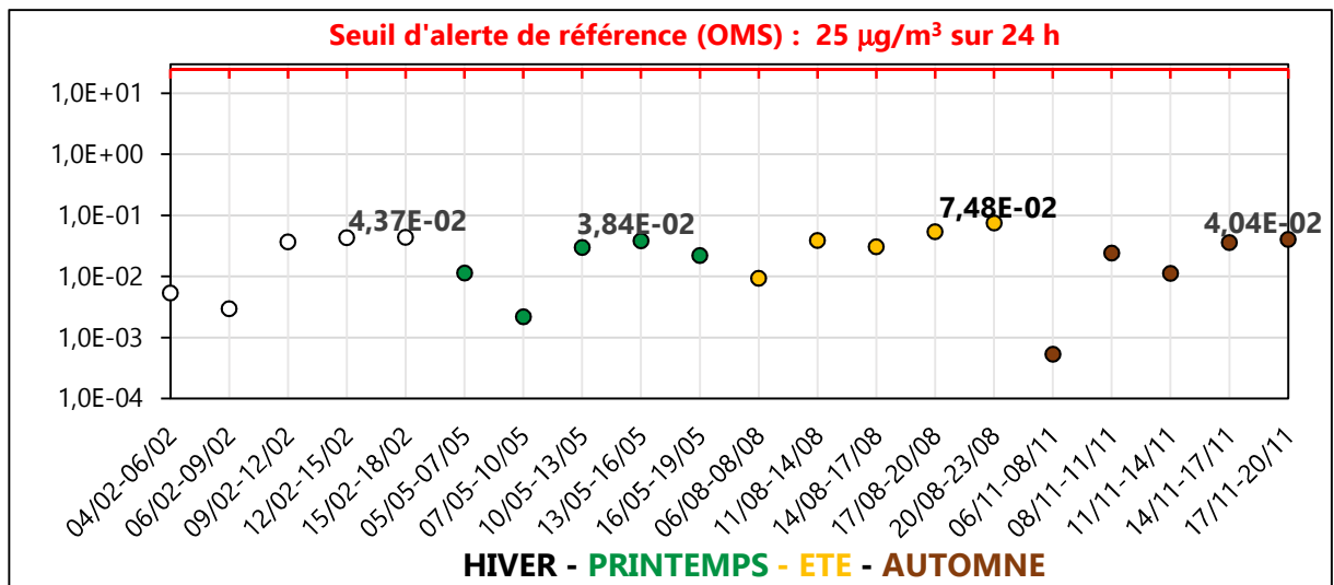
Figure III. 41 : Concentration potentielle moyenne/24h de NO x (µg/m 3 ) à Z3-C en 2020
