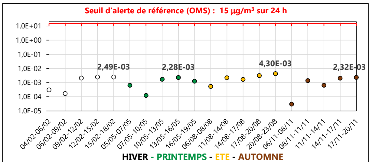
Figure III. 42 : Concentration potentielle moyenne/24h de PM 2,5 (µg/m 3 ) à Z3-C en 2020
