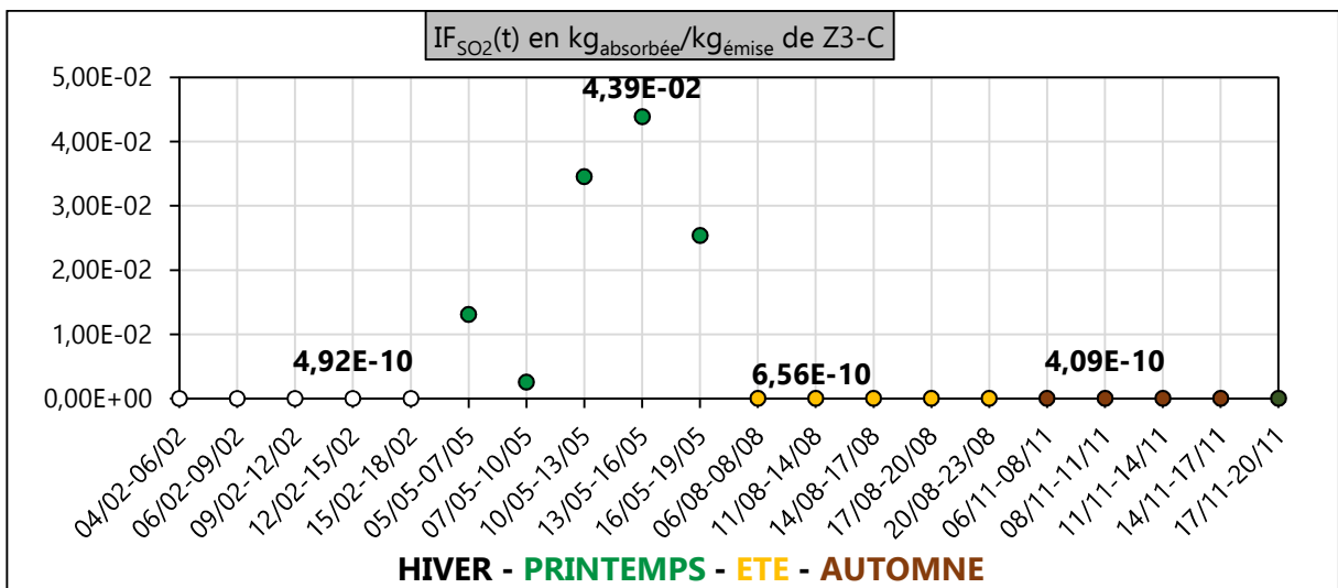
Figure III. 85 : IF SO2 (t) en kg àbsorbée /kg émise de Z3-C en 2020
