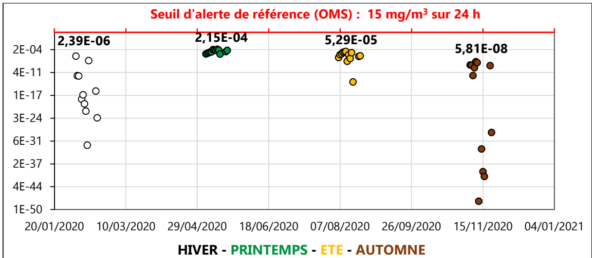
Figure III. 30 : Concentration potentielle moyenne/24h de PM 2,5 (Fe) (µg/m 3 ) en zone Z4-PS en 2020
