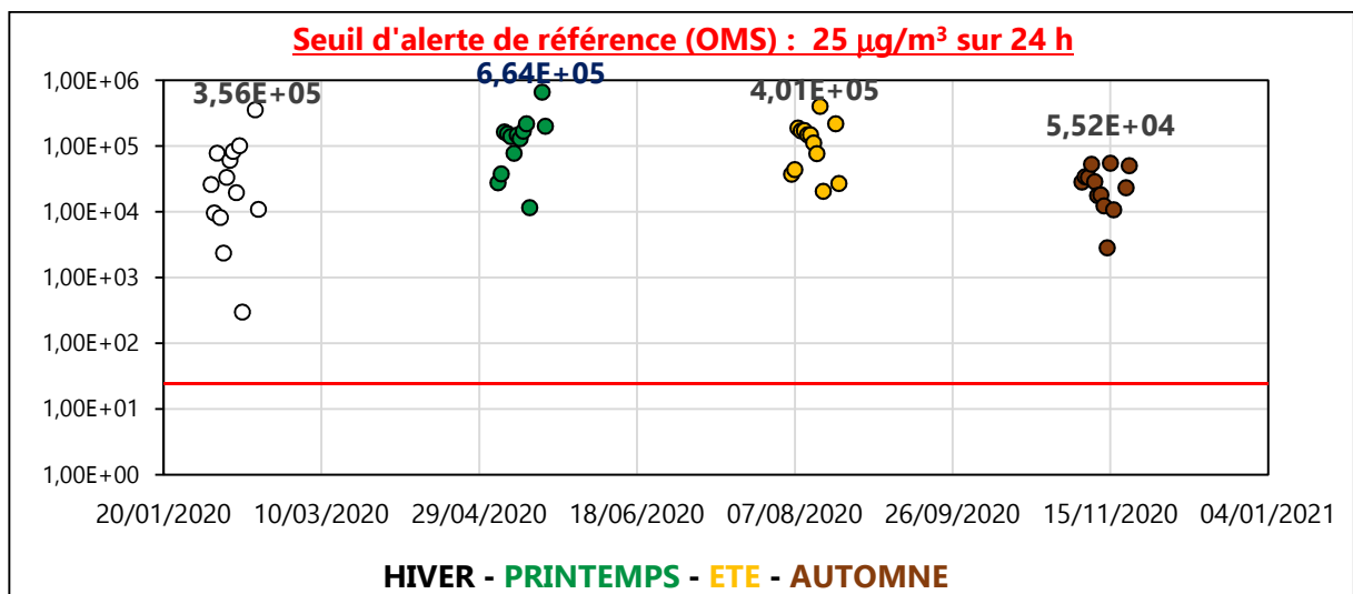
Figure III. 20 : Concentration potentielle moyenne/24h par saison de \text{NO}_x ( \mu\text{g}/\text{m}^3 ) en zone Z1-GS en 2020
