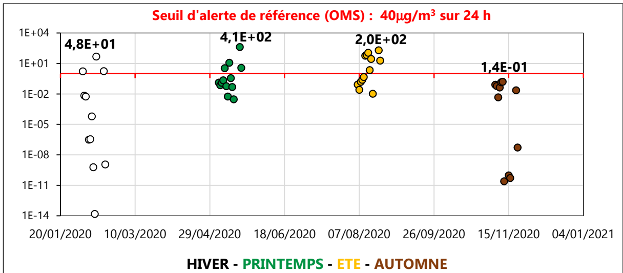
Figure III. 28 : Concentration potentielle moyenne/24h par saison de SO 2 (µg/m 3 ) en zone Z3-SP en 2020
