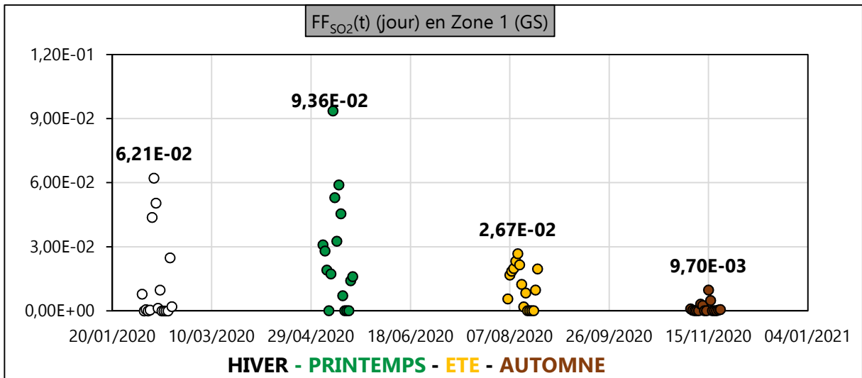
Figure III. 46 : FF SO 2 (t) (jour) en zone Z1-GS en 2020
