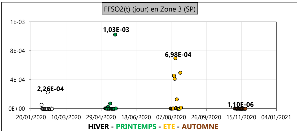
Figure III. 52 : FF SO2 (t) (jour) en zone Z3-SP en 2020
