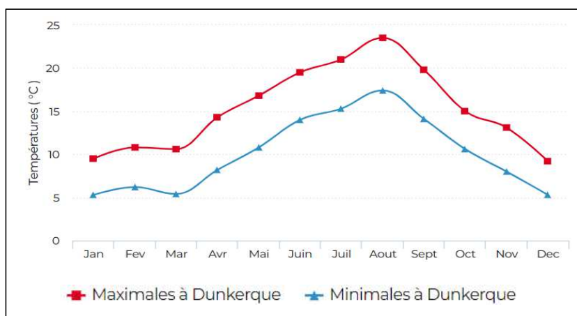
Figure III. 17 : températures relatives à Dunkerque en 2020 (Source : Linternaute.com d'après Météo France)
