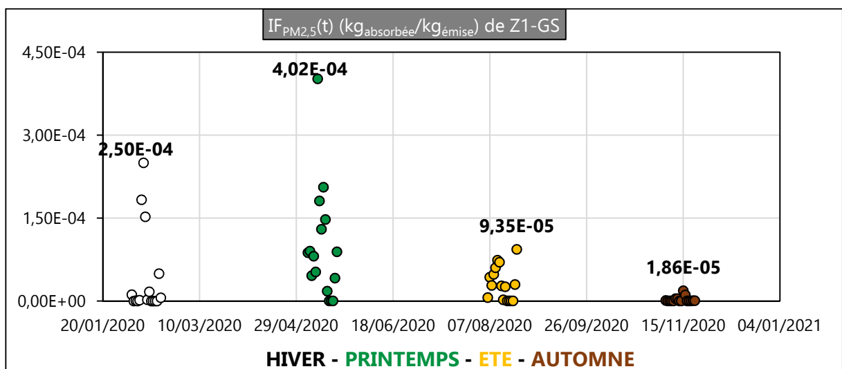
Figure III. 66 : IF_{PM_{2,5}}(t) ( kg_{\text{absorbée}}/kg_{\text{émise}} ) de Z1-GS en 2020
