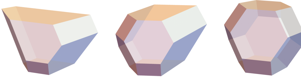
FIGURE 1.2 : Quelques permutoèdres généralisés de dimension trois, faisant partie de la sous-famille des opératoèdres.
