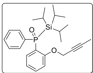
(2-(but-2-yn-1-yloxy)phenyl)(phenyl)(triisopropylsilyl)phosphine oxide
