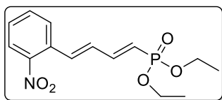
diethyl ((1E,3E)-4-(2-nitrophenyl)buta-1,3-dien-1-yl)phosphonate
