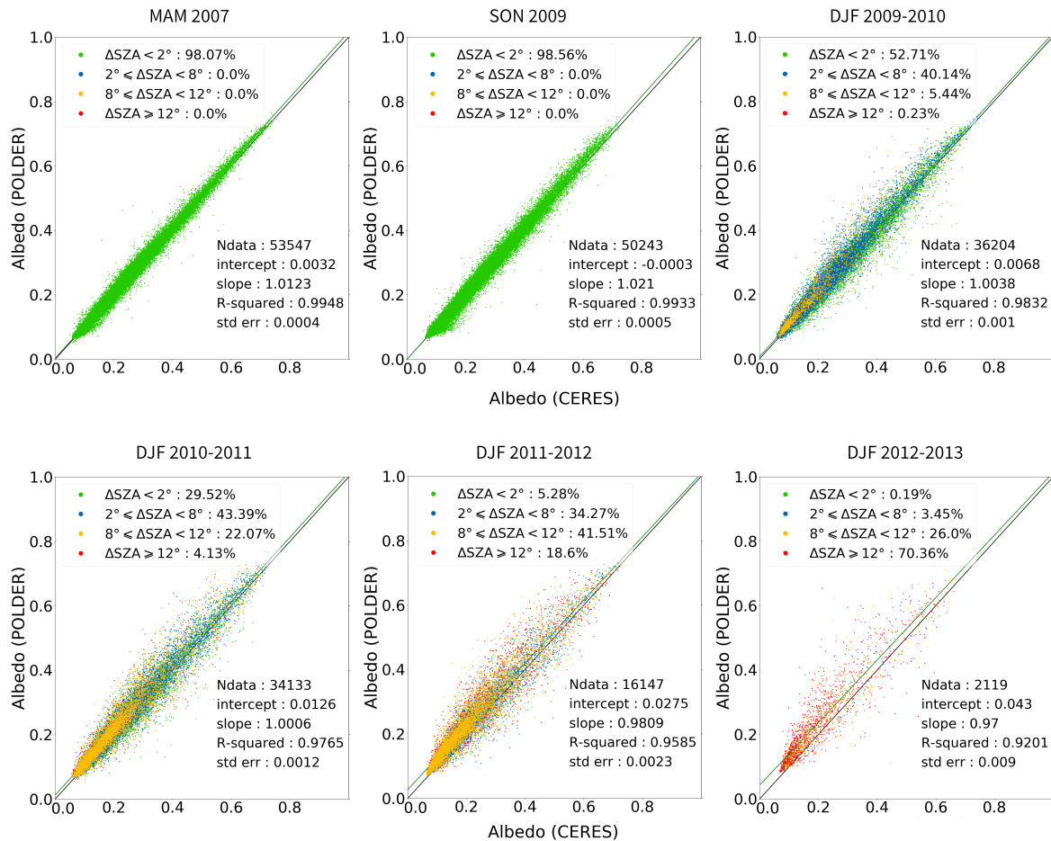
FIGURE 3.17 : Albédos instantanés POLDER RB2 représentés en fonction des albédos instantanés CERES SSF1deg-hour Aqua. Cas général, tous les albédos colocalisés sont choisis sans distinction terre/océan.
