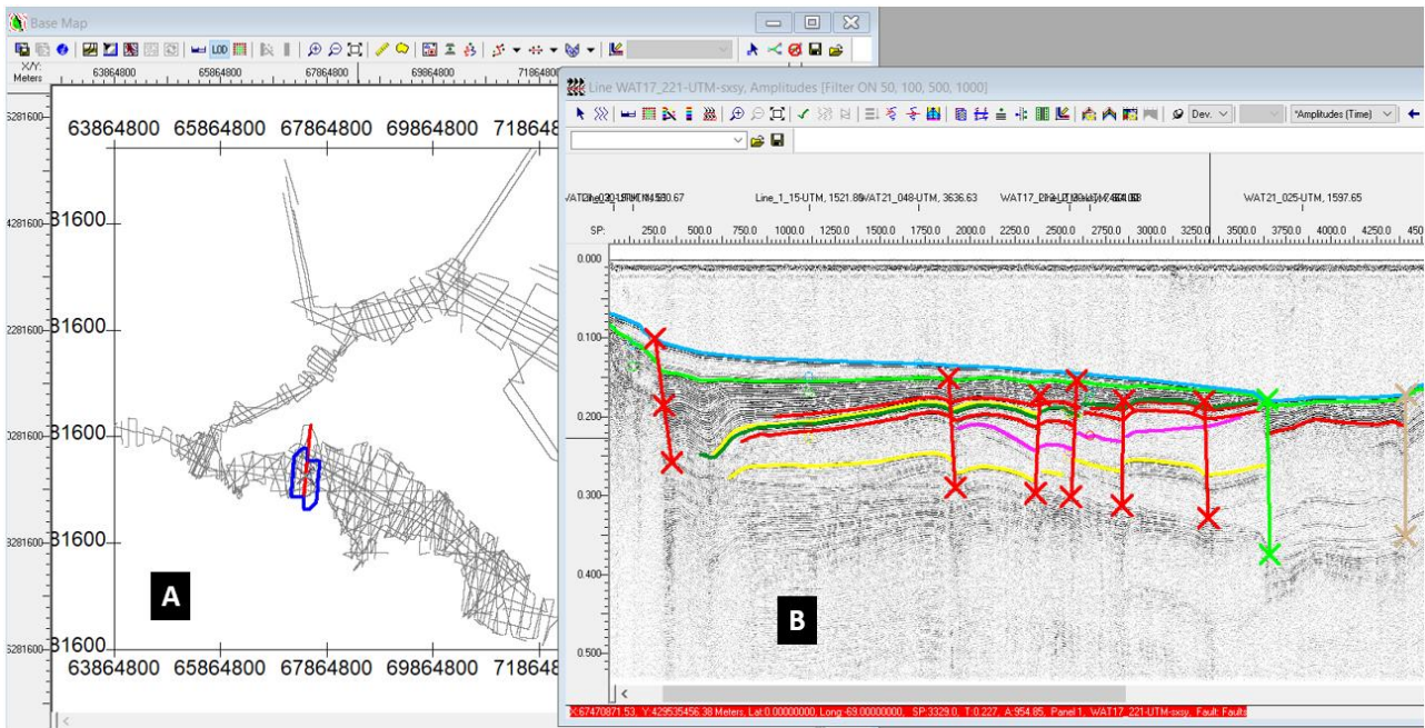
Figure 2.12 : Capture d'écran du logiciel d'interprétation sismique IHS Kingdom Suite. A) Plan de position des profils sismiques des campagnes de D. Sakellariou et WATER ; B) Profil sismique en cours d'interprétation.
