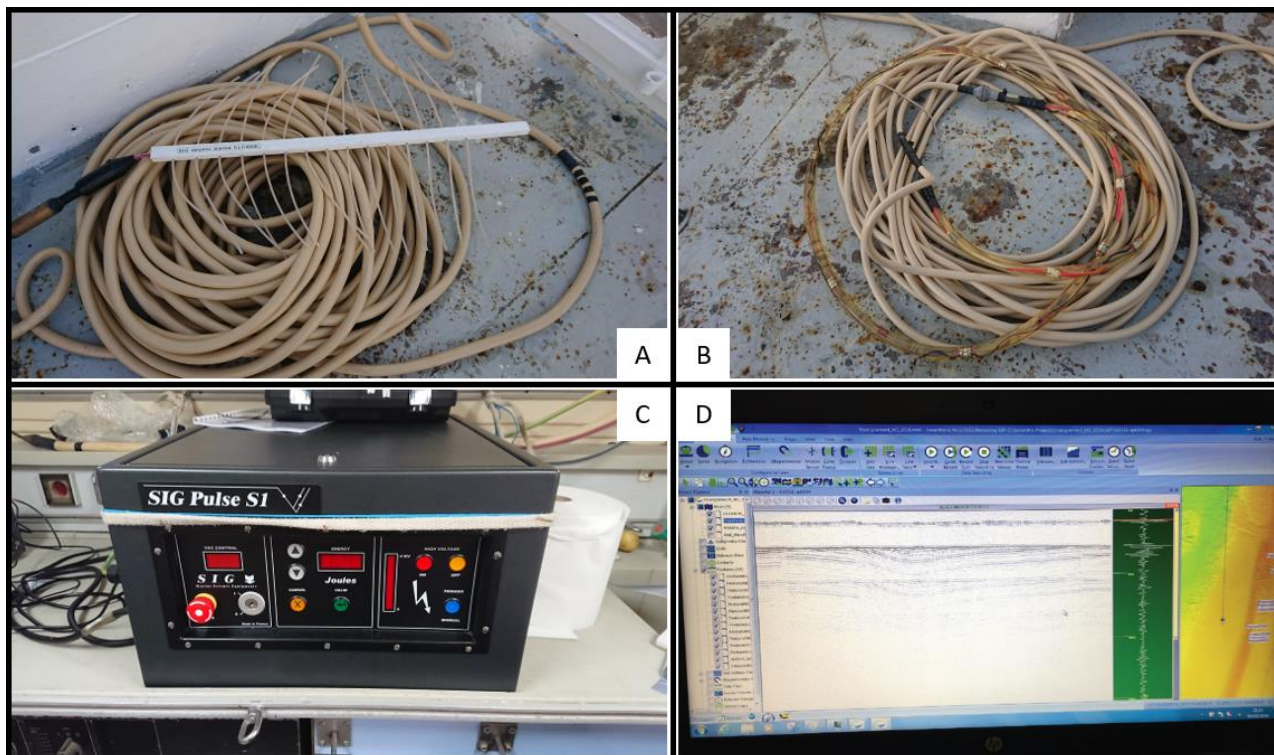
Figure 2.6 : Dispositif d'acquisition de type Sparker. A : le peigne, B : la flûte monotrace, C : la génératrice SIG, D : acquisition en cours sur le logiciel SonarWiz, photographie de Jollivet-Castelot (2018).
