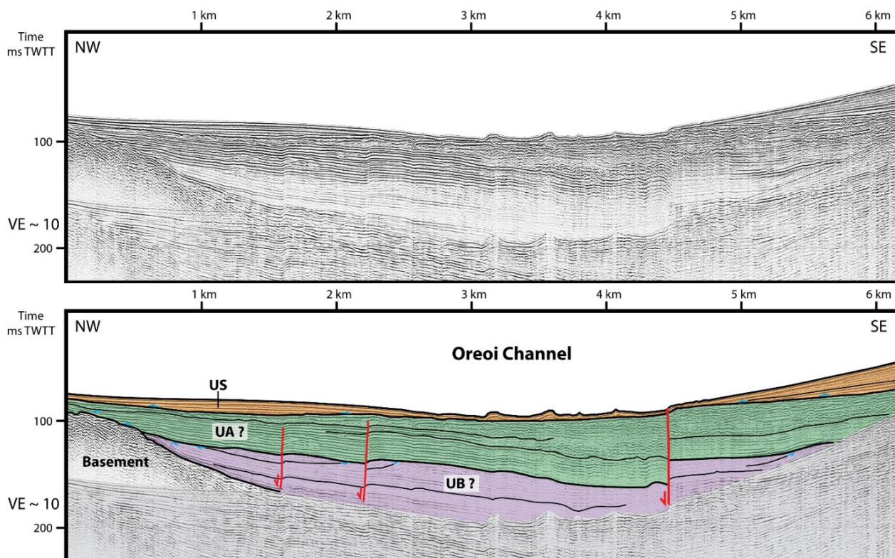
Figure 5.15 : Profil sismique Sparker WAT17_085 localisé sur la Figure 5.14. Ce profil perpendiculaire à l'axe du Chenal d'Oreoi met en évidence les différences de faciès sismique entre les deux unités sous-jacentes de l'Upper Sequence qui peuvent être corrélées aux unités A et B identifiées dans le Golfe Nord Eubée.
