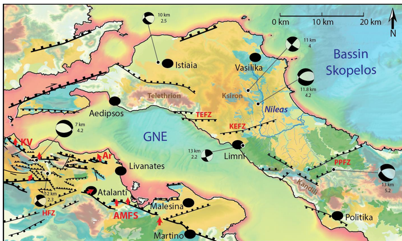
Figure 1.36 : Carte tectonique du sud du Golfe Nord Eubée (GNE) et du Nord de l'Eubée d'après les études suivantes : Palyvos et al. , 2006 ; Kranis, 2007 ; Kiliias et al. , 2008 ; Savvaïdis et al. , 2012. Quelques mécanismes au foyer ont été ajoutés afin d'illustrer l'activité sismique de cette zone (ISC / CMT, Storchak et al. , 2013 ; 2015 ; Di Giacomo et al. , 2018 / Dziejowski et al. , 1981 ; Ekström et al. , 2012). Les grands ensembles lithologiques à terre ont également été reportés (Vert : ophiolites, Bleu : Jurassique, Orange : Néogène et Vert pâle : Quaternaire) d'après les cartes géologiques au 1:50 000. Les flèches représentent le sens de glissement du bloc supérieur des failles normales.
