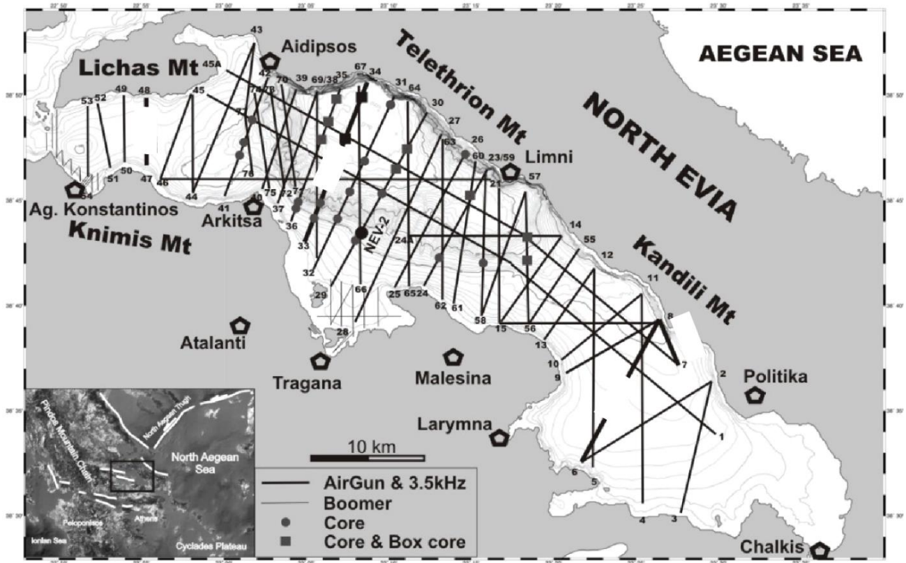
Figure 2.4 : Carte de localisation des profils sismiques Air-gun et Boomer et des carottes réalisées pendant la même campagne (Sakellariou et al. , 2007).
