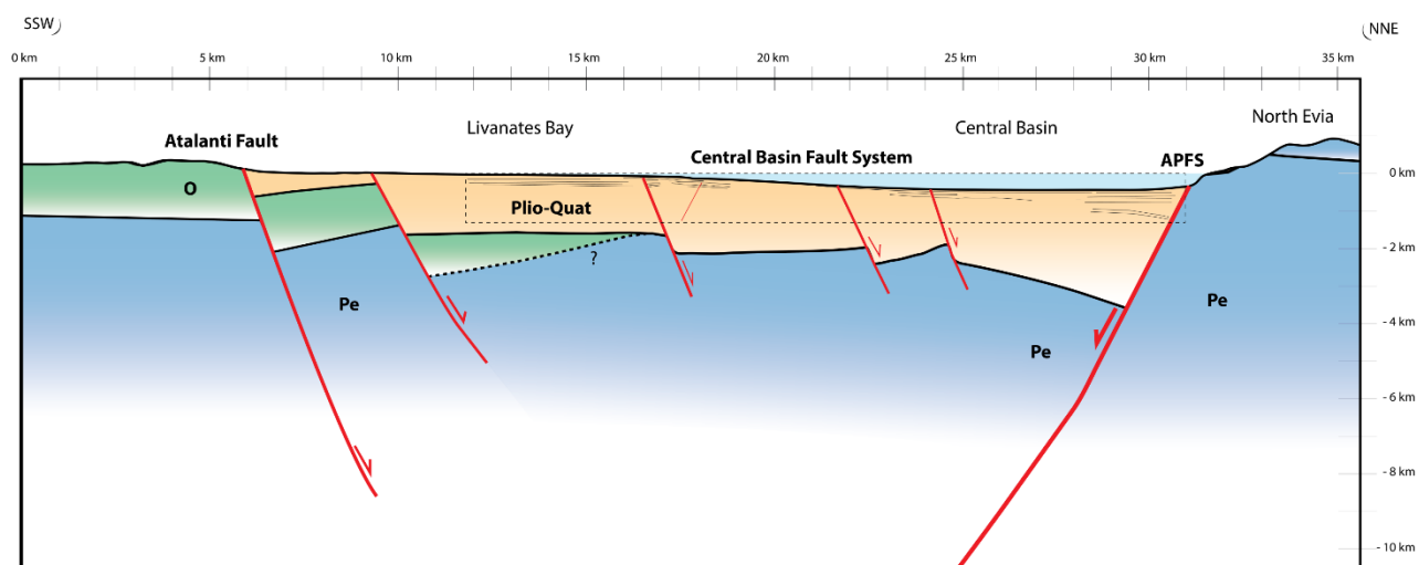
Figure 4.21 : Coupe schématique n°3 orientée SSW-NNE à travers le Bassin Central du Golfe Nord Eubée, localisée sur la Figure 4.1. Le rectangle en tirets matérialise la position d'un des profils sismiques Air-gun. APFS : Aedipsos Politika Fault System ; O : Ophiolites ; Pe : séries pélagoniennes.
