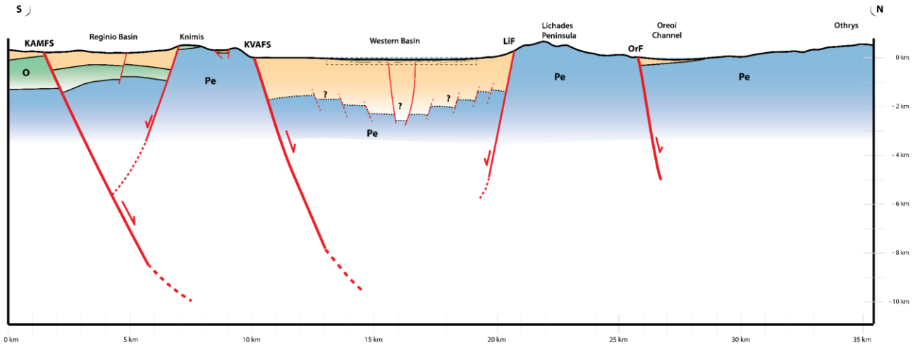
Figure 4.20 : Coupe schématique n°2 orientée S-N à travers le Bassin de Réginio, le Bassin Occidental et le Chenal d'Oreoi, localisée sur la Figure 4.1. Le rectangle en tirets matérialise la position d'un des profils sismiques Air-gun. KAMFS : Kallidromon Atalanti Martino Fault System ; KVAFS : Kamena Vourla Arkitsa Fault System ; LiF : Lichades Fault ; O : Ophiolites ; OrF : Oreoi Fault ; Pe : séries pélagoniennes.
