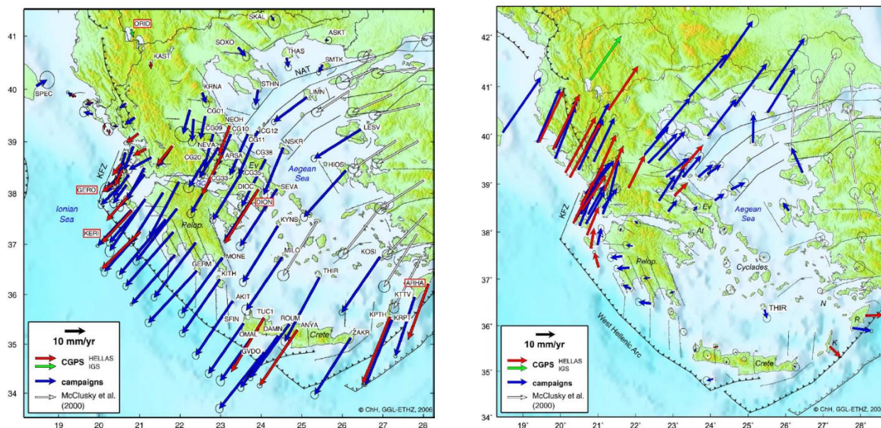
Figure 1.5 : Vitesses GPS enregistrées dans le domaine égéen entre 1993 et 2003 (Hollenstein et al. , 2008). À gauche) Vitesses GPS par rapport à l'Eurasie fixe. À droite) Vitesses GPS par rapport au centre de la Mer Égée fixe.
