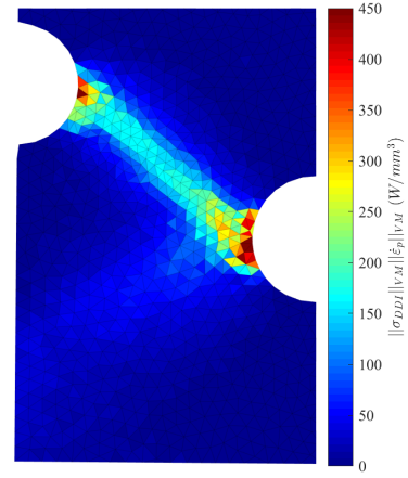
(b) Cartography of \|\sigma_{DDI}\|_{VM} \|\dot{\varepsilon}_p\|_{VM} ,
