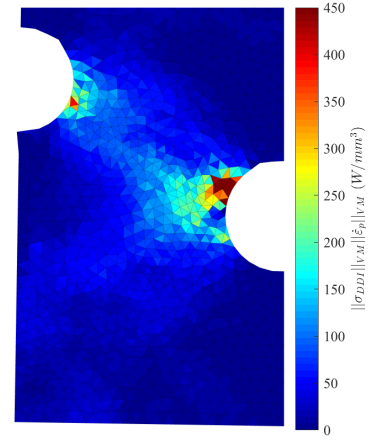
(b) Cartography of \|\sigma DDI\|_{VM} \|\dot{\varepsilon}_p\|_{VM} ,
