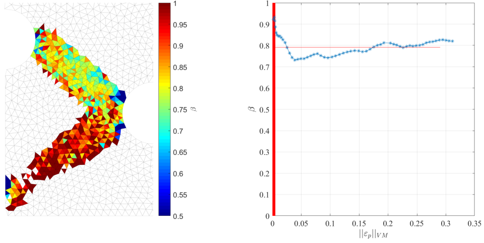
(c) Cartography of \beta at t = 793 \mu s , (d) \beta versus \|\varepsilon_p\|_{VM} ,
