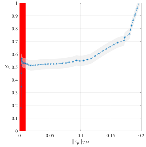
(d) \beta versus \|\varepsilon_p\|_{VM} ,
