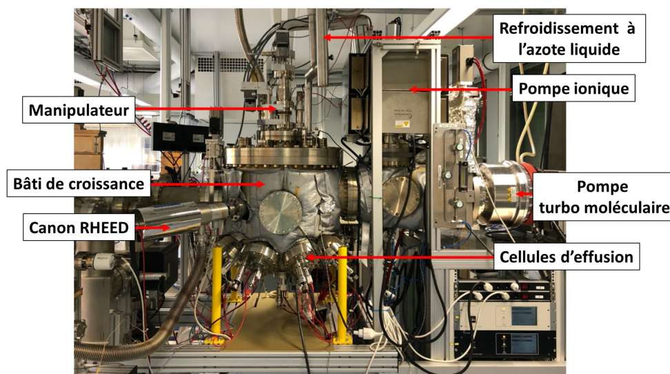
FIGURE I.1 – Bâti de croissance et ses composants.
