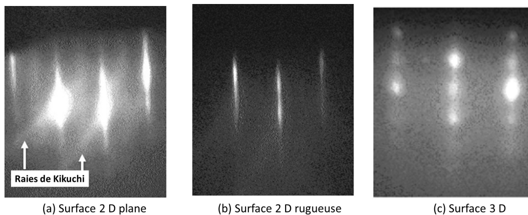
FIGURE I.12 – Cliché de diffraction RHEED. (a) cas d'une surface plane. (b) cas d'une surface 2D rugueuse. (c) Cas d'une surface 3D.
