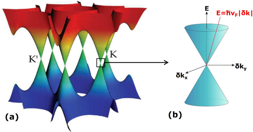
FIGURE II.3 – (a) Représentation graphique en 3 dimensions de la relation structure de bande du graphène idéale . (b) Les deux bandes se rejoignent aux extrémités de la zone de Brouillon [70].
