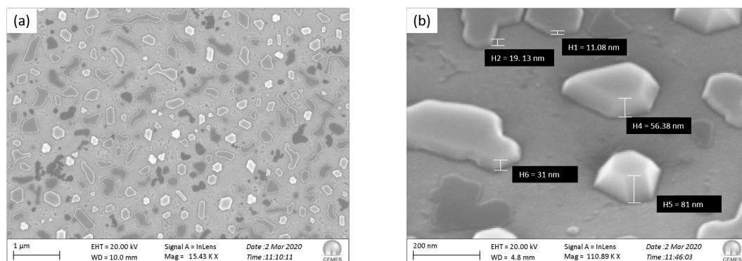
FIGURE IV.13 – (a) Image MEB à grand champ montrant la distributions des îlots sur la surface d'AlN oxydée après 20 nm de dépôt d'au. (b) Zoom sur les îlots d'or et mesure des hauteurs.
