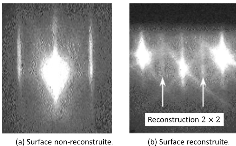
FIGURE I.13 – Cliché de diffraction RHEED. (a) cas d'une surface non reconstruite. (b) cas d'une surface reconstruite 2 \times 2 .
