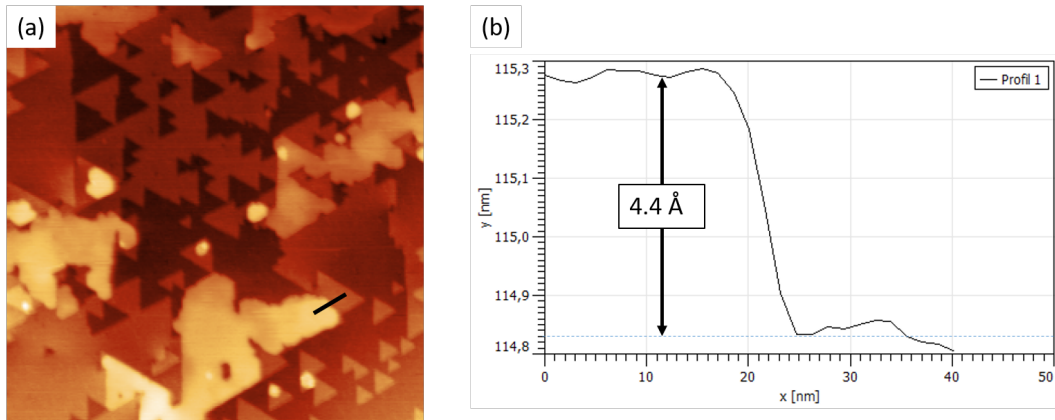
FIGURE IV.10 – (a) : Paramètre de l'image : (400 \times 400\text{ nm}^2) , \Delta f = -30\text{ Hz} , A = 5\text{ nm} , A_{KPFM} = 500\text{ mV} , f_{KPFM} = 937\text{ Hz} .
