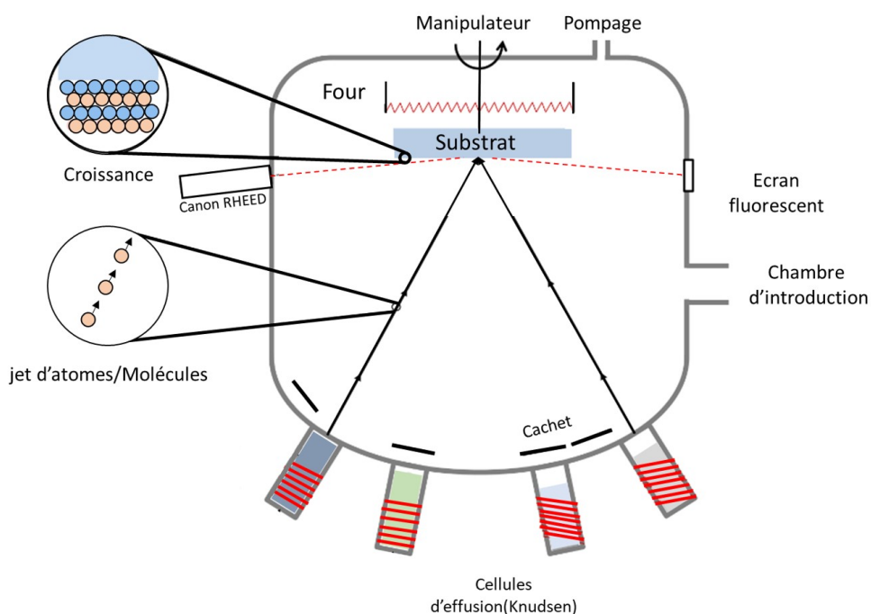
FIGURE I.5 – Représentation schématique d'une chambre MBE typique.
