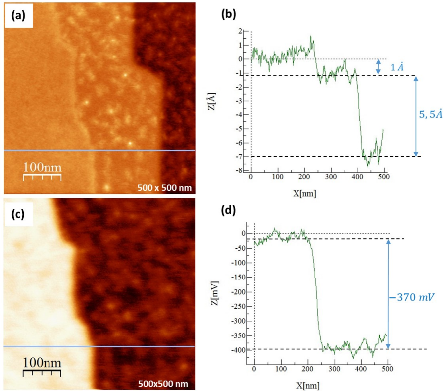
FIGURE II.13 – (a) Image NC-AFM de la surface du graphène épitaxié sur 6H-SiC(0001) sous UHV. (b) Coupe topographique montrant l'existence de trois marches de hauteurs différentes. (c) Image KPFM de la surface du graphène (à gauche) et SiC (à droite). (d) Coupe réalisée sur l'image KPFM.
