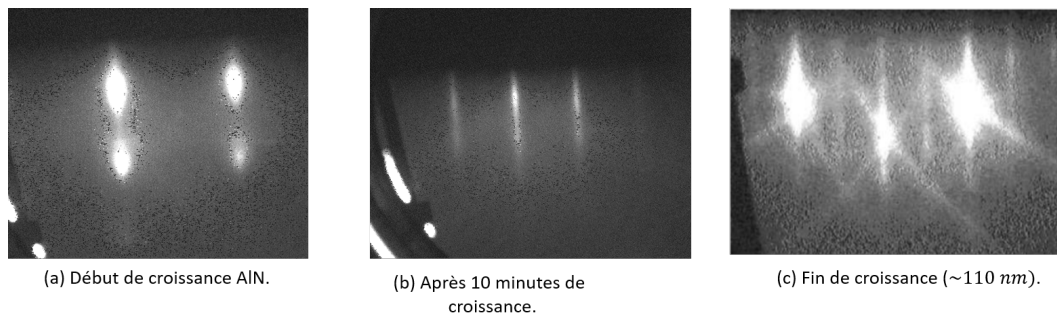
FIGURE IV.6 – (a) Cliché RHEED après quelques secondes de croissance. (b) Après dix minute de croissance, les raies s'affinent (2D) (c) La reconstruction (2 \times 2) apparaît en fin de croissance.
