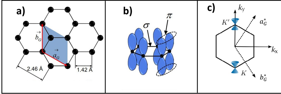
FIGURE II.2 – (a) Structure cristalline du graphène. (b) Représentation des liaisons \sigma et les orbitales \pi . (c) La première zone de Brouillon et les coins de cette zone ( K et K' ).
