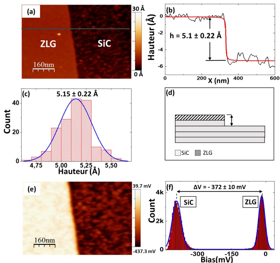
FIGURE II.16 – (a) Image NC-AFM de la surface. (b) Une coupe topographique (noir) et son fit avec la fonction topo(x) (en rouge). (c) Histogramme des hauteurs avec un fit gaussien (en bleu) (d) Représentation schématique de la structure ZLG/6H-SiC. (e) Cartographie KPFM de la surface. (f) Histogramme des potentiels Kelvin.
