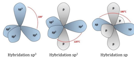
FIGURE II.1 – Les différentes orbitales formées par le carbone. Images issues de [63].
