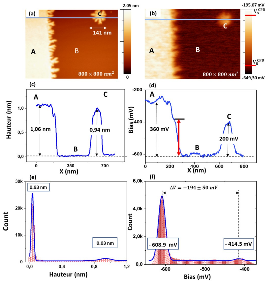
FIGURE III.9 – (a) Image NC-AFM de la surface après le deuxième dépôt de Si. (b) Image KPFM de la surface. (c) Profil topographique correspondant au trait bleu de l'image NC-AFM (d) Coupe correspondant au trait bleu de l'image KPFM. (e) Histogramme des hauteurs avec fit gaussien. (f) Histogramme des potentiels avec fit gaussien. Paramètres de l'image : 800 \times 800 , \Delta f = -20 Hz, A = 5 nm, A_{KPFM} = 500 mV, f_{KPFM} = 957 Hz.
