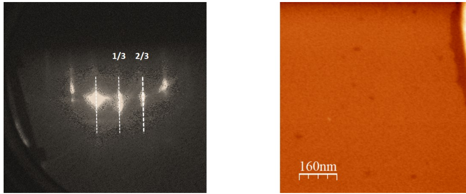
FIGURE IV.5 – (a) Cliché RHEED indiquant la reconstruction (\sqrt{3} \times \sqrt{3})R30^\circ après 6 cycle de dépôt Si à très faible flux et un recuit de 10 minutes après chaque dépôt. (b) Image NC-AFM de la surface après les six de dépôt Si. Paramètres de l'image NC-AFM : Paramètre de l'image : (800 \times 800 nm^2) , \Delta f = -5 Hz , A = 5 nm , A_{KPFM} = 500 mV , f_{KPFM} = 937 Hz .
