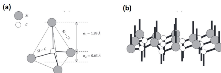
FIGURE II.7 – (a) Représentation de la géométrie du tétraèdre formé par l'atome C et trois atomes de Si. (b) Représentation graphique du bicouche SiC.
