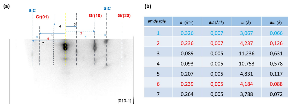
FIGURE II.14 – (a) Image RHEED de la surface élaborée par sublimation Si dans la direction [010\bar{1}] . (b) Analyse des raies et détermination des paramètres de maille du graphène.
