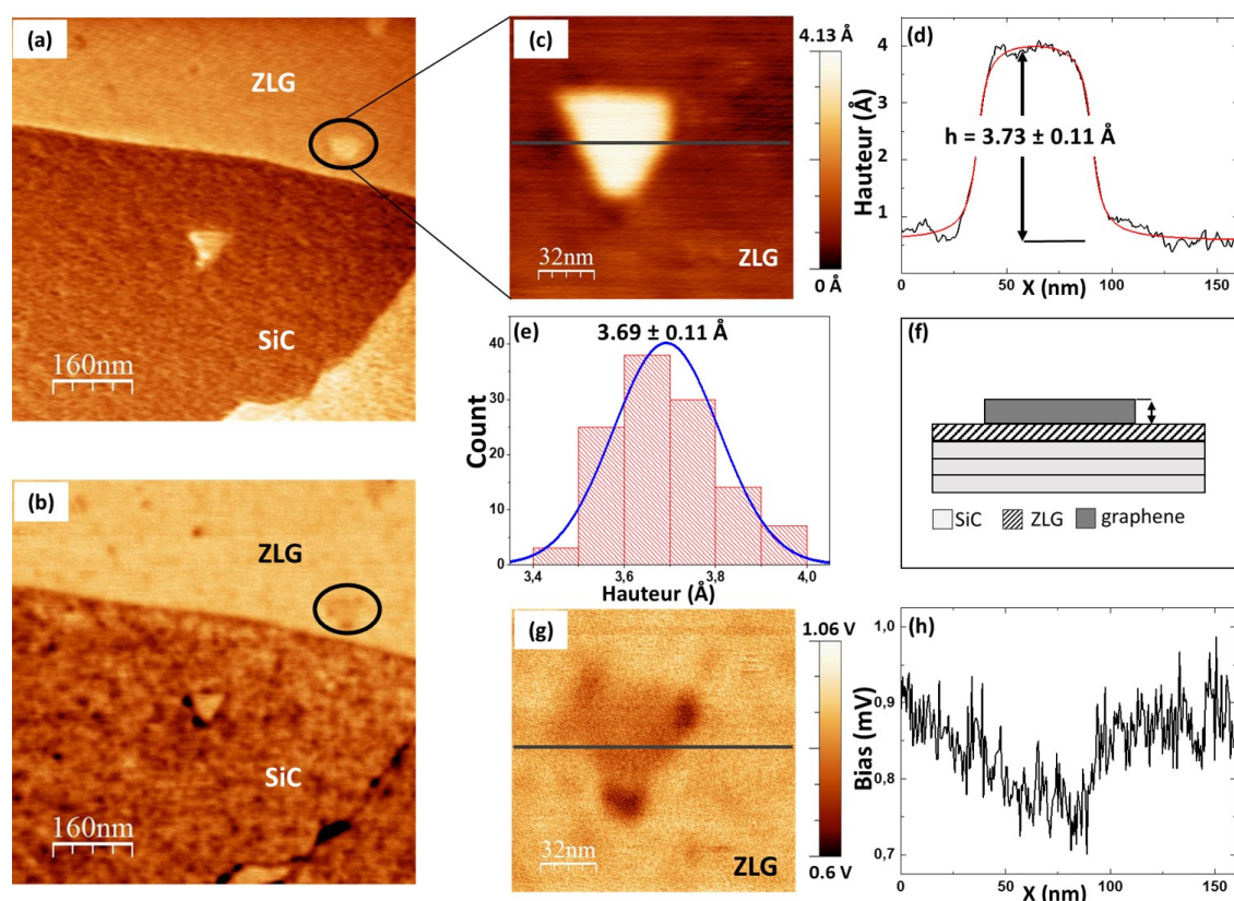
FIGURE II.20 – (a) Image NC-AFM ( 600 \times 600 \text{ nm}^2 ) de la surface de l'échantillon.(b) Image KPFM de la surface à grand champ. (c) Image NC-AFM de l'îlot( 150 \times 150 \text{ nm}^2 ). (d) Coupe topographique de l'îlot (noir) et son fit avec la fonction \text{topo}(x) (rouge). (e) Histogramme des hauteurs réalisées sur l'îlot. (f) Représentation schématique de la structure identifiée. (g) Image KPFM de l'îlot ( 150 \times 150 \text{ nm}^2 ). (h) Coupe KPFM sur l'îlot.
