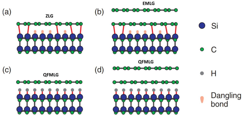
FIGURE II.9 – Représentation en coupe de (a) la ZLG et (b) l'EMLG. Après l'intercalation hydrogène (c) et (d) la ZLG est découplée du substrat et donne naissance à une nouvelle structure "QFMLG". D'après Riedl et al [93].
