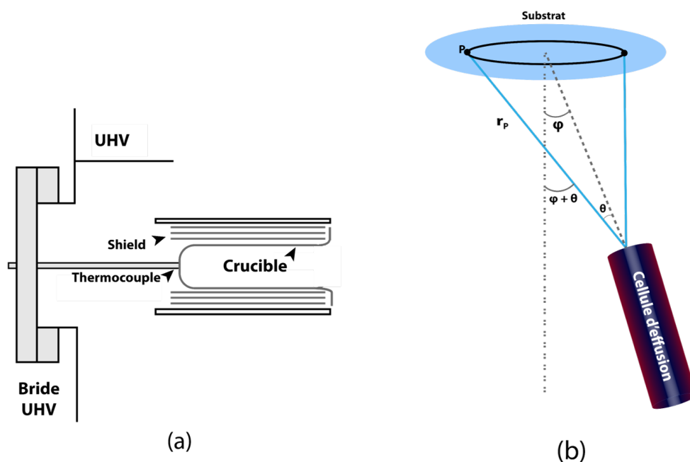
FIGURE I.6 – a) Schéma typique d'une cellule Knudsen. (b) Schéma de la dépendance du flux en fonction du substrat.
