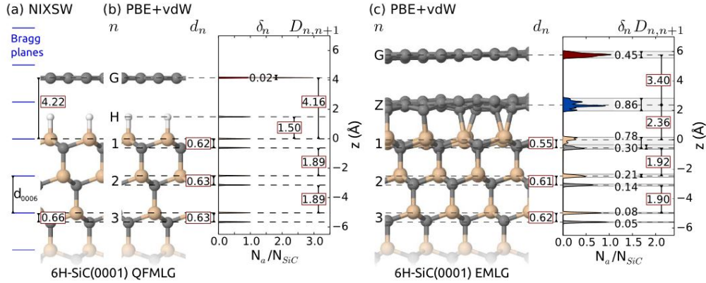
FIGURE II.10 – (a) Les hauteurs d’adsorption mesurées par NIXSW sur la couche QFMLG. Calculs DFT (PBE+vdW) pour (b) la structure QFMLG et pour (c) la structure EMLG sur 6H-SiC(0001). Issue de [94].
