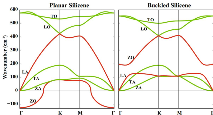
FIGURE III.2 – Phonons du silicène planaire et alterné. Les modes acoustiques et optiques hors plan, transversaux et longitudinaux sont désignés par ZA, TA, LA, ZO, TO et LO, respectivement. Les modes LA et ZO changent de manière significative lors de la transformation structurale. Ces modes sont représentés par des lignes rouges pour attirer l'attention sur ce changement. D'après [107]
