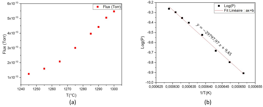
FIGURE I.7 – a) Exemple de calibration de la cellule de Si. (b) Fit linéaire de la courbe \text{Log}(P) en fonction de l'inverse de la température absolue.
