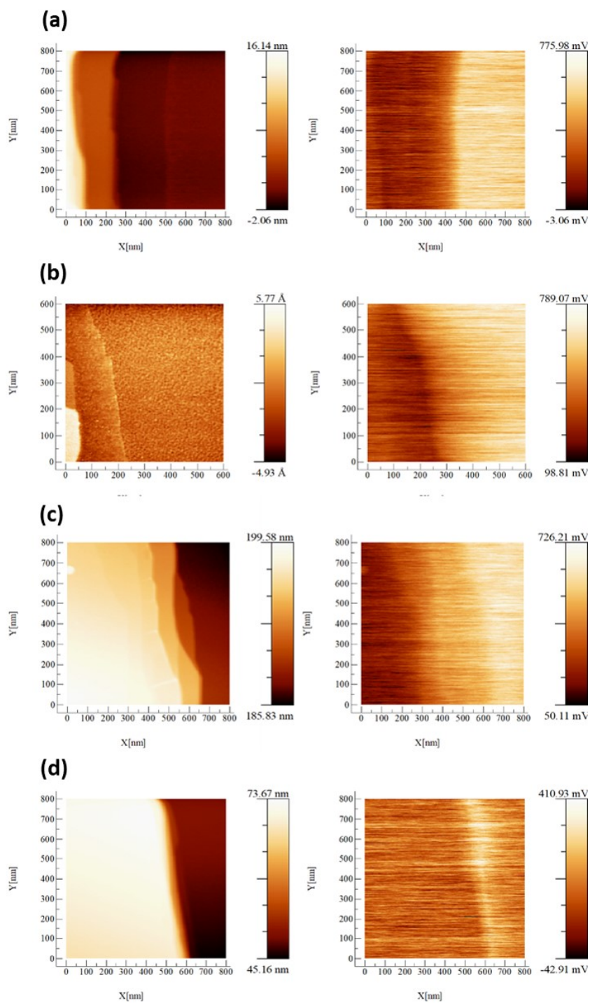
FIGURE III.7 – (a) (b) (c) (d) Images NC-AFM et KPFM des différentes régions de la surface. Paramètres de l'image : 800 \times 800 , \Delta f = -20 Hz, A = 5 nm, A_{KPFM} = 500 mV, f_{KPFM} = 957 Hz.
