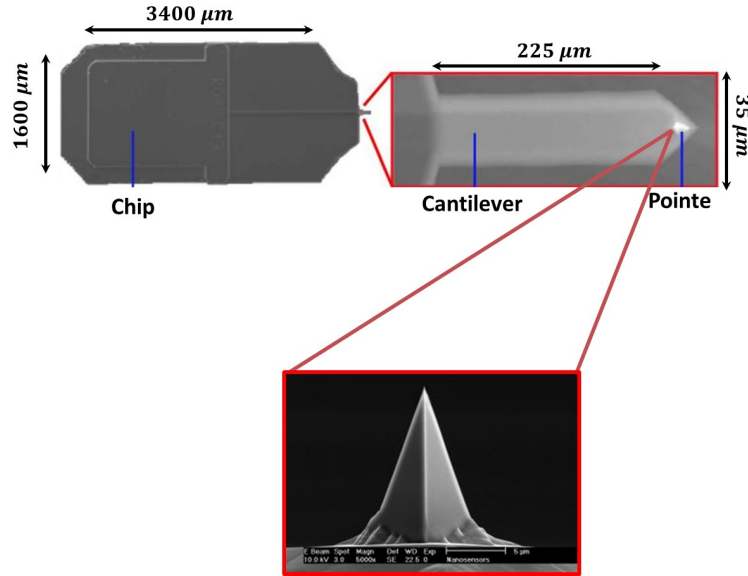
FIGURE I.15 – Image MEB et dimensions du constructeur [43] de l'ensemble : Chip, cantilever et pointe.
