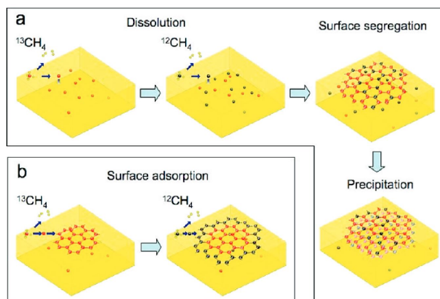
FIGURE II.5 – Schéma représentatif du mécanisme surfacique lors d'une synthèse CVD sur un substrat de cuivre. D'après Li et al. [84].
