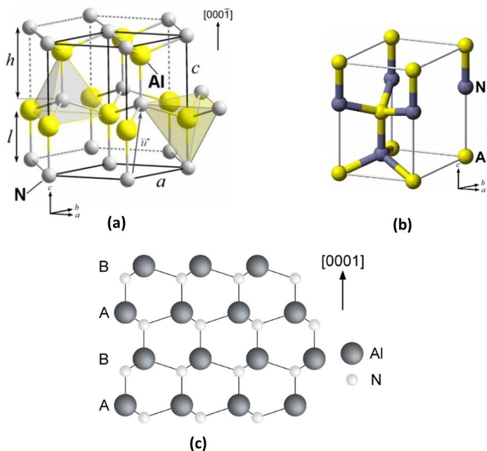
FIGURE IV.1 – (a) La phase wurtzite du nitrure d'aluminium indiquent les sites tétraédriques formés par les atomes d'Al et N. (b) La cellule élémentaire de la phase hexagonale. (c) Vue en coupe de l'alternance des plans ABAB selon la direction [0001] . Image issue de [56].
