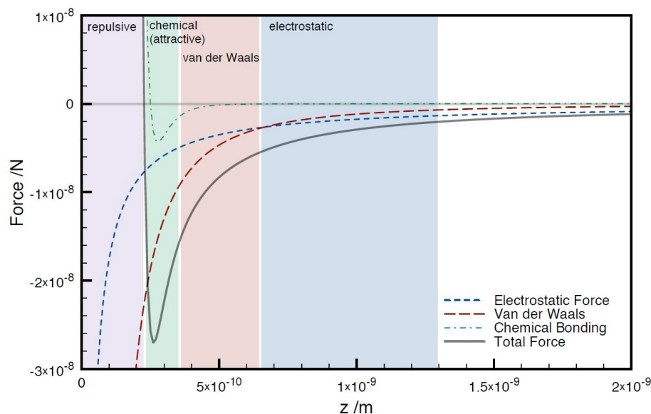
FIGURE I.16 – Les forces de surface qui s'exercent sur la sonde en fonction de la distance. Image issue de [46]
