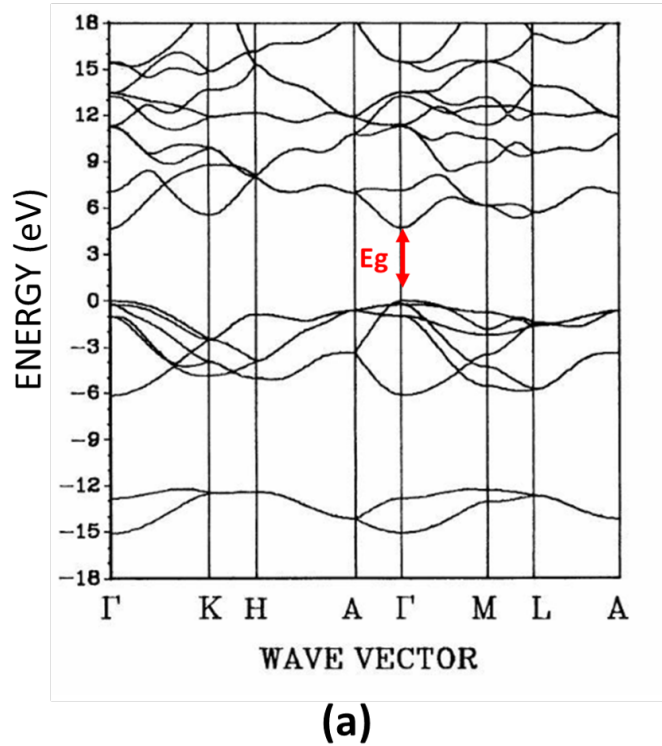
FIGURE IV.2 – (a) Diagramme de bandes de l'AlN. Issue de [155].
