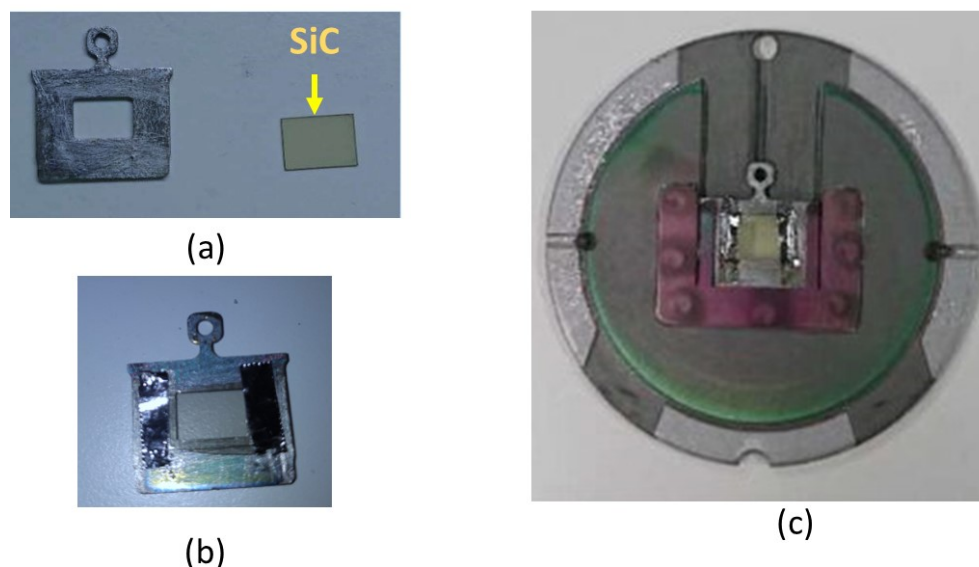
FIGURE IV.4 – (a) Substrat SiC et son porte échantillons. (b) Fixation de l’échantillon sur le support Omicron à l’aide d’une soudure par point. (c) Fixation du support Omicron sur le disque porte-échantillon.
