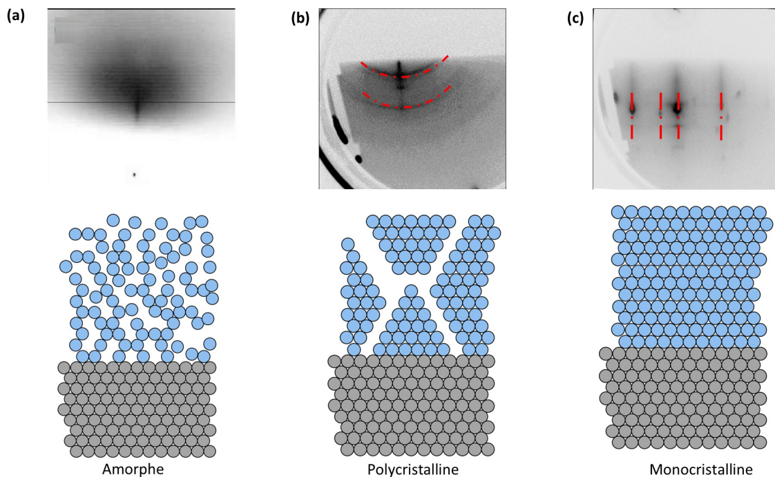
FIGURE I.11 – Images RHEED pour des surfaces de différentes cristallinités : (a) Amorphe. (b) Polycristalline. (c) Monocristalline.
