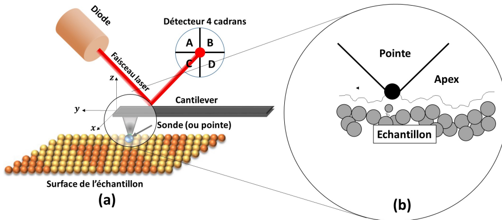
FIGURE I.14 – (a) Illustration du Principe de la microscopie à force atomique. (b) Schéma illustratrice de l'apex proche de la surface.
