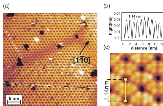
FIGURE III.4 – (a) Image STM à grande échelle de la structure (4 \times 4) de silicène sur Ag(111). (b) Coupe topographique correspondant aux pointillés de l'image STM. (c) Image haute résolution (3 \times 3) de la reconstruction (4 \times 4) . D'après [123].
