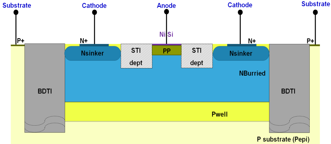
Figure 48 : Vue en coupe du frontend des diodes de bruit (Schottky) nouvelle génération
