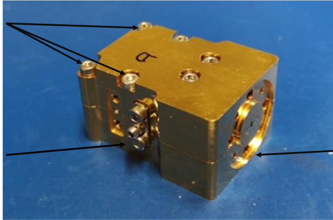
Figure 133 : Photographie d'un des deux split blocks . La dénomination utilisée est SBA et SBD pour split block A et split block D.
