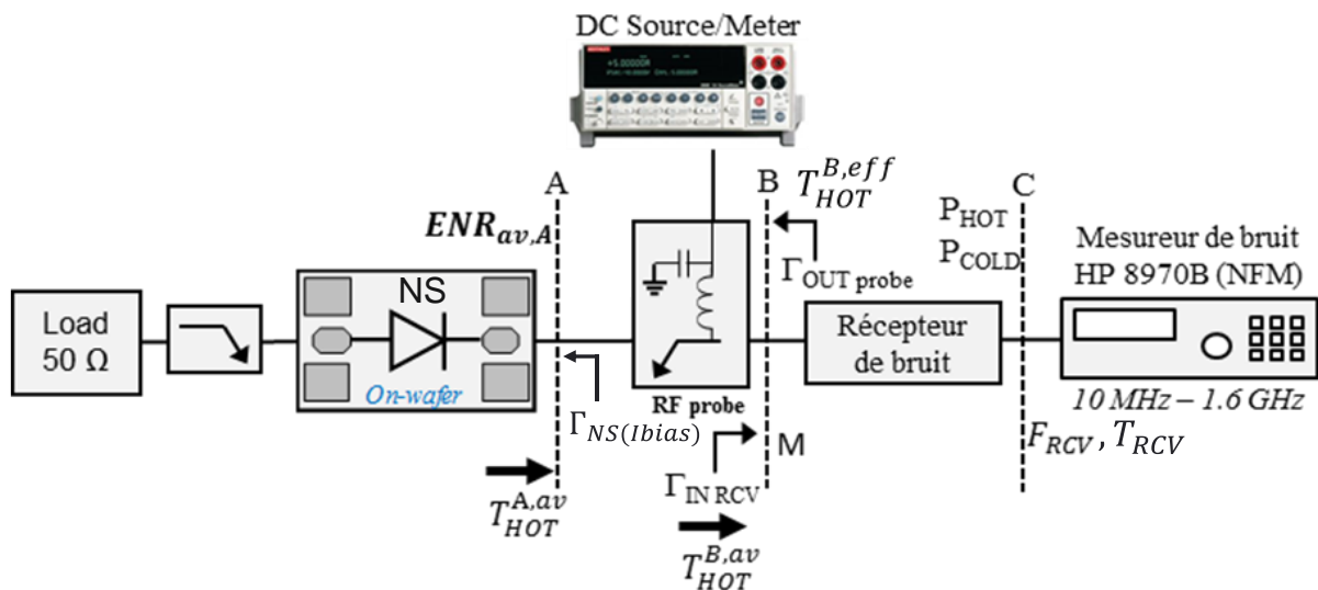
Figure 68 : Schéma bloc du banc de test utilisé à l'EMN pour la mesure en puissance de bruit des diodes en configuration série. Un premier récepteur de bruit couvre la bande 140-170 GHz, un deuxième la bande 170-220 GHz. Pour émuler une mesure en 1 port, une source de bruit ELVA a été reliée à la sonde de gauche. Son isolateur garantit la présentation d'une impédance très proche de 50 Ω.
