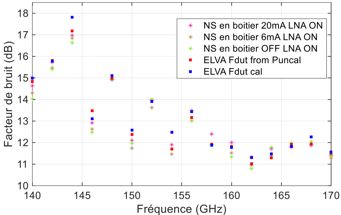
Figure 166 : F_{DST} {WR5+iso+WR5+ampli+WR5} extraits avec la NS en boîtier et la source ELVA en puissance non calibrée, comparaison avec la mesure du NF faite avec la source ELVA. La méthode utilisée ici fait intervenir F_{tot} .
