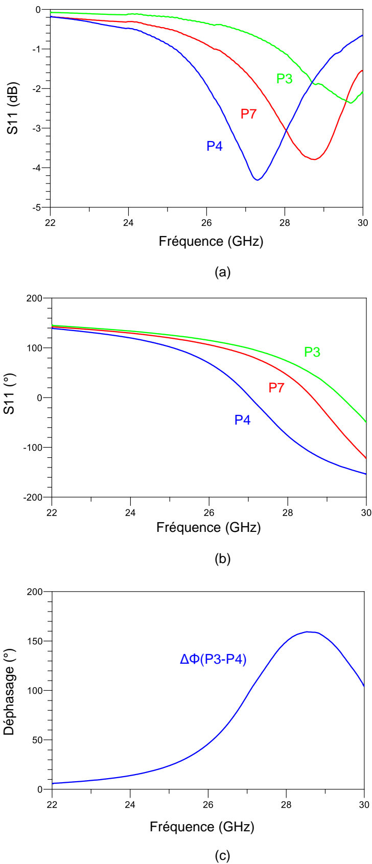
Figure IV-28 : Résultats de mesures pour, (a) les puces 3, 4 et 7 en module, (b) en phase, (c) et le déphasage obtenu entre les puces 3 et 4.
