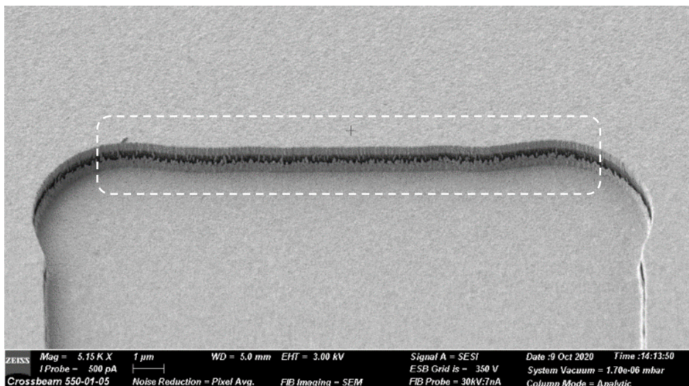
Figure II-14 : Image MEB des reprises de contact entre les deux couches d'au formant la membrane.
